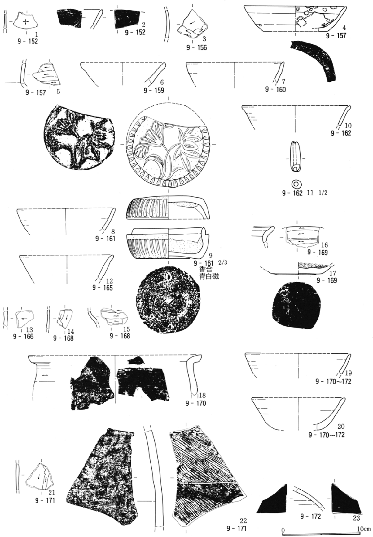
第647图 9区土坑出土遗物实测图(8)
