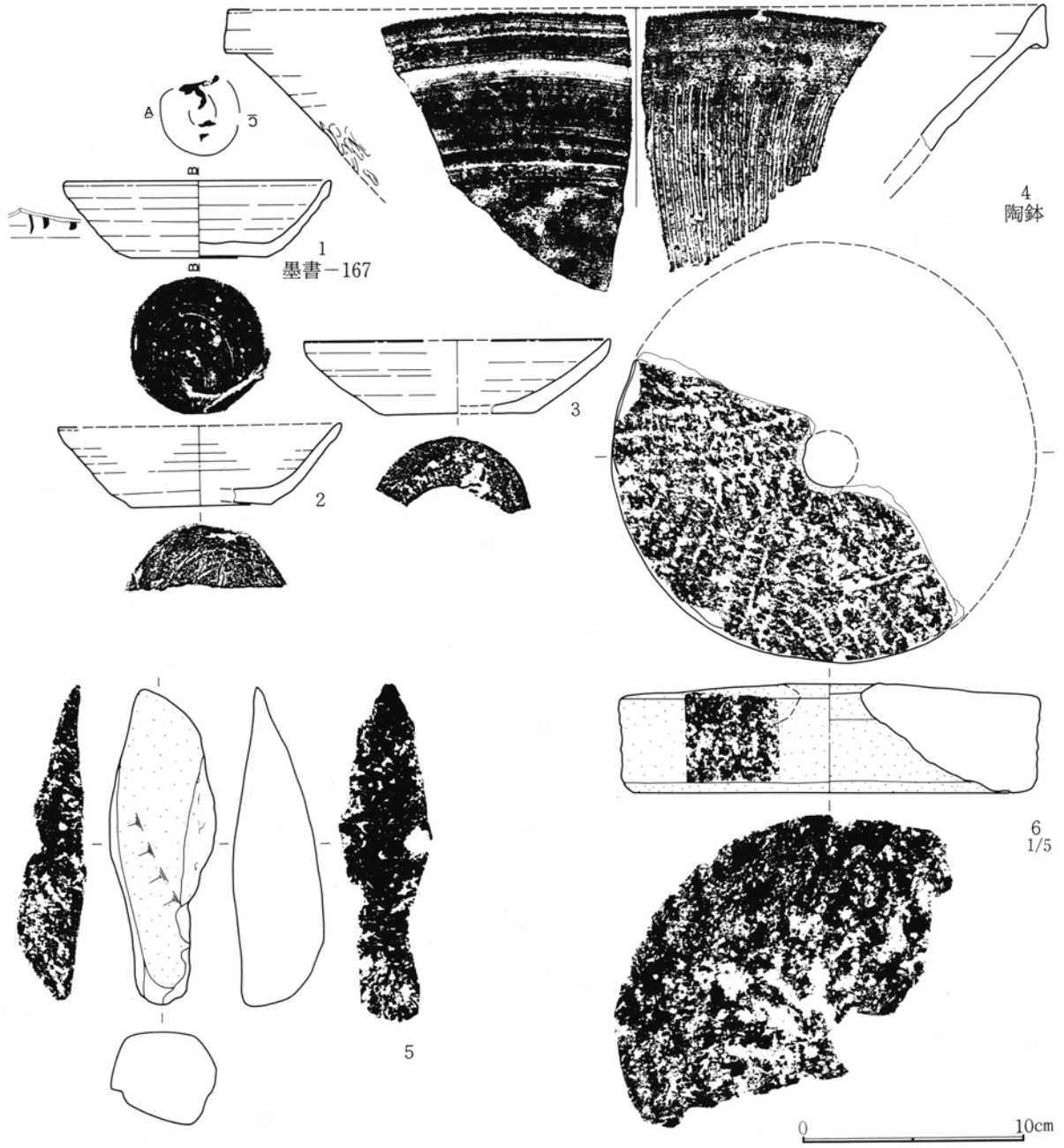
第737图 7区遺構外出土遺物実測図
