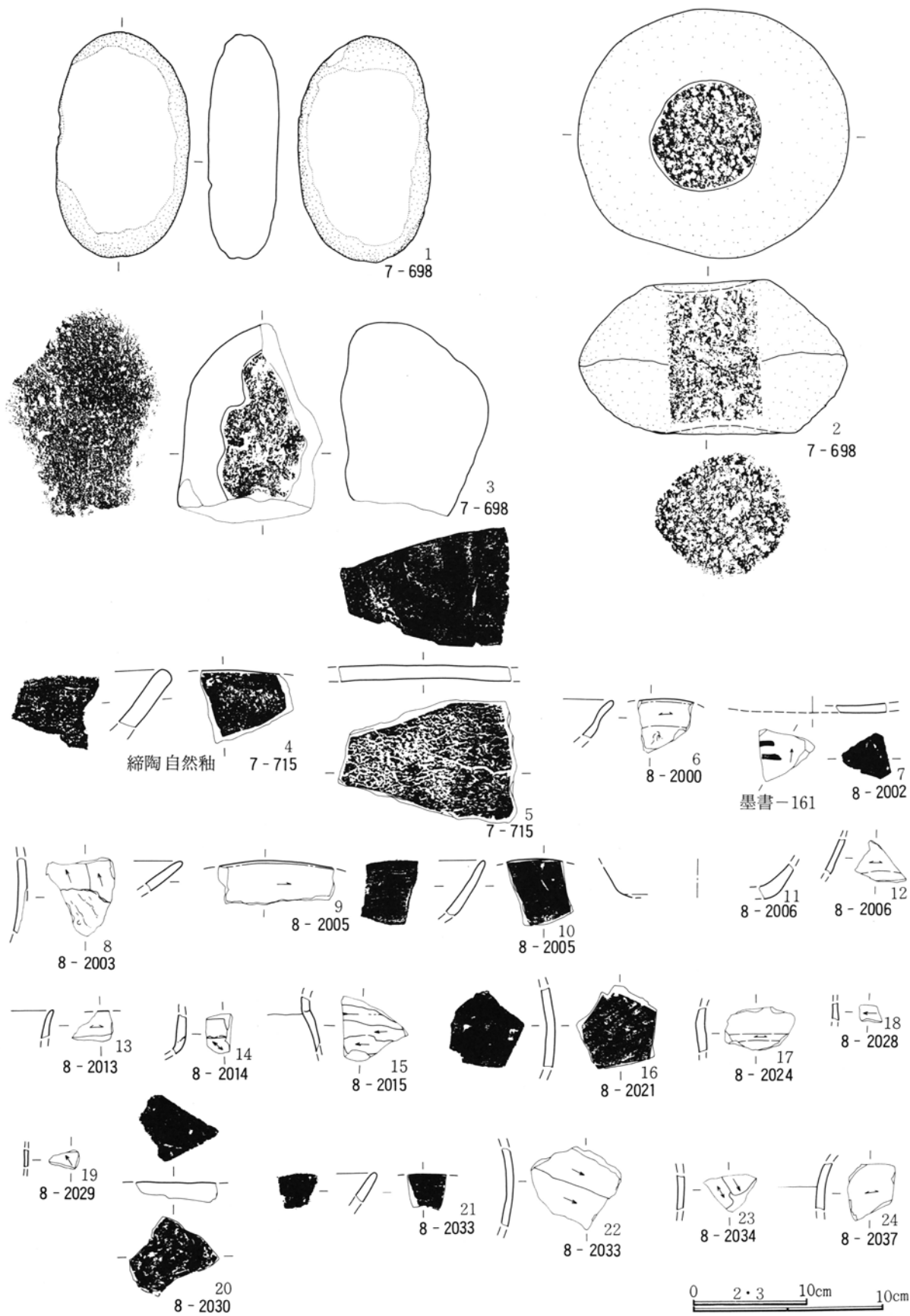
第674図 7区ピット出土遺物実測図(4)・8区ピット出土遺物実測図(1)
