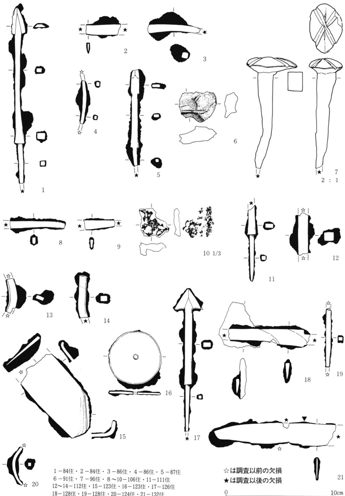
第687図 出土金属器実測図(4)
