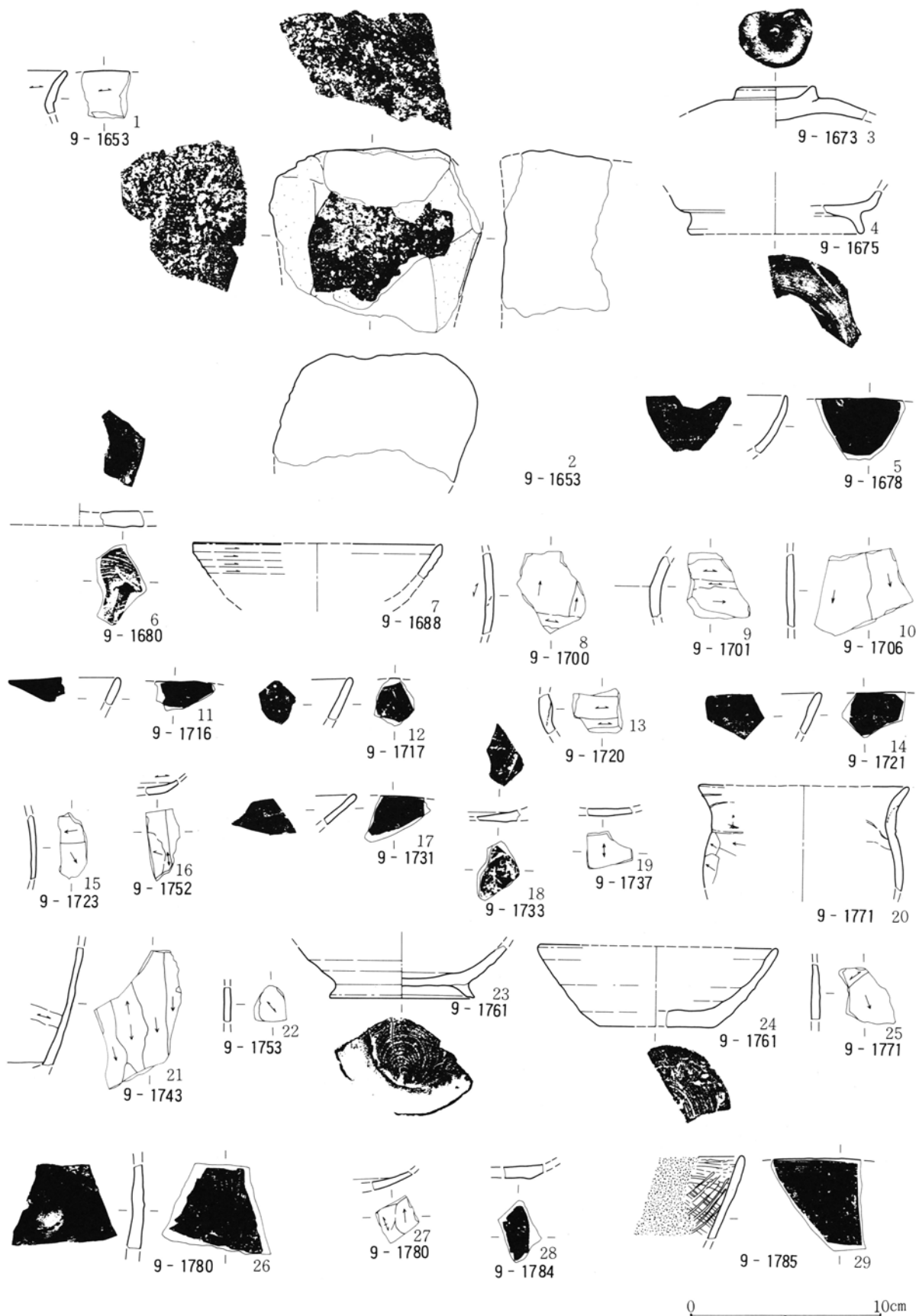
第680図 9区ピット出土遺物実測図(6)
