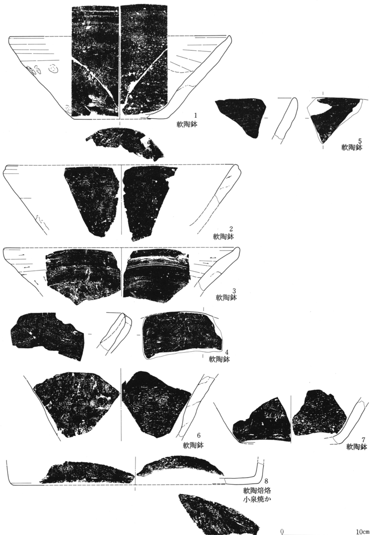
第547図 6区第17号井戸跡出土遺物実測図
