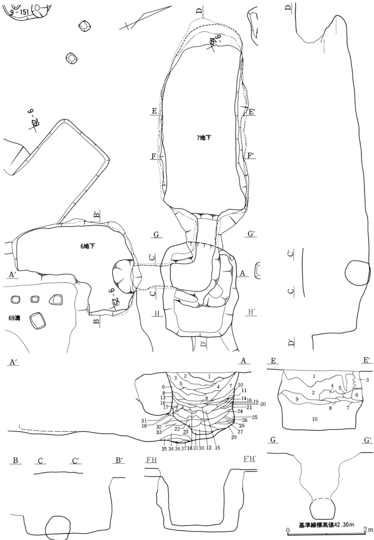
第478図 第6・7号地下式土坑実測図
