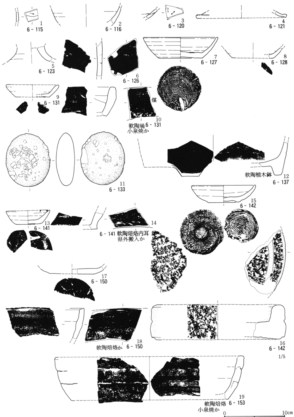
第629図 6区土坑出土遺物実測図(6)
