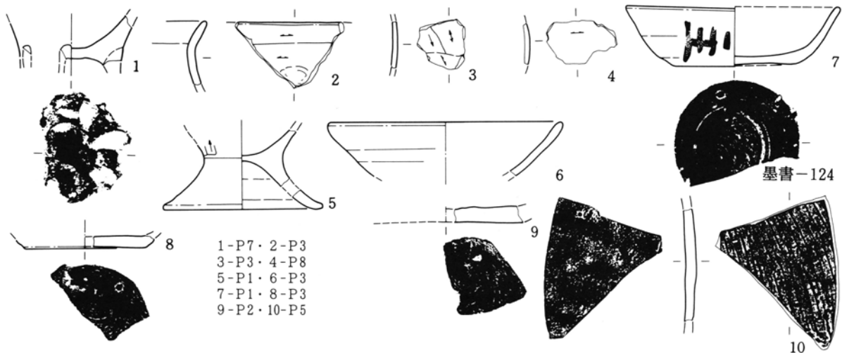
第444図 第14号掘立柱建物跡出土遺物実測図
