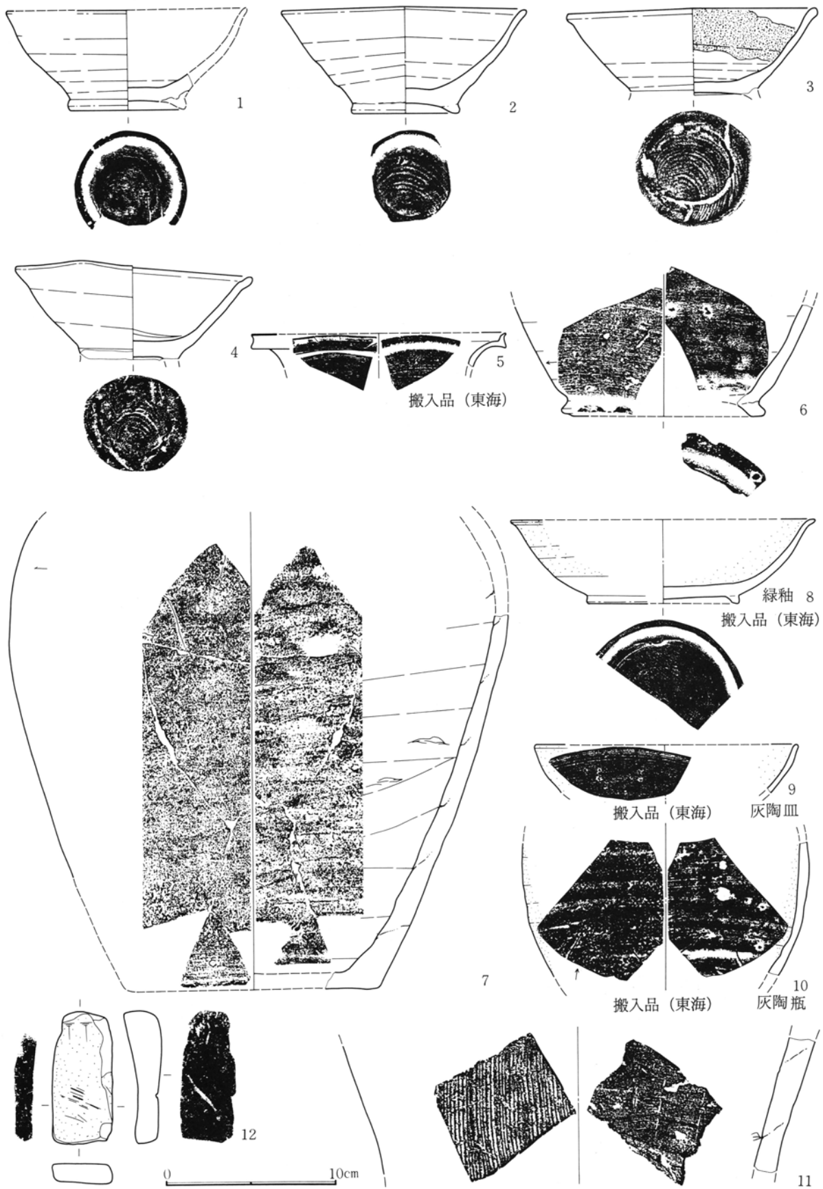
第353図 第162号住居跡出土遺物実測図(2)
