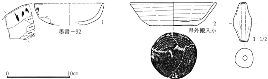
第337図 第180号住居跡出土遺物実測図
