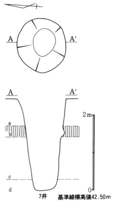
第539图 6区第7号井戸跡実測図
