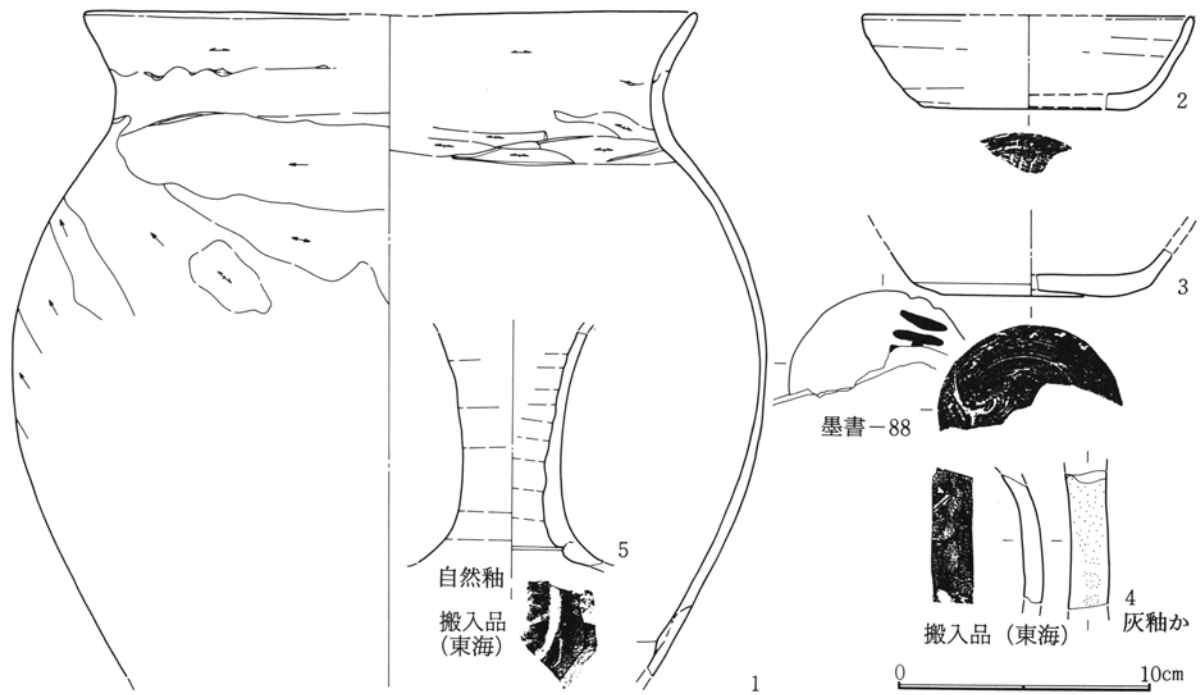
第318図 第146号住居跡出土遺物実測図(3)
