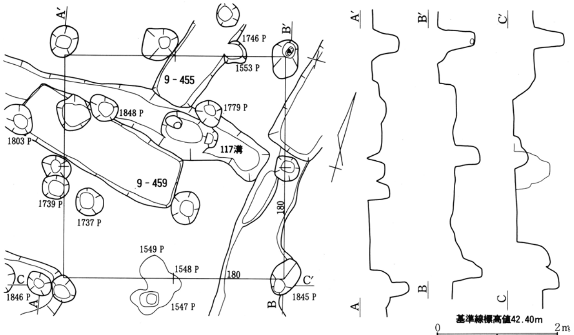
第421図 第20号掘立柱建物跡実測図
