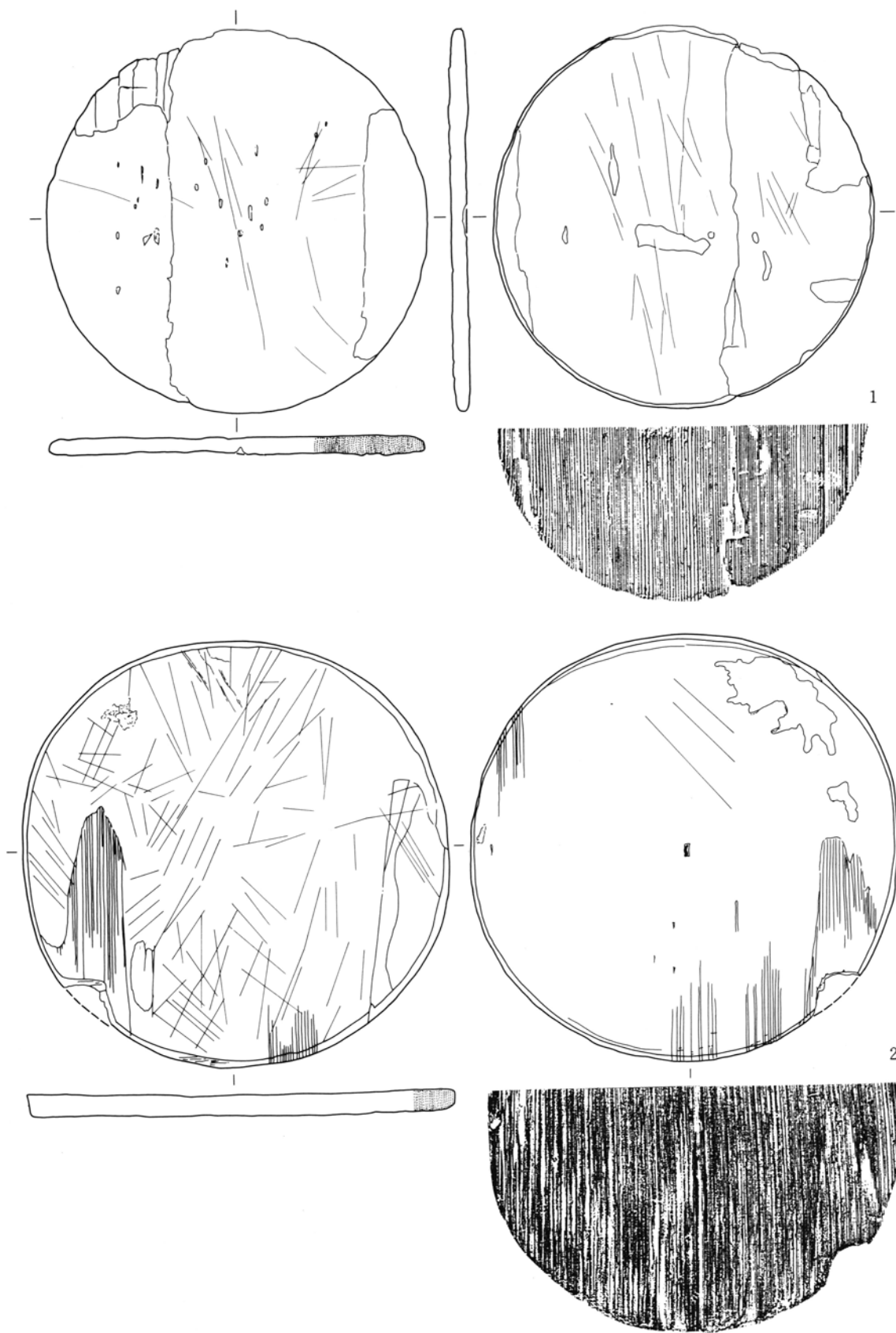
第509图 6区第1号井戸跡出土遺物実測図(4)
