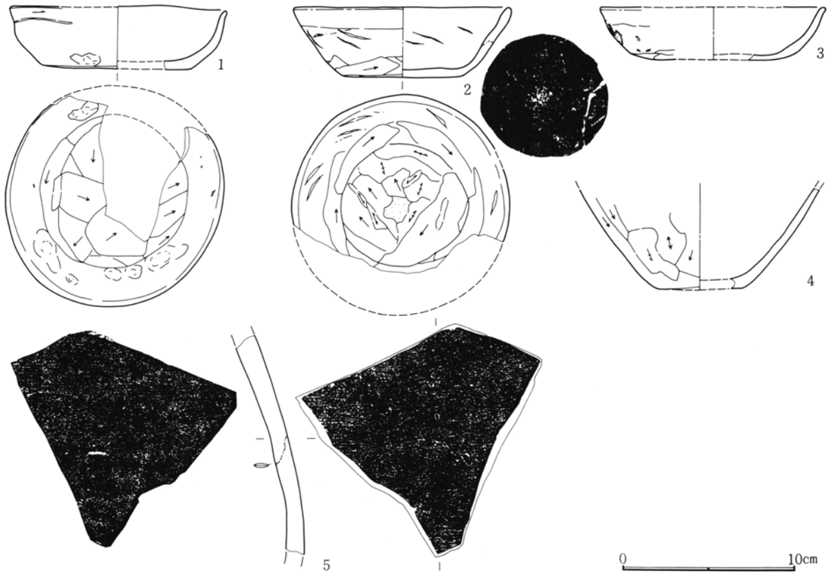
第354図 第163号住居跡出土遺物実測図
