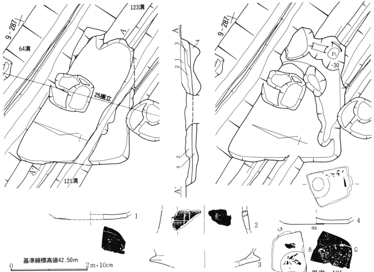
第368図 第175号住居跡・出土遺物実測図
