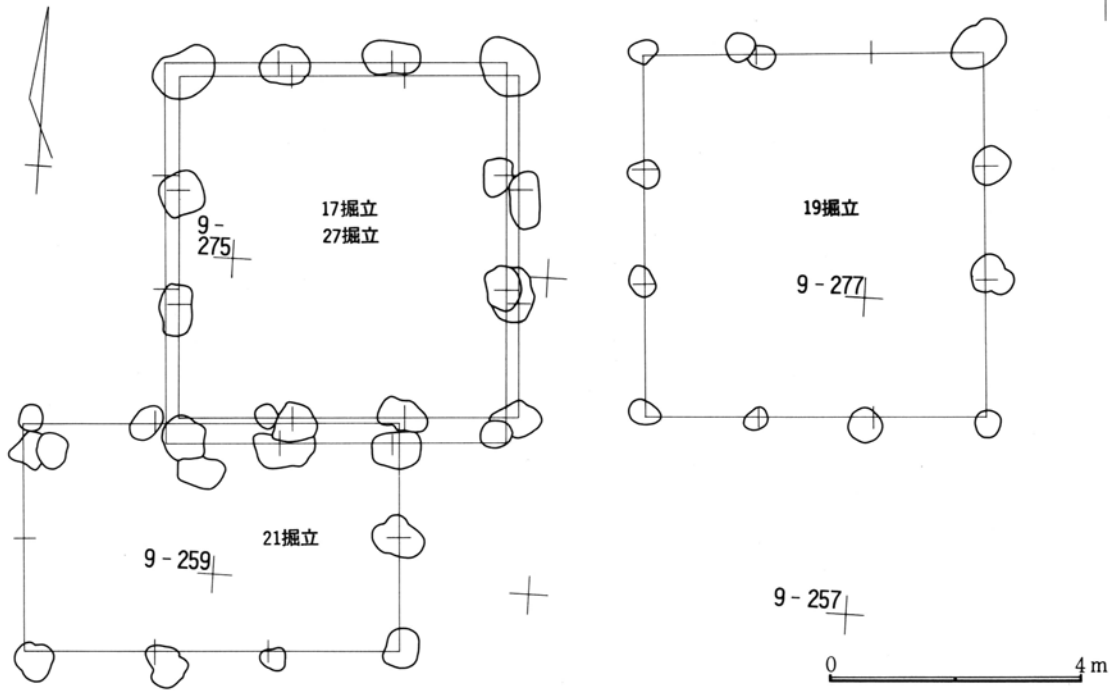
第420図 第17・27・19・21号掘立柱建物跡配置図 (1:120)
