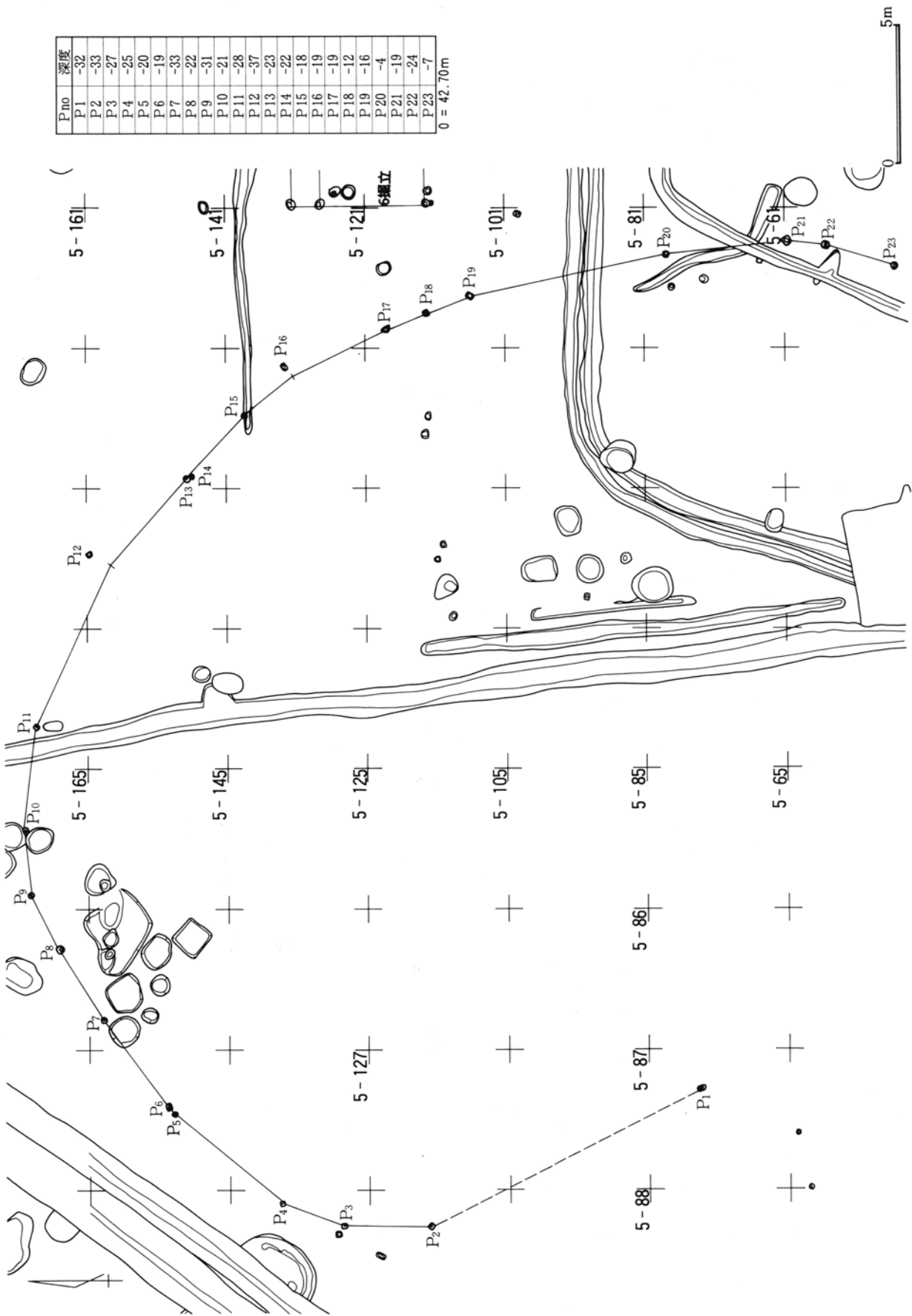
第435図 第3号柵状遺構実測図
