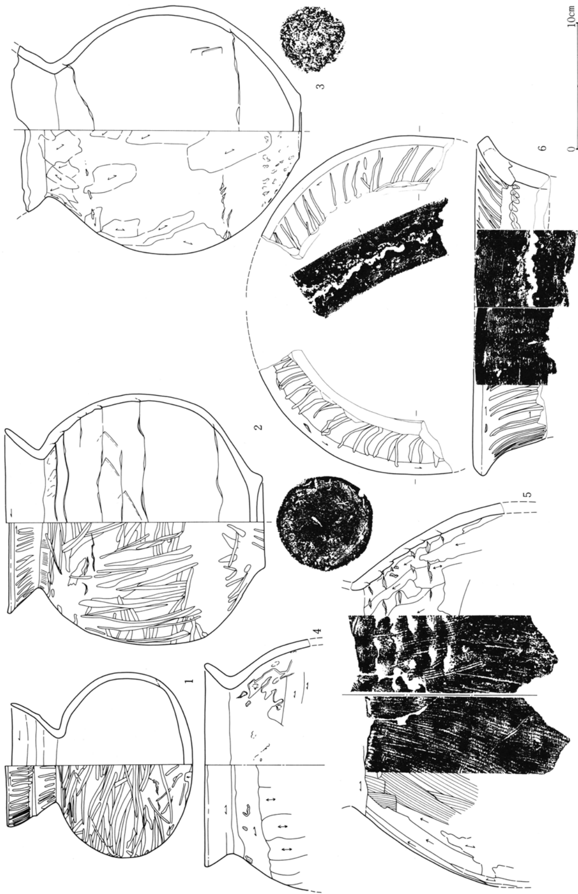
第560图 9区第9号井跡出土遺物実測図(2)
