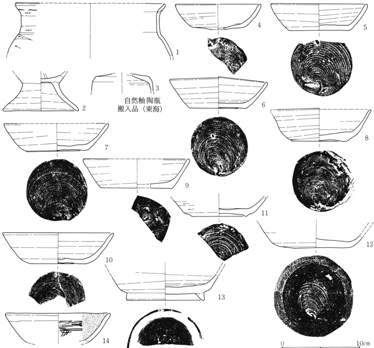
第335図 第179号住居跡出土遺物実測図(1)
