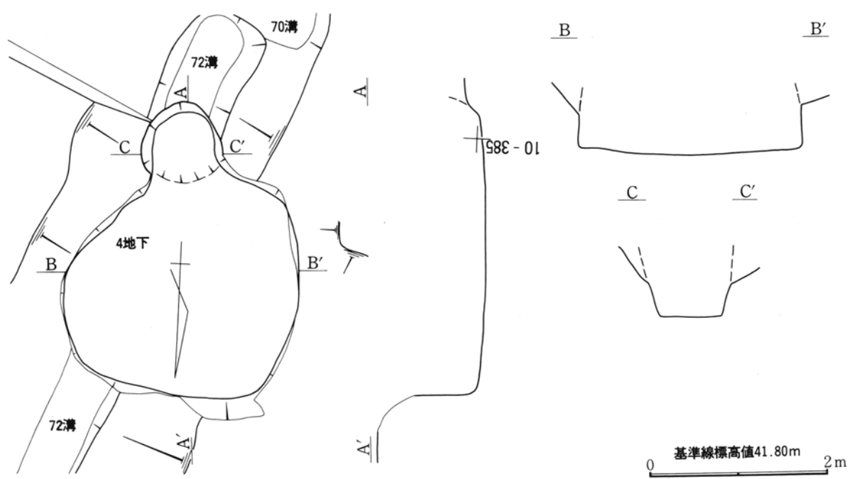
第476図 第4号地下式土坑実測図
