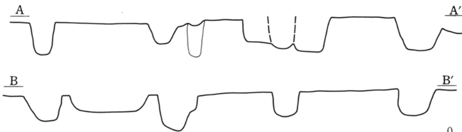
第419図 第21号掘立柱建物跡実測図
