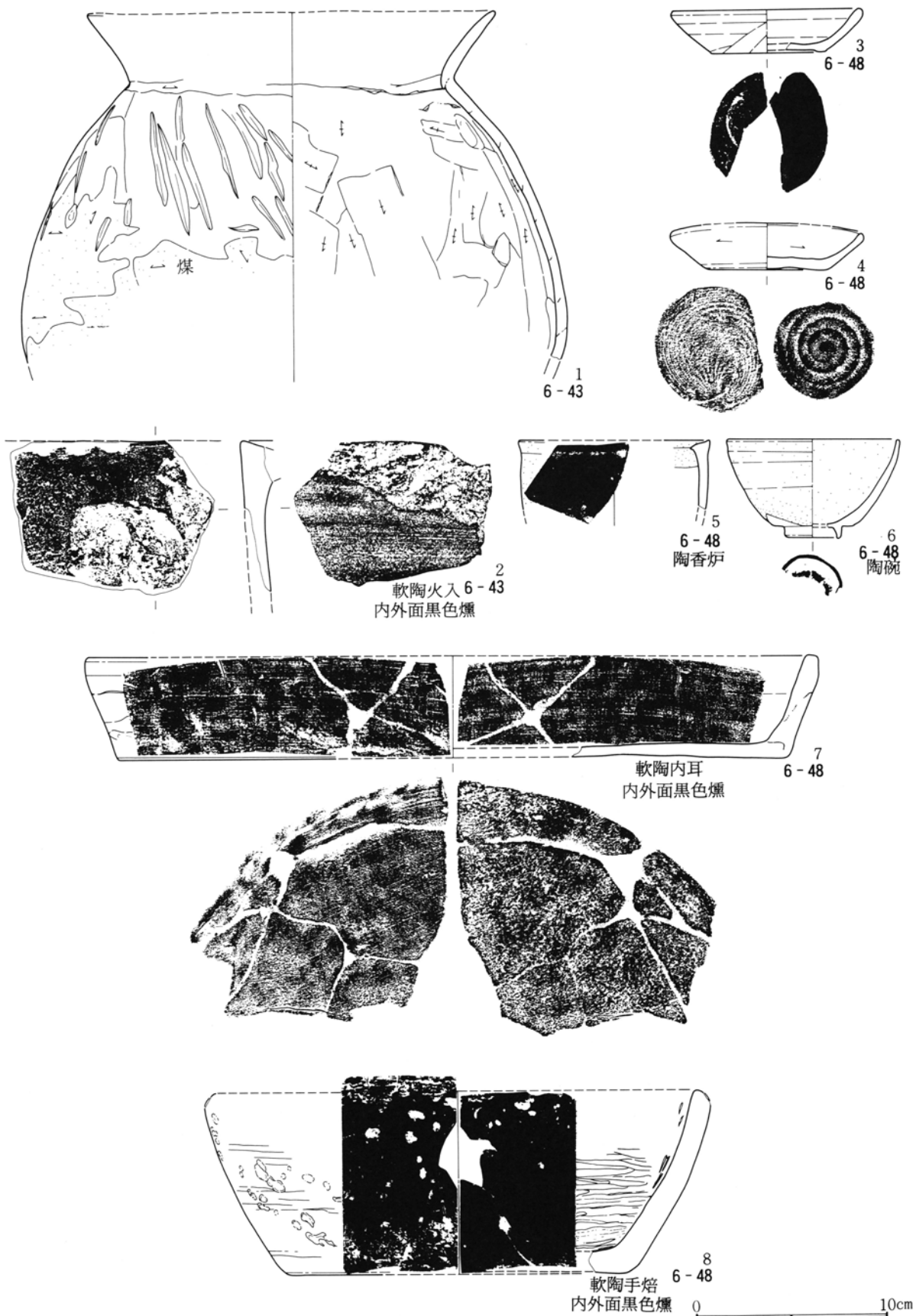
第626图 6区土坑出土遺物実測図(3)
