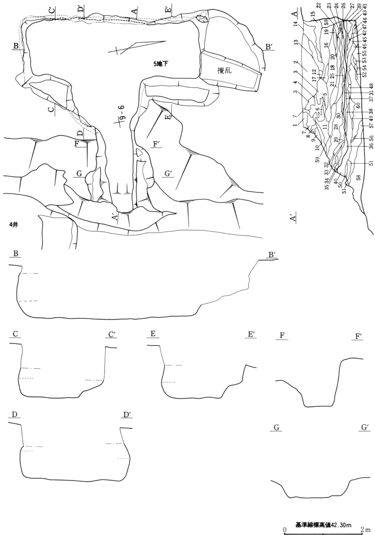
第477图 第5号地下式土坑实测图
