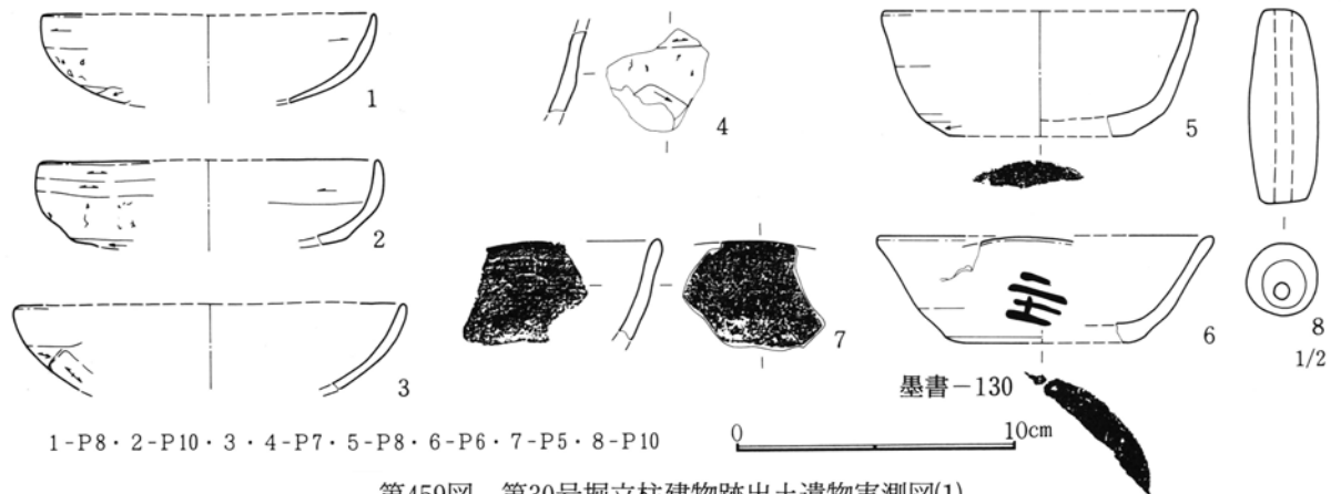
第459图 第30号掘立柱建物跡出土遺物実測図(1)
