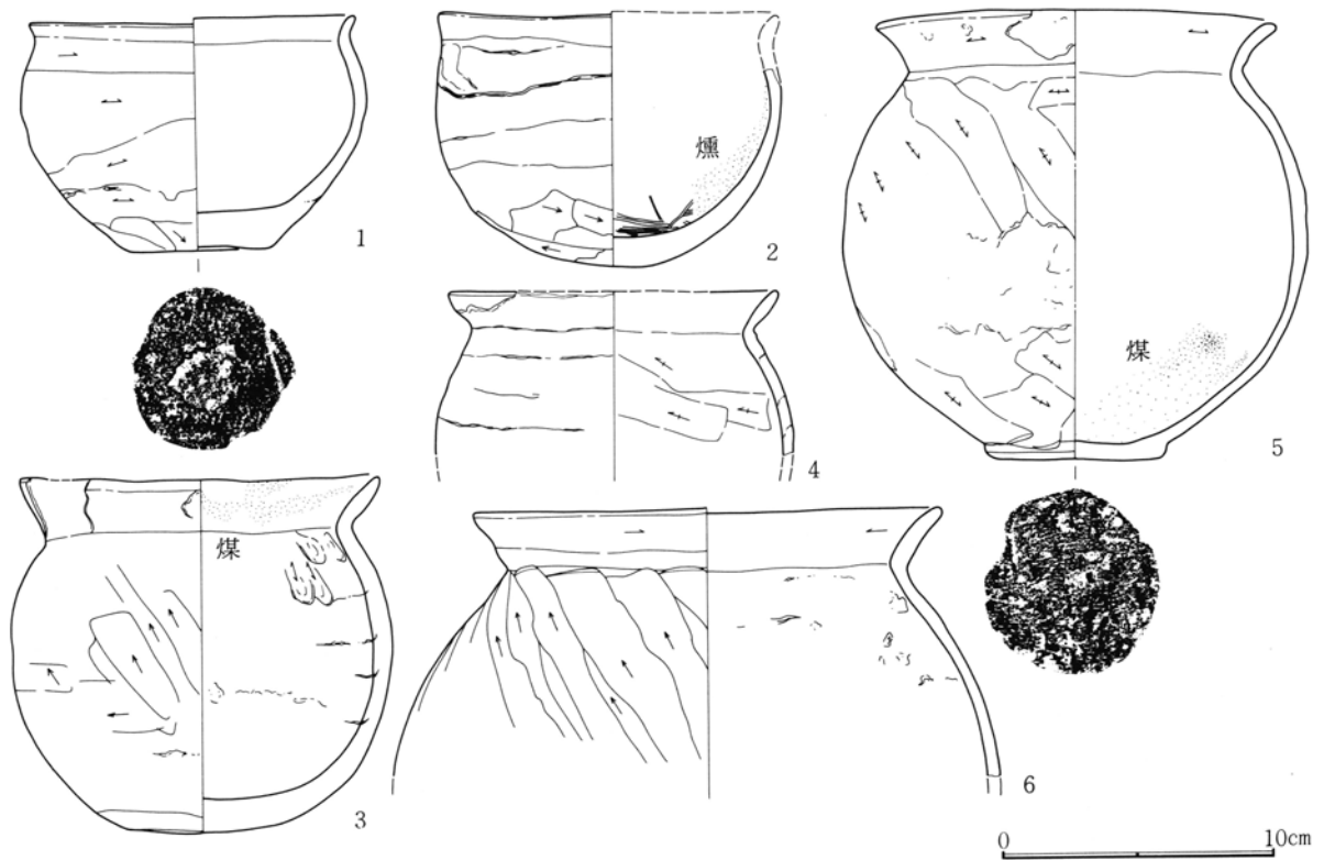
第369図 第176号住居跡出土遺物実測図(1)
