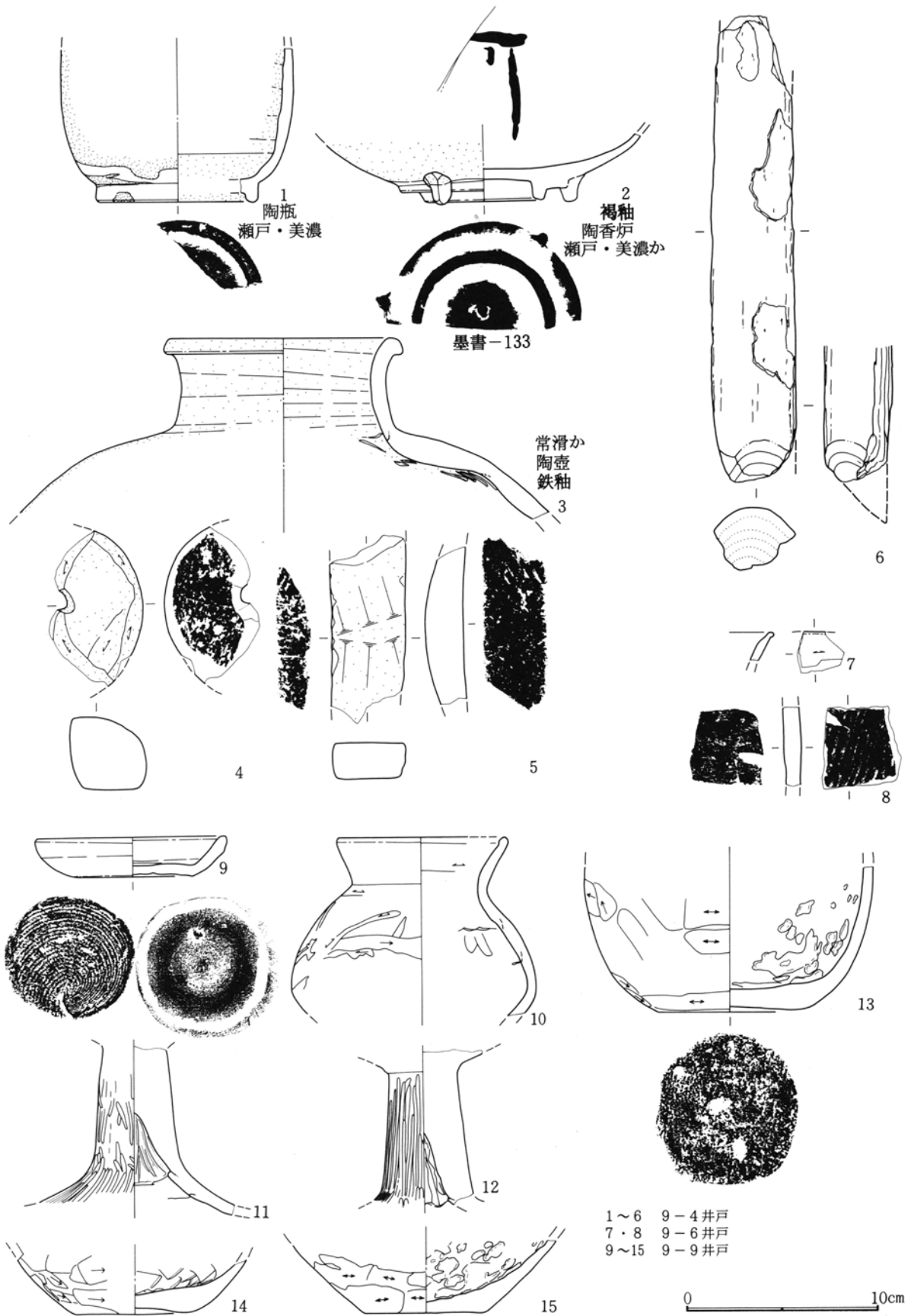
第559図 9区第4・6・9号井戸跡出土遺物実測図
