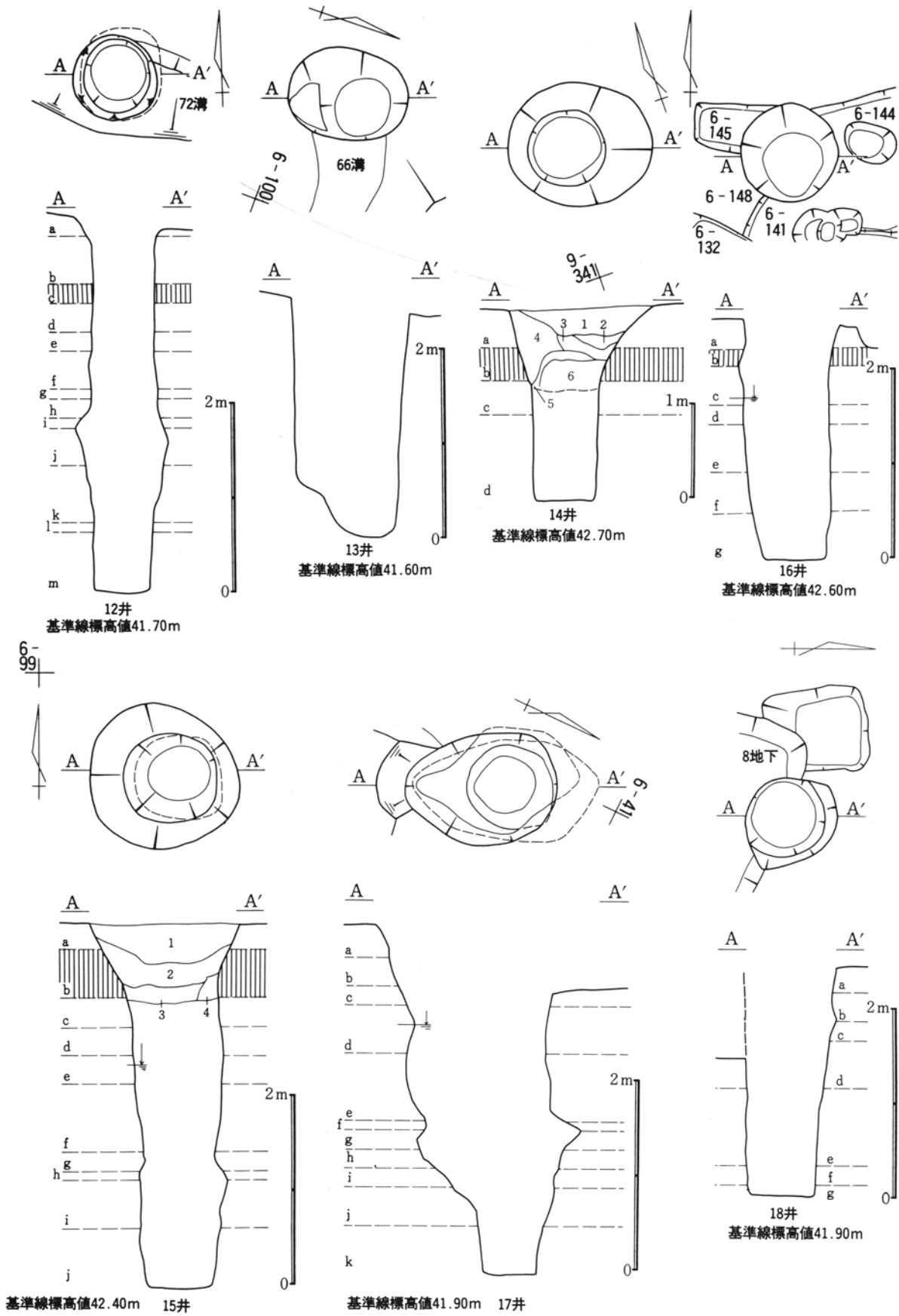
第541図 6区第12~18井戸跡実測図
