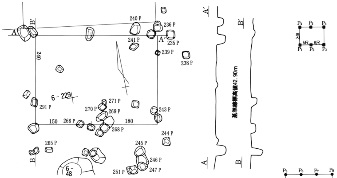
第400图 第2号掘立柱建物跡実測図
