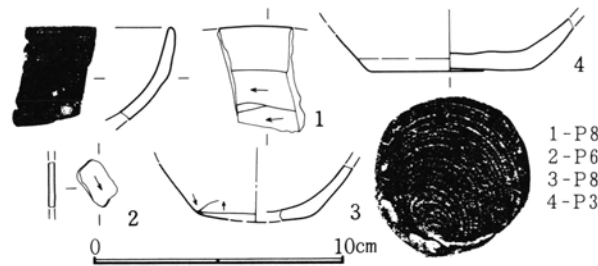
第454图 第25号掘立柱建物跡出土遺物実測図
