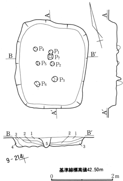
第381図 第6号竖穴状遺構実測図
