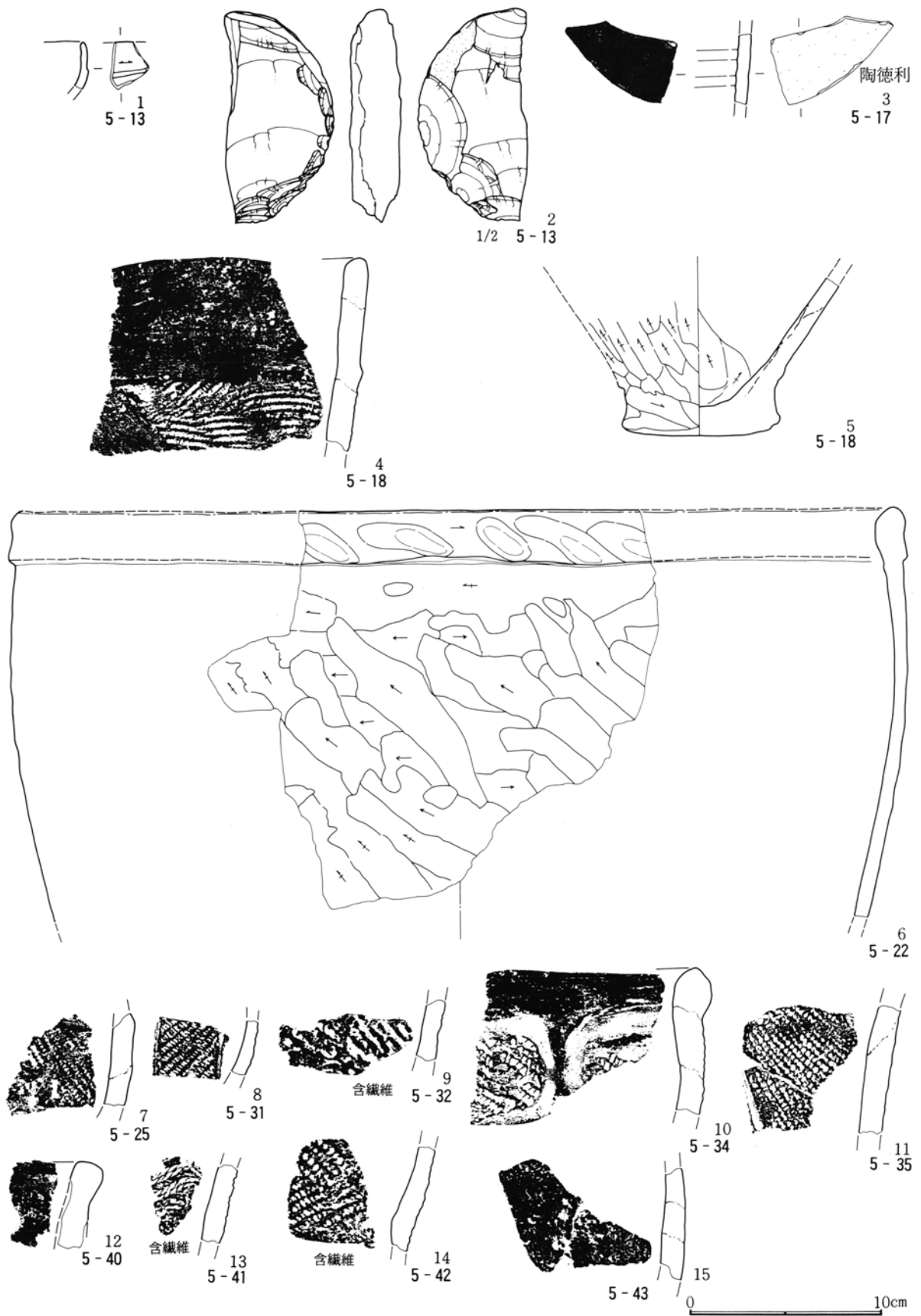
第616図 5区土坑出土遺物実測図(2)
