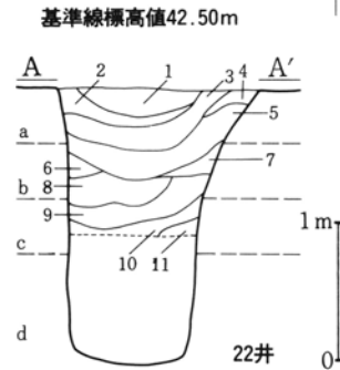
第563図 9区第18・19・20・22・25・26・27・28号井戸跡実測図
