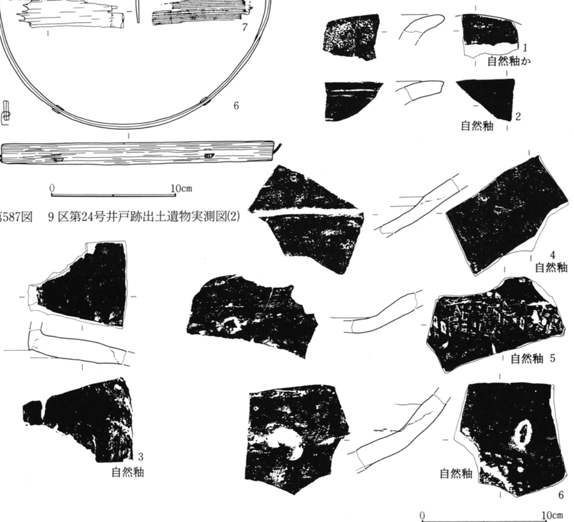
第589图 9区第26号井戸跡出土遺物実測図
