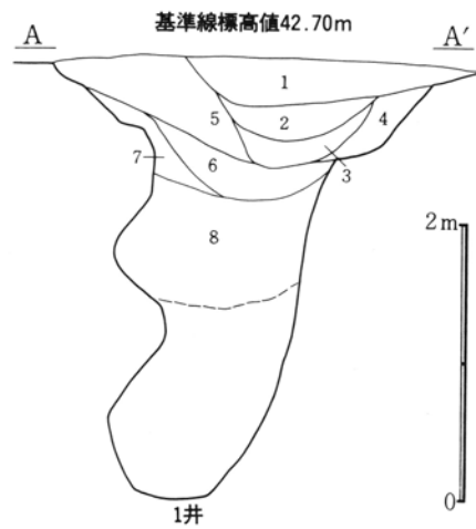
第496图 3区第1号井戸跡実測図
