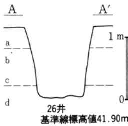
第563図 9区第18・19・20・22・25・26・27・28号井戸跡実測図
