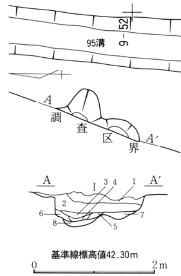
第360図 第167号住居跡実測図
