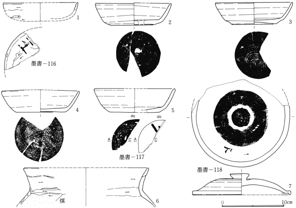
第364図 第170号住居跡出土遺物実測図
