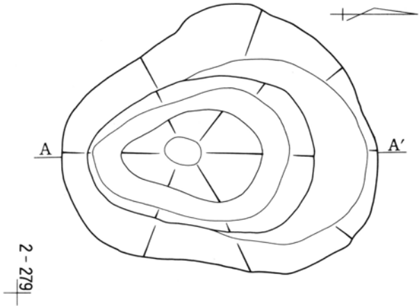
第492図 2区第1号井戸跡実測図
