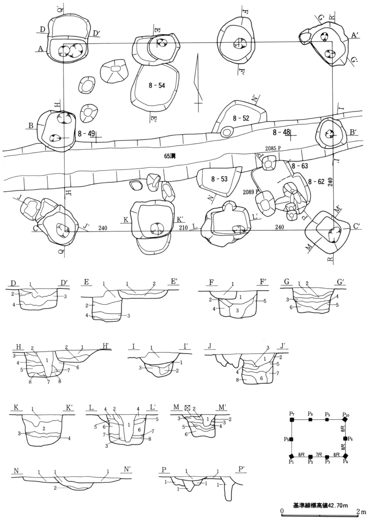
第411図 第13号掘立柱建物跡実測図(1)
