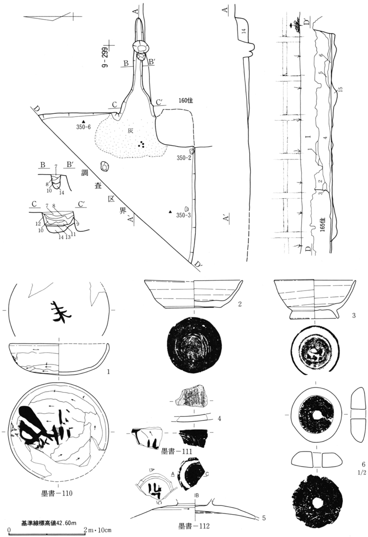
第350図 第161号住居跡・出土遺物実測図(2)
