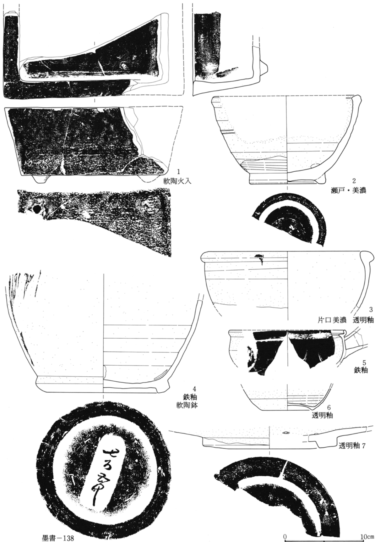
第570図 9区第11号井戸跡出土遺物実測図(3)
