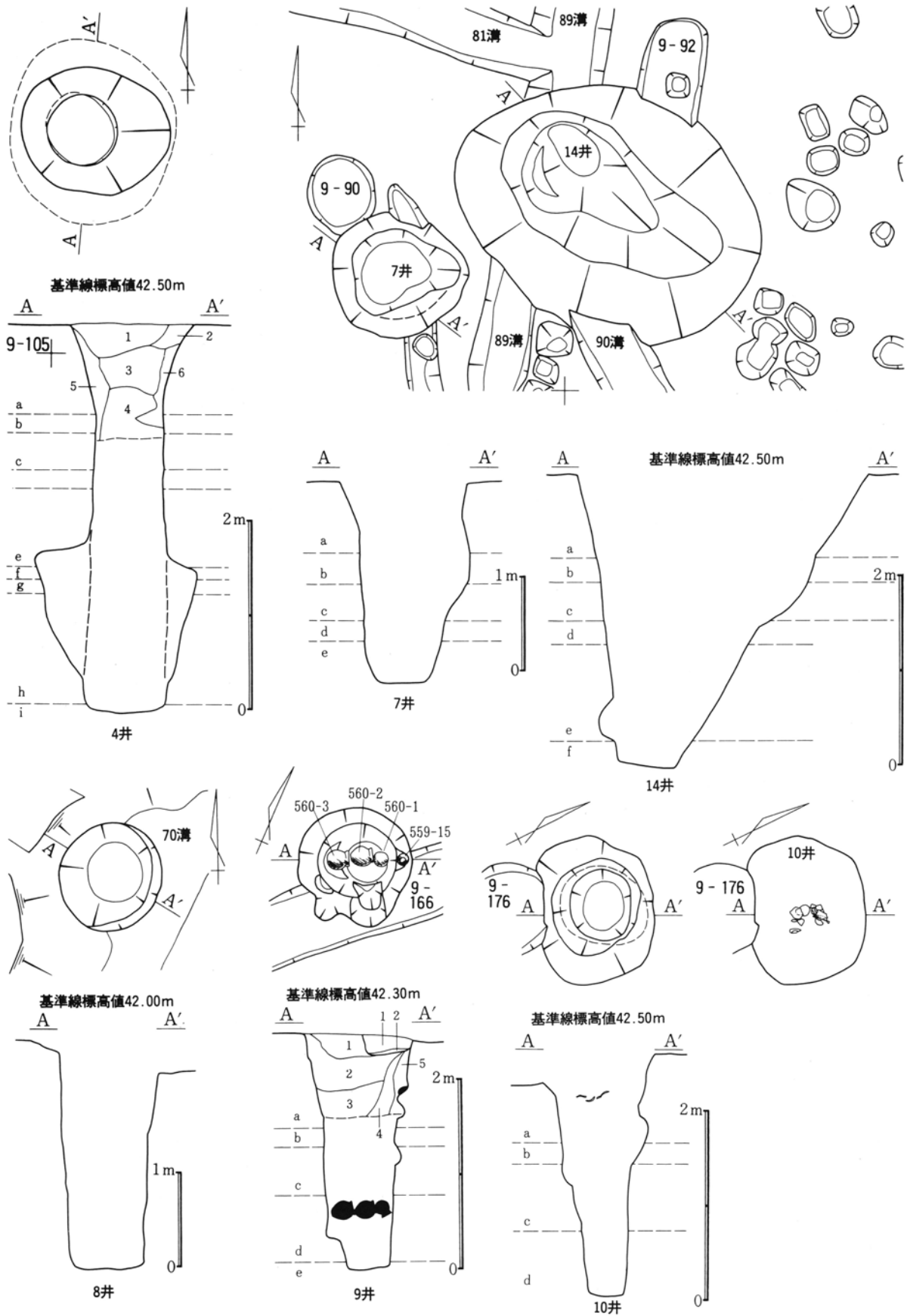
第561図 9区第4・7・8・9・10・14号井戸跡実測図
