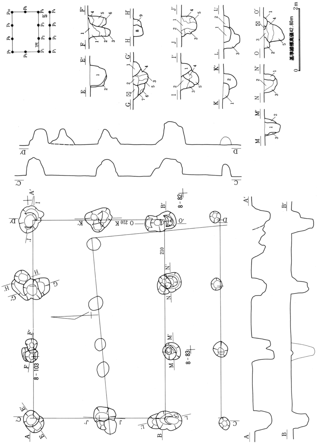
第402图 第4号掘立柱建物跡美測図
