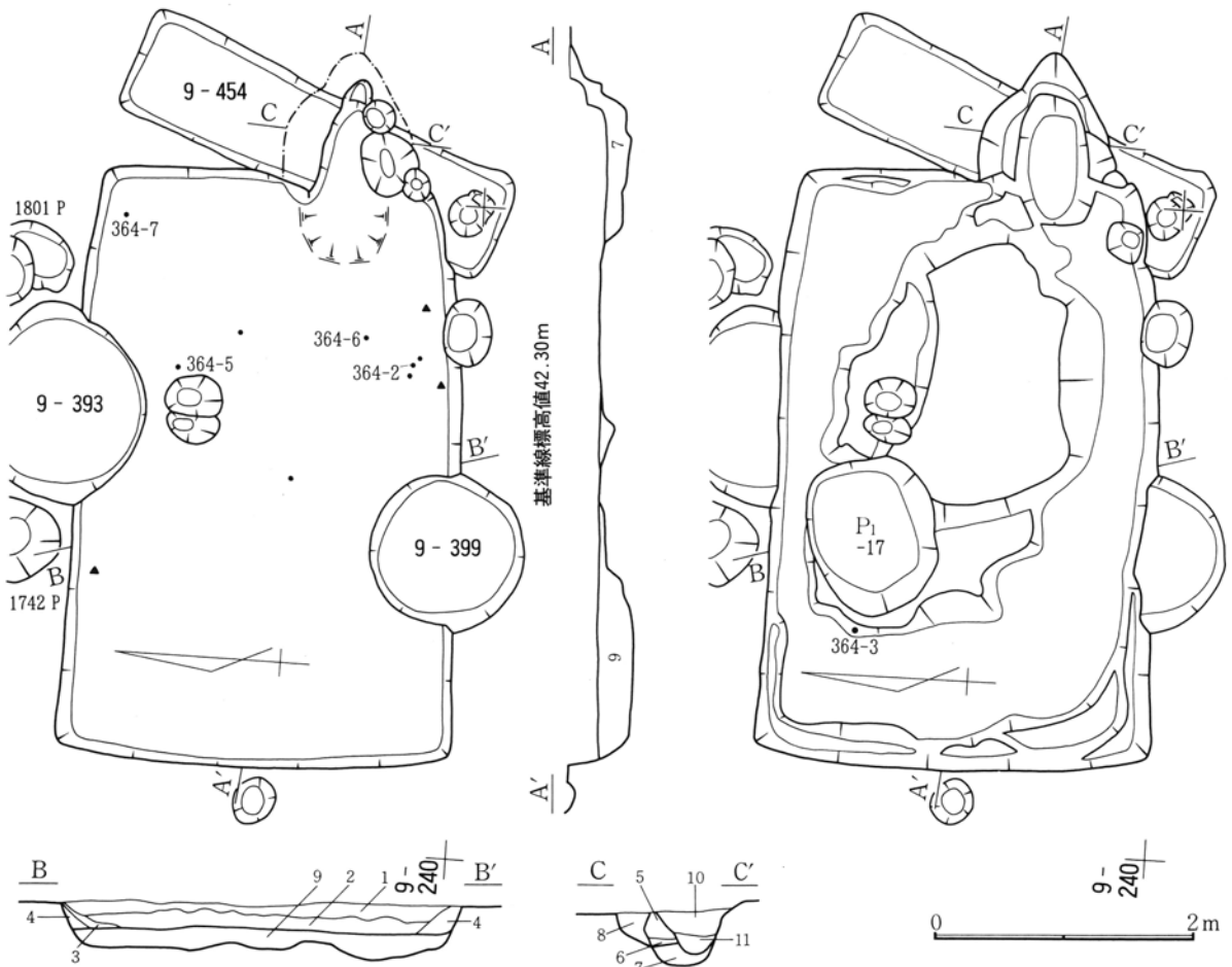
第363図 第170号住居跡実測図
