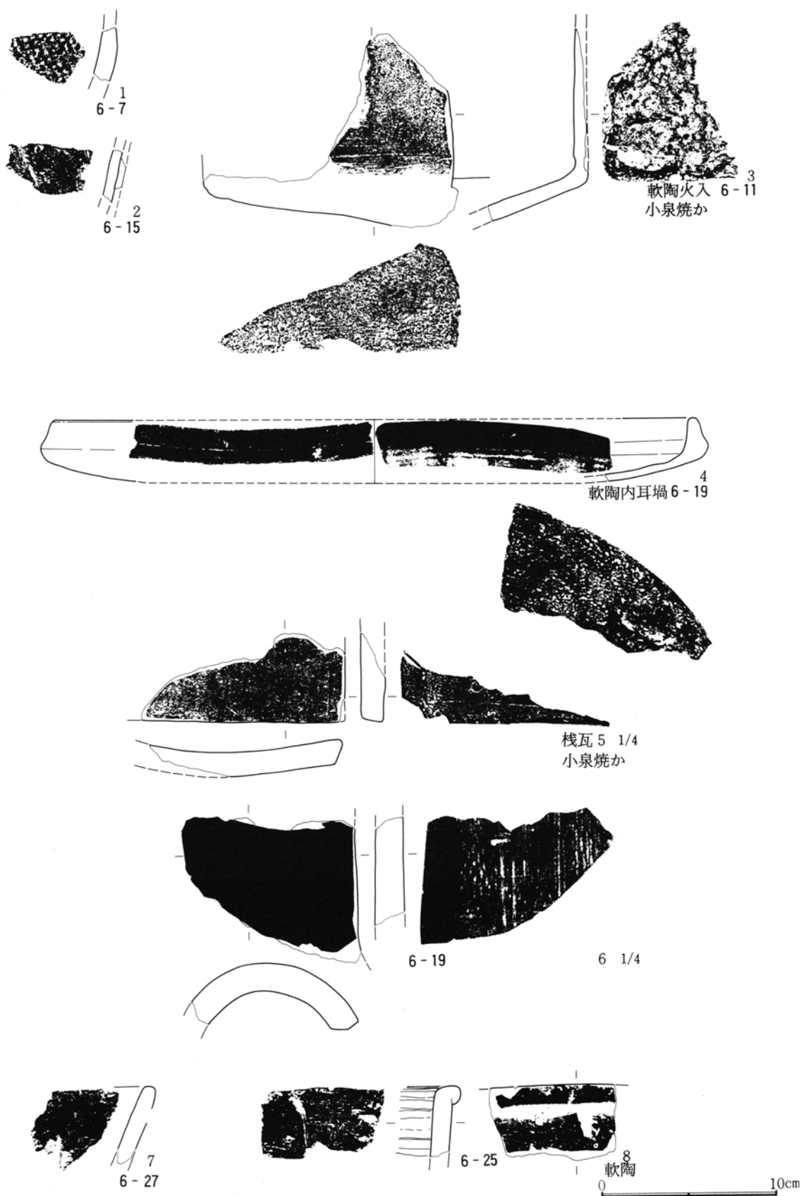
第624図 6区土坑出土遺物実測図(1)
