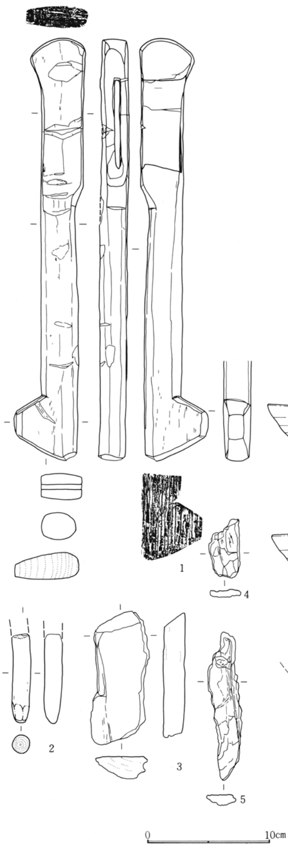
第585図 9区第23号井戸跡出土遺物実測図(2)
