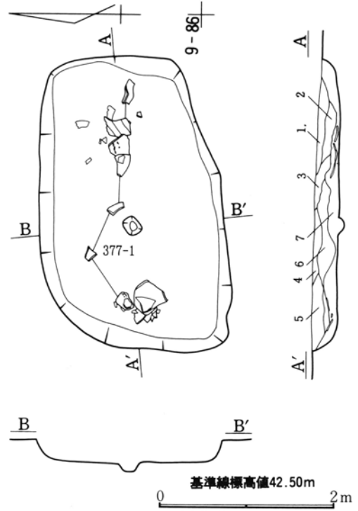
第375図 第3号竖穴状遺構実測図
