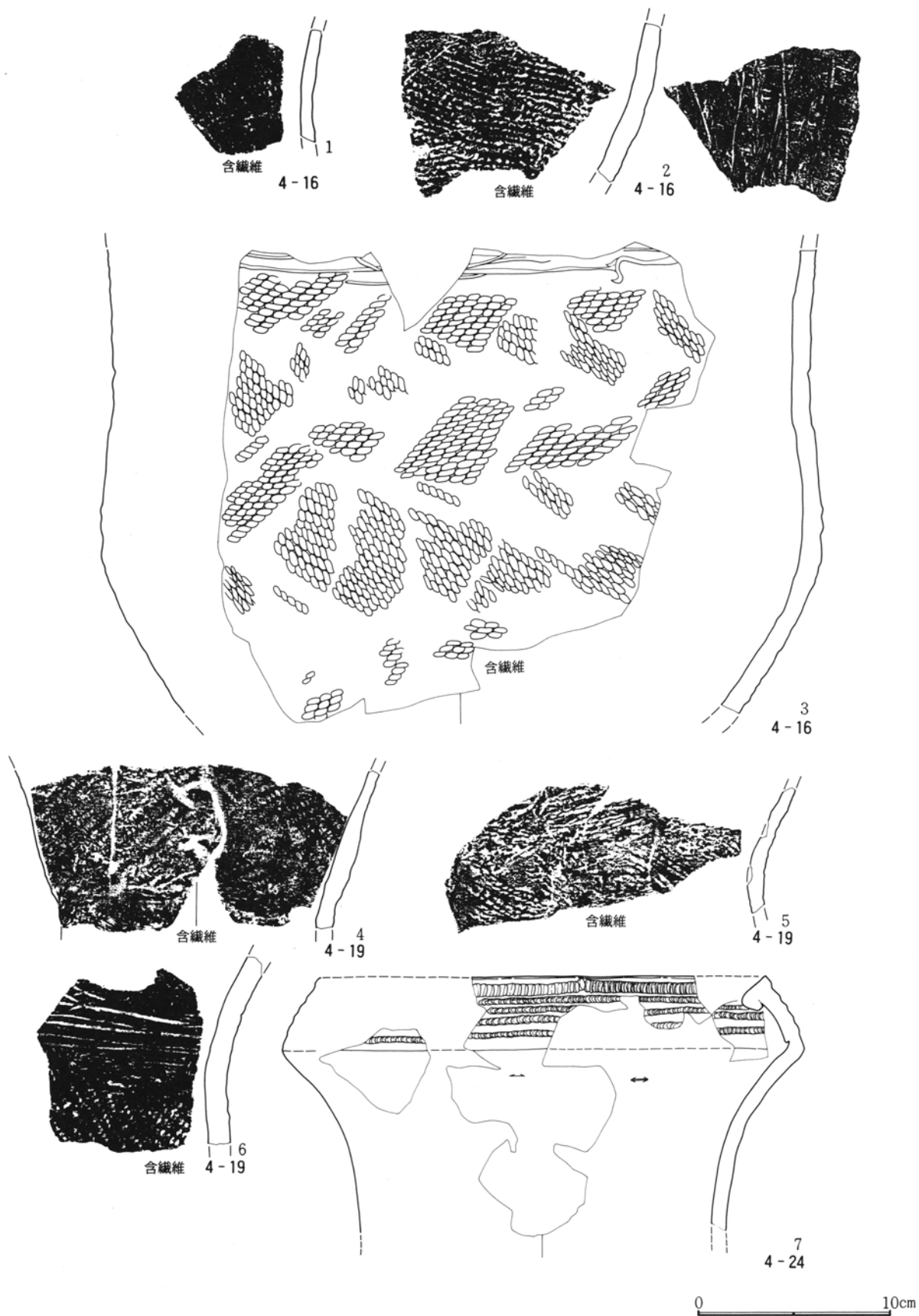
第603図 4区土坑出土遺物実測図(2)
