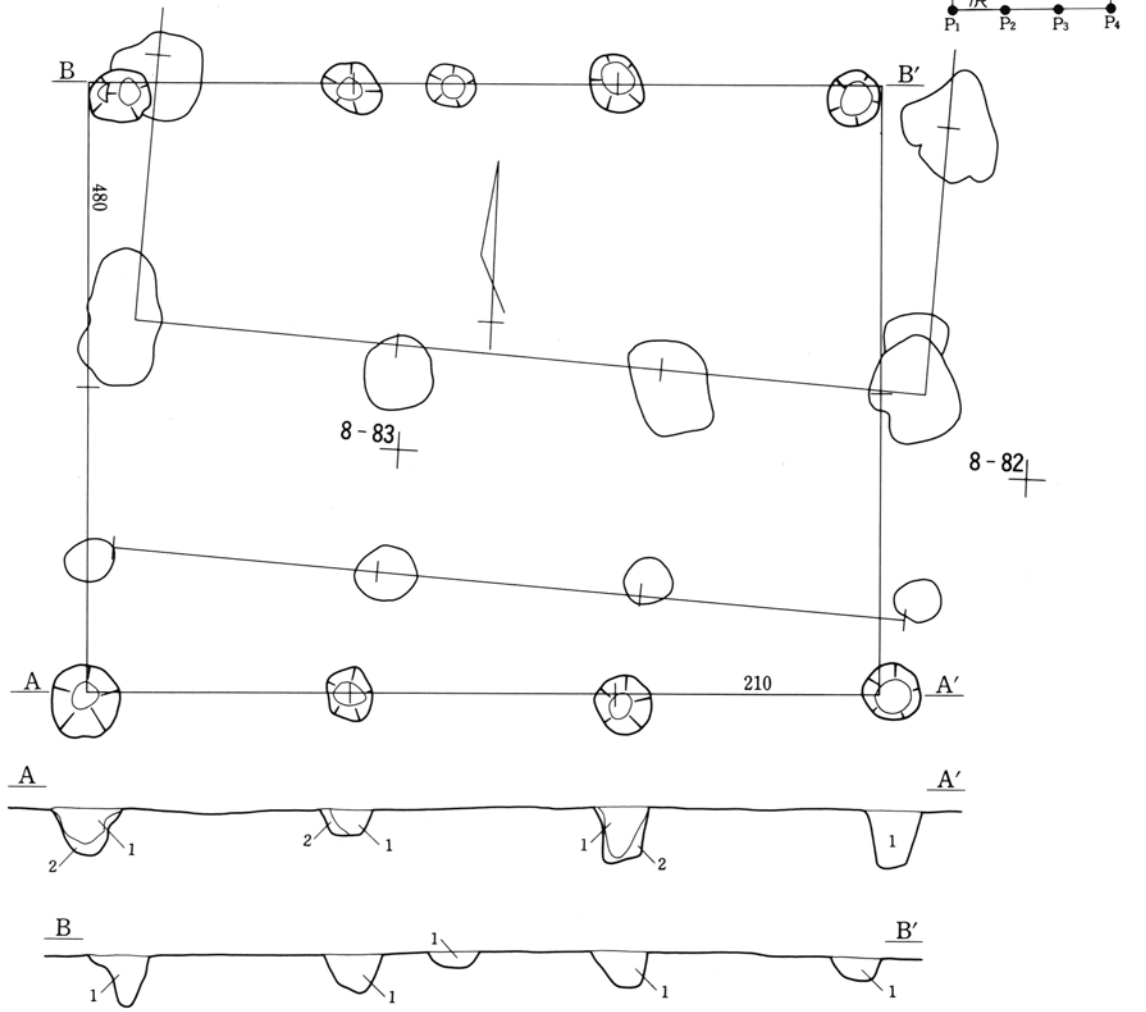
第401图 第3号掘立柱建物跡実測図
