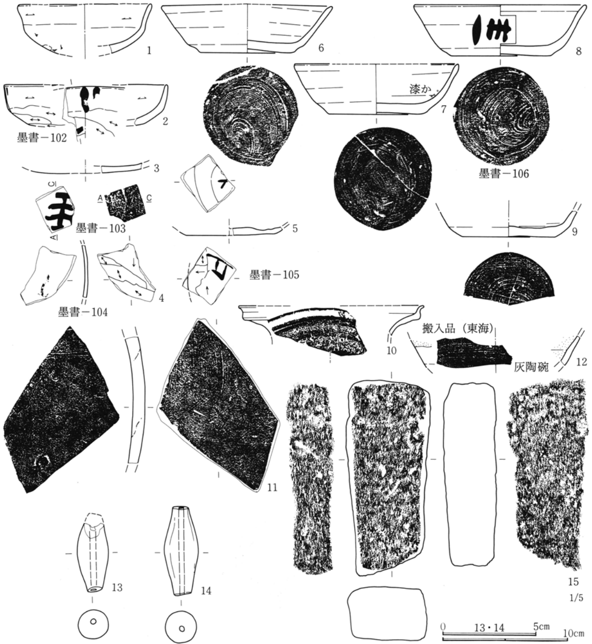
第348図 第160号住居跡出土遺物実測図
