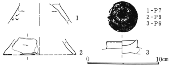
第453图 第24号掘立柱建物跡出土遺物実測図
