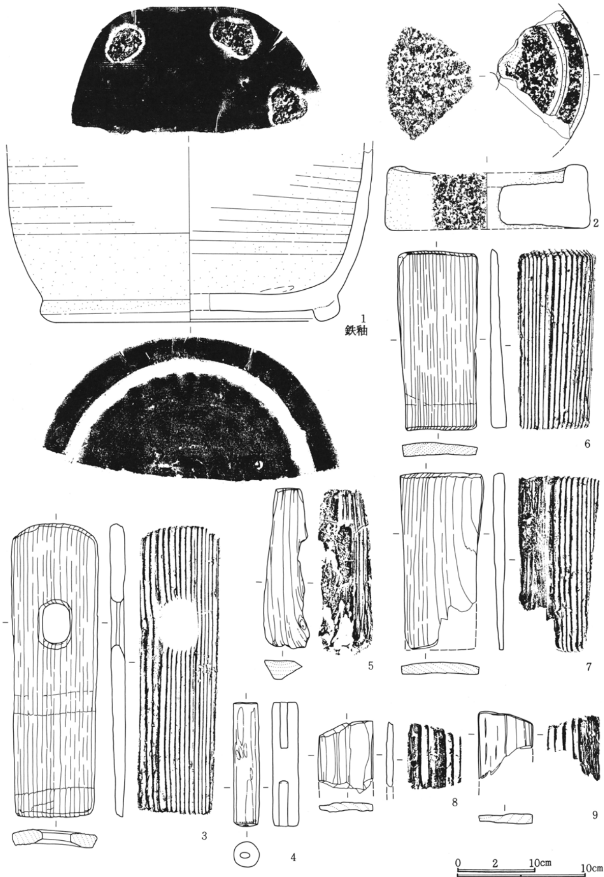
第537图 6区第4号井戸跡出土遺物実測図(1)
