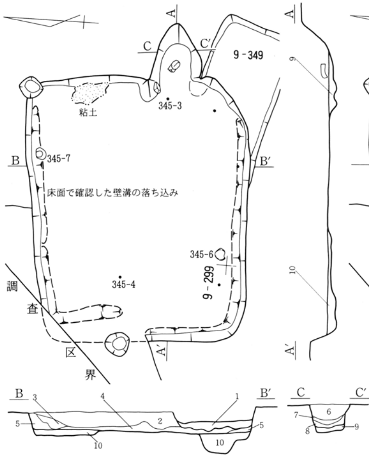
第346図 第159号住居跡実測図
