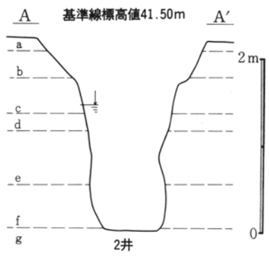
第550図 7区第2号井戸跡実測図
