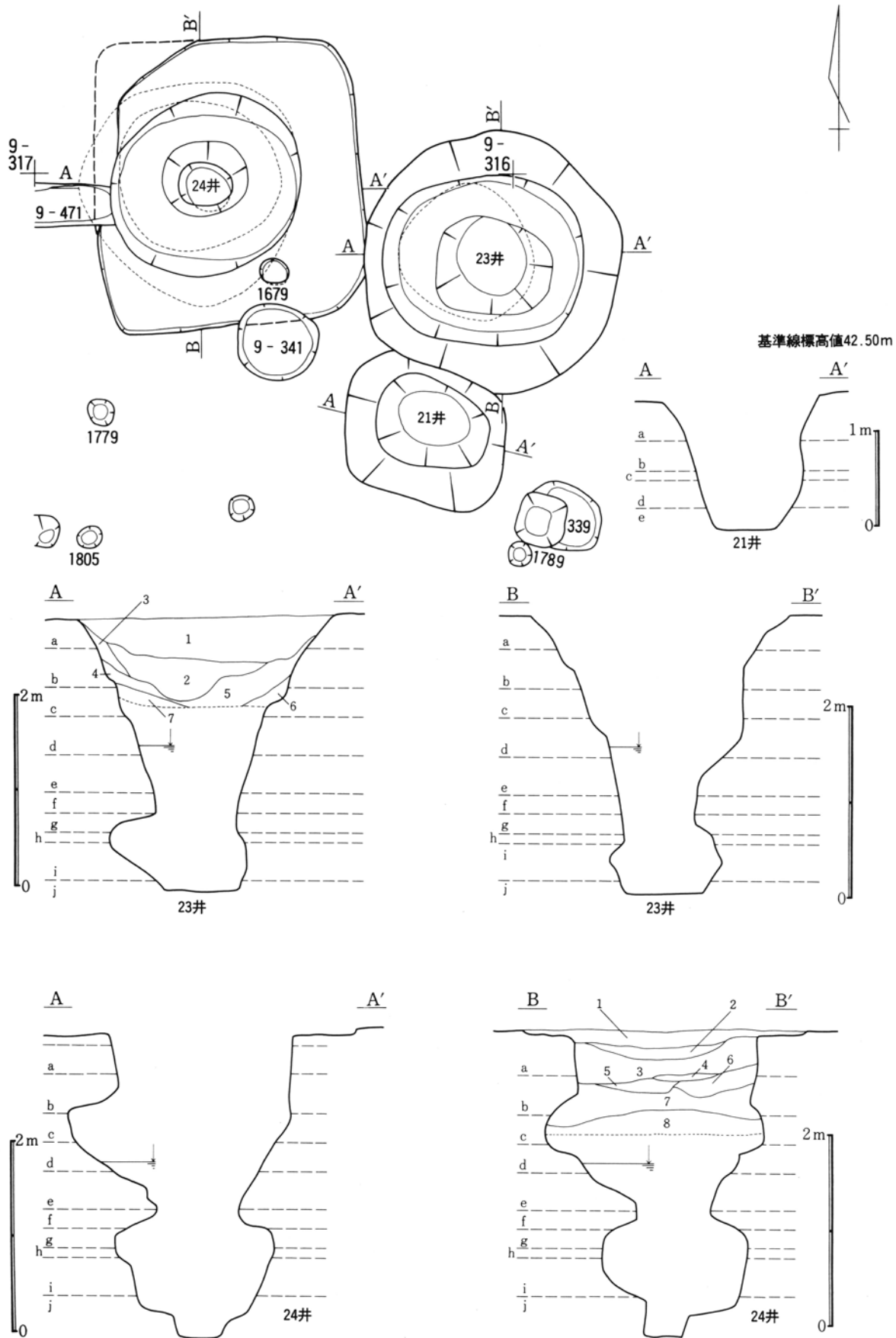
第564図 9区第21・23・24号井戸跡実測図
