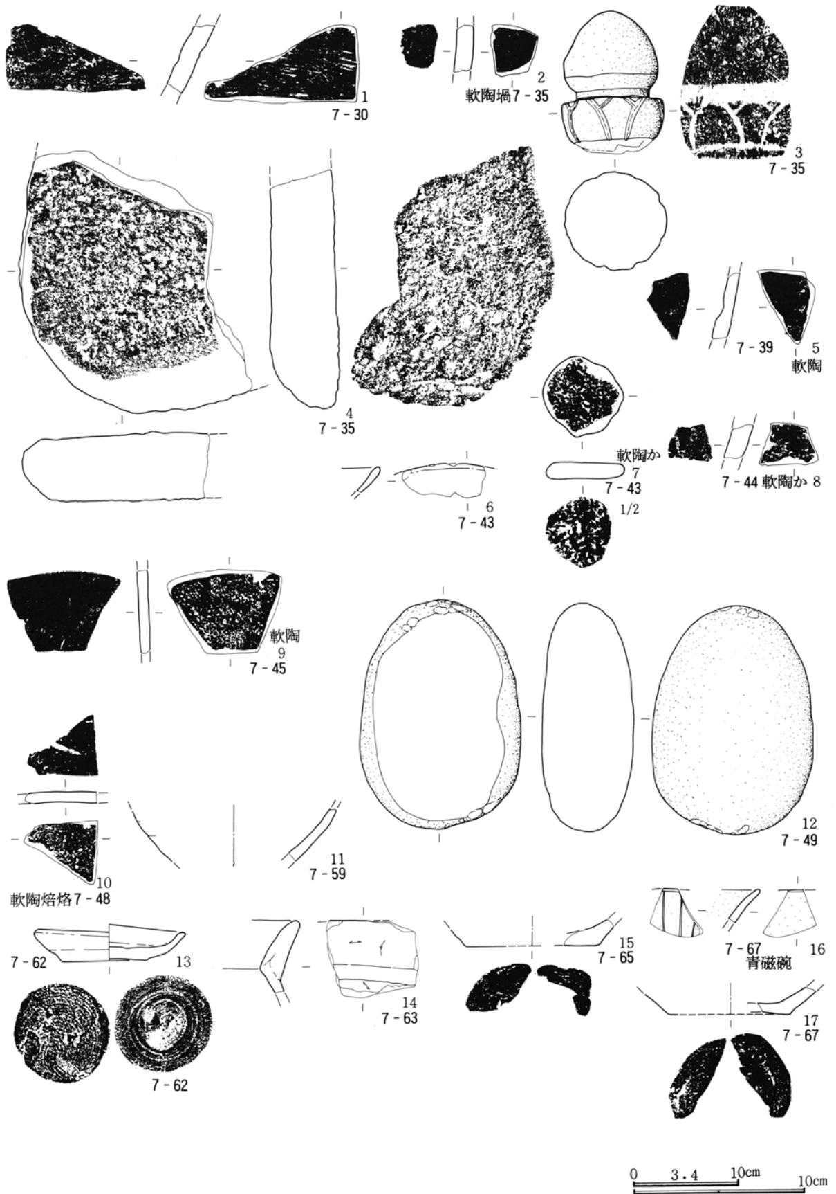
第634図 7区土坑出土遺物実測図(5)
