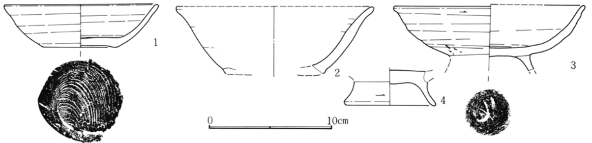
第324図 第148号住居跡出土遺物実測図(1)
