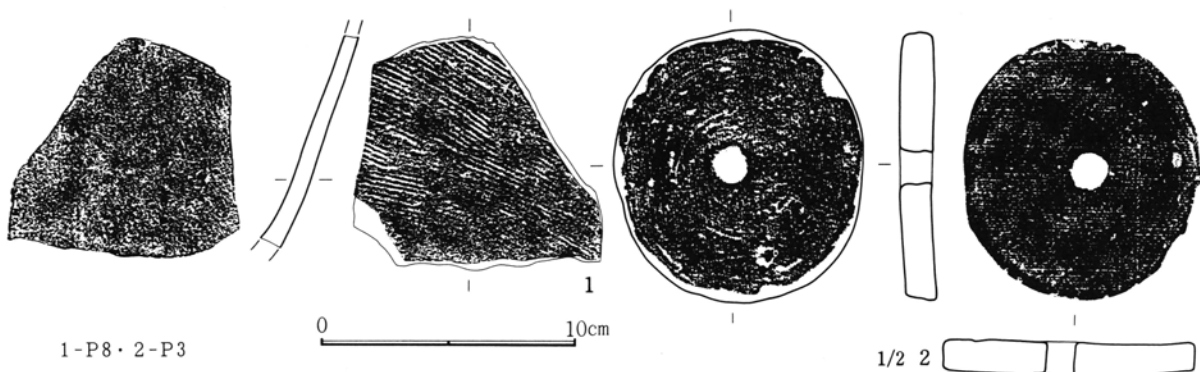
第460图 第30号掘立柱建物跡出土遺物実測図(2)
