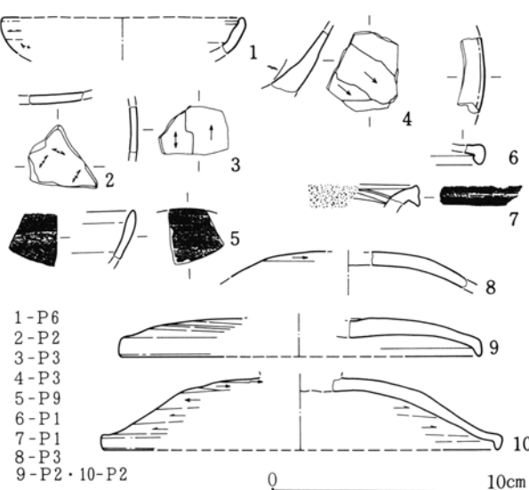
第462图 第32号掘立柱建物跡出土遺物実測図
