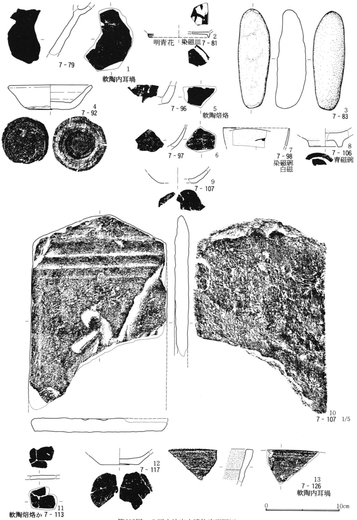
第635图 7区土坑出土遺物実測図(6)
