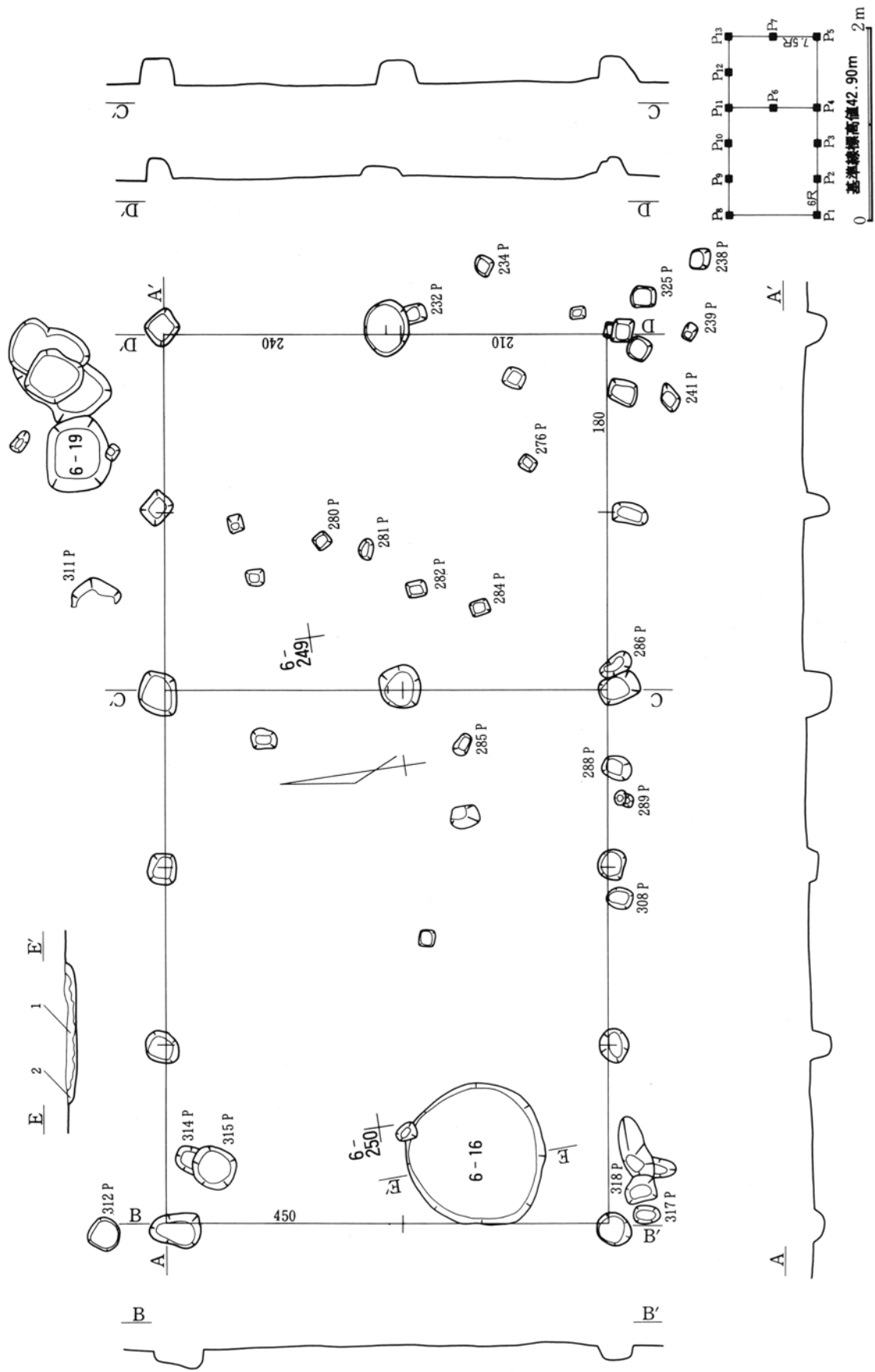
第399图 第1号掘立柱建筑物实测图
