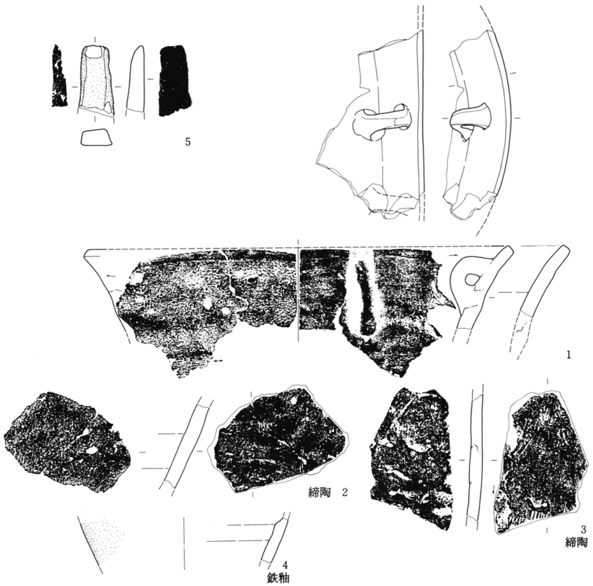
第485図 第10号地下式土坑出土遺物実測図(3)
