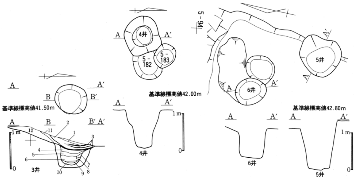
第502図 5区第3号井戸跡実測図
