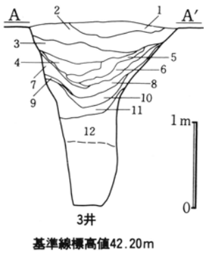
第495图 2区第3号井戸跡実測図
