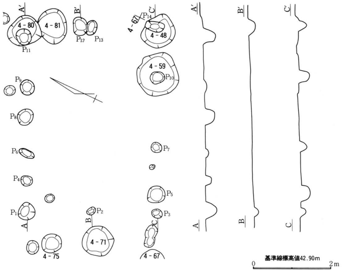
第426図 第26号掘立柱建物跡実測図
