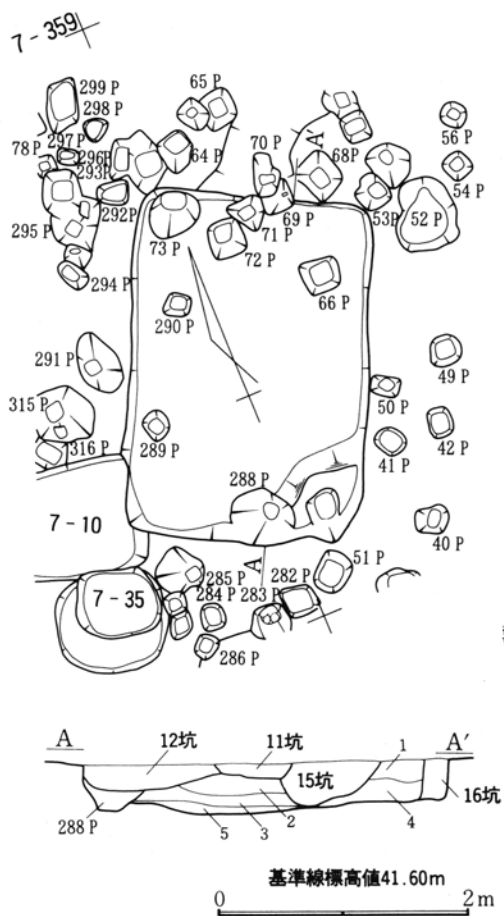
第394図 第21号豎穴状遺構実測図
