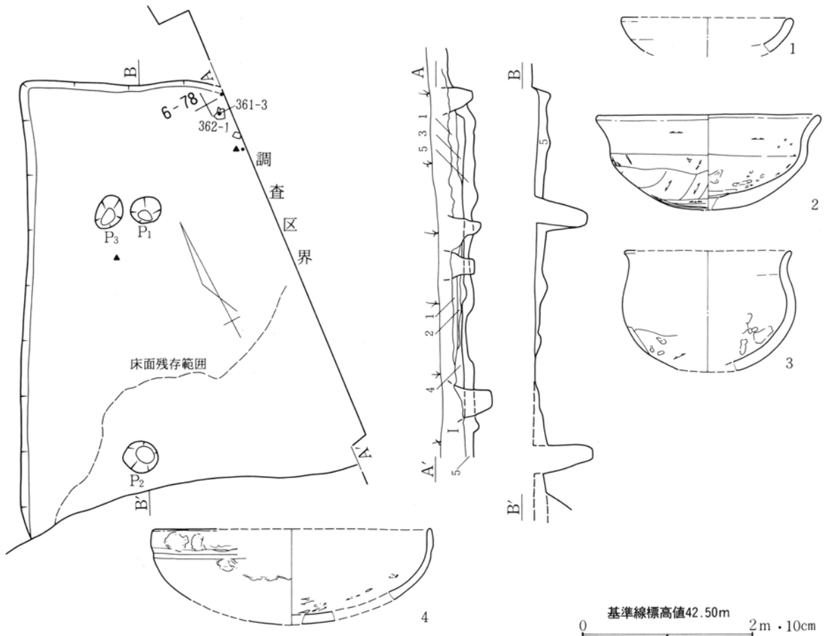
第361図 第168号住居跡・出土遺物実測図(1)
