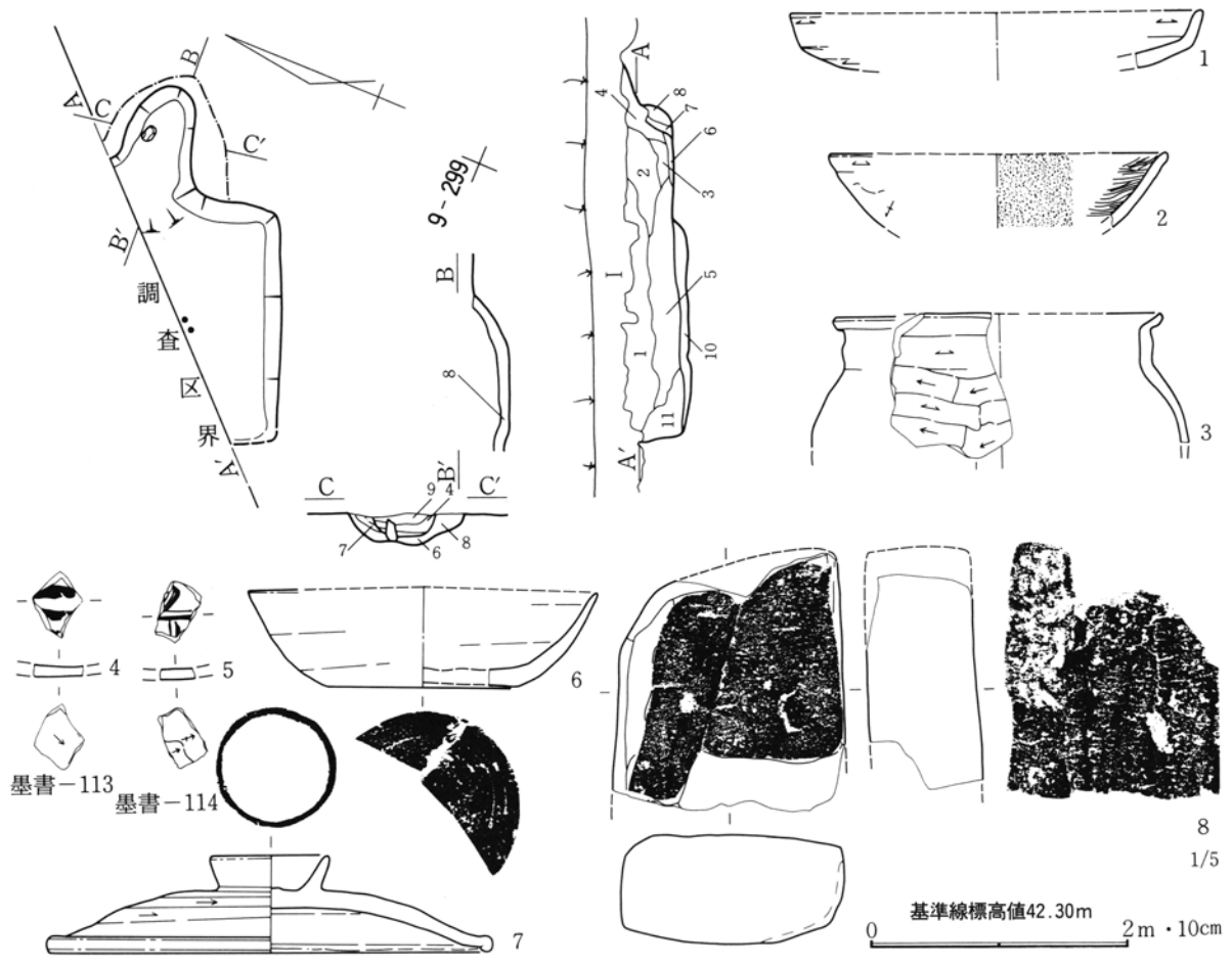
第357図 第165号住居跡・出土遺物実測図
