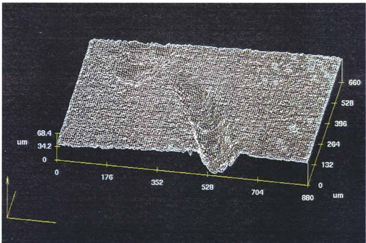
第617図 レーザ顕微鏡による鏡面の整痕の観察
