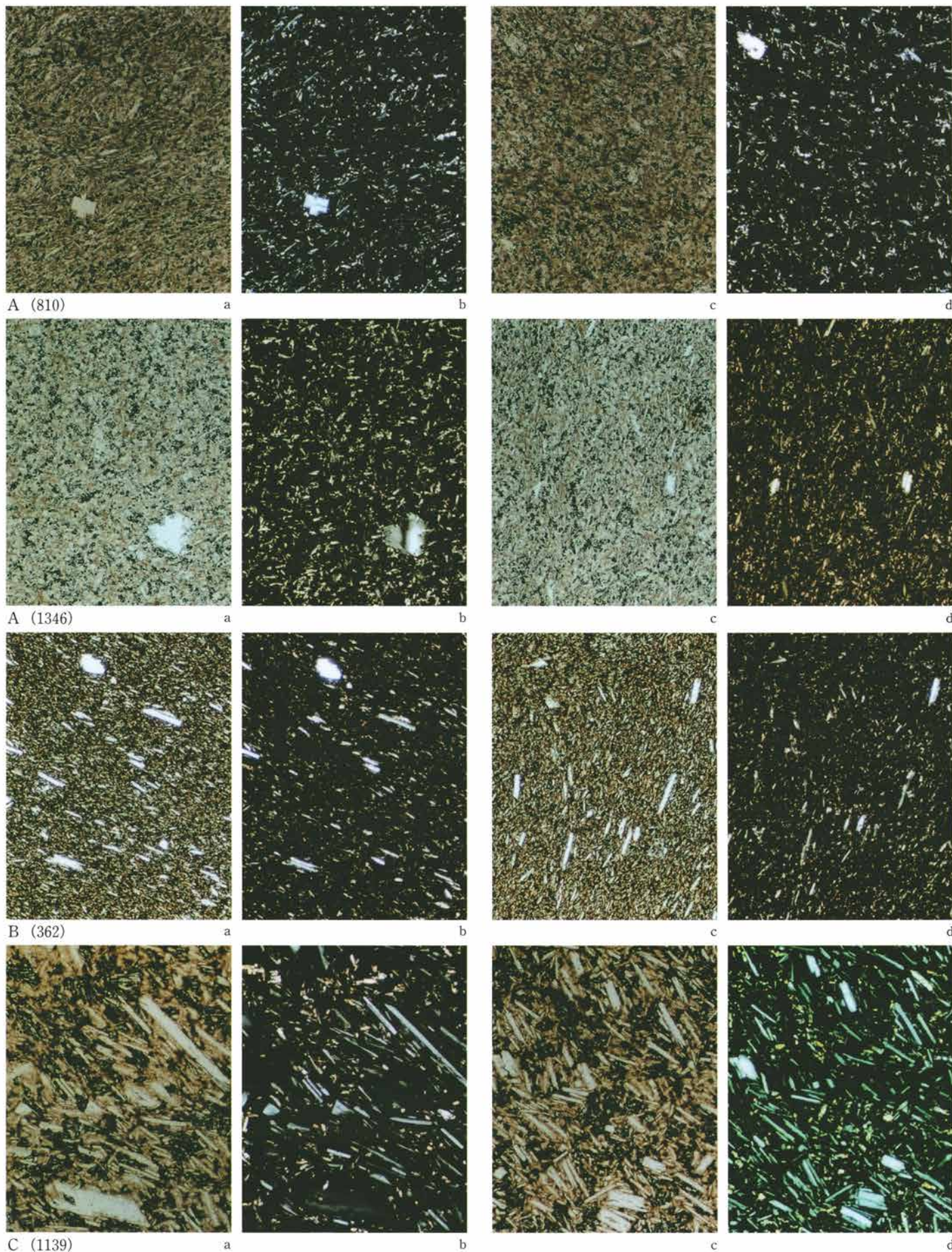
黒色安山岩のプレパラートの偏光顕微鏡写真 (3) (a, c: 平行ニコル b, d: 直交ニコル×50)
