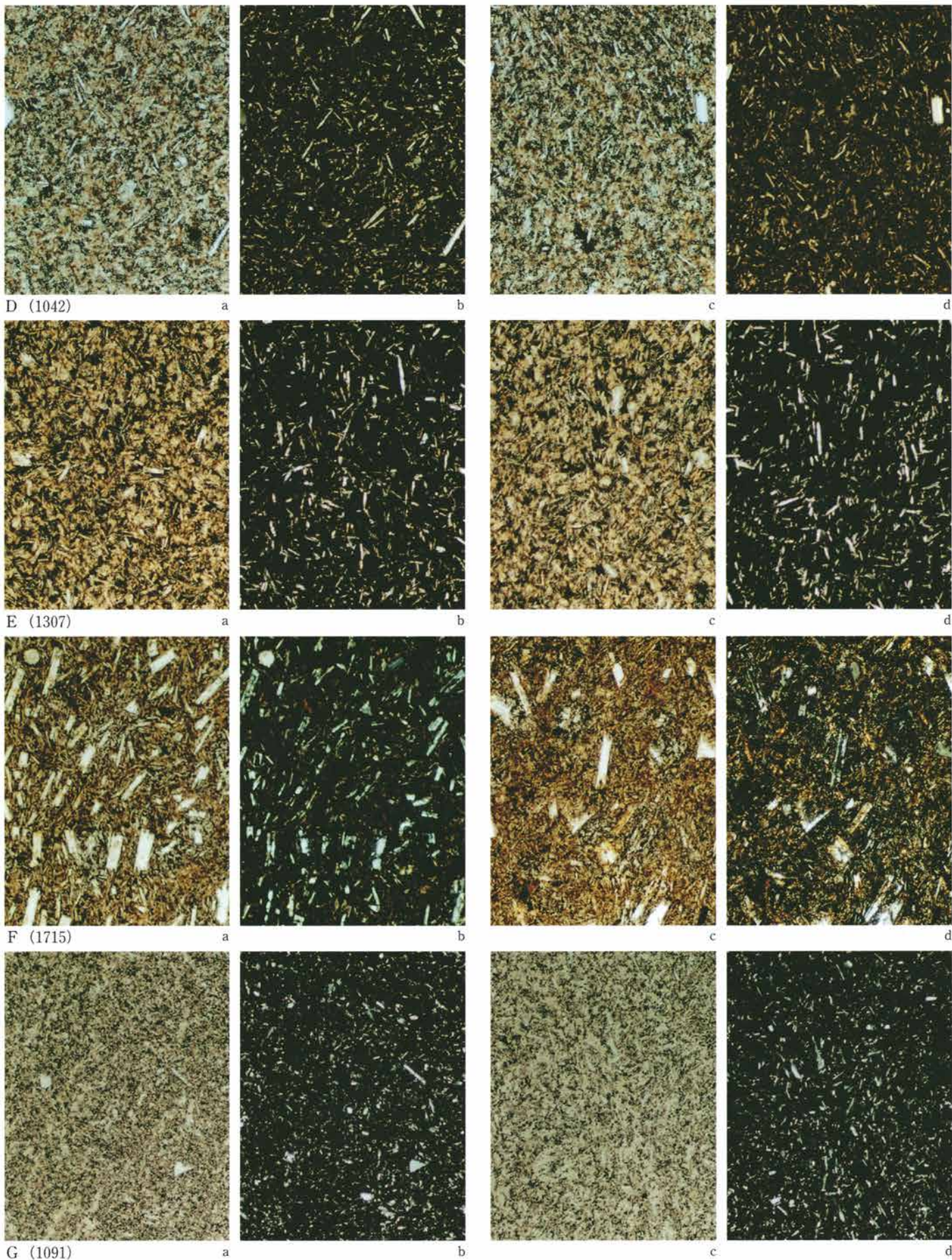
黒色安山岩のプレパラートの偏光顕微鏡写真(4) (a, c: 平行ニコル b, d: 直交ニコル×50)
