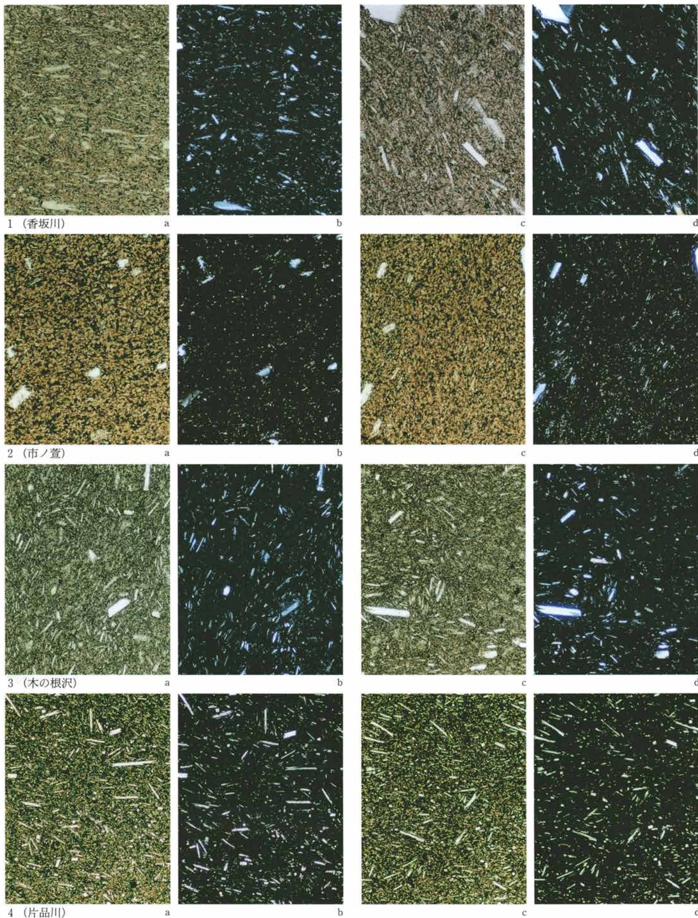
黒色安山岩のプレパラートの偏光顕微鏡写真 (1) (a, c: 平行ニゴル b, d: 直交ニゴル×50)
