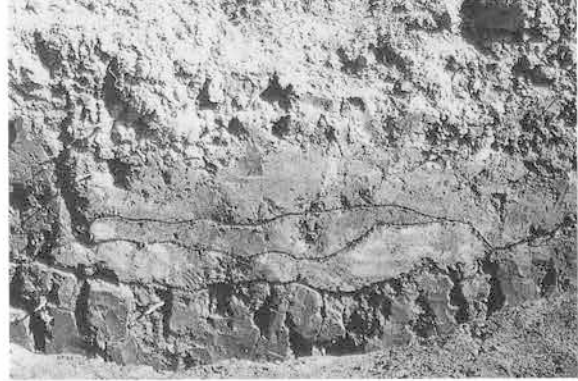
20号溝跡土層断面 西→
