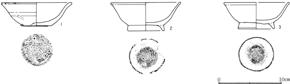
第558図 6号住居状遺構出土遺物実測図
