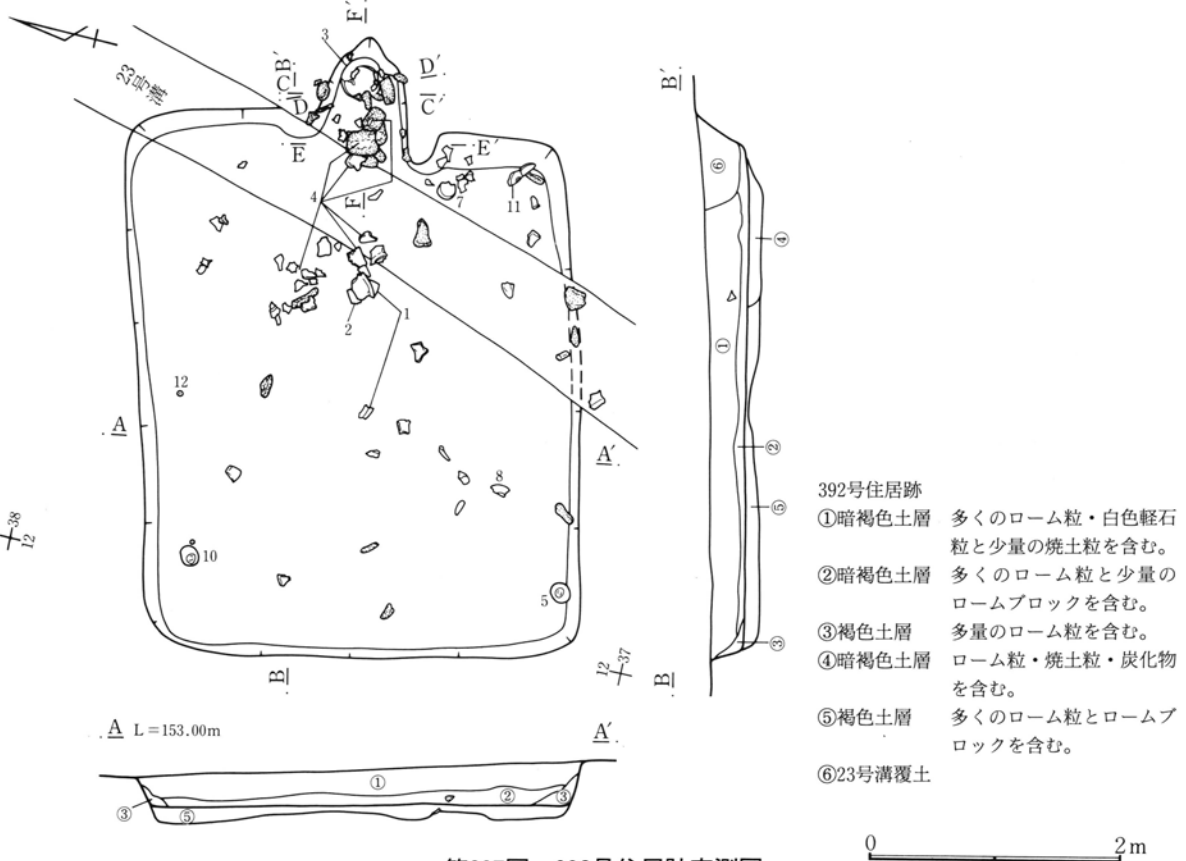
第297図 392号住居跡実測図
