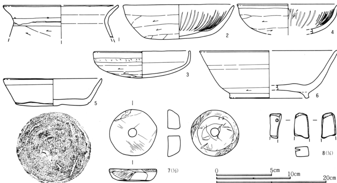
第426図 616号住居跡出土遺物実測図
