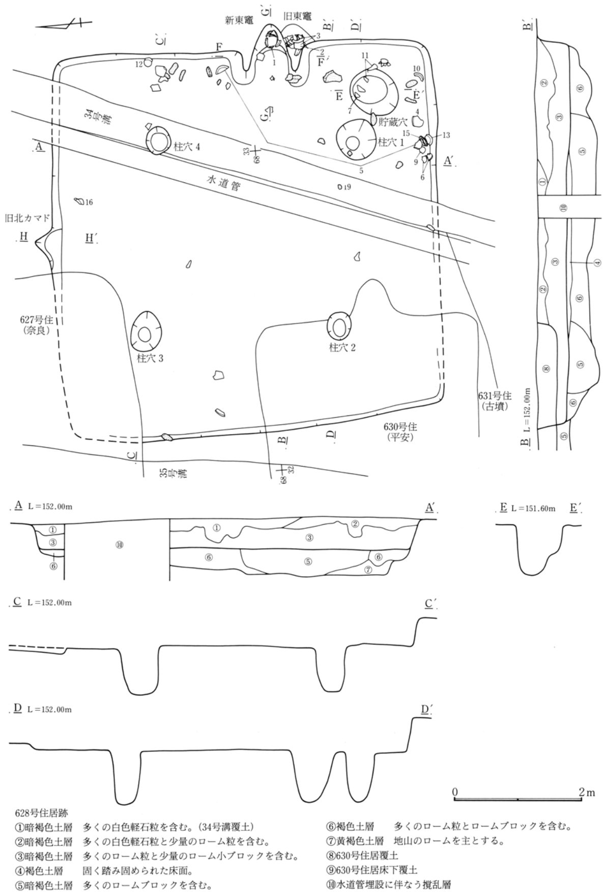
第435図 628号住居跡実測図
