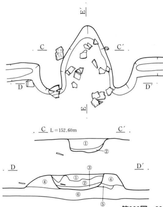
第303図 399号住居跡竈実測図
