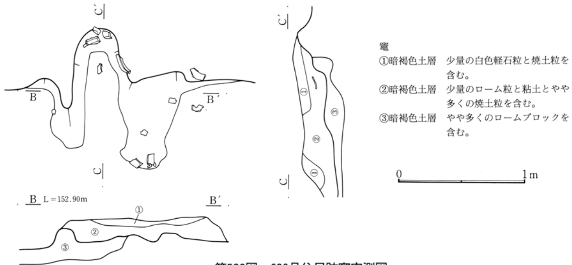
第528図 630号住居跡竈実測図
