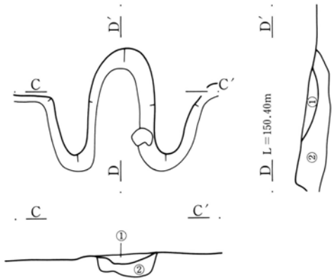
第465図 701号住居跡竈・出土遺物実測図
