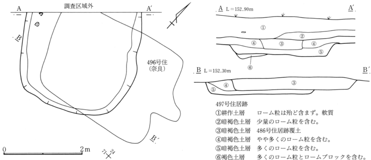
第546図 497号住居跡実測図
