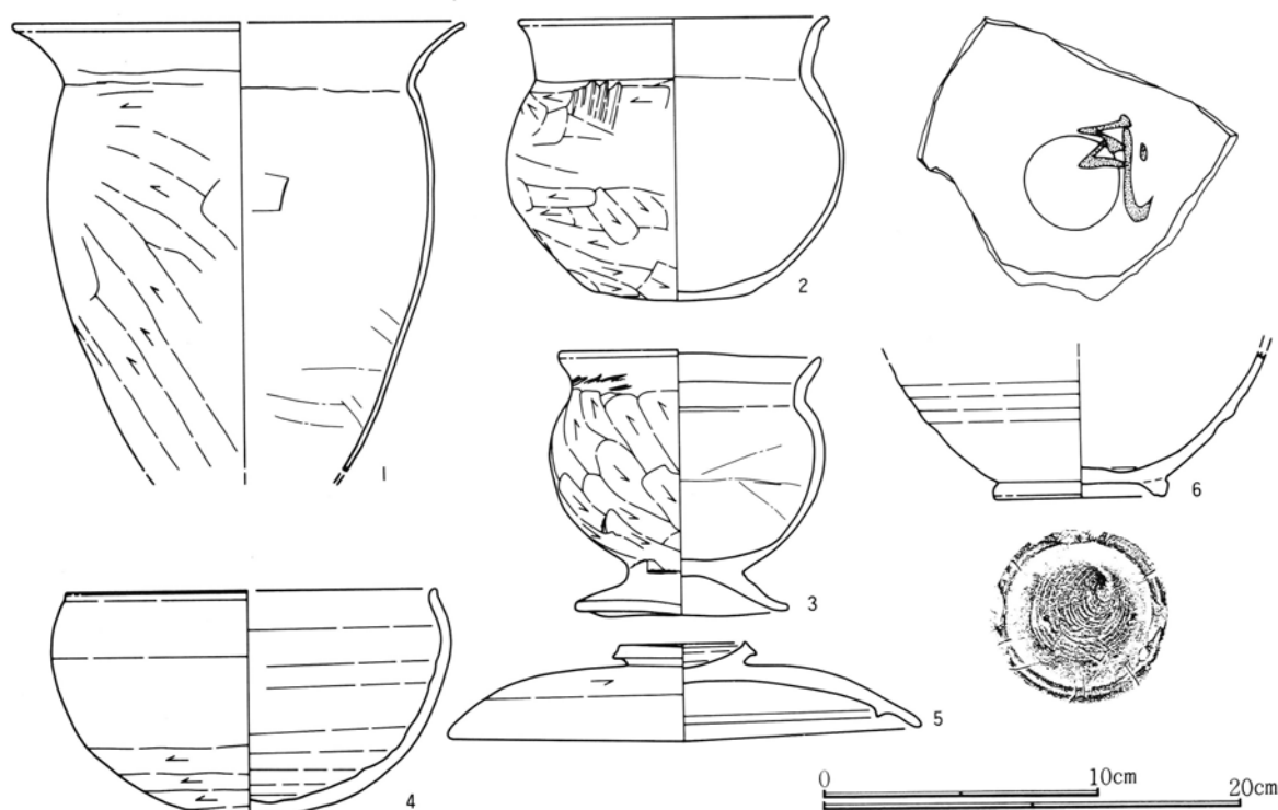
第416図 599号住居跡出土遺物実測図
