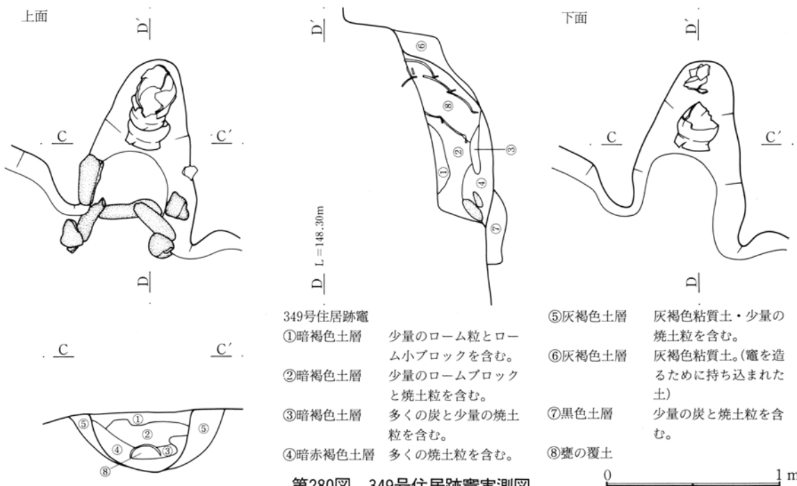
第280図 349号住居跡竈実測図
