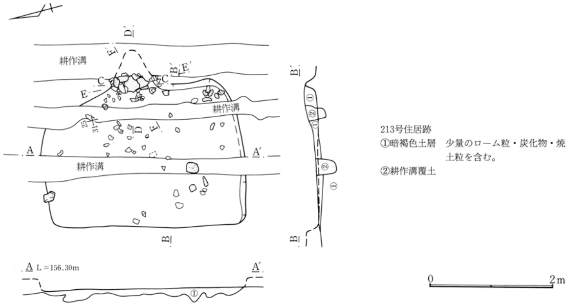
第512図 213号住居跡実測図
