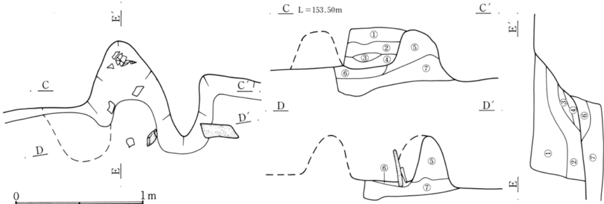
第325図 455号住居跡竈実測図
