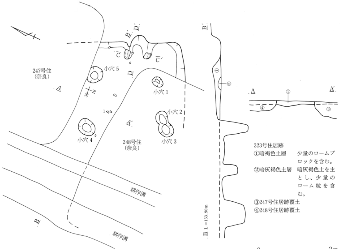
第271図 323号住居跡実測図
