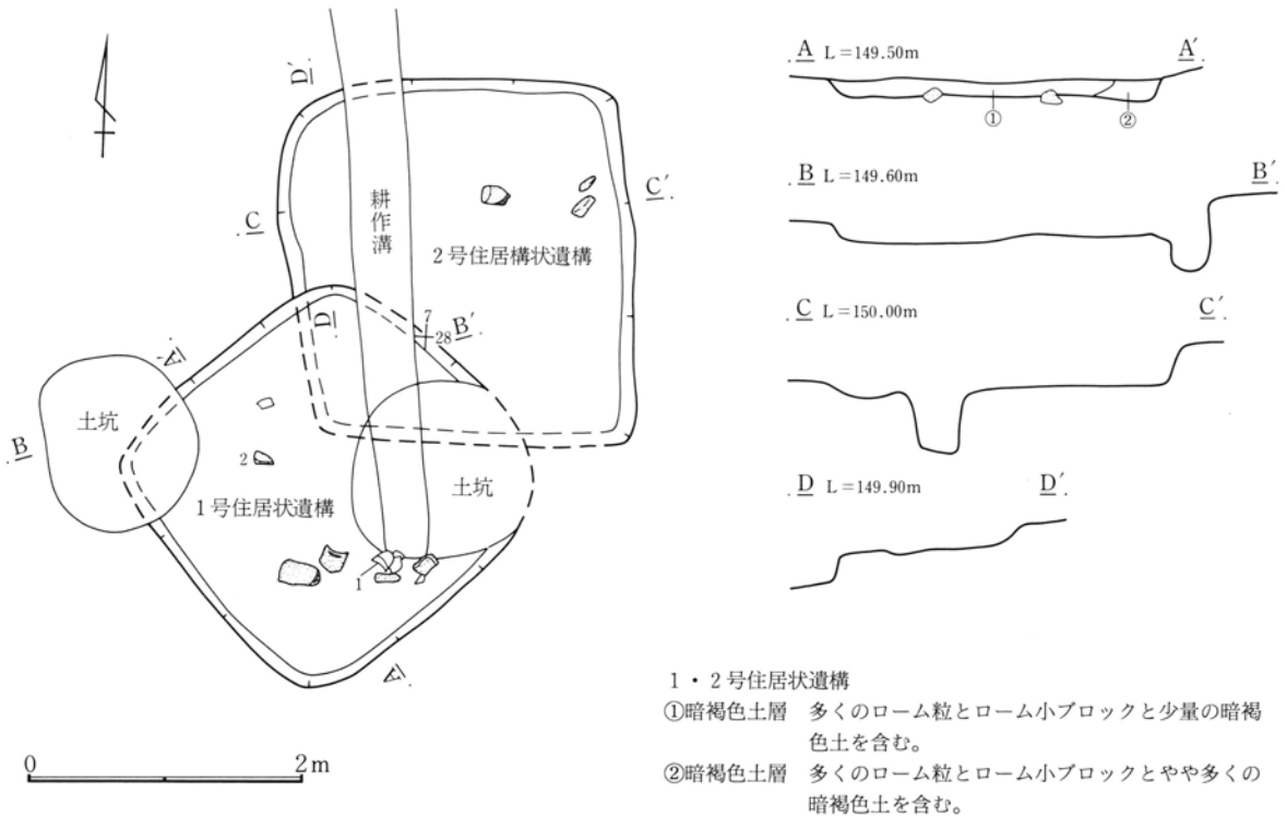
第554図 1・2号住居状遺構実測図
