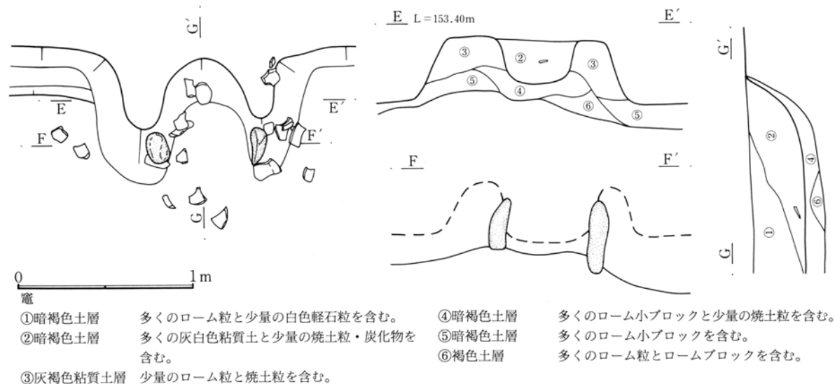
第328図 458号住居跡竈実測図
