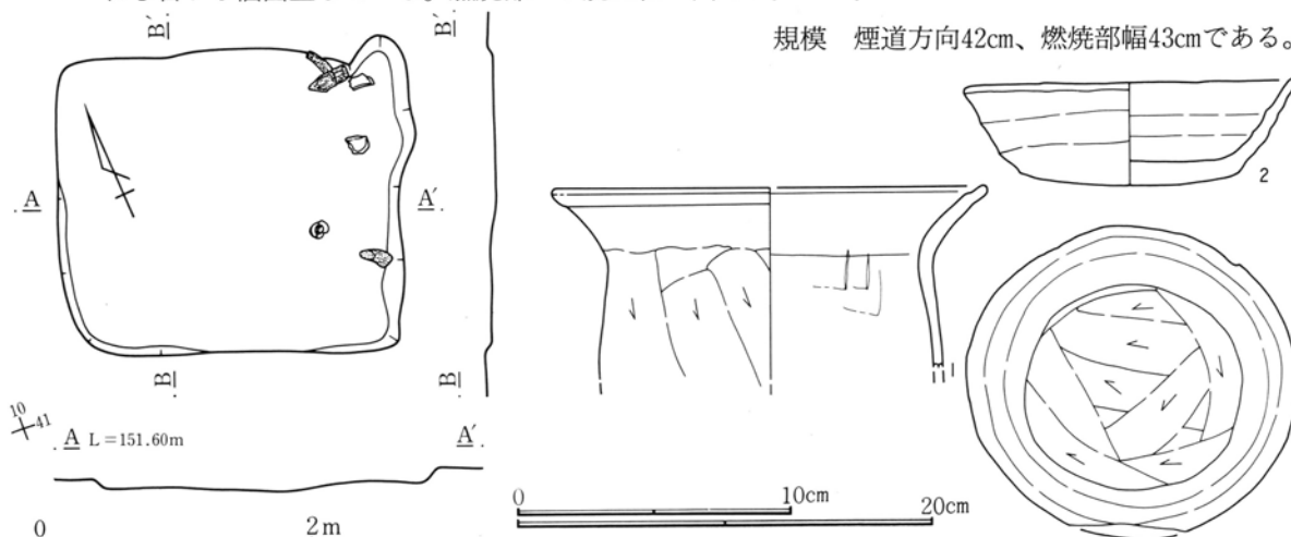
第310図 429号住居跡・出土遺物実測図
