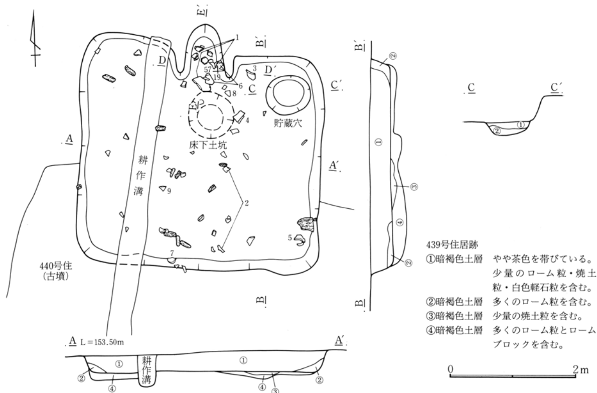
第318図 439号住居跡実測図
