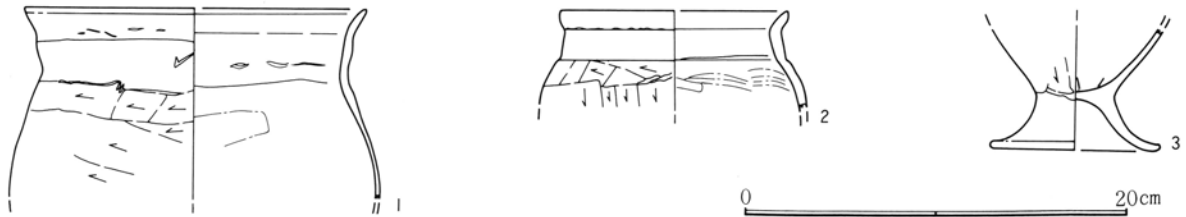
第526図 480号住居跡出土遺物実測図
