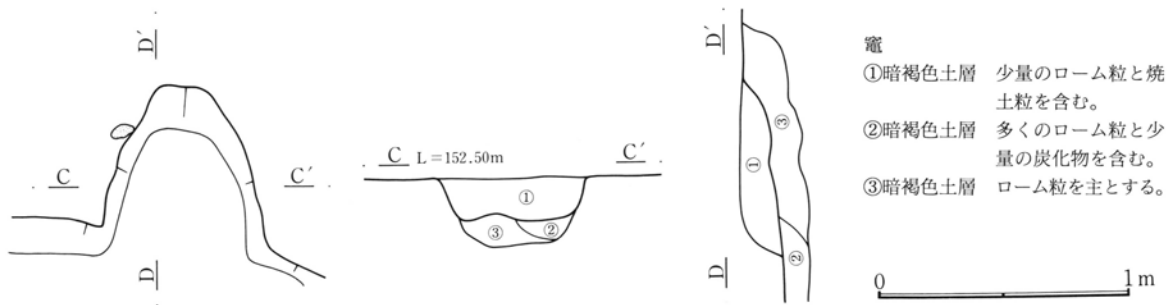
第336図 487号住居跡竈実測図
