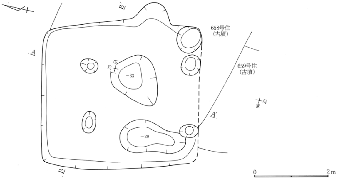
第456図 655号住居跡床下実測図
