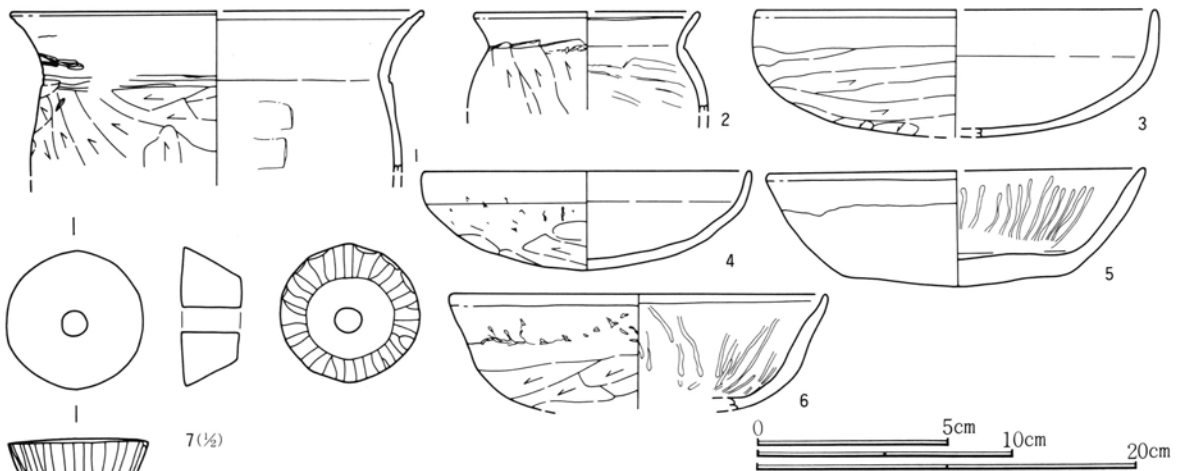
第375図 551号住居跡出土遺物実測図
