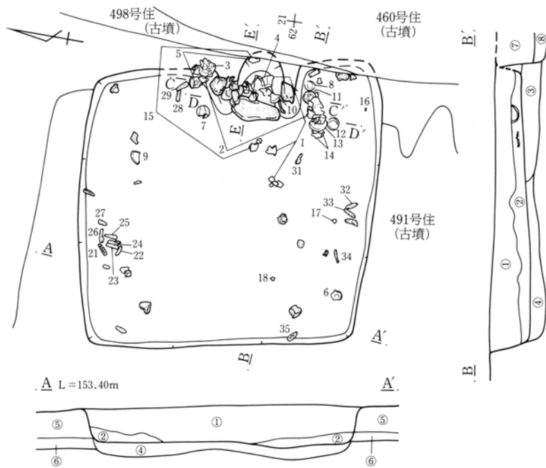
第341図 490号住居跡実測図
