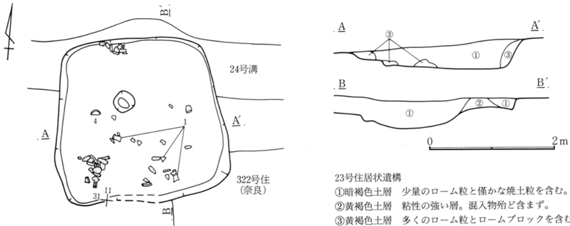
第567図 23号住居状遺構実測図
