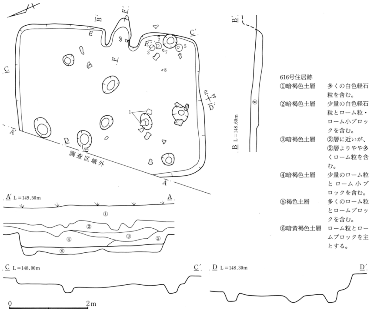
第424図 616号住居跡実測図
