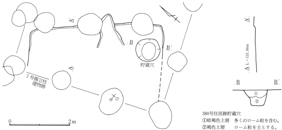
第287図 380号住居跡実測図
