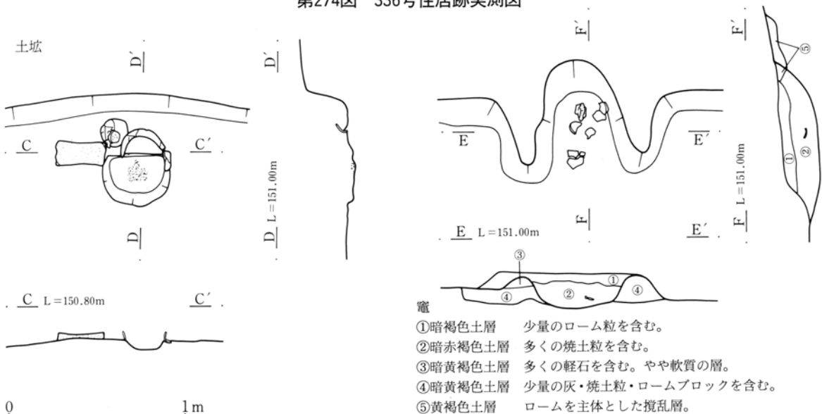
第275図 336号住居跡土塚・竈実測図
