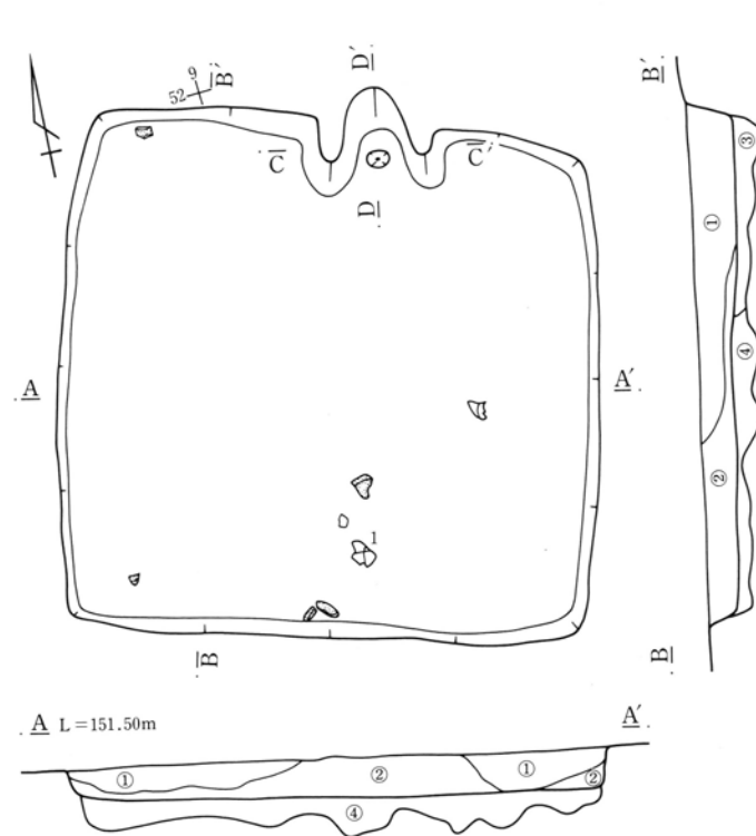
第401図 583号住居跡実測図
