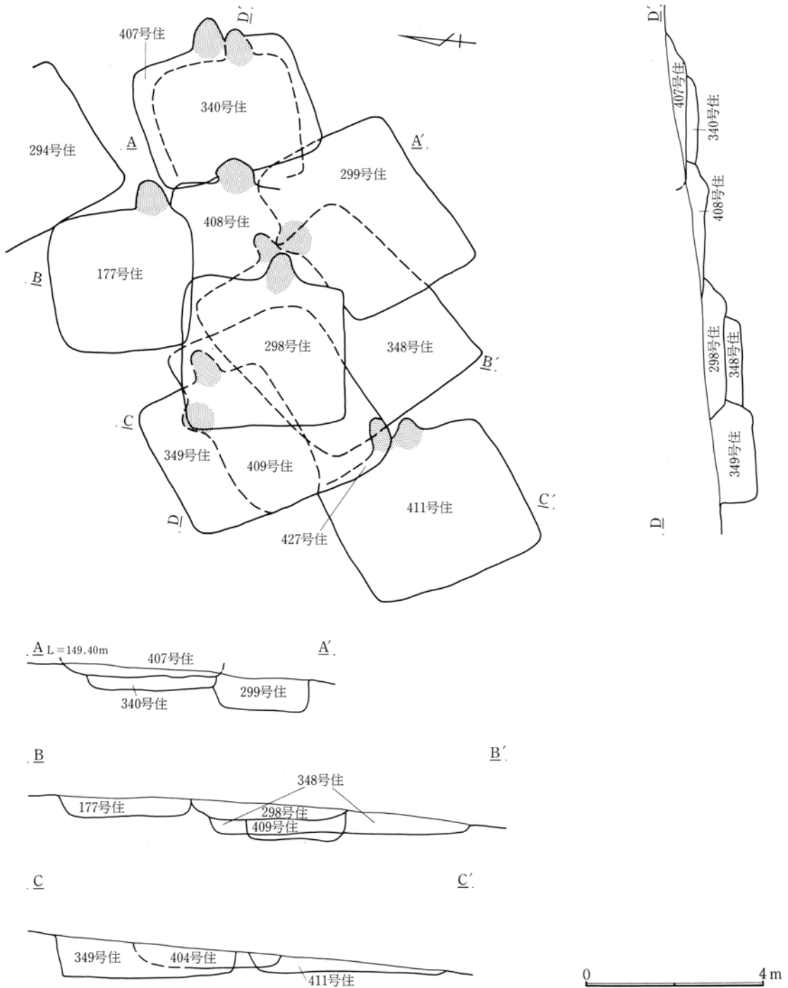
第261図 299号住居跡周辺遺構重複関係図
