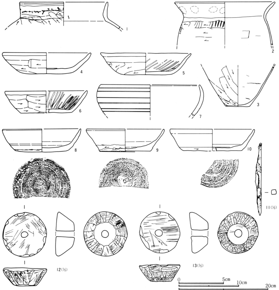
第378図 552号住居跡出土遺物実測図
