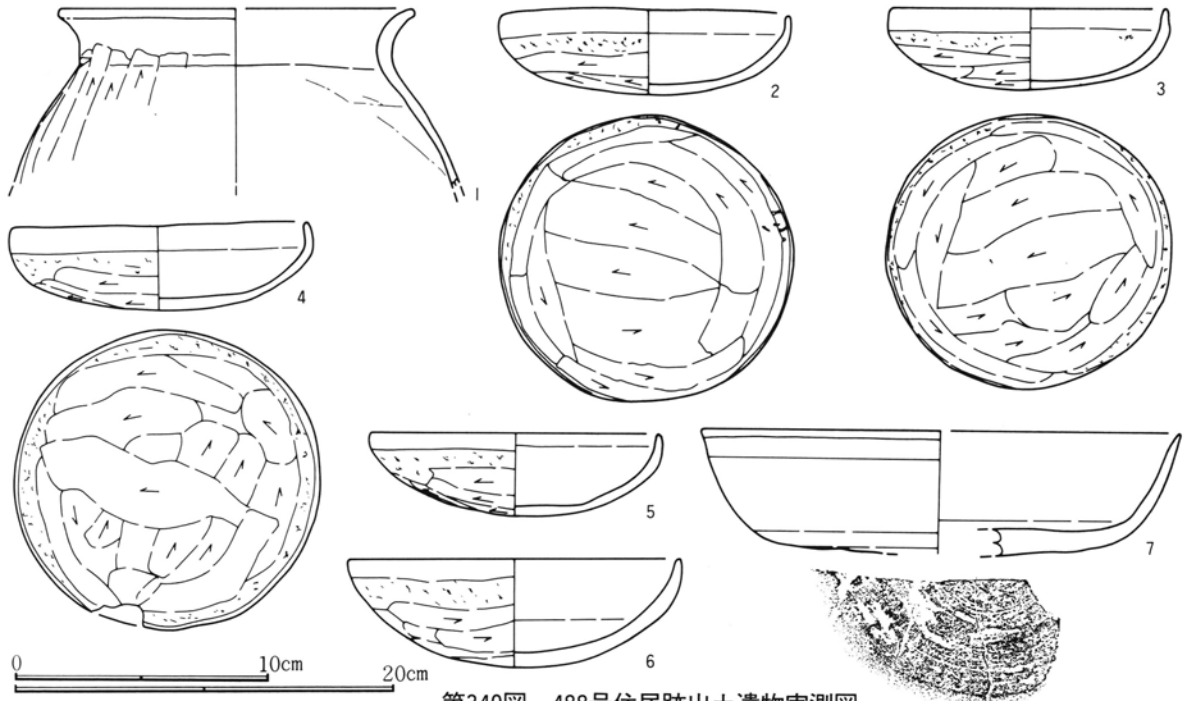
第340図 488号住居跡出土遺物実測図
