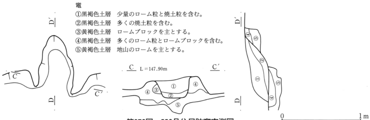
第372図 550号住居跡竈実測図
