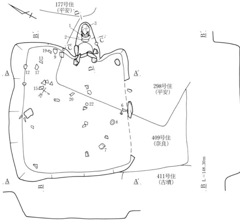
第279図 349号住居跡実測図
