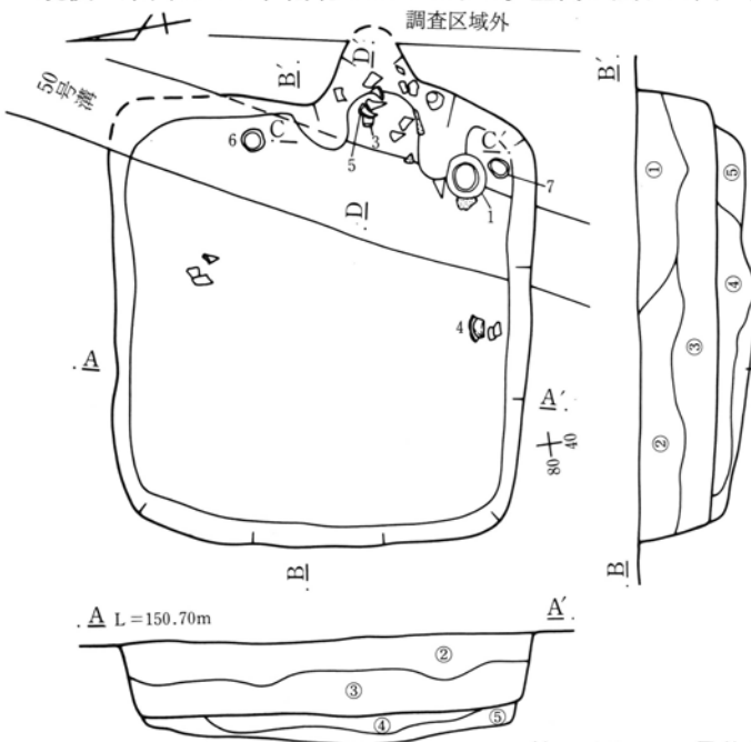
第398図 577号住居跡実測図
