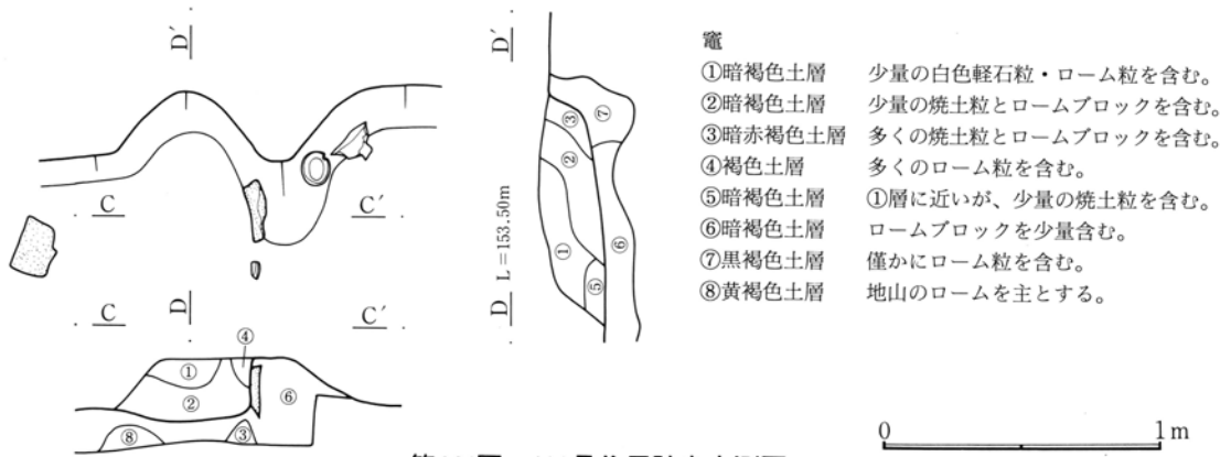
第444図 639号住居跡竈実測図
