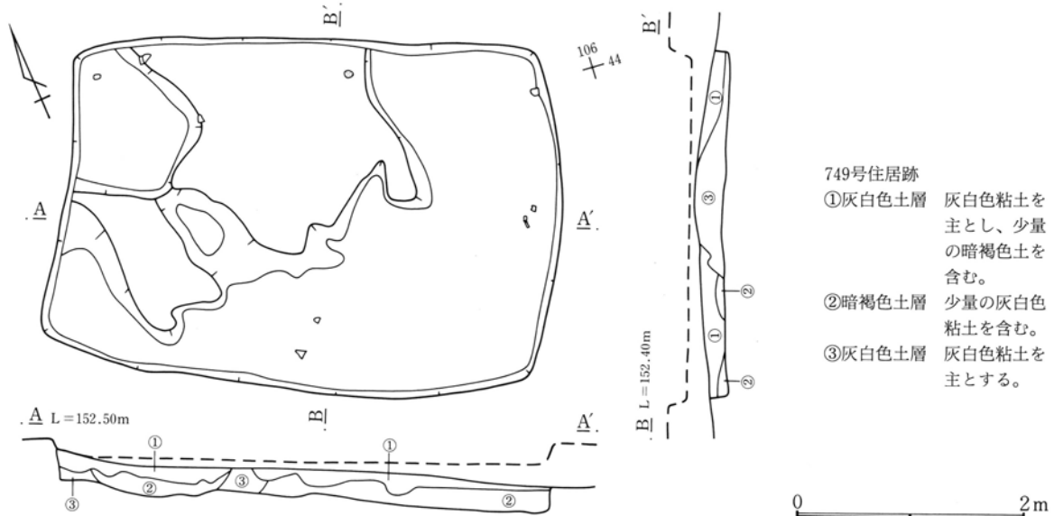
第509図 749号住居跡実測図
