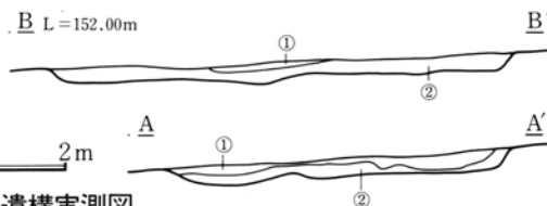
第560図 10号住居状遺構実測図
