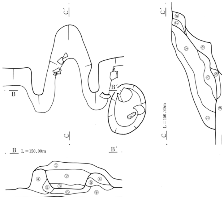
第415図 599号住居跡竈実測図
