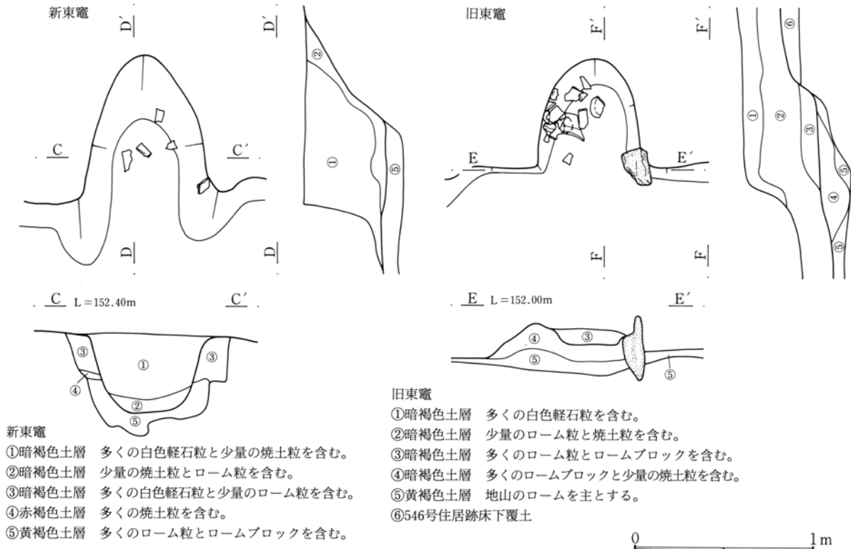
第366図 543号住居跡新東竈・旧東竈実測図
