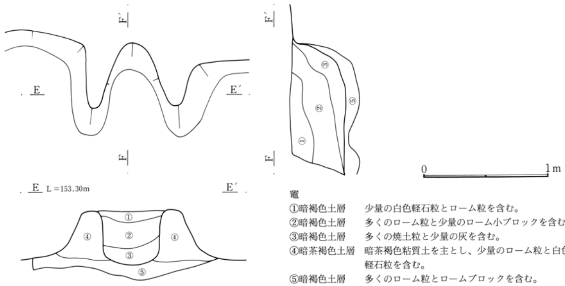
第347図 494号住居跡竈実測図
