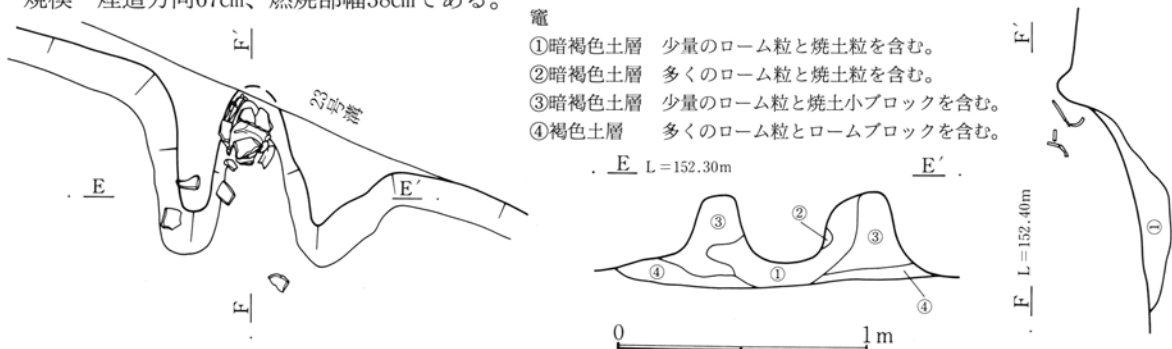
第269図 322号住居跡竈実測図
