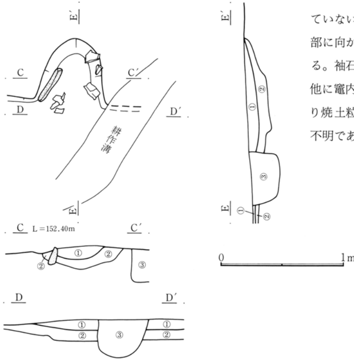
第525図 480号住居跡竈実測図
