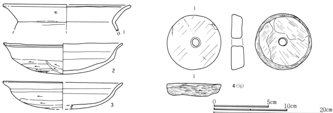
第491図 731号住居跡出土遺物実測図
