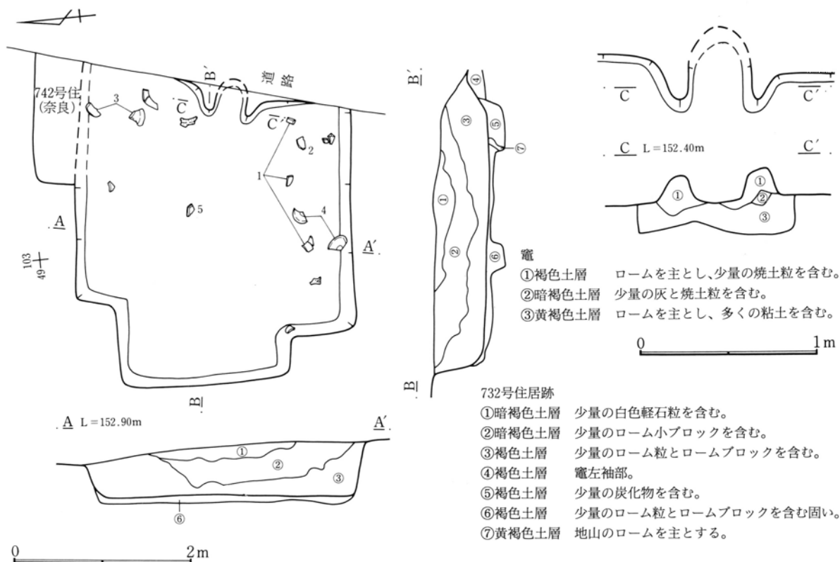
第492図 732号住居跡・竈実測図
