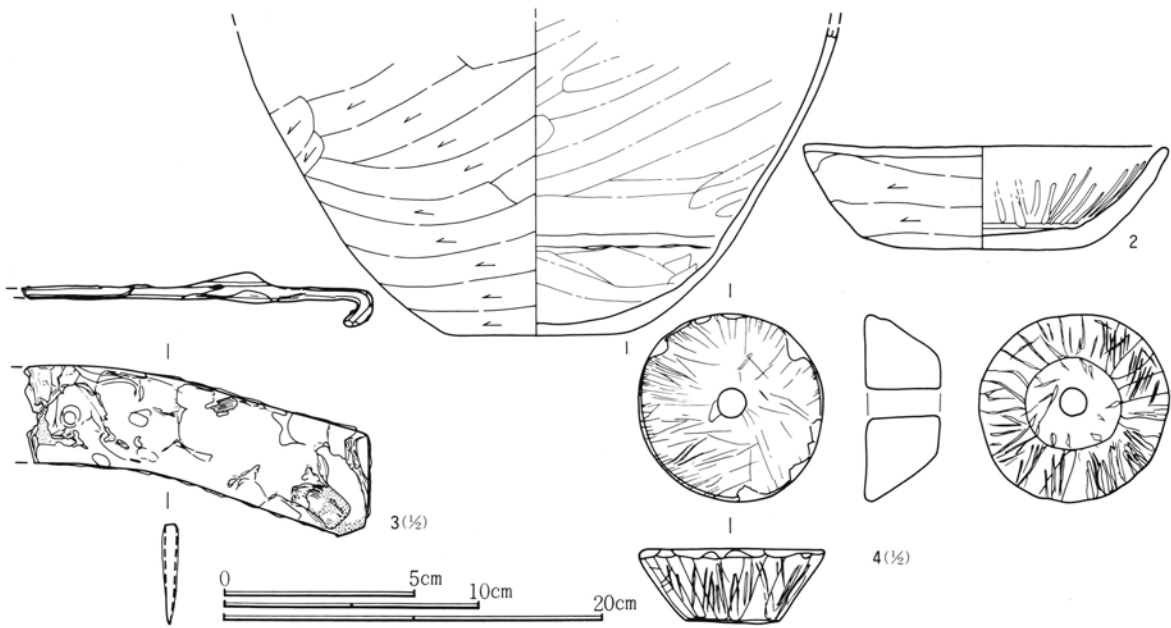
第352図 496号住居跡出土遺物実測図
