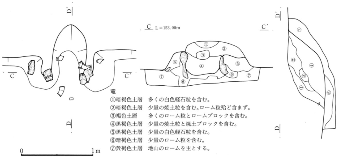
第360図 522号住居跡竈実測図
