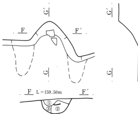
第462図 671号住居跡竈実測図
