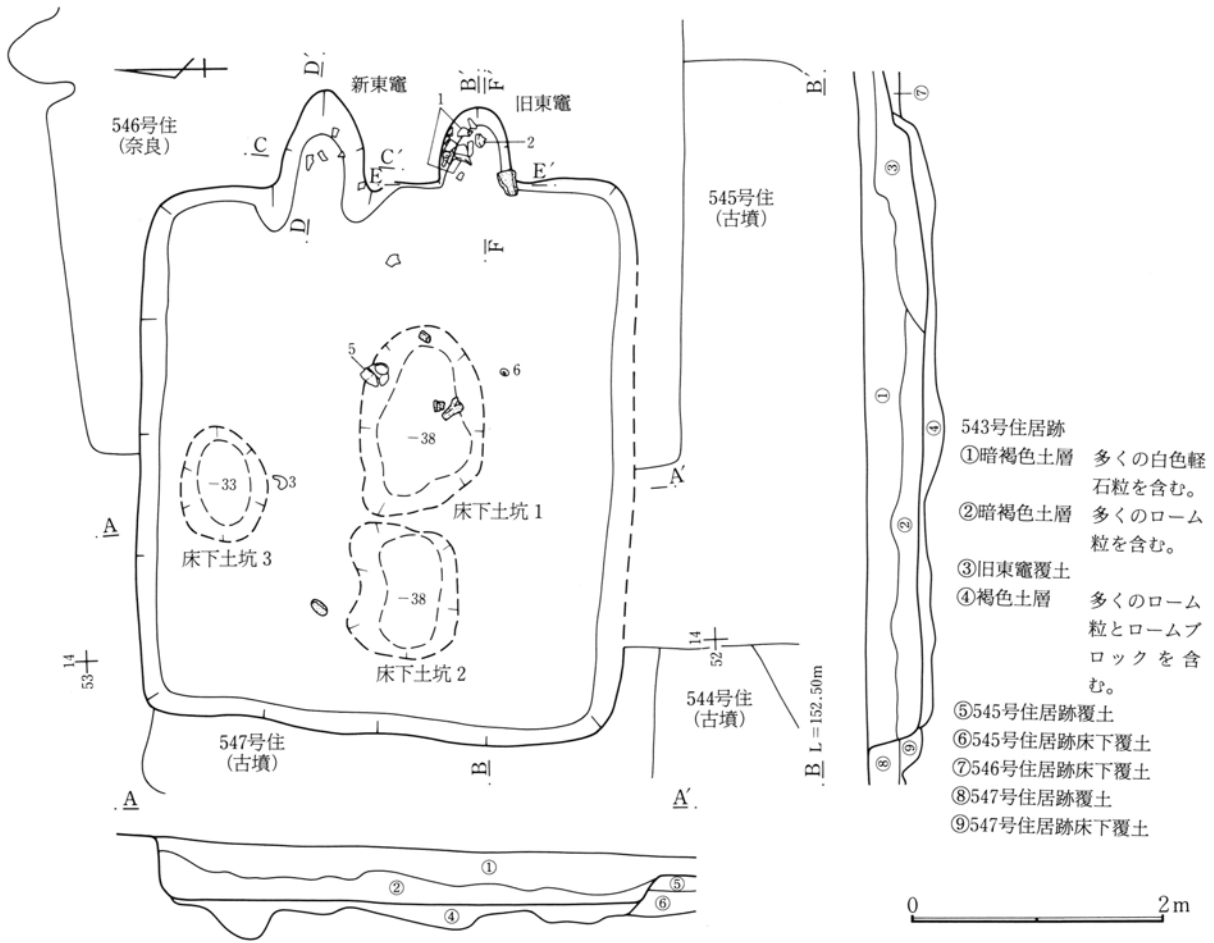
第365図 543号住居跡実測図
