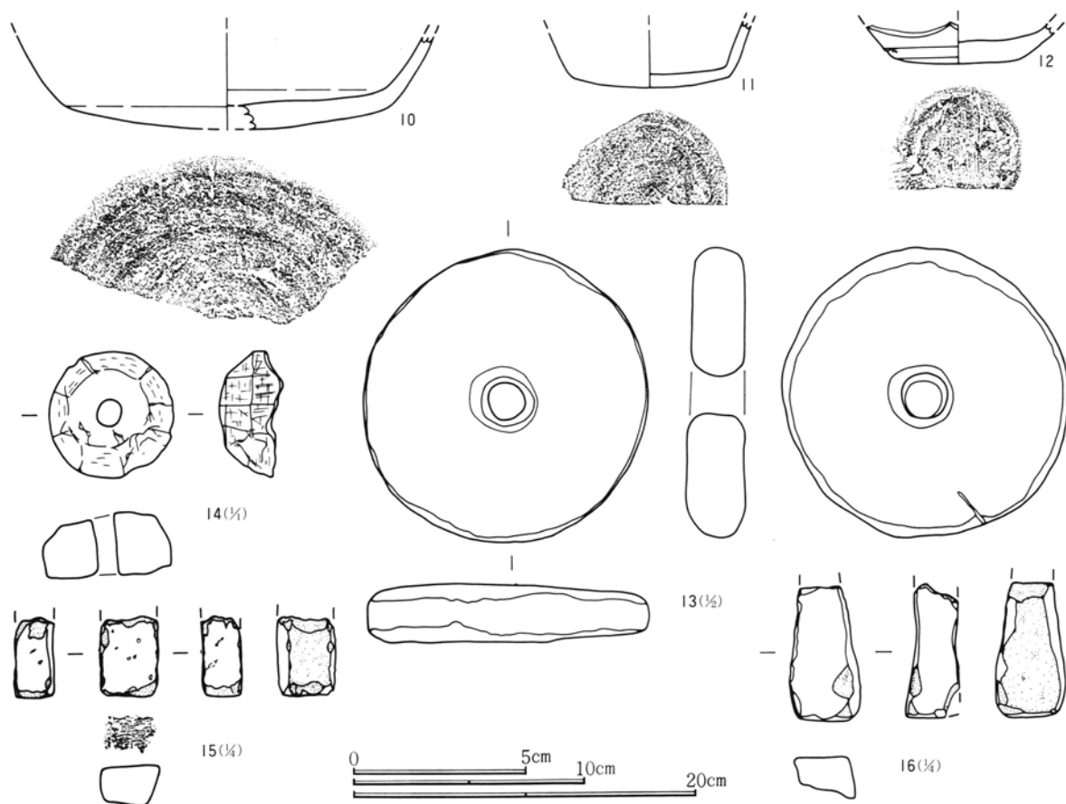
第330図 458号住居跡出土遺物実測図(2)
