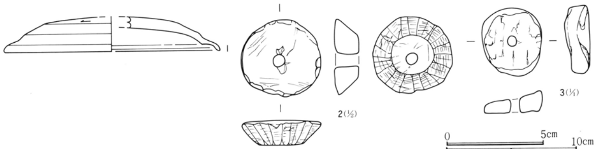
第337図 487号住居跡出土遺物実測図
