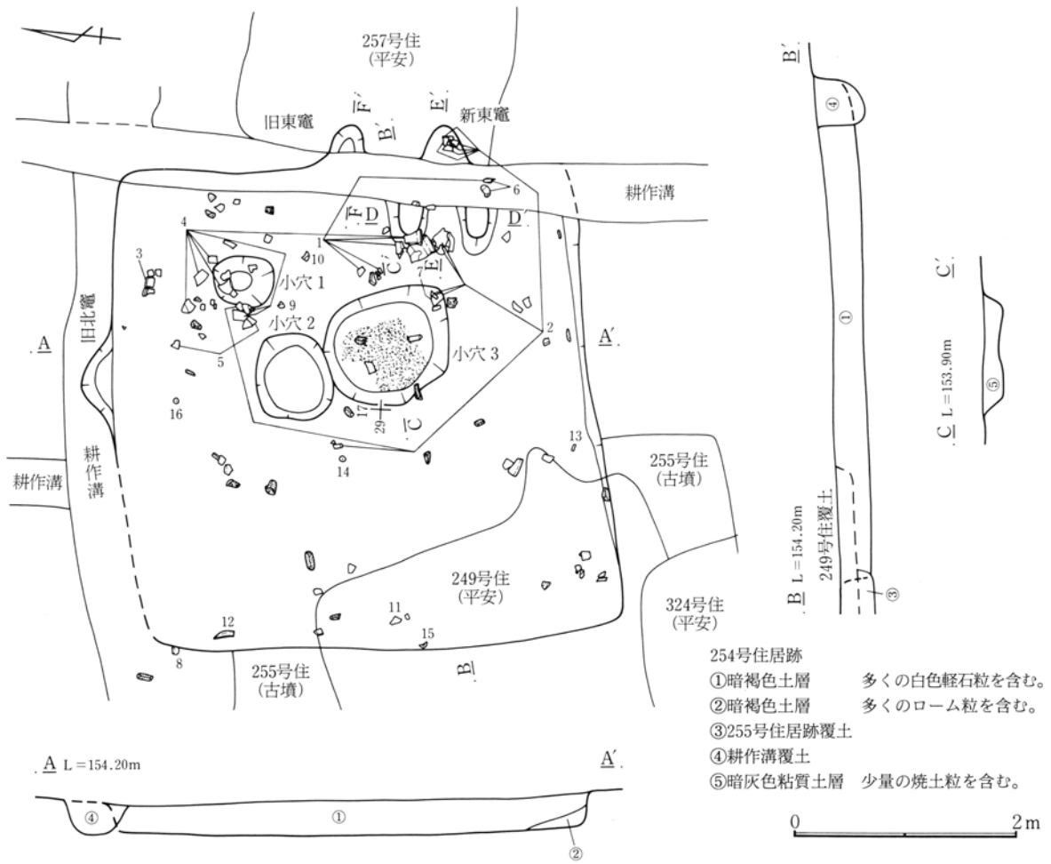
第253図 254号住居跡実測図
