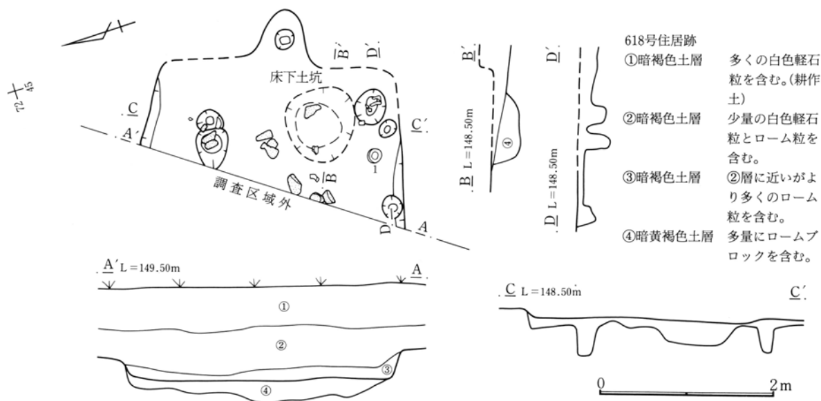
第430図 618号住居跡実測図
