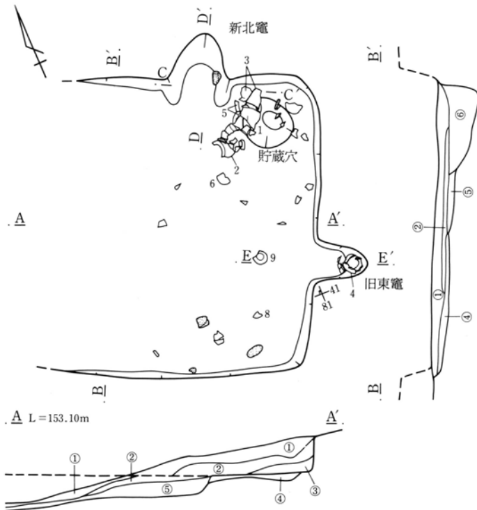
第472図 717号住居跡実測図
