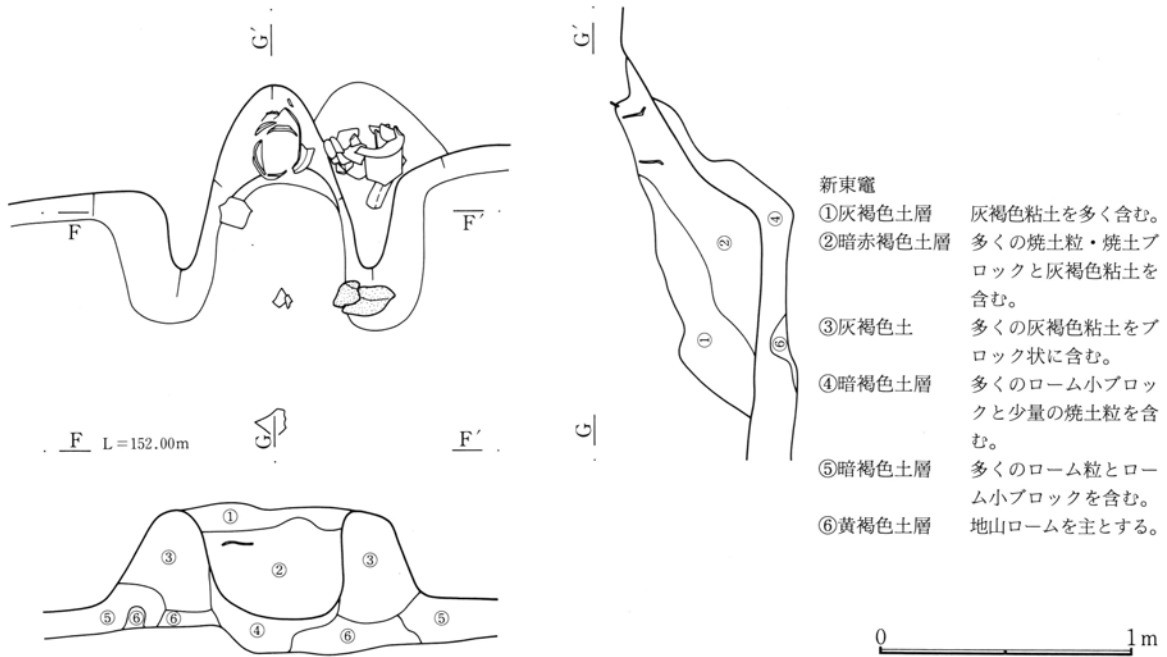
第436図 628号住居跡新東竈実測図
