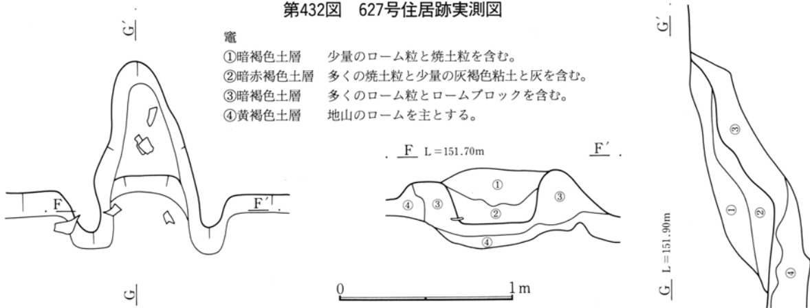
第433図 627号住居跡竈実測図
