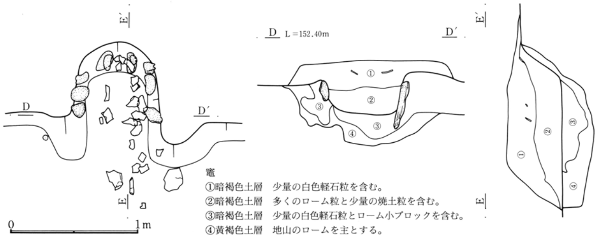
第377図 552号住居跡竈実測図
