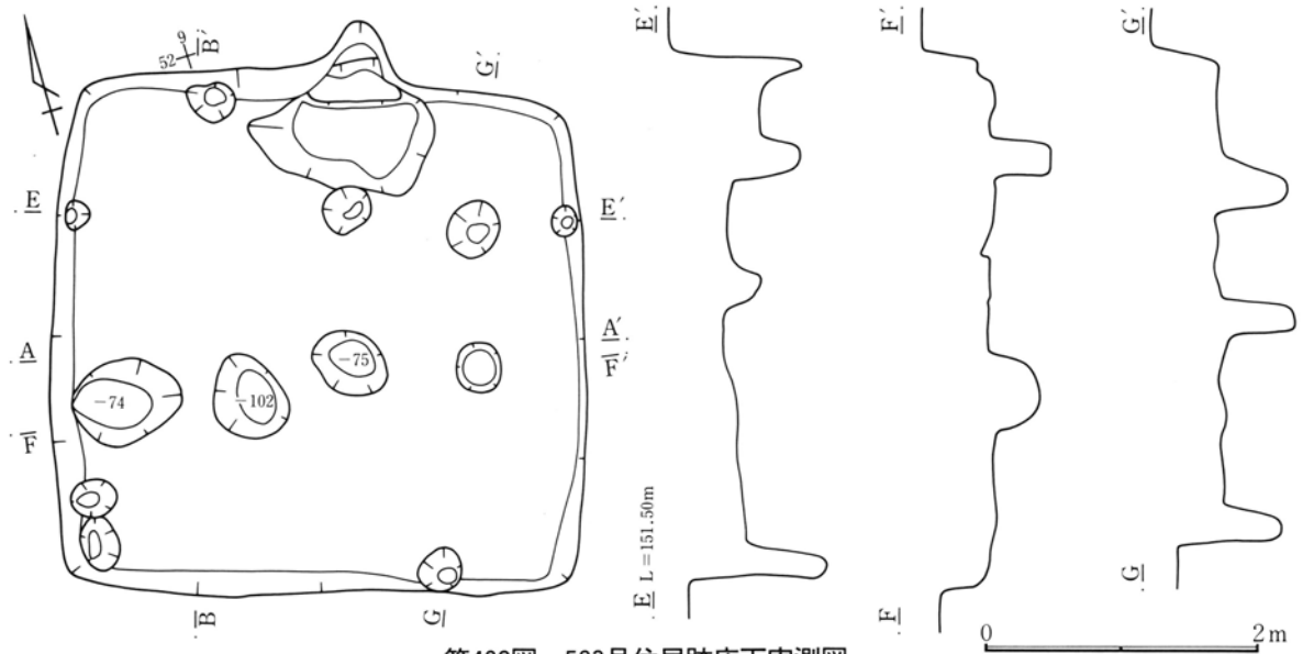
第402図 583号住居跡床下実測図
