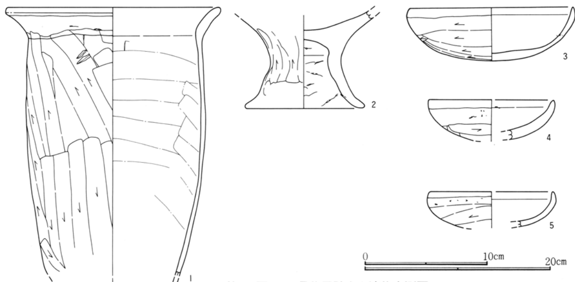
第358図 516号住居跡出土遺物実測図
