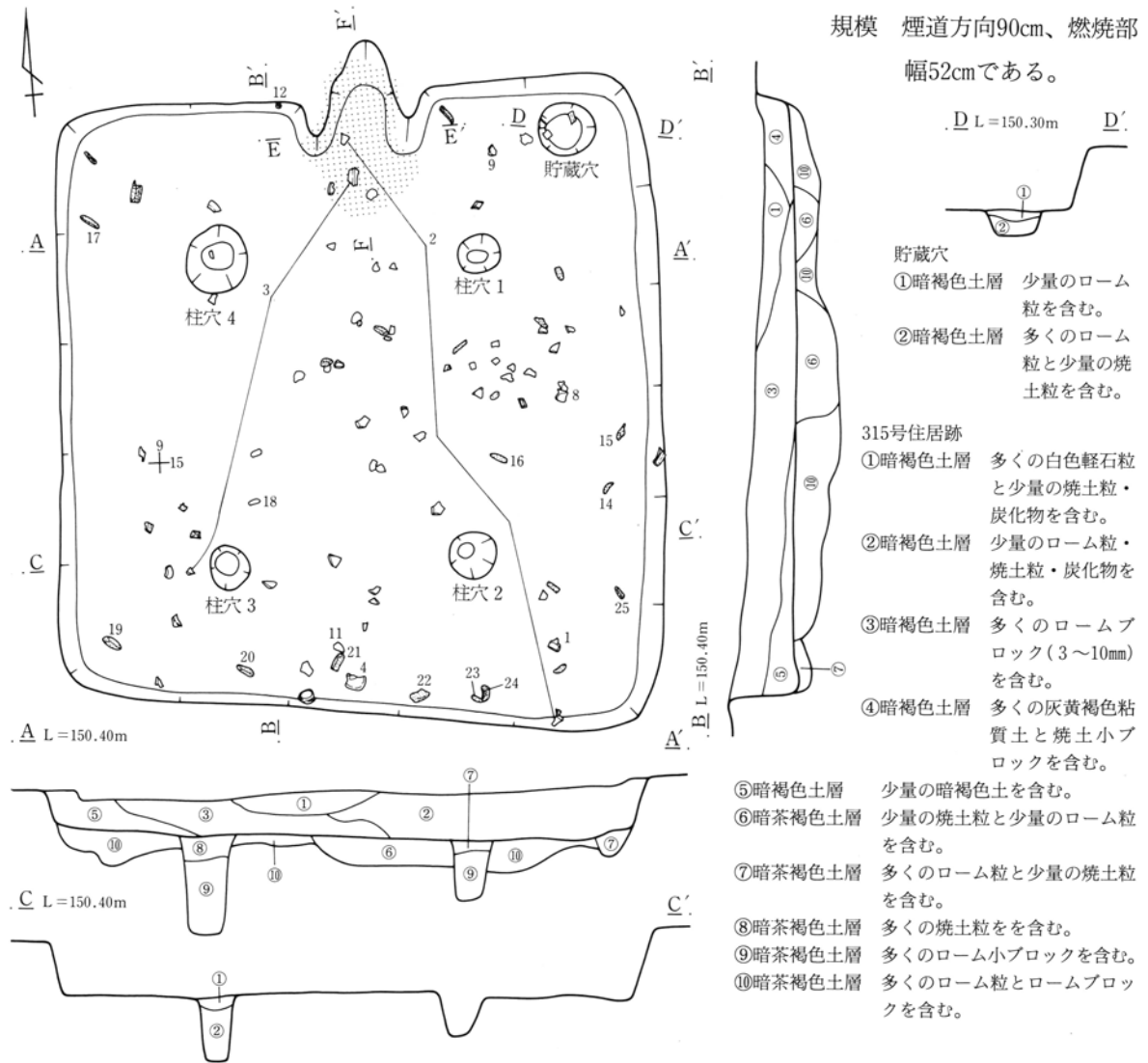
第263図 315号住居跡実測図
