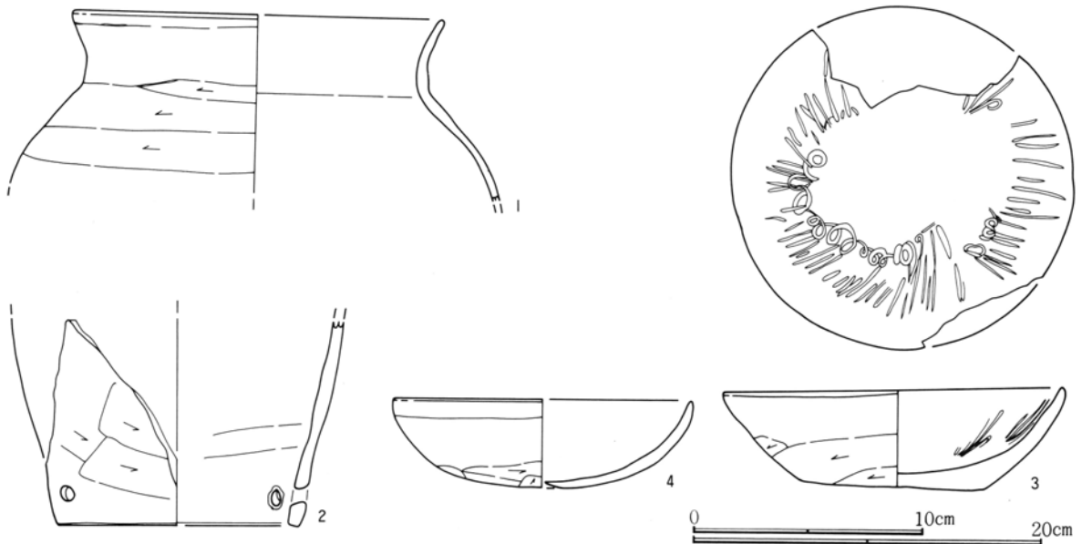
第487図 730号住居跡出土遺物実測図(1)
