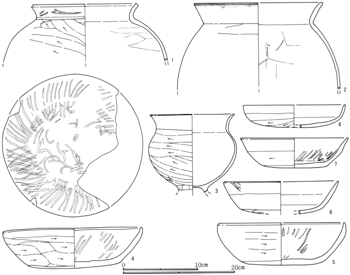
第482図 728号住居跡出土遺物実測図(1)
