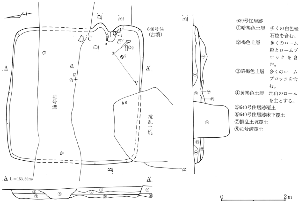
第443図 639号住居跡実測図
