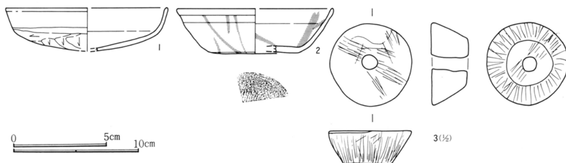
第381図 555号住居跡出土遺物実測図
