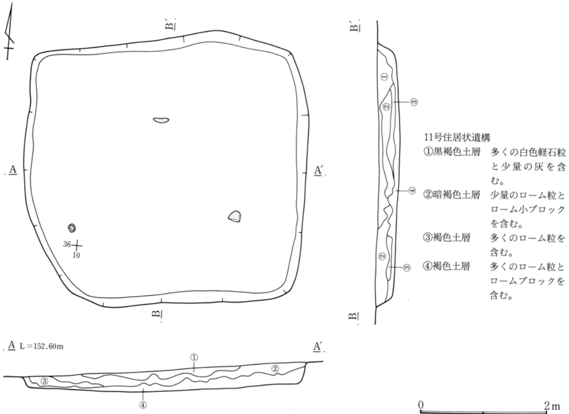
第561図 11号住居状遺構実測図
