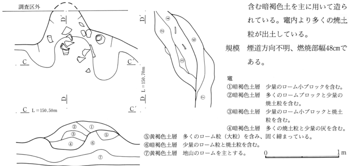
第399図 577号住居跡竈実測図
