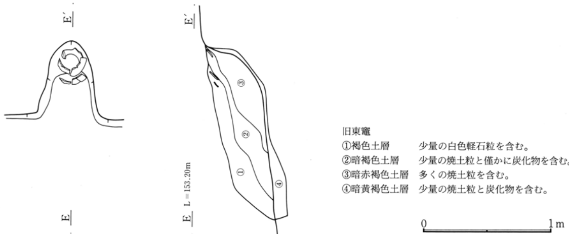
第475図 717号住居跡旧東竈実測図
