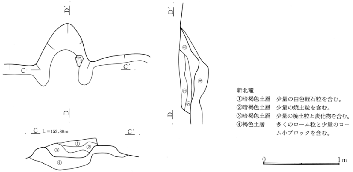
第474図 717号住居跡新北竈実測図
