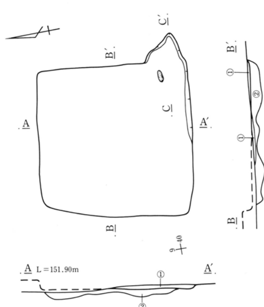
第314図 436号住居跡実測図
