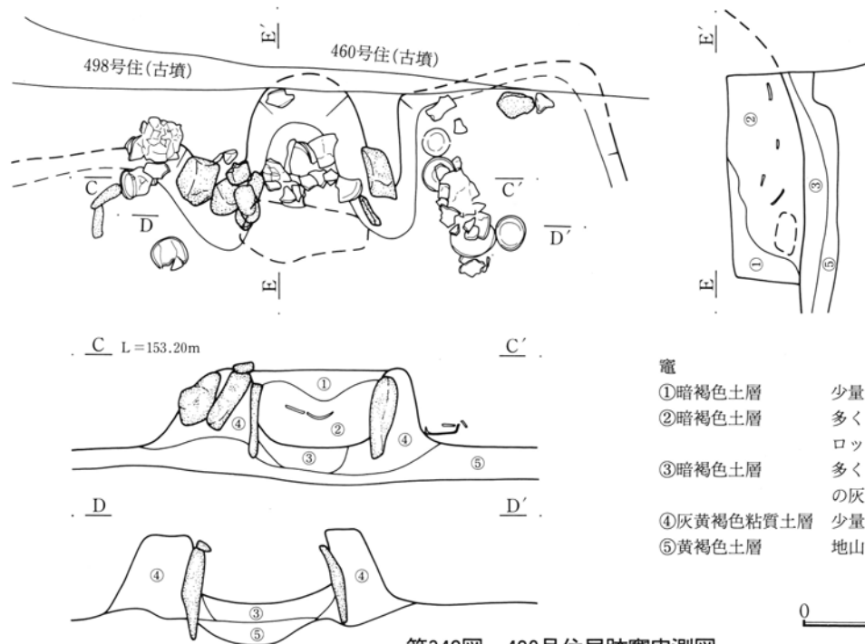
第342図 490号住居跡竈実測図
