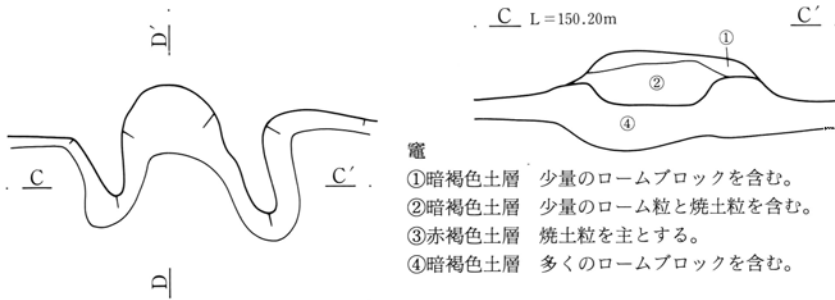
第413図 598号住居跡竈実測図
