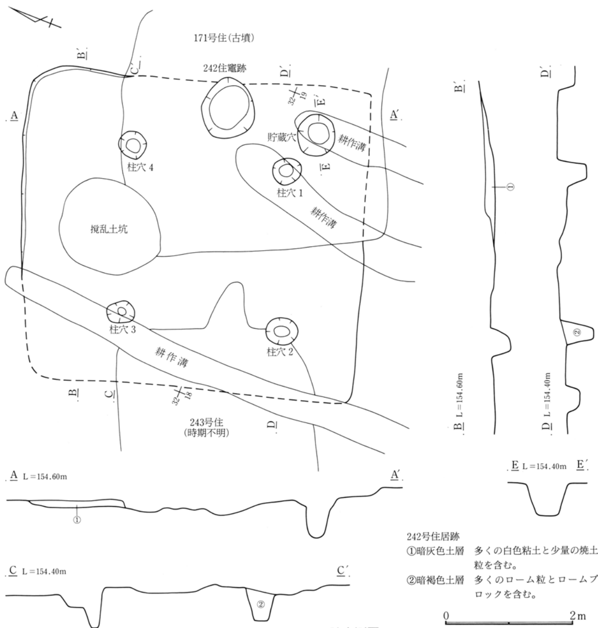
第541図 242号住居跡実測図
