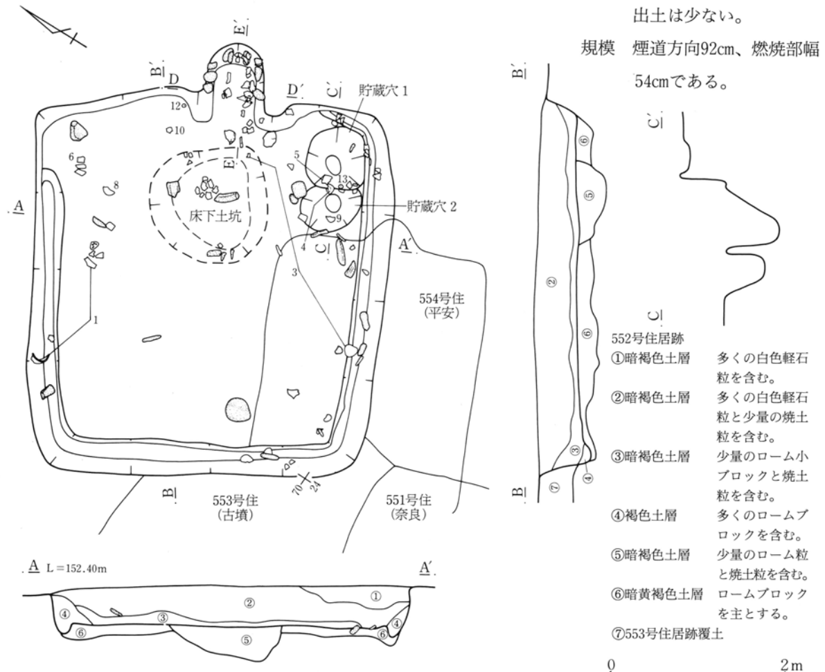
第376図 552号住居跡実測図
