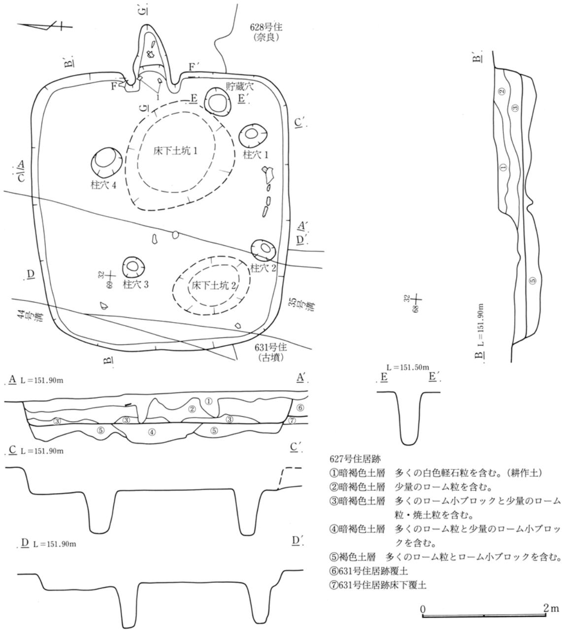
第432図 627号住居跡実測図
