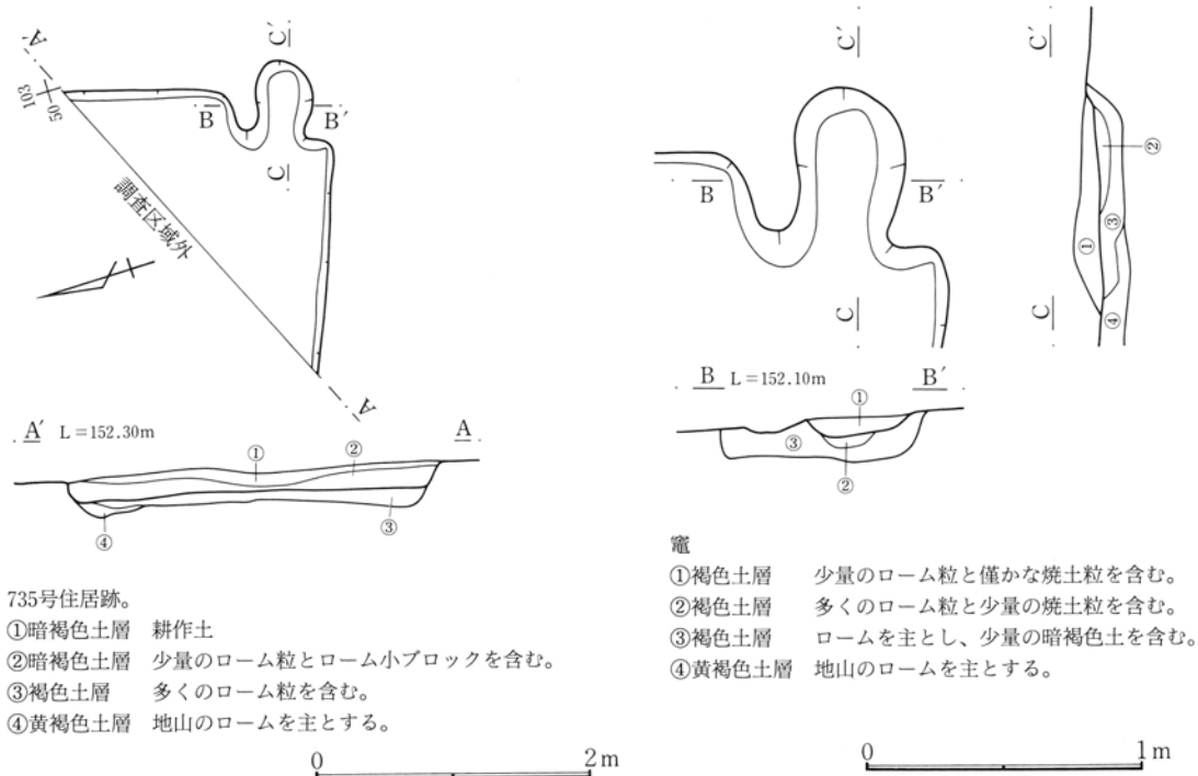
第550図 735号住居跡・竈実測図
