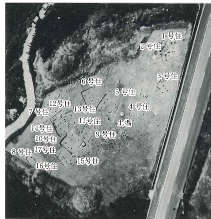
スキサキ遺跡遺構配置図
