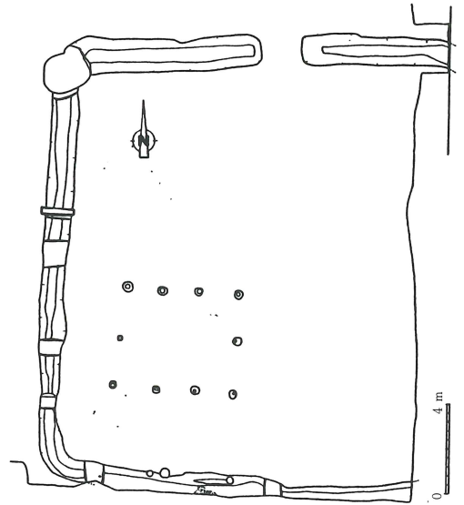
3号環濠居館跡平面図
