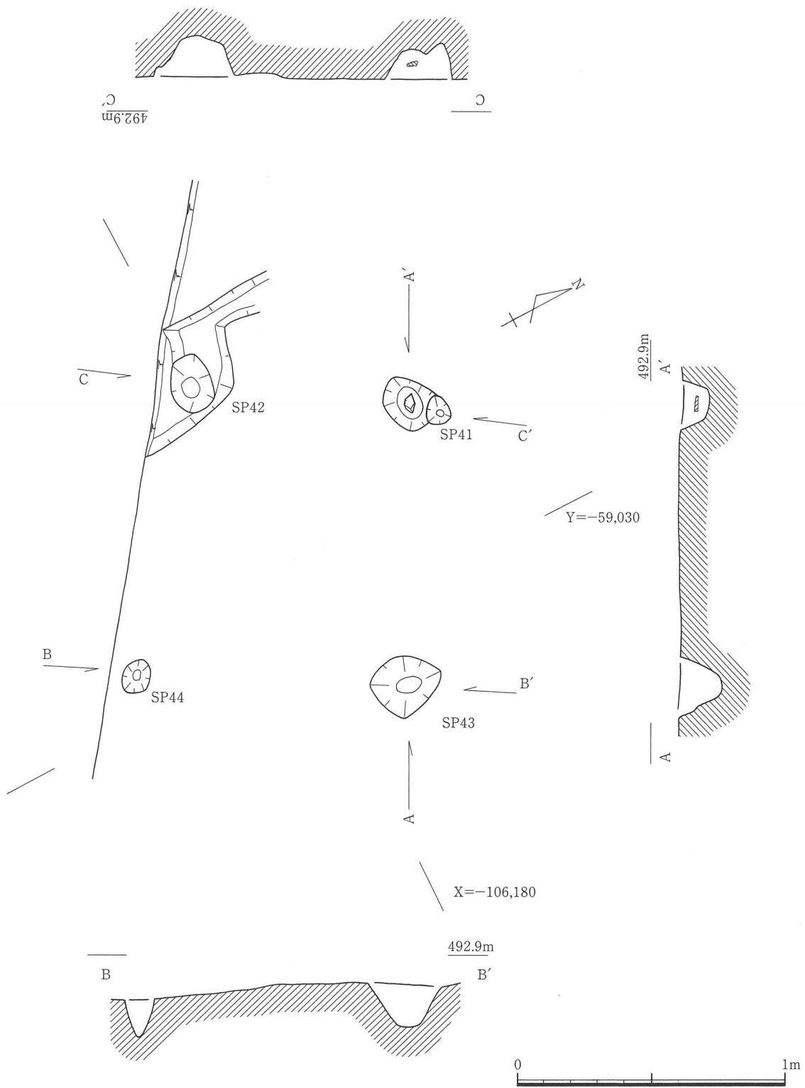
第6図 建物1平面・断面図
