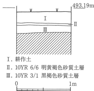
第16図 2区基本層序図
