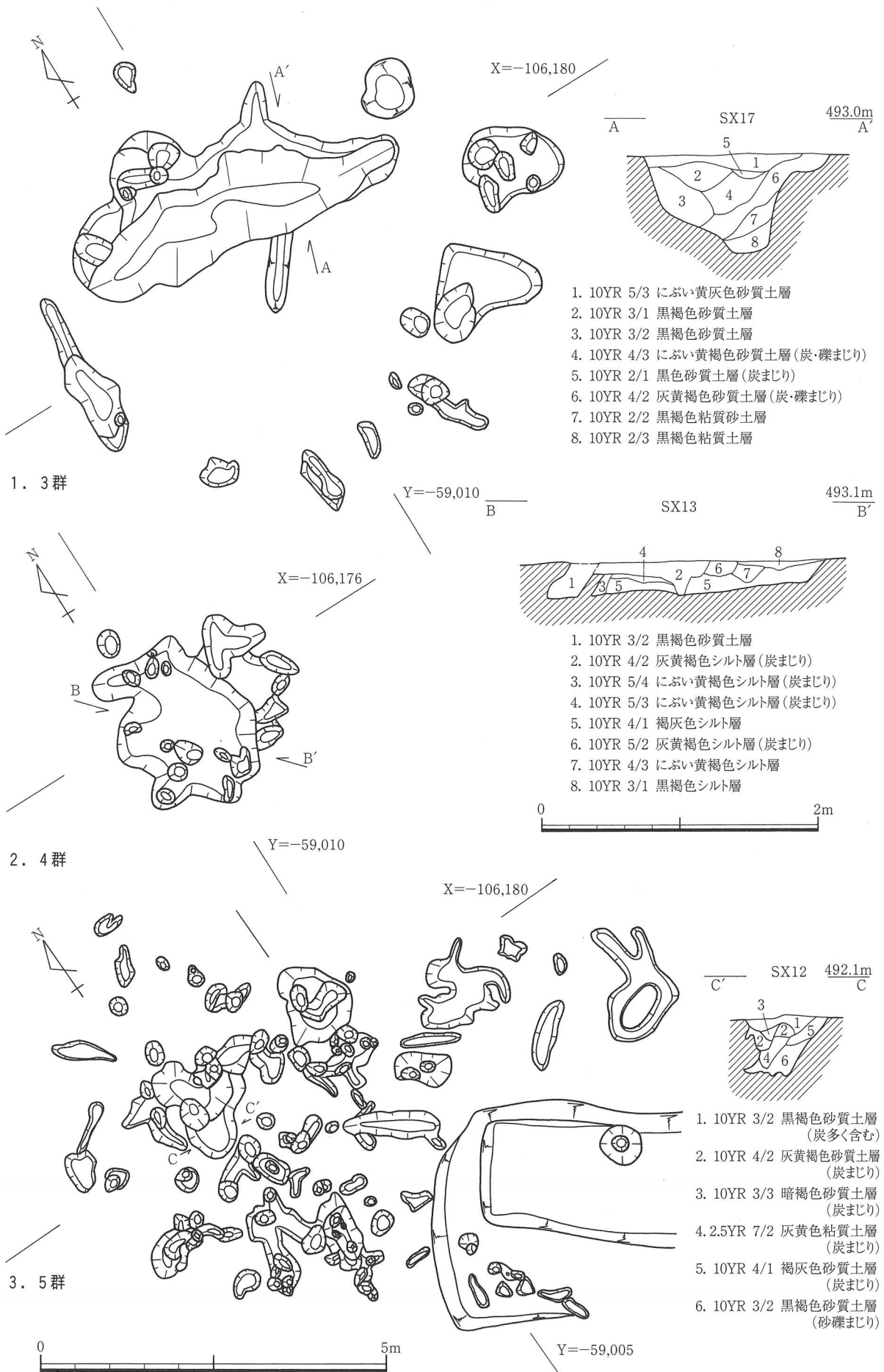
第11図 樹木根痕跡平面・断面図 2
