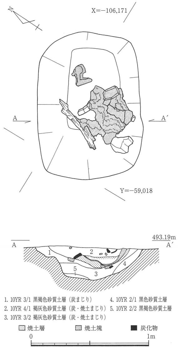
第8図 土坑14平面・断面図
