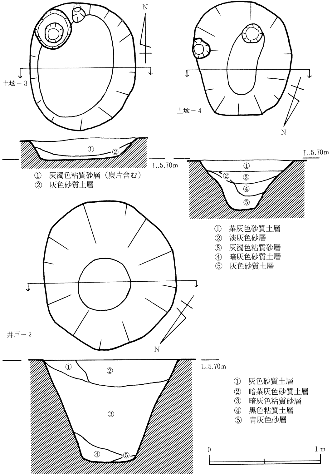
遺構セクション図
