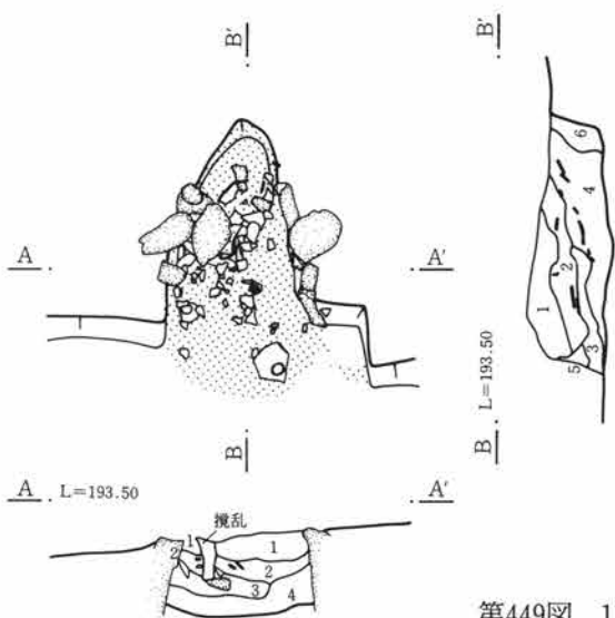
第449図 112号住居跡竈
