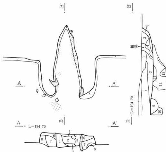
第188図 120号住居跡竈
