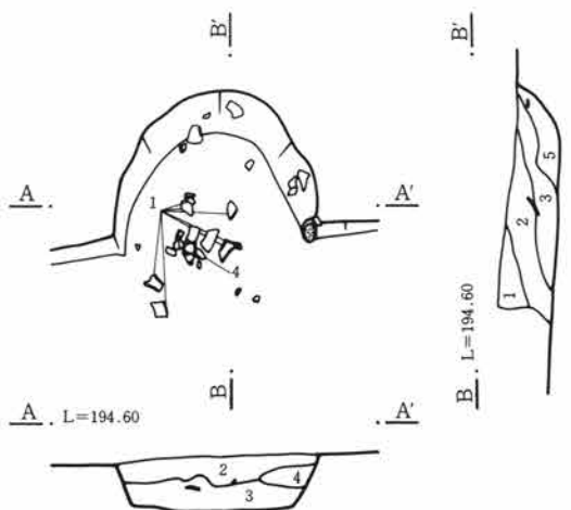
第470図 119号住居跡竈
