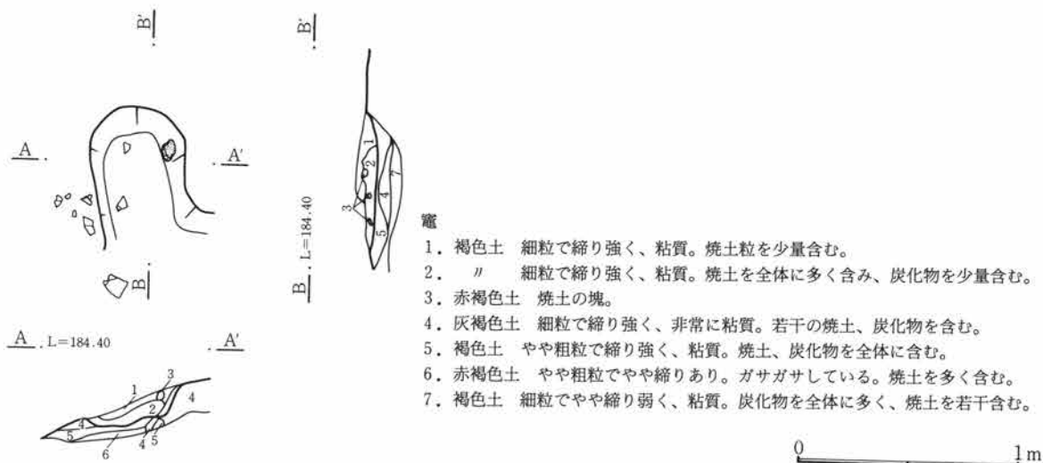
第505図 132号住居跡竈
