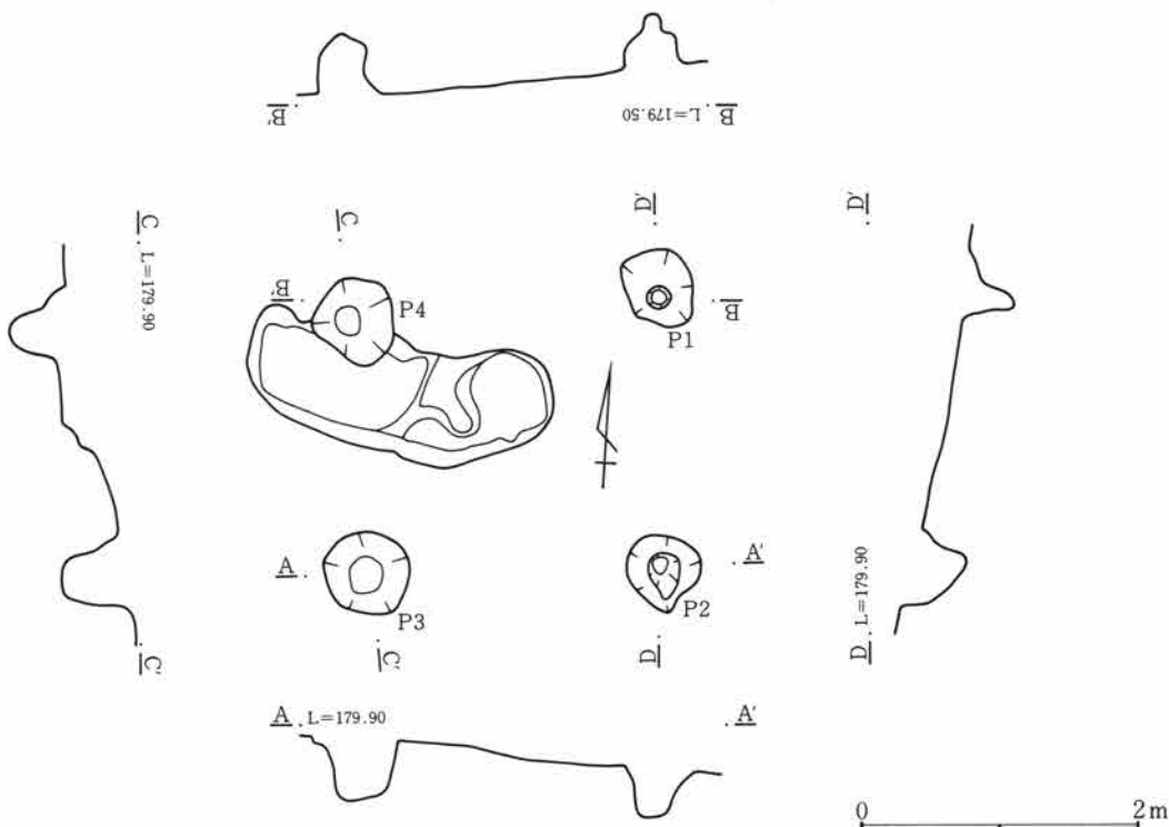
第632図 1号掘立柱建物跡
