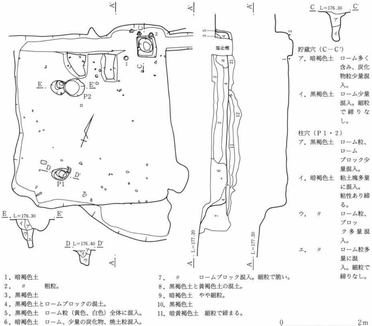
第118図 36号住居跡
