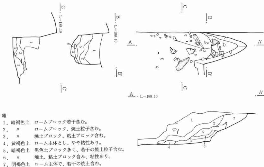
第220図 4号住居跡竈
