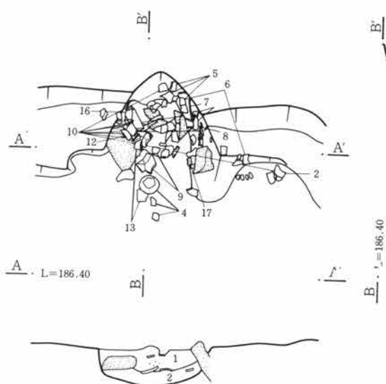
第249図 12号住居跡竈
