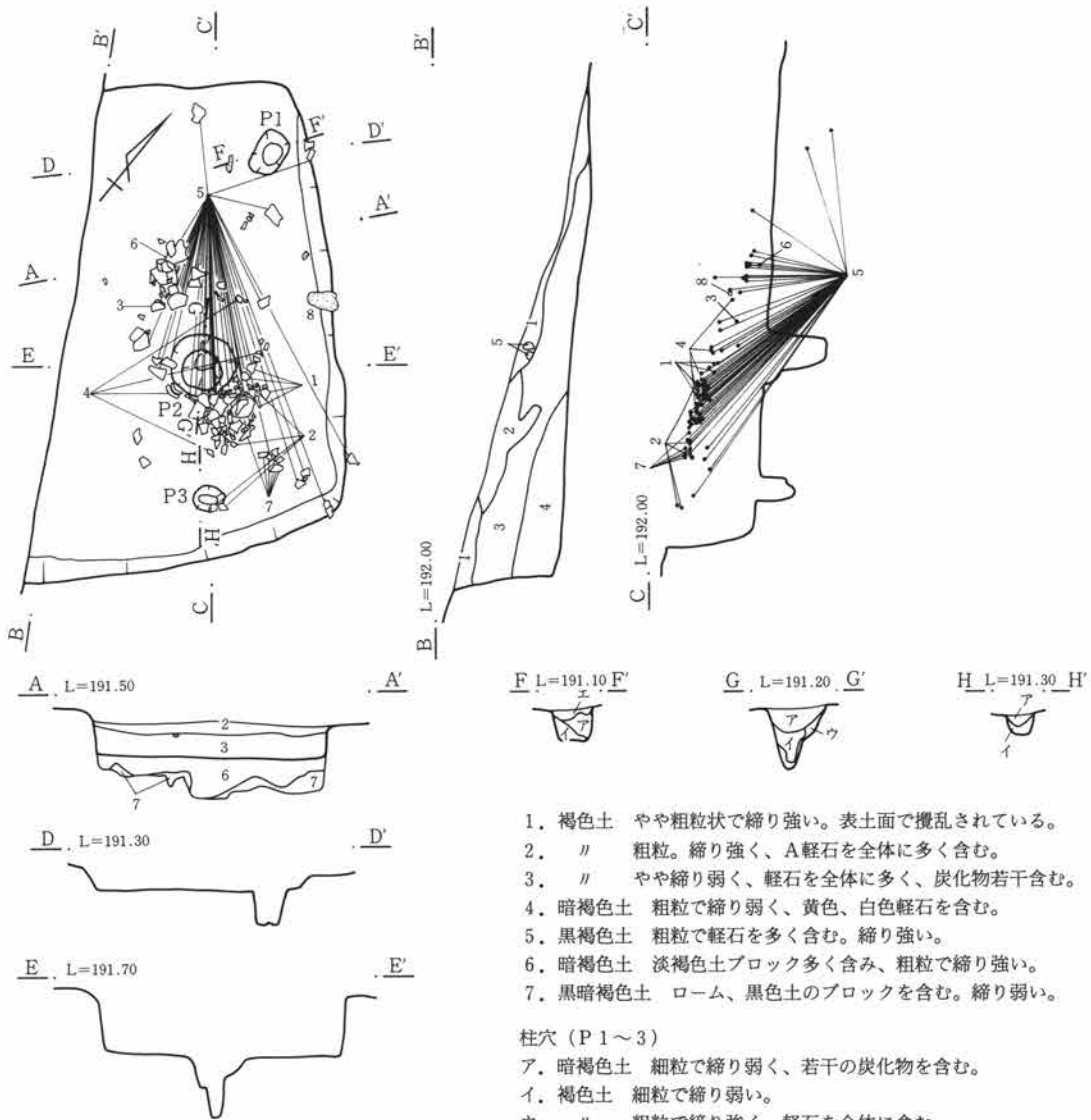
第475図 122号住居跡
