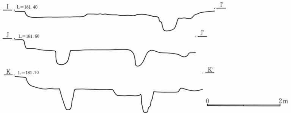
第380図 83号住居跡(2)
