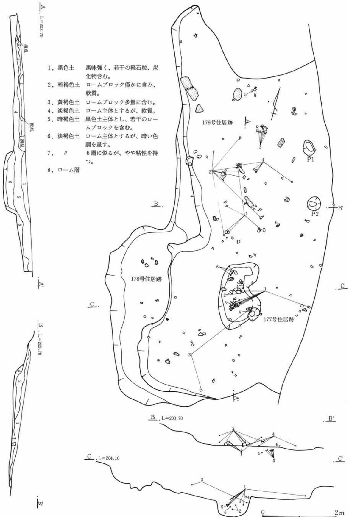
第613図 177~179号住居跡
