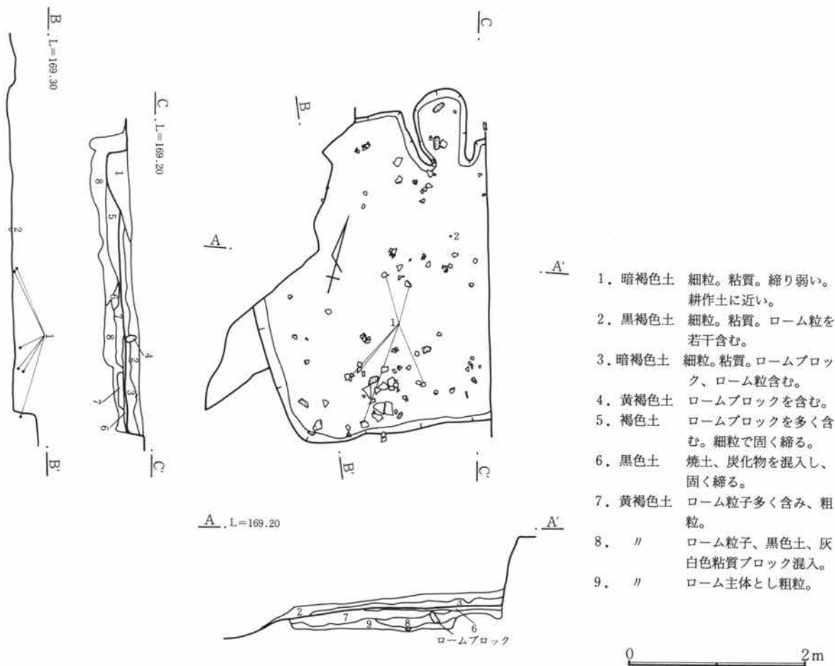
第581図 163号住居跡
