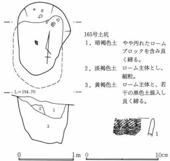
第61図 165号土坑及び出土遺物
