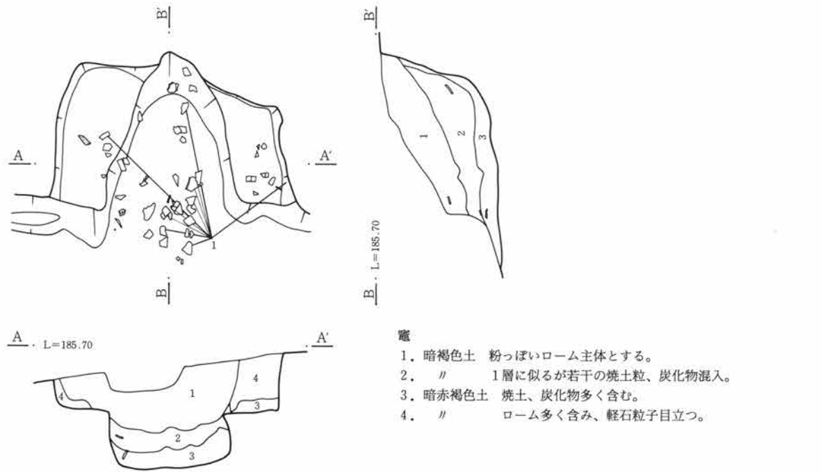
第253図 13号住居跡竈
