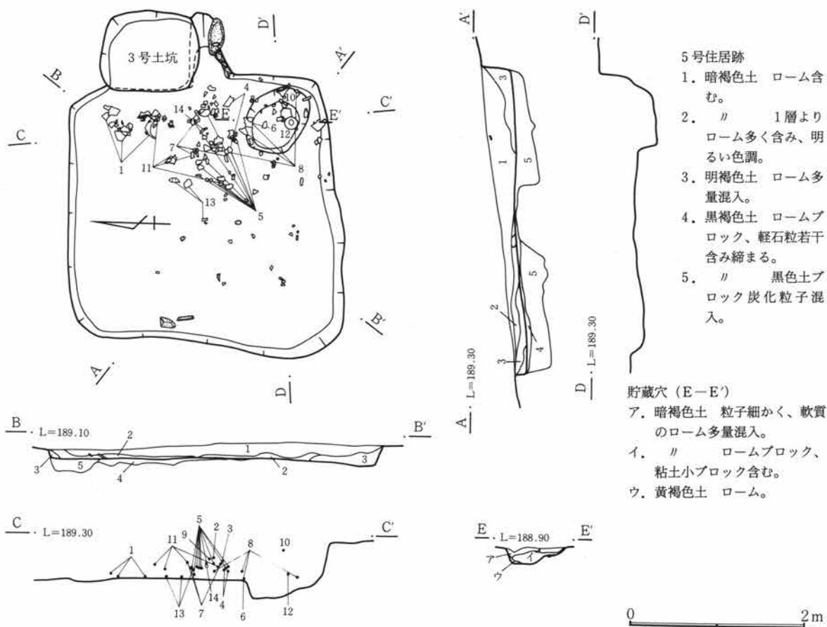
第222図 5号住居跡
