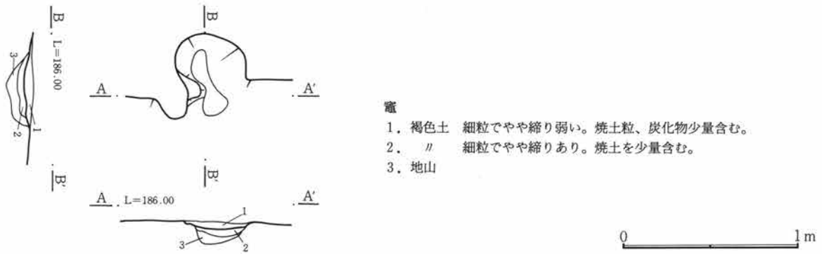
第493図 129号住居跡竈
