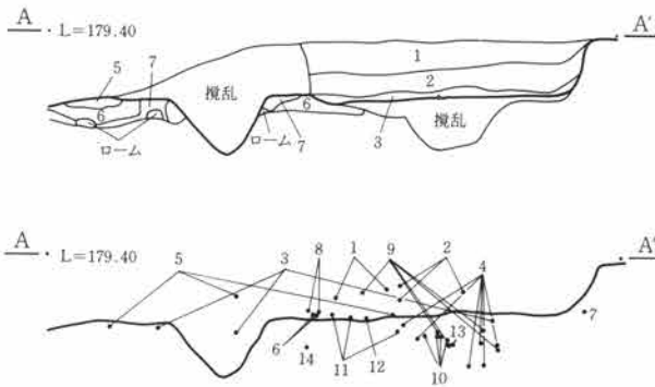
第319図 56号住居跡
