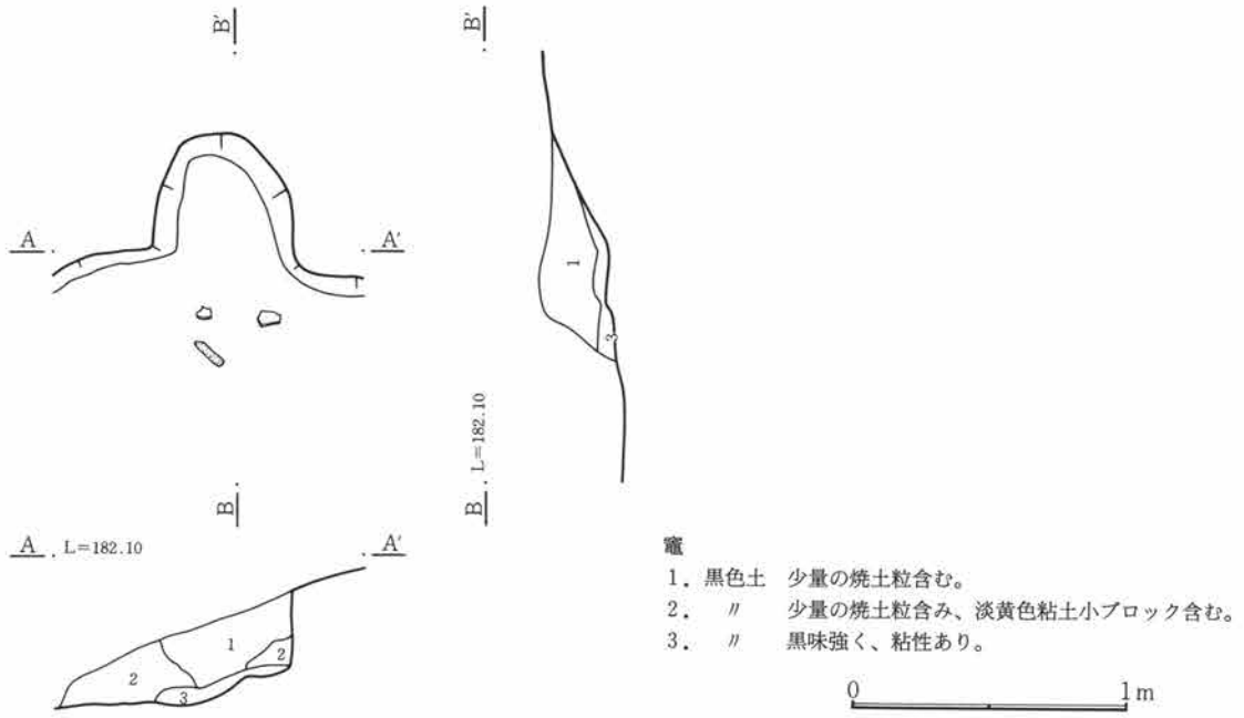
第433図 106号住居跡竈
