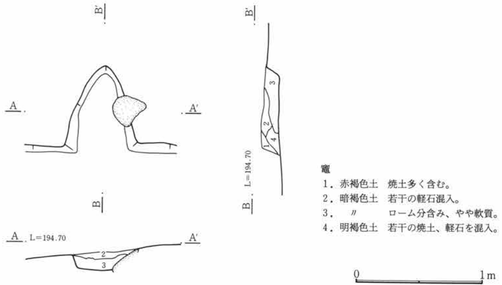
第441図 109号住居跡竈
