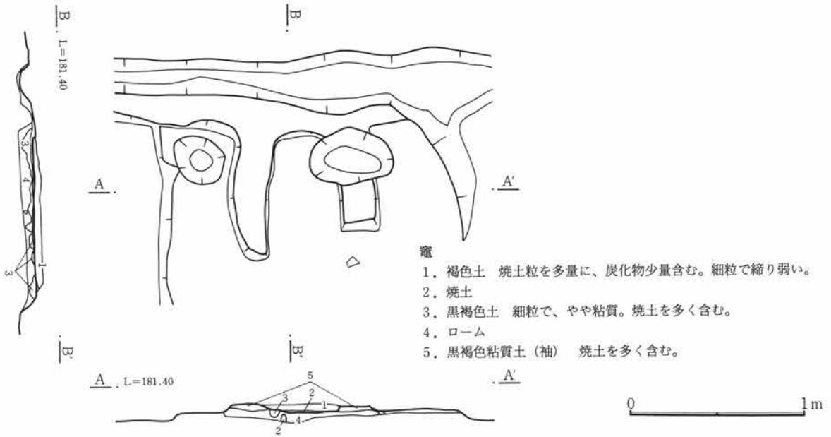
第381図 83号住居跡竈
