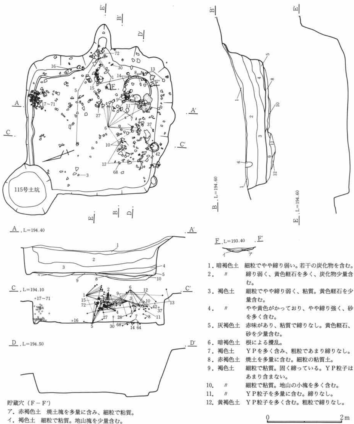
第499図 131号住居跡
