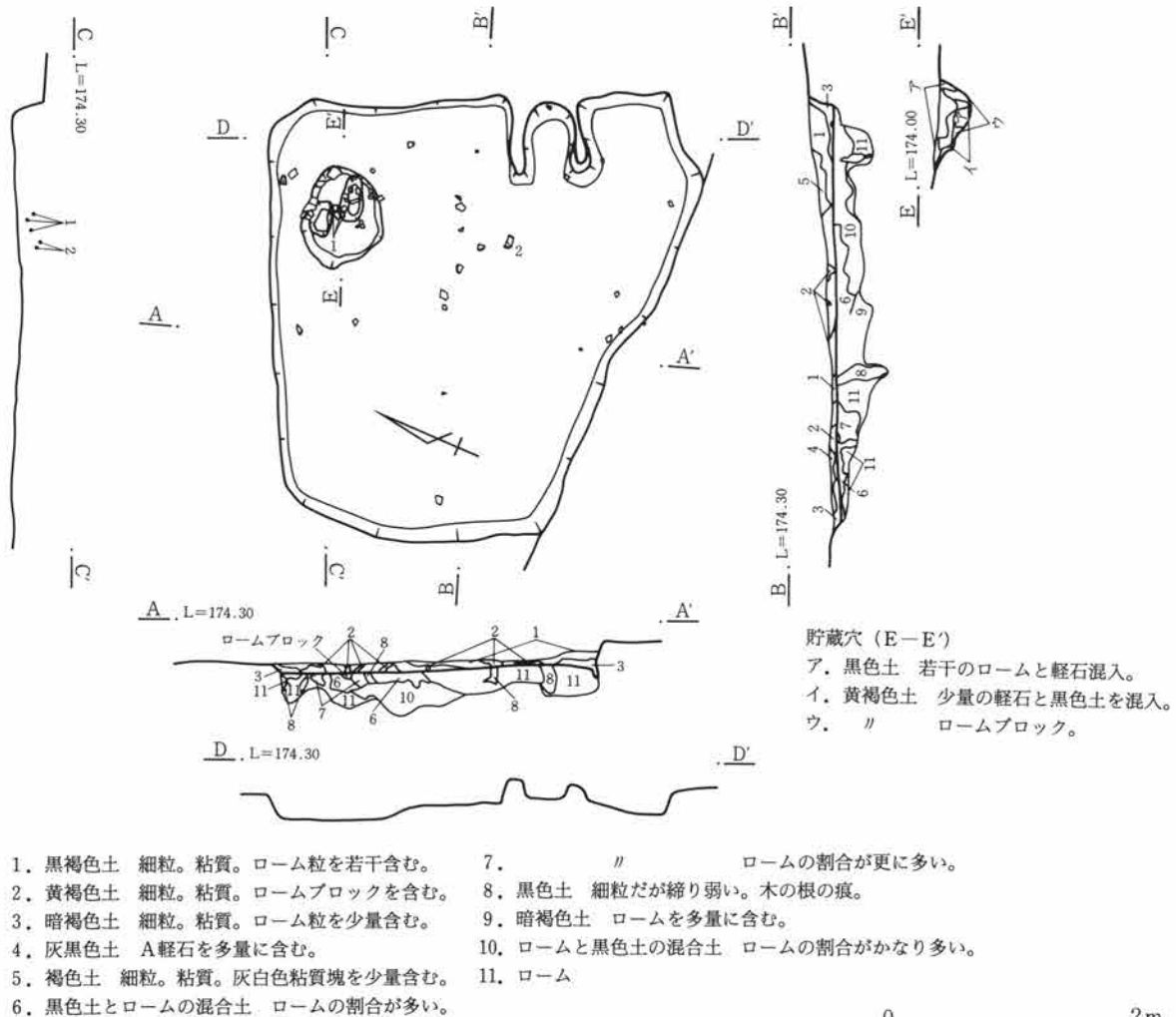
第574図 160号住居跡
