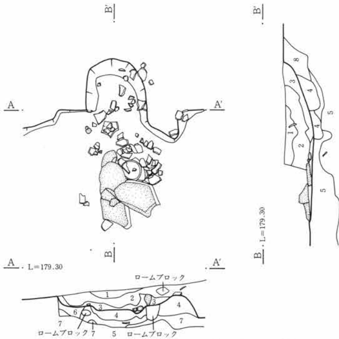
第305図 47号住居跡竈
