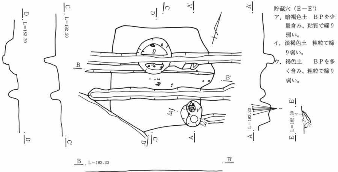
第414図 99号住居跡
