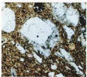
7. 樽式土器 累帯構造を示す斜長石(中央)のまわりに基質との反応縁がみられる
