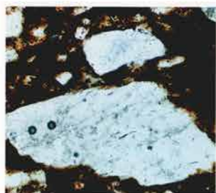
1. 二軒屋式土器 パーサイト構造のカリ長石(下)と斜長石
