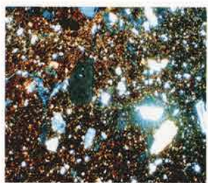
5. 赤井戸式土器 斜方輝石、斜長石および単結晶石英の破片、基質多い
