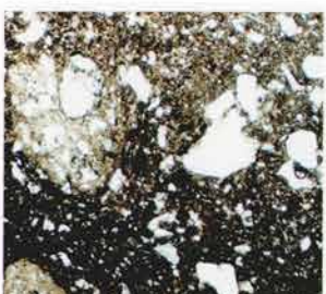
10. 石田川式土器 土器片(左)と累帯構造の斜長石(右)
