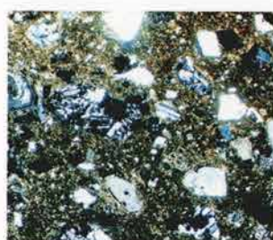
8. 樽式土器 累帯構造を示す斜長石、火山岩片
