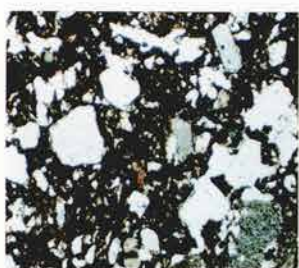
6. 赤井戸式土器 斜方輝石(中央)、火山砂岩(右下)、文象構造を示す石英
