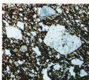
4. 赤井戸式土器 斜方輝石(上)と砂岩の岩片(右)および破片状の斜長石
