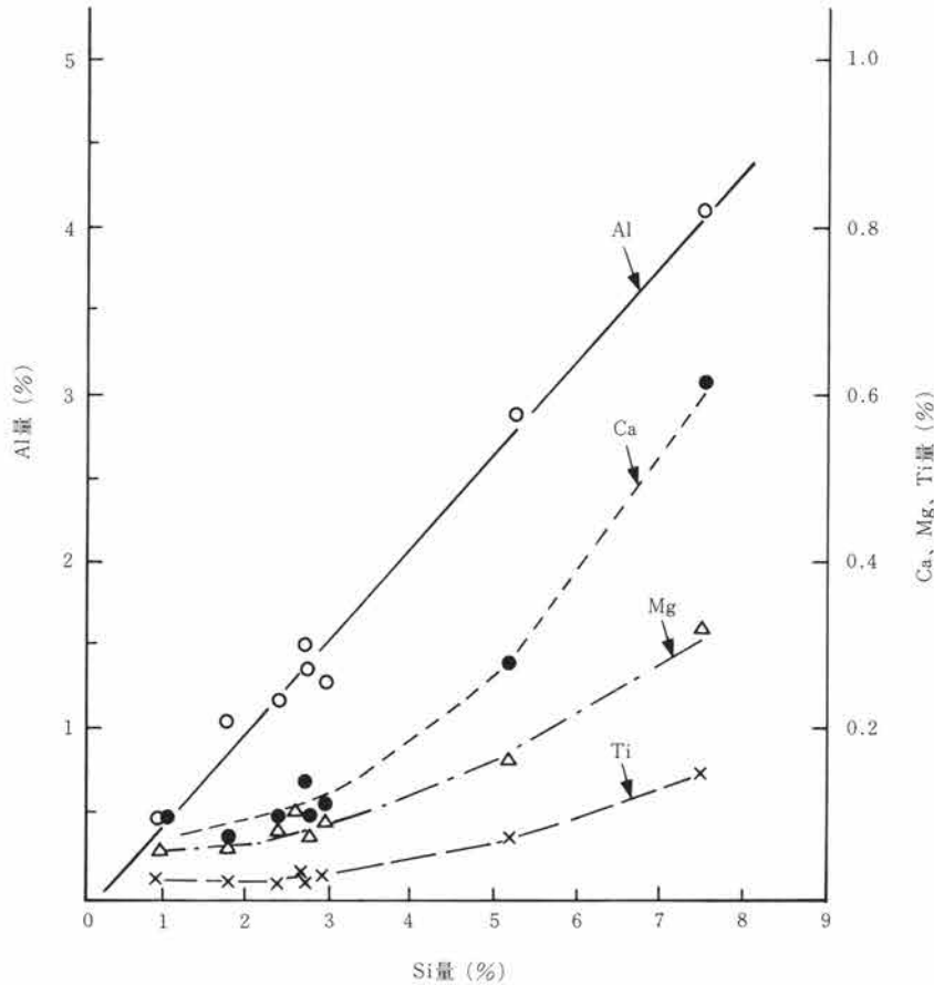
第395図 Si量に対するAl、Ca、Mg、Ti量の相関
