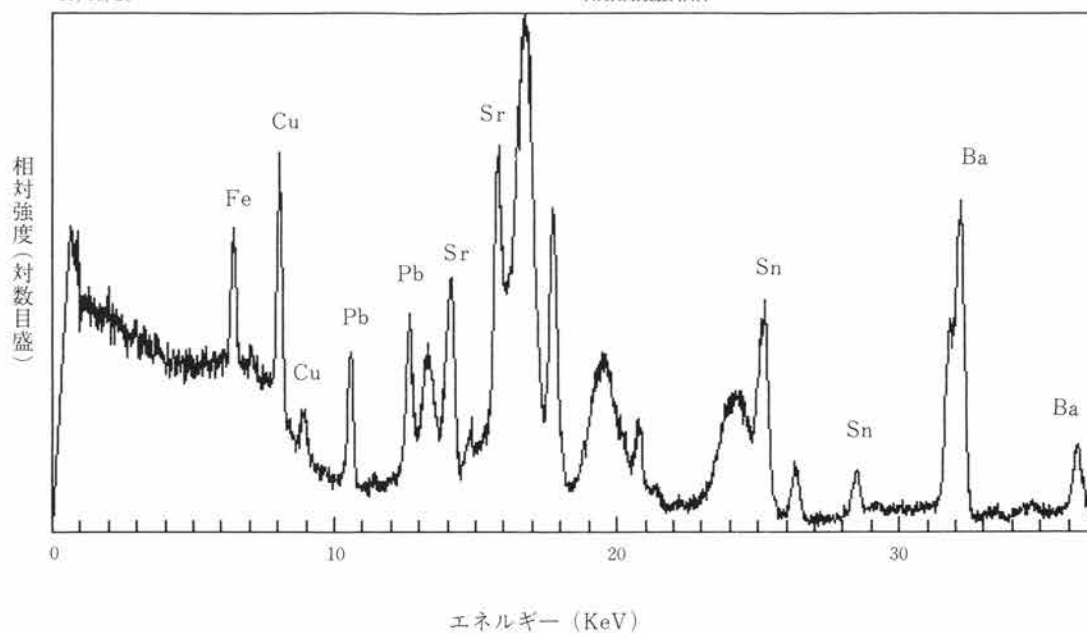
第398図 蛍光X線分析スペクトル(バリウムに富む鉛アルカリガラス、試料番号303)
