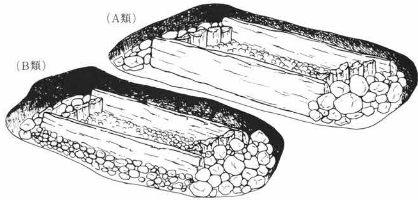
第400図 礫床墓想定復元図
