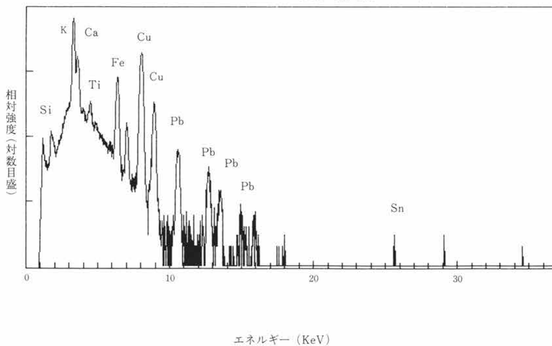
第399図 PIXEスペクトル(鉛アルカリガラス、試料番号344)
