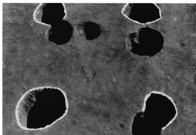
1号掘立柱建物跡全景
