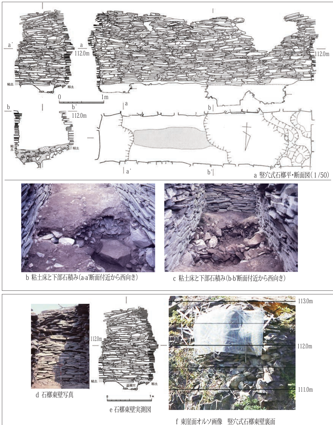
第2図 鶴尾神社4号墳竪穴式石槨 実測図・写真
