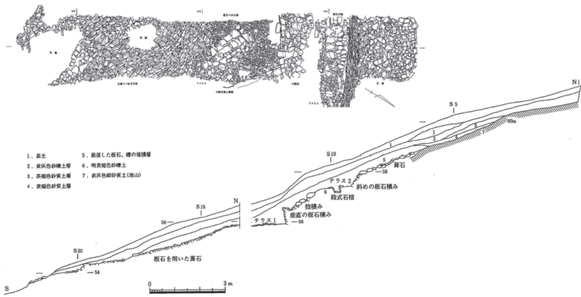
図3 松岳山古墳 くびれ部 (1/150)
