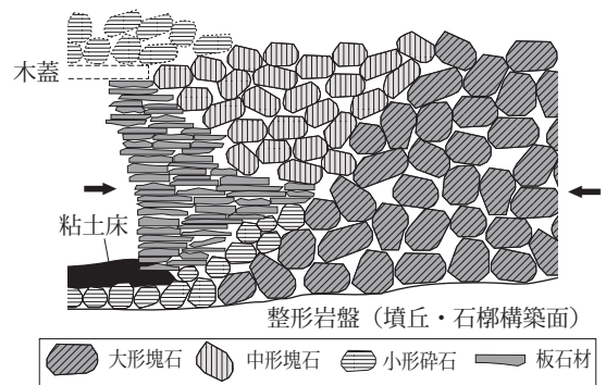
第 4 図 竪穴式石槨・積石墳丘関係模式図
