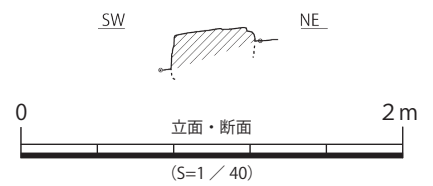
前方部前端断面図 (断面 A)
