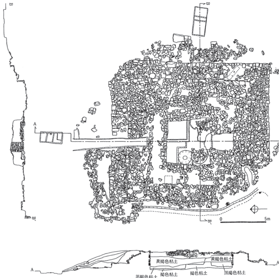
図7 石村洞4号墳 (1/250)
