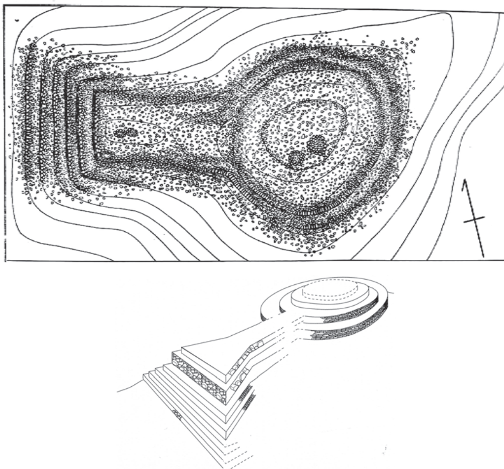
図 6 稲荷山姫塚古墳 測量図 (1/600) および復元イメージ図
