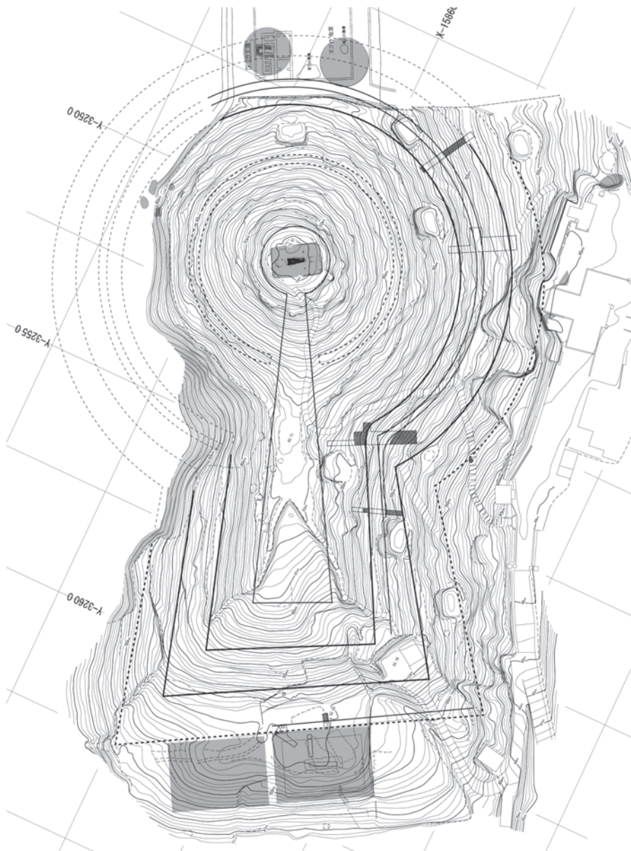
図4 松岳山古墳 測量図 (1/1200)
