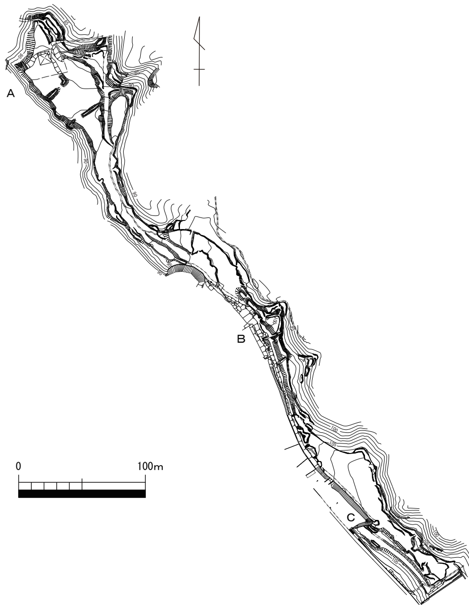
第5図 八幡谷ノ上明石道付城跡A・B・C 測量図
