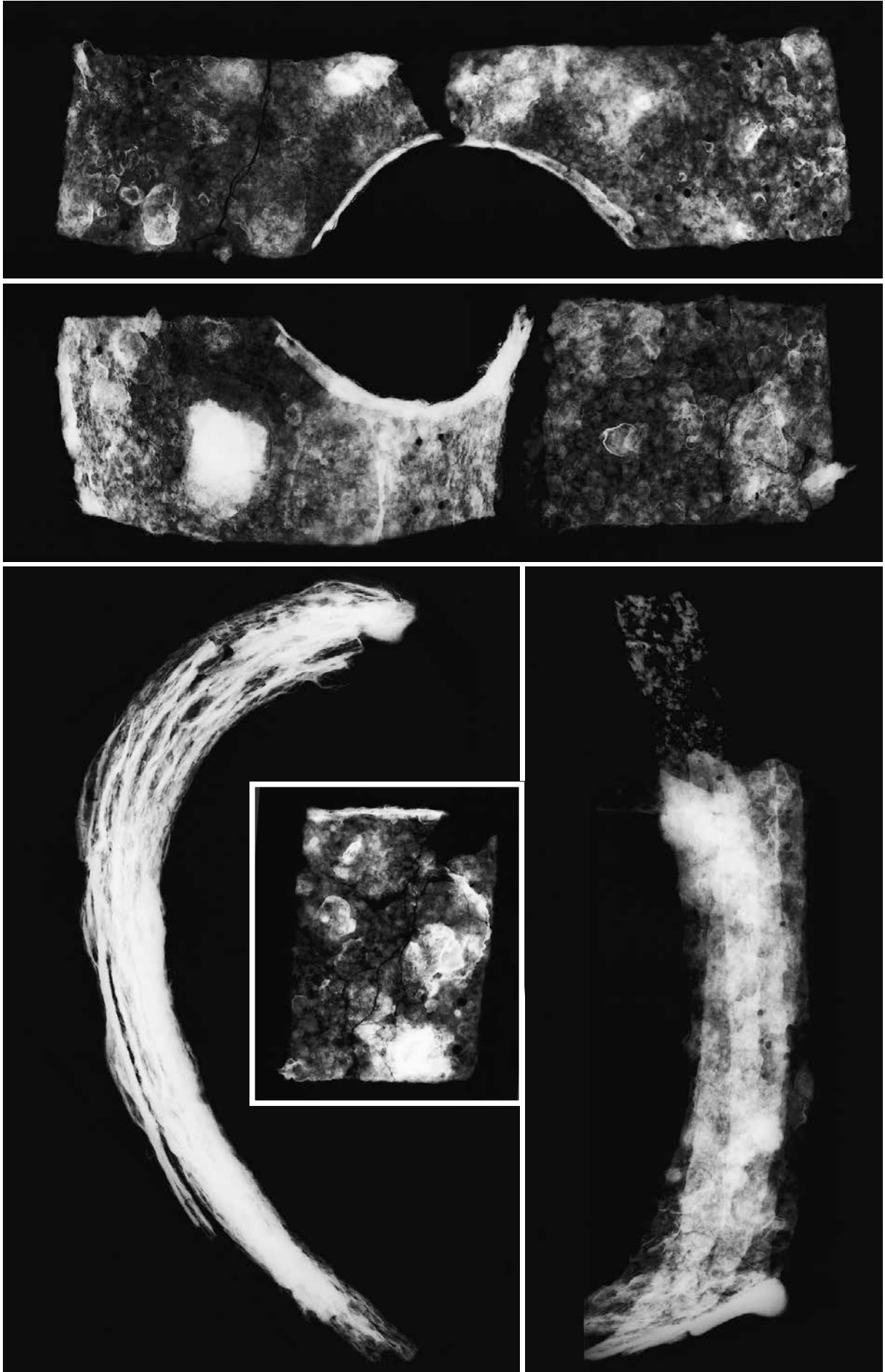
頸甲・肩甲 X線写真
