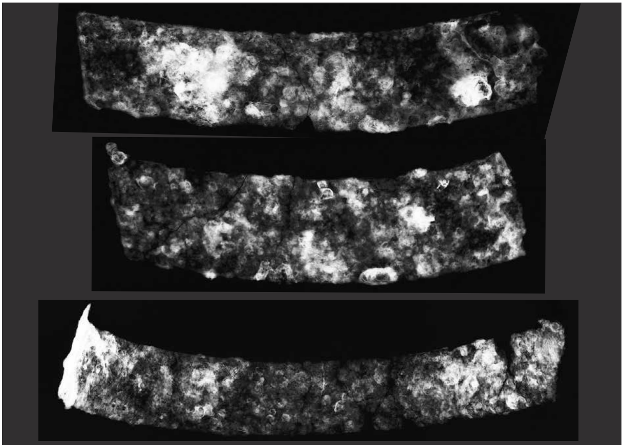
三段鍔X線写真
