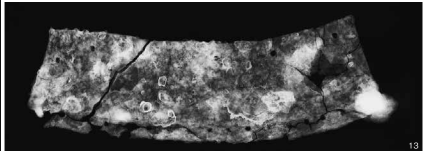
長方板革綴短甲 各部X線写真
