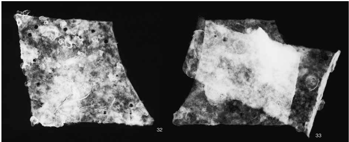
三角板革綴襟付短甲 後胴豎上第2段および頸甲背面引合板X線写真
