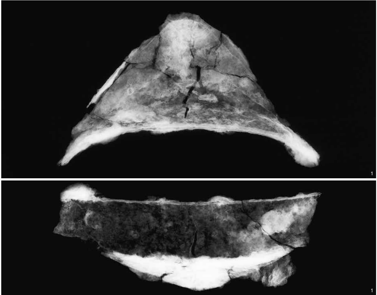
豎矧板鋏留衝角付冑 衝角底板・豎眉庇X線写真
