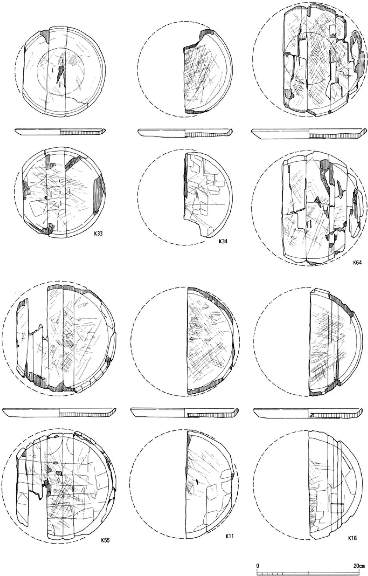
図面82 窪地東岸出土木製品9 (挽物A)
