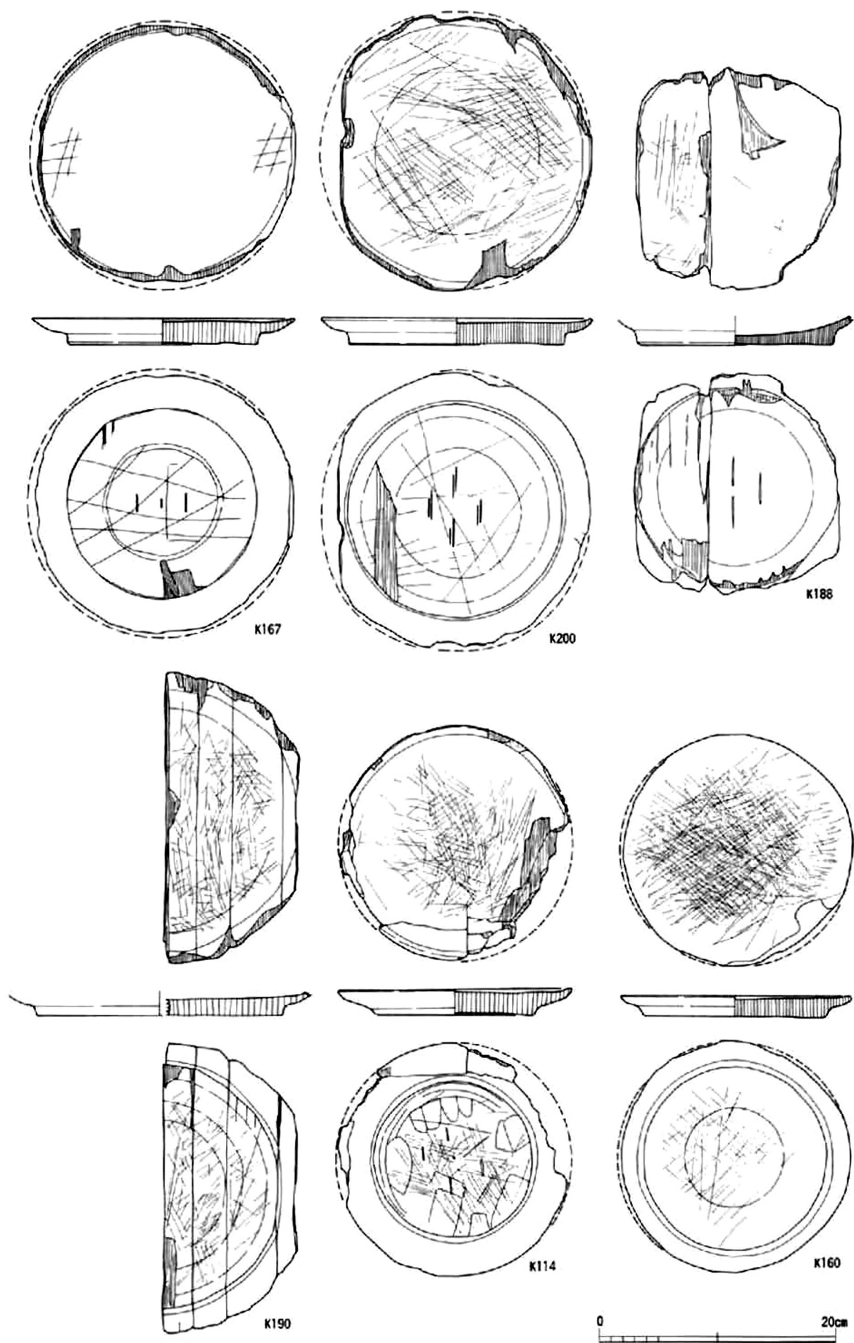
図面68 窪地西岸出土木製品10 (挽物B)
