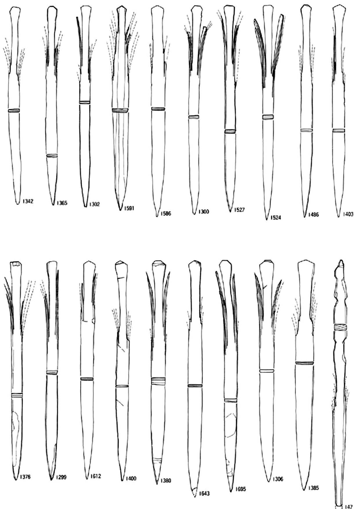
図面62 窪地西岸出土木製品 4 (斎串)
