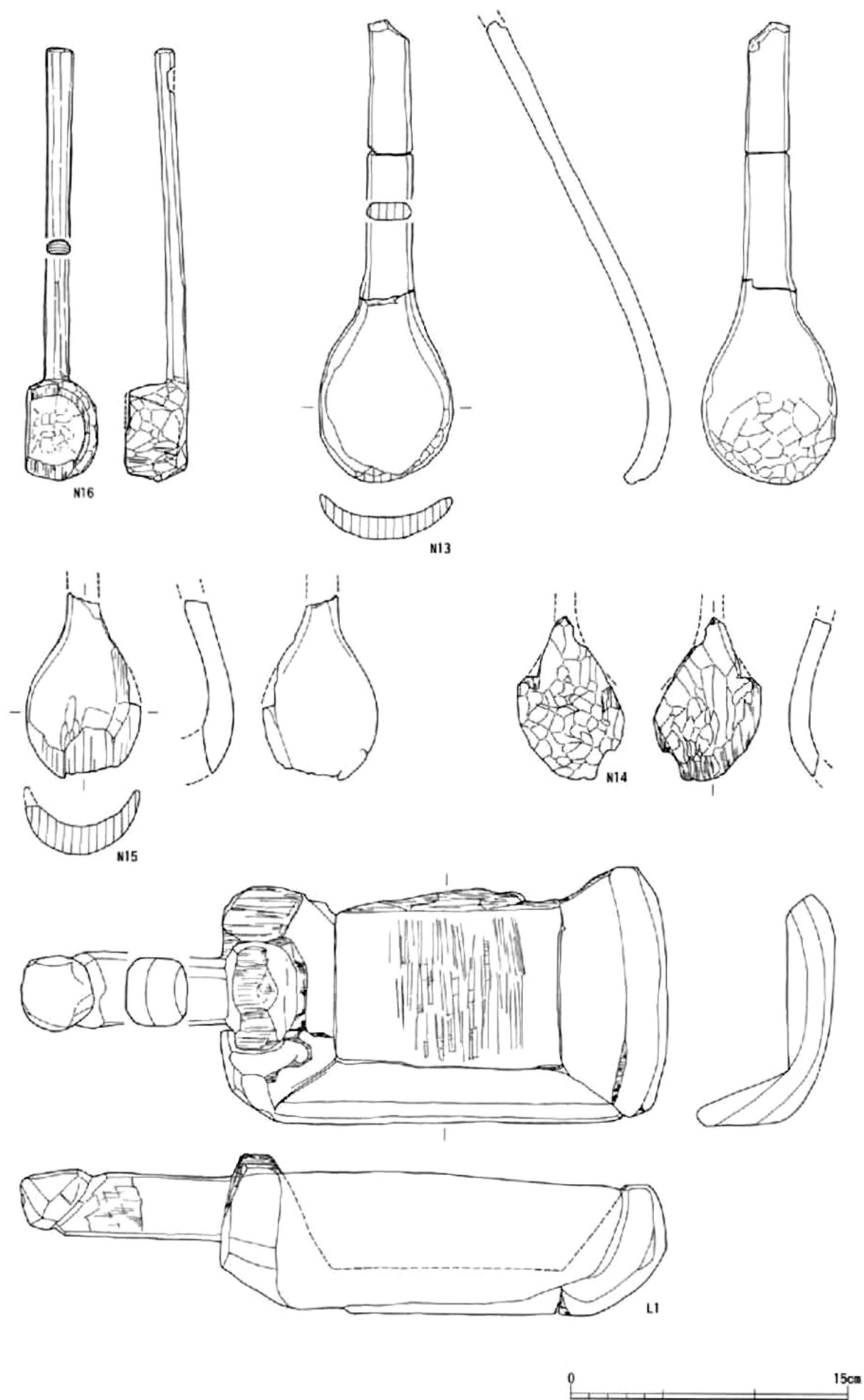
図面88 窪地東岸出土木製品15 (刮物・柄杓形木器・刮物匙)
