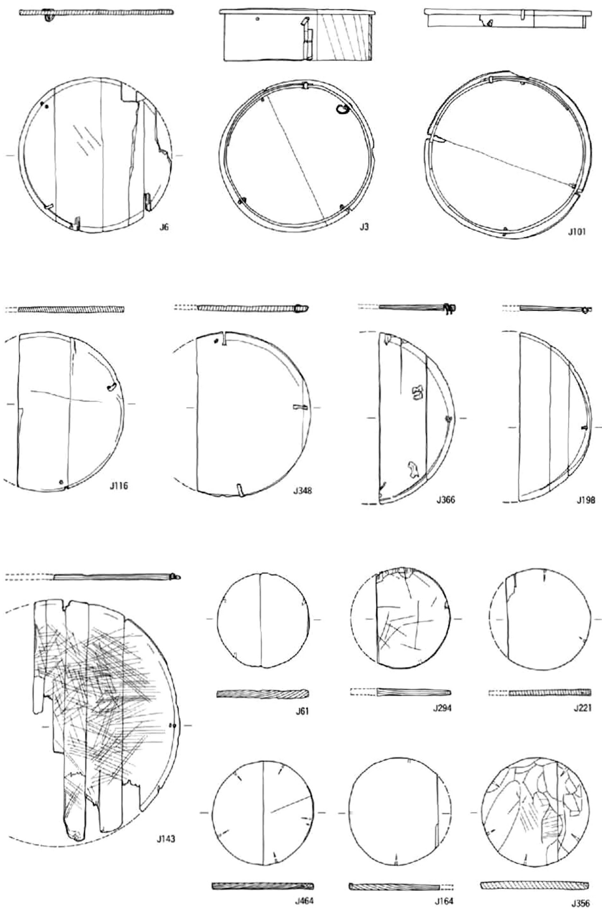
図面80 窪地東岸出土木製品7 (蓋・曲物)
