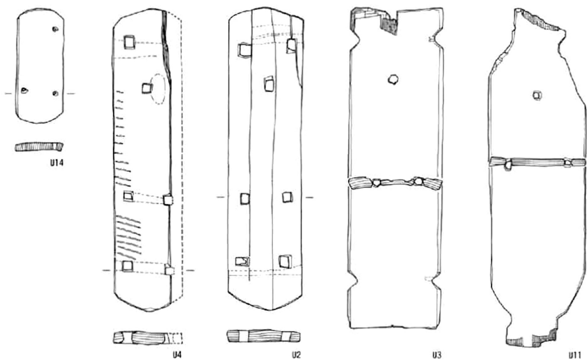
図面94 窪地東岸出土木製品21 (田下駄)
