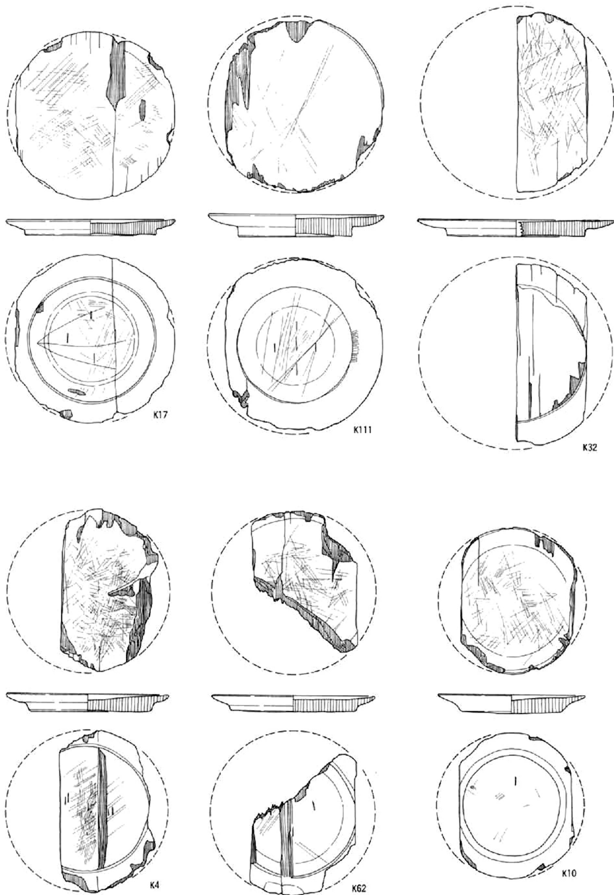
図面86 窪地東岸出土木製品13 (挽物B)
