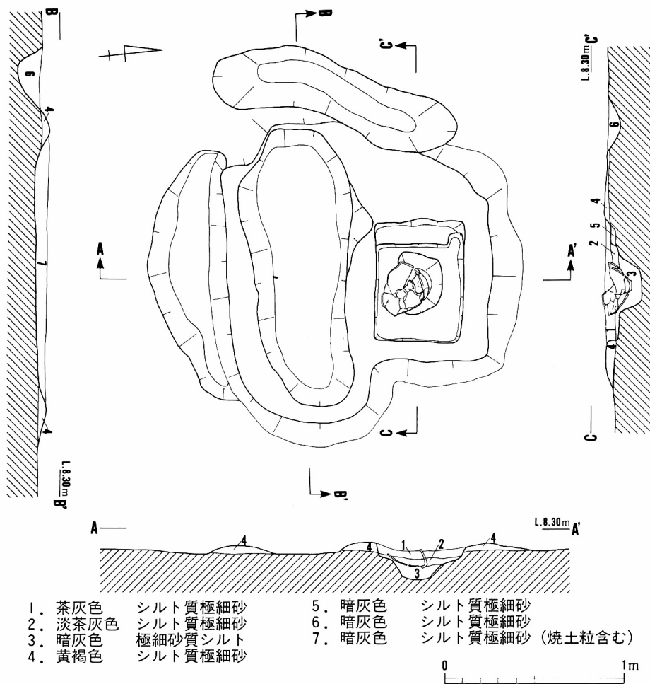
第18図 竪穴住居4 中央土壇と炉
