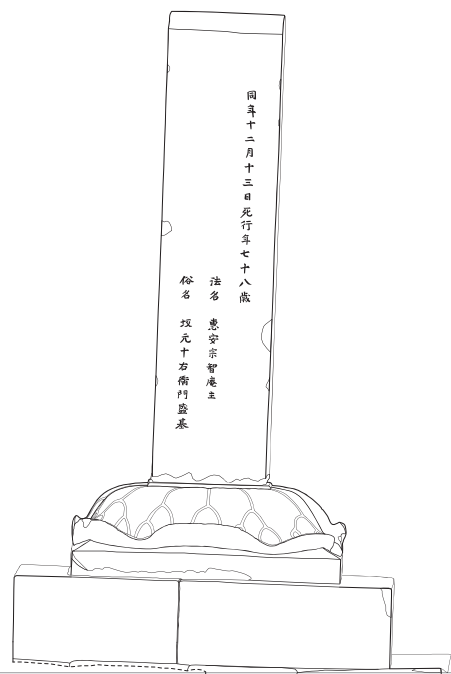
右側面図
