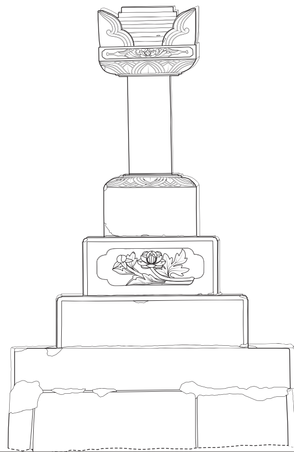
右側面図
