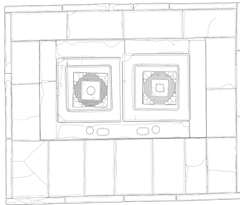
上面図
