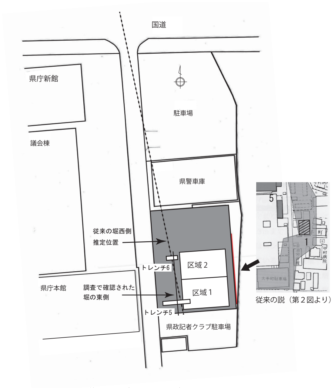
第3図 調査区配置図 (1/1000)
