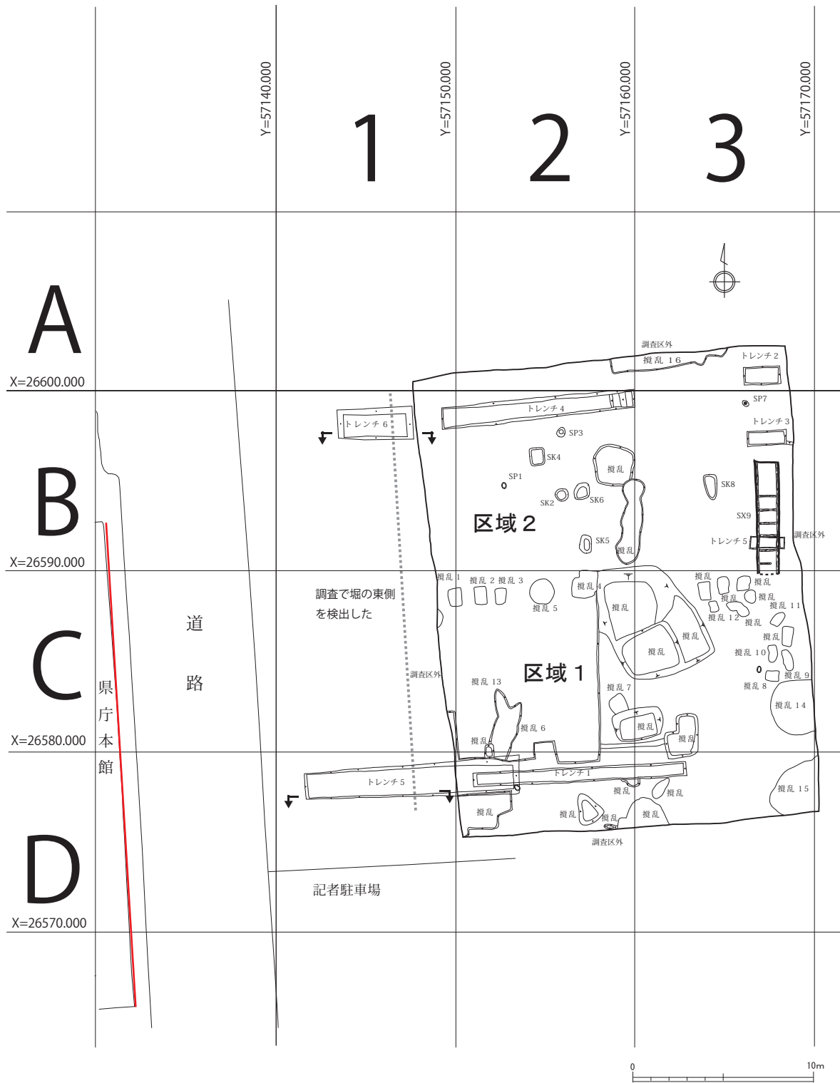
第 4 図 調査区平面図 (1/300)
