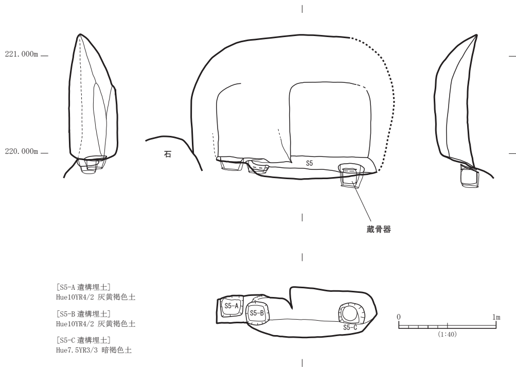
第32図 S 5 遺構実測図
