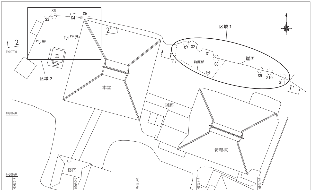
第2図 大應寺平面図 (1/300)
