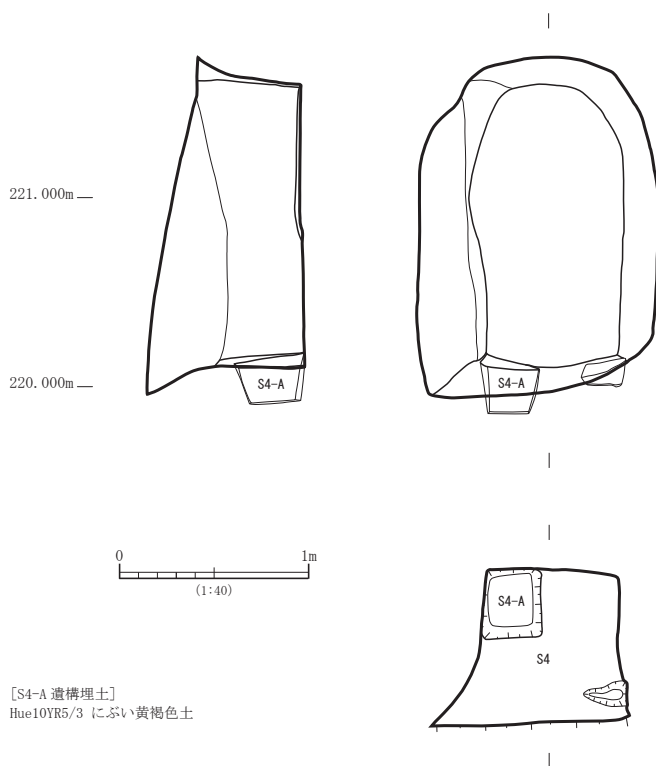
第31図 S4遺構実測図
