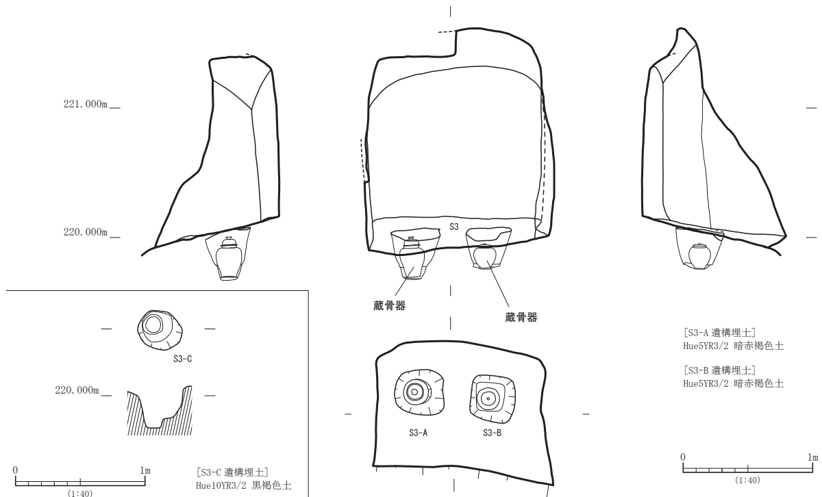
第30図 S3遺構実測図
