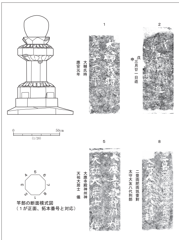
第9図 石塔1実測図
