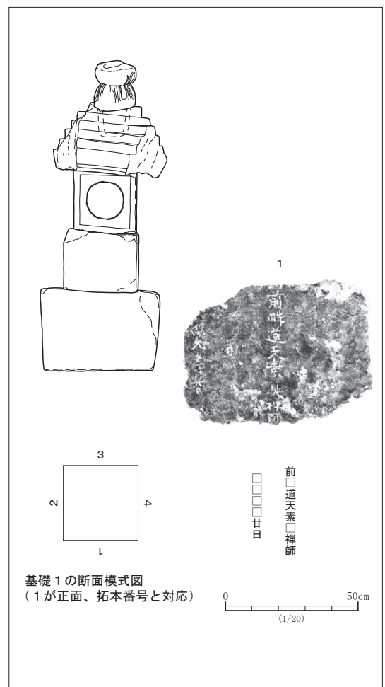
第10図 石塔4実測図
