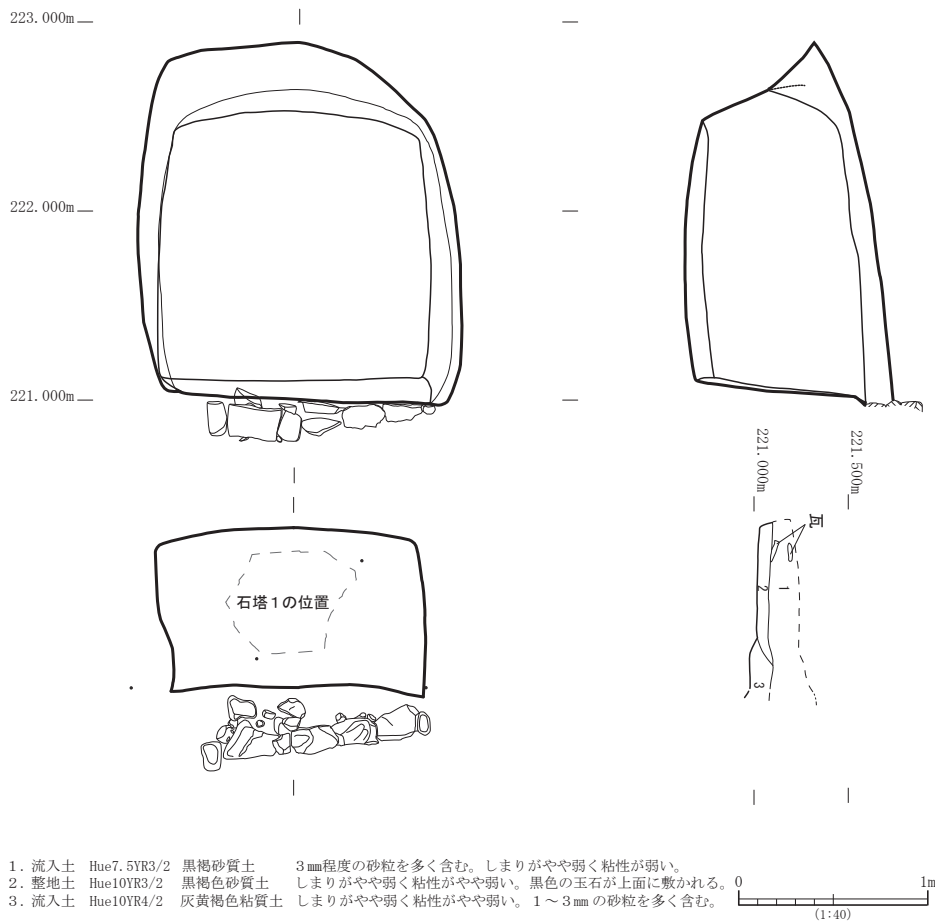
第8図 S2遺構実測図および土層断面図
