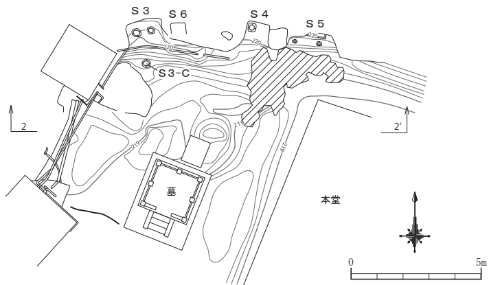
第4图 区域2测量图 (1/200)
