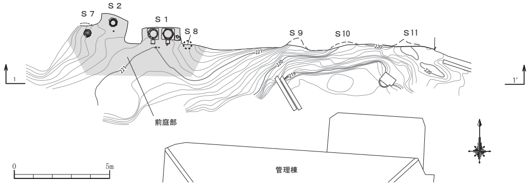
平面图
