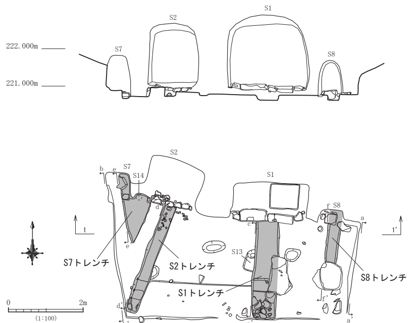
第15図 区域1前庭部トレンチ配置図 (1/100)
