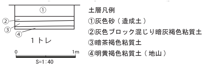
図7: 土層図
