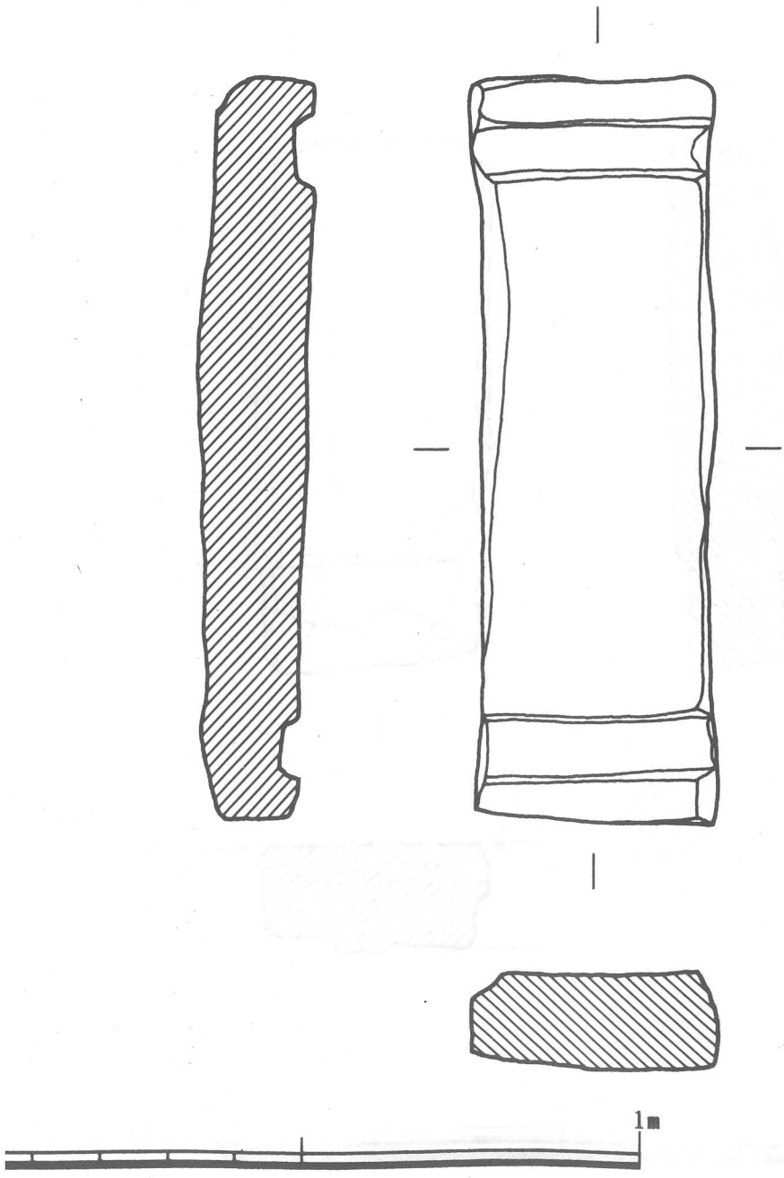
第4図 石棺実測図 3 (郷ノ谷5号墳 1)
