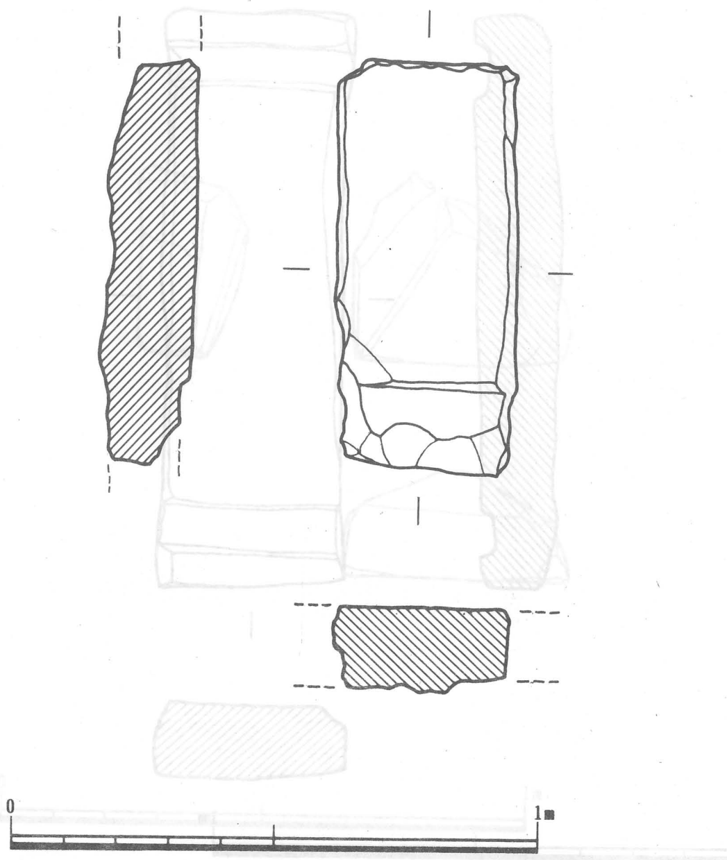
第3図 石棺実測図 2 (佐用岡 2)
