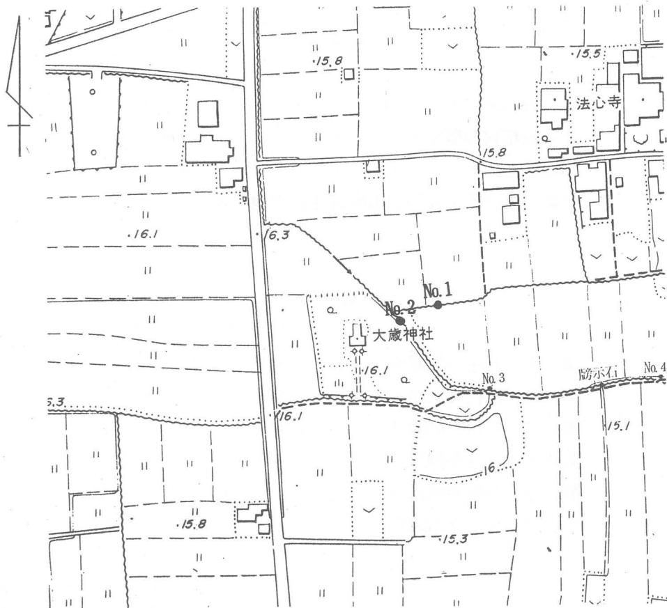
第1図 石棺位置図 (S=1/2500)
