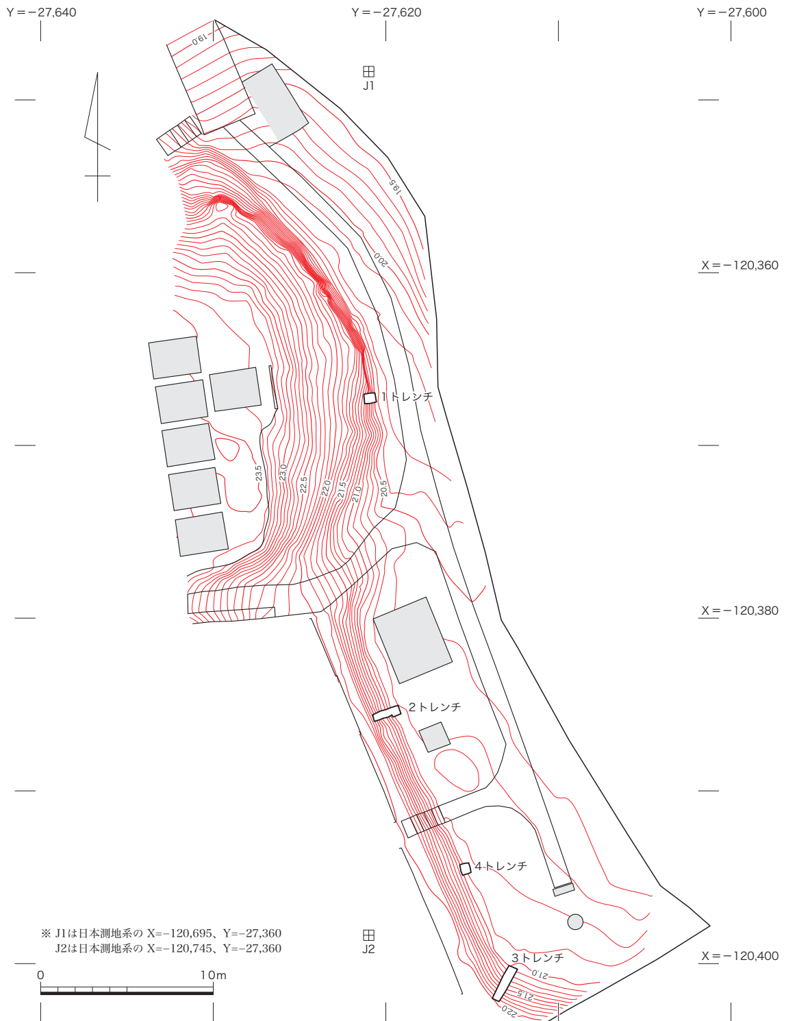
第7図 現況の墳丘と調査区の配置 (1/300)
