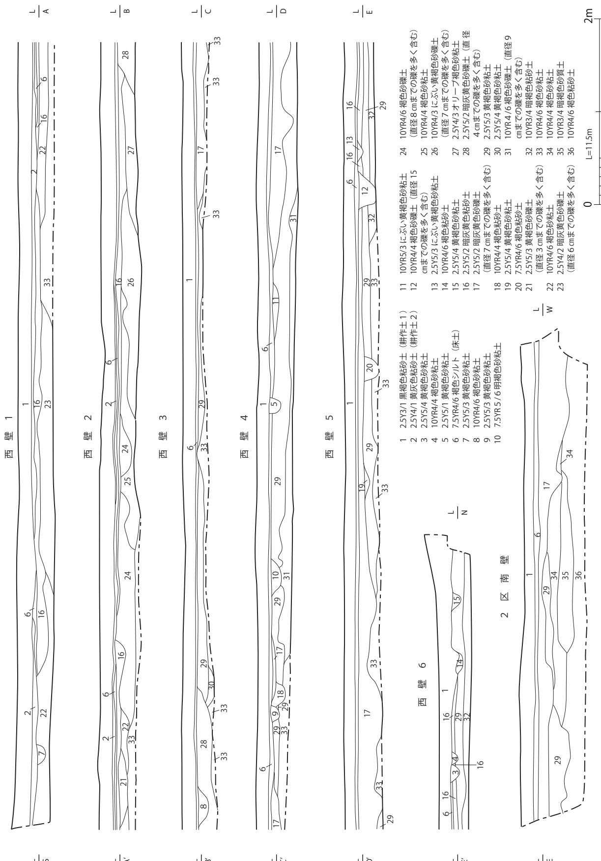
第2図 調査区断面図 (1/40)
