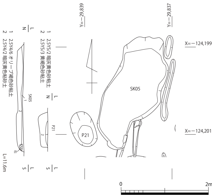
第4図 P 21・SK 05 (1/50)
