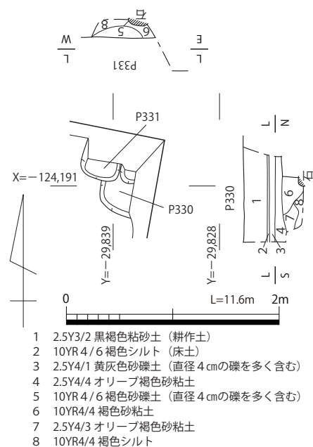
第8図 P 330・P 331 (1/50)
