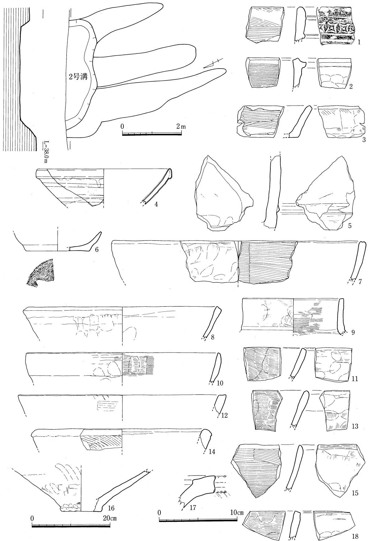
第8図 2号溝実測図及びその出土遺物 (1/80, 1/6, 1/3)
