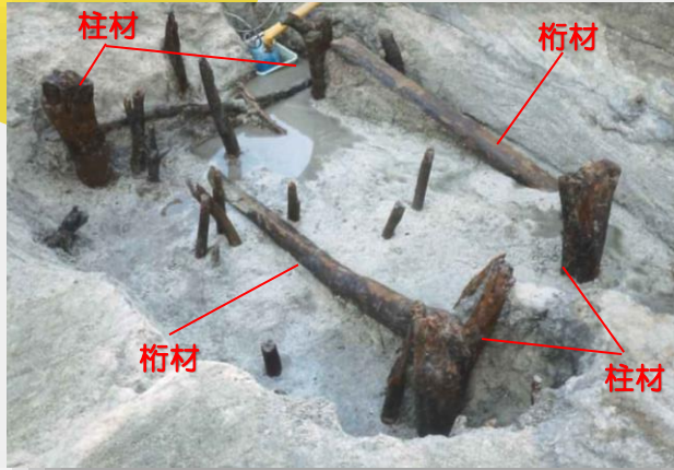
木橋の出土状況
