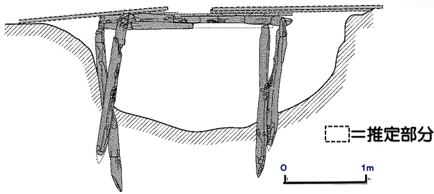
木橋の復元図
