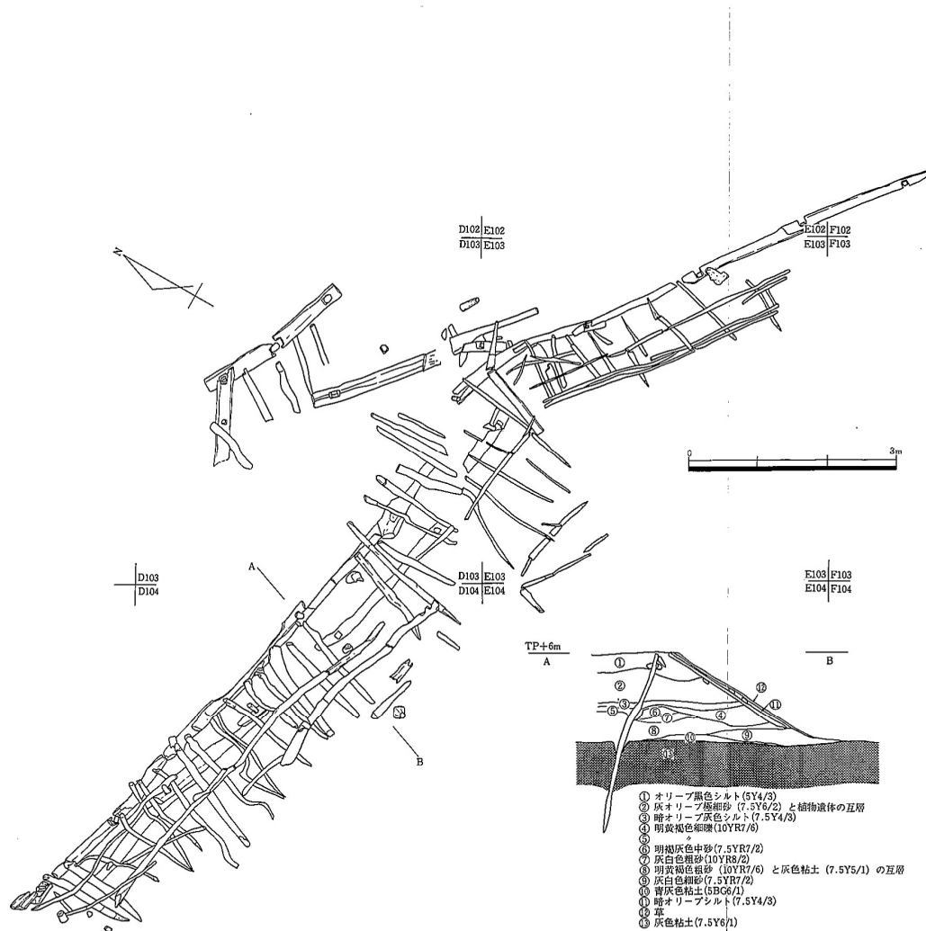
第238図 S S 5003遺構平面図・土層断面図
