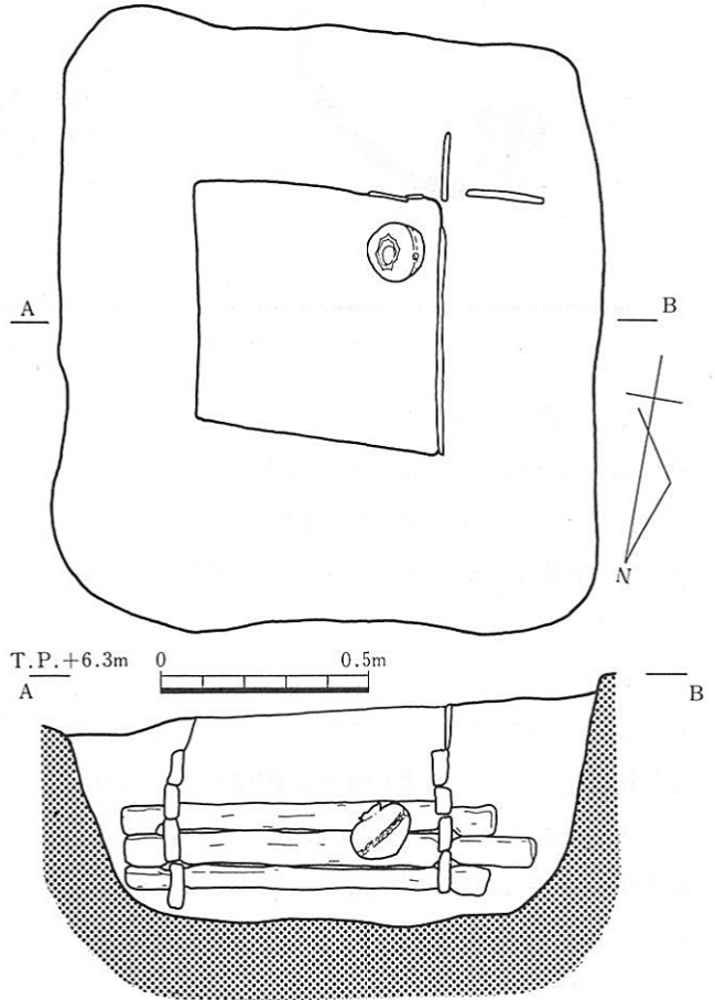
第205図 S E 5002遺構平面図・断面図
