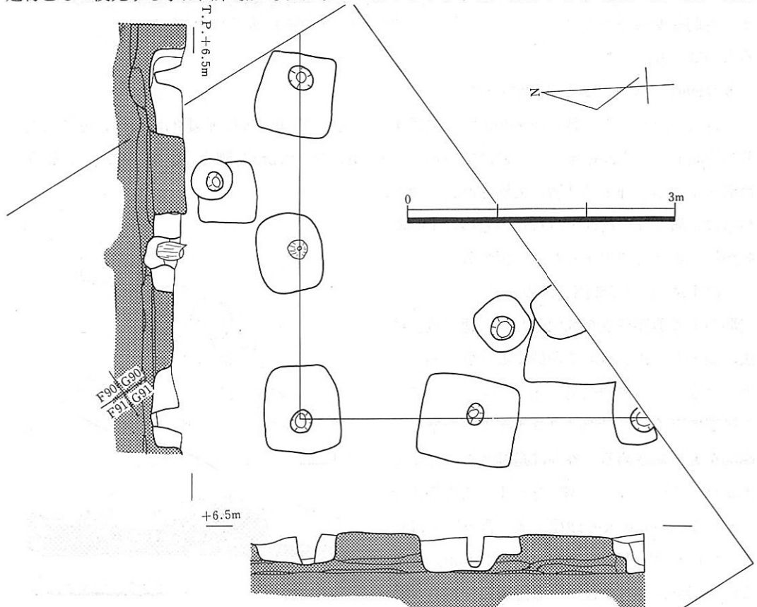
第257図 S B 6004遺構平面図・断面図
