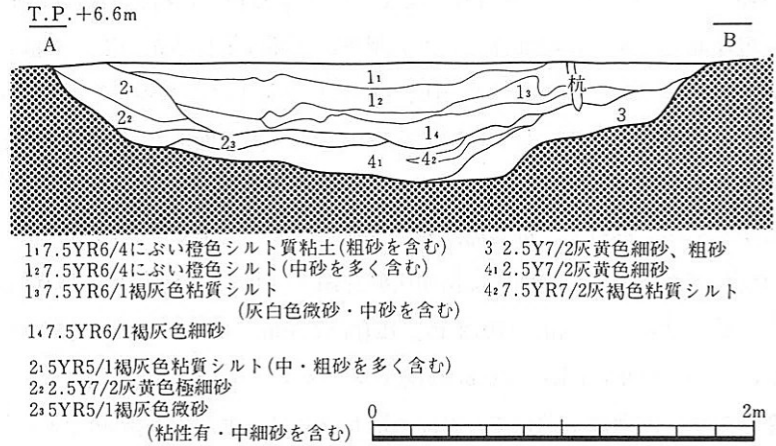
第263図 S D6003土層断面図
