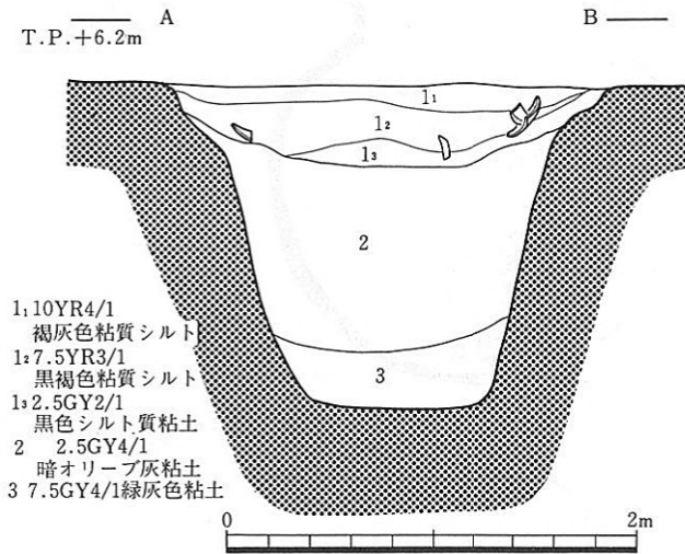
第267図 S E 6001土層断面図
