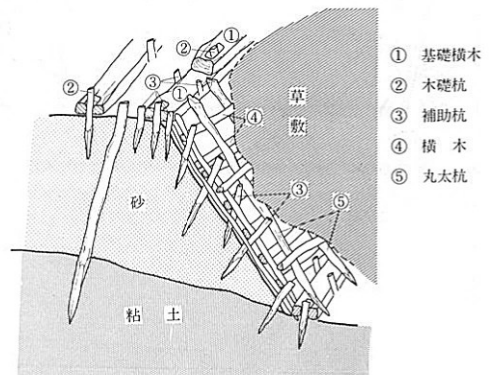
第233図 杭列構造模式図
