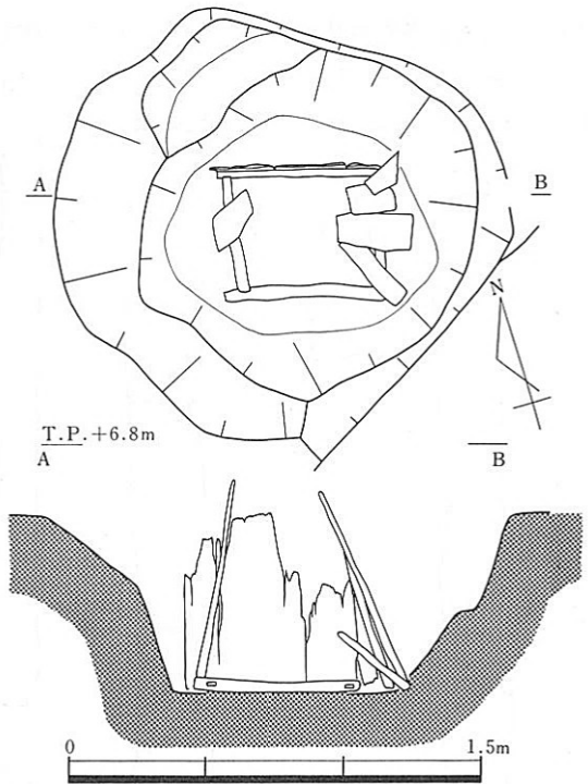
第271図 S E 6003遺構平面図・断面図
