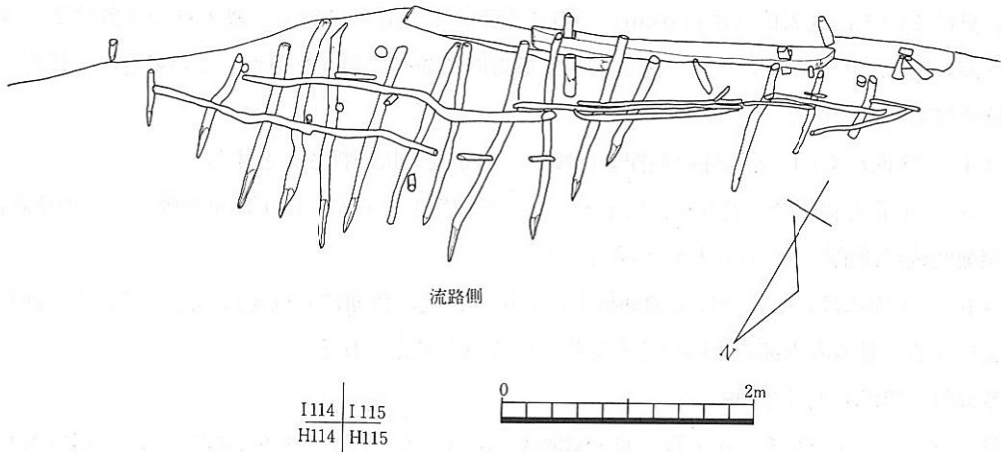
第236図 S S 5005遺構平面図(1)
