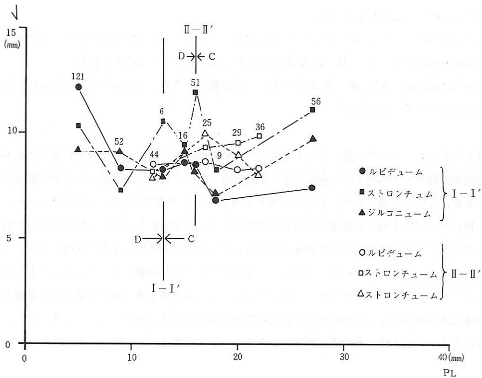
第9図 Pl-Rb · Sr · Zr 相関図
