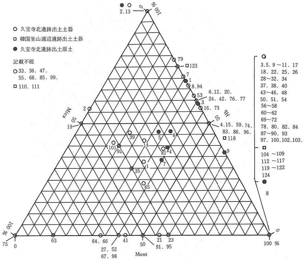
第2図 Mo-Mi-Hb三角ダイヤグラム
