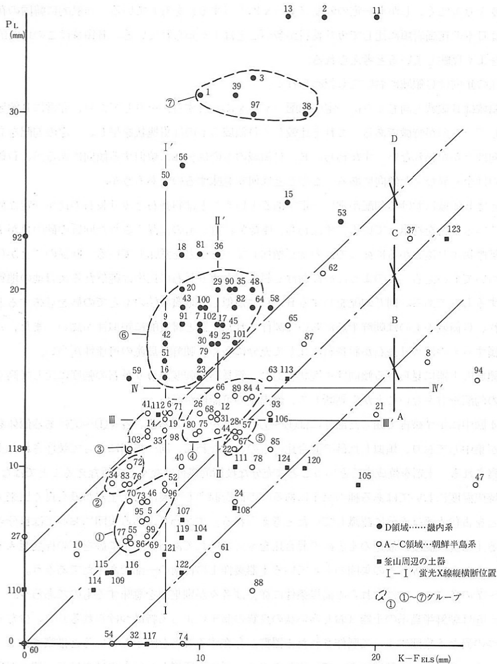
第4図 Pl-K-fels相関図
