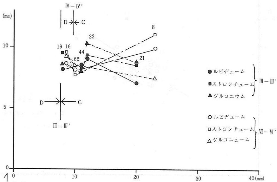
第8図 K-fels-Zr · Sr · Rb 相関図
