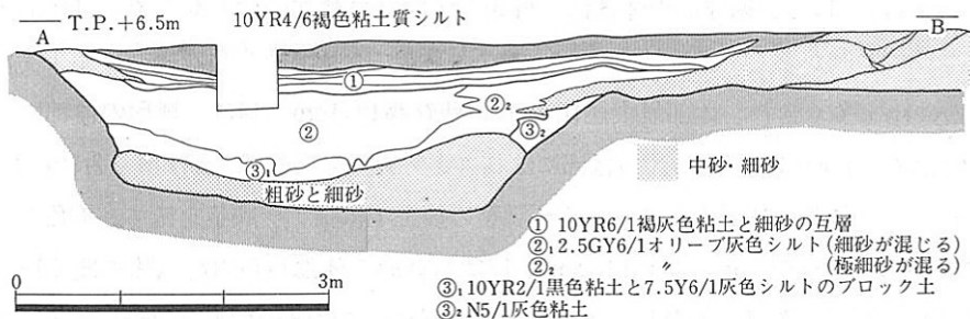
第199図 S D 5001土層断面図
