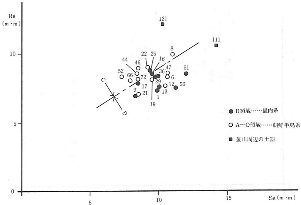
第7図 Rb-Sr相関図
