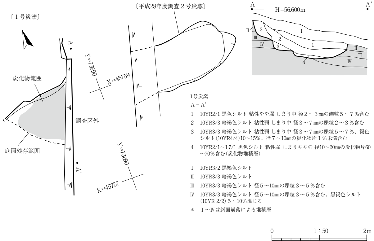
第18図 1号炭窯
