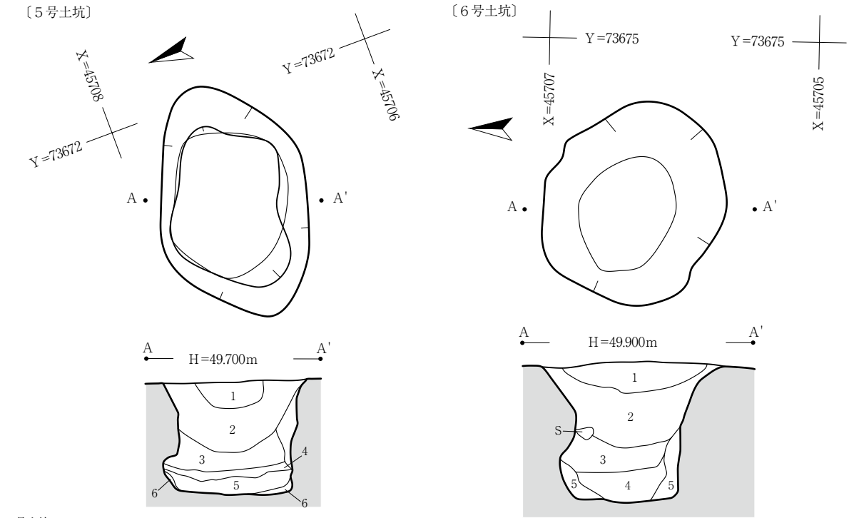
5号土坑 A-A'
