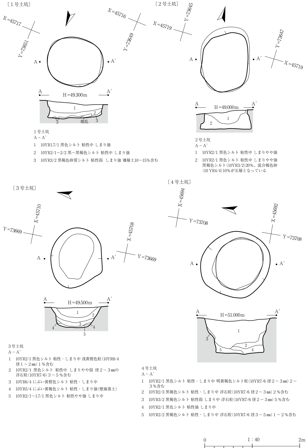
第16図 1~4号土坑
