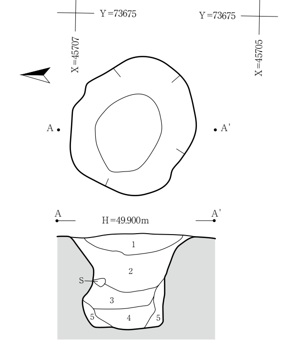
6号土坑 A-A'
