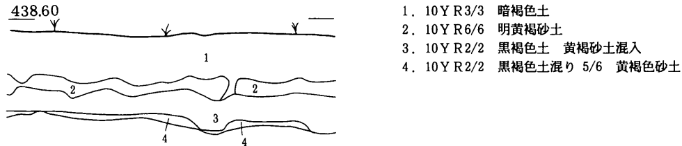
挿図4 基本層序
