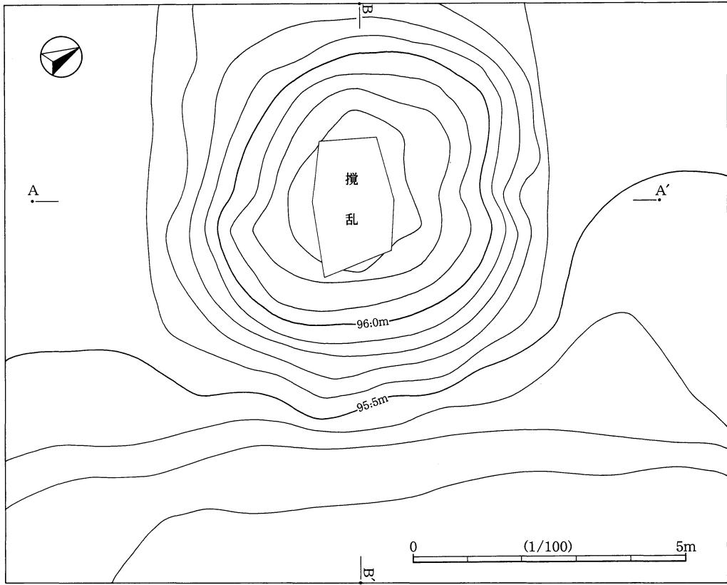
第4図 SM-001表土除去後測量図
