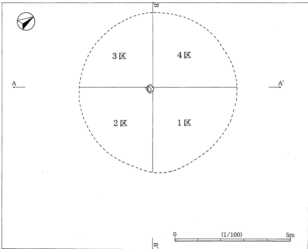
第5図 SM-001盛土除去後平面図
