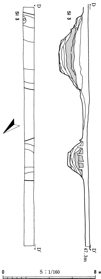
第8図 Dトレンチ実測図
