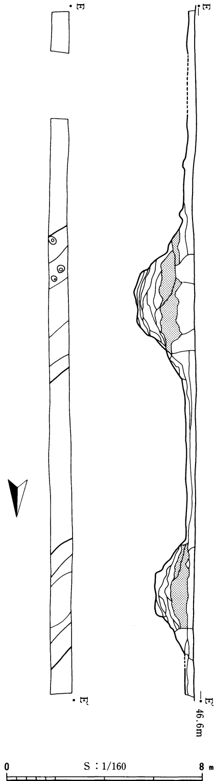
第9図 Eトレンチ実測図
