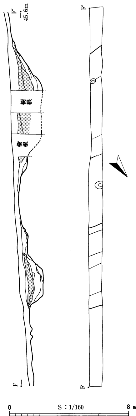
第10図 Fトレンチ実測図
