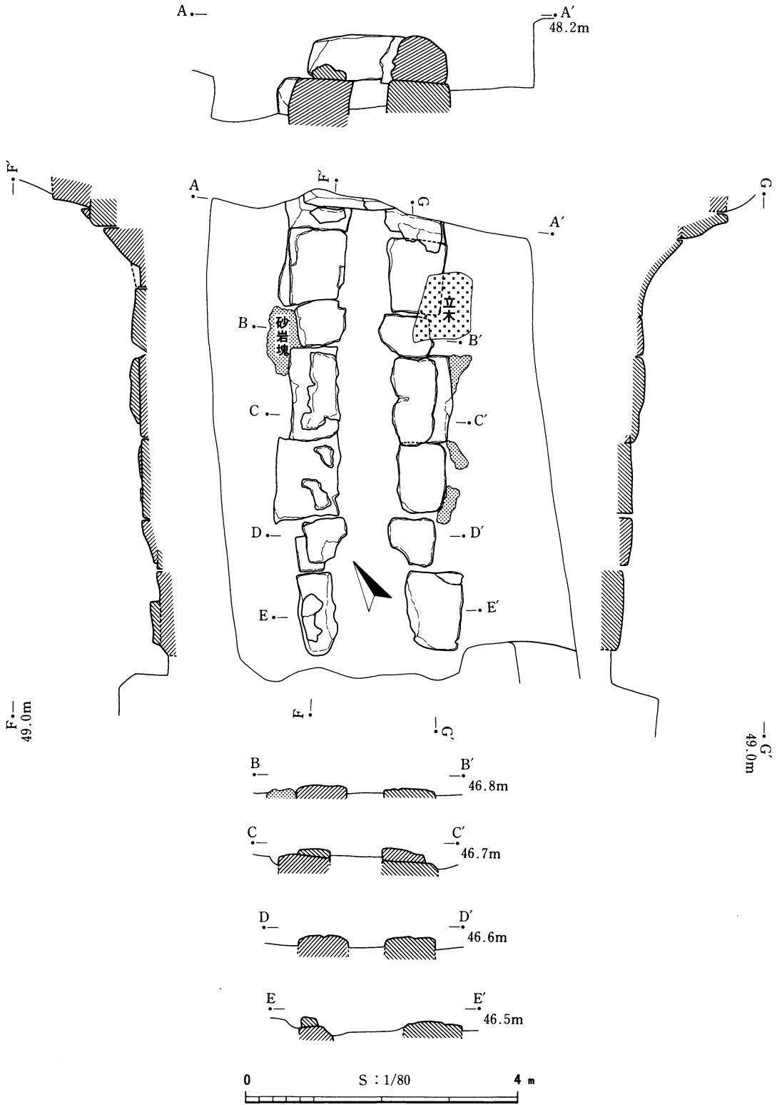
第 4 図 横穴式石室実測図
