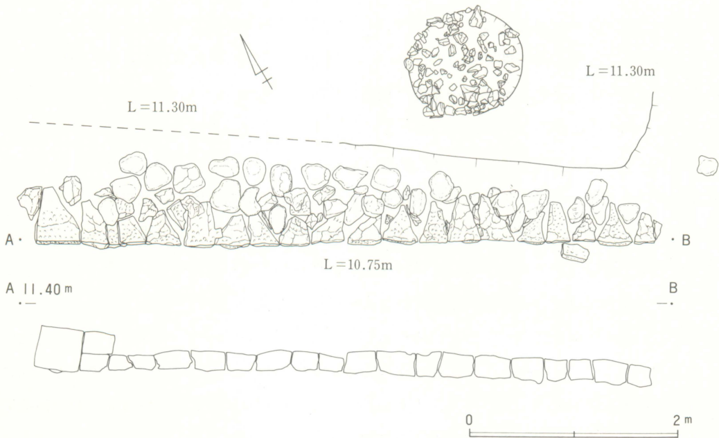
第3図 石積跡実測図
