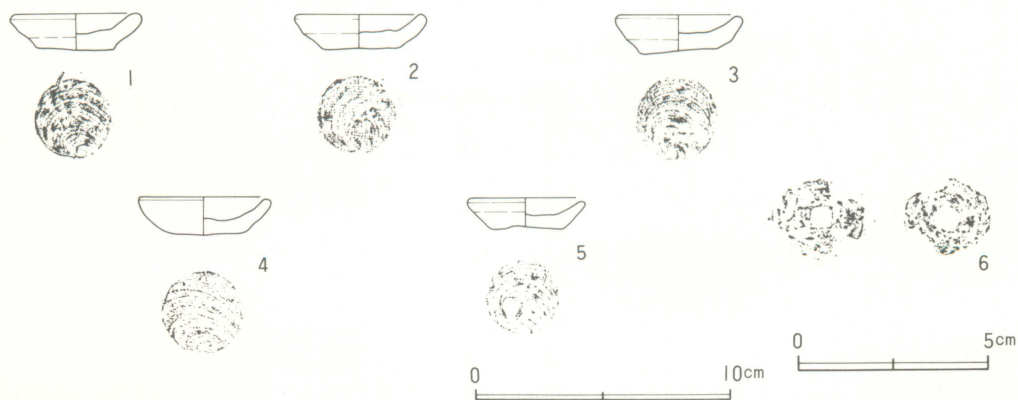
第6図 F-001号跡出土遺物実測図
