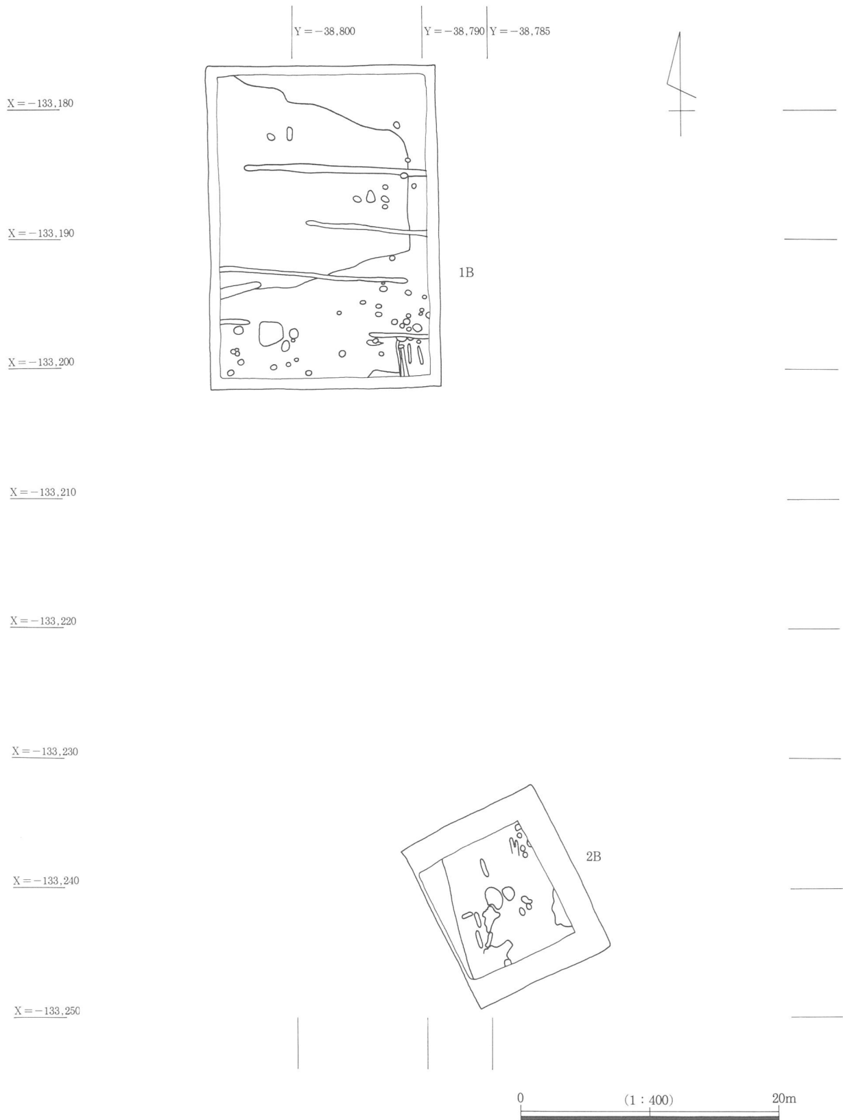
第162図 1B・2B区第2遺構面平面図
