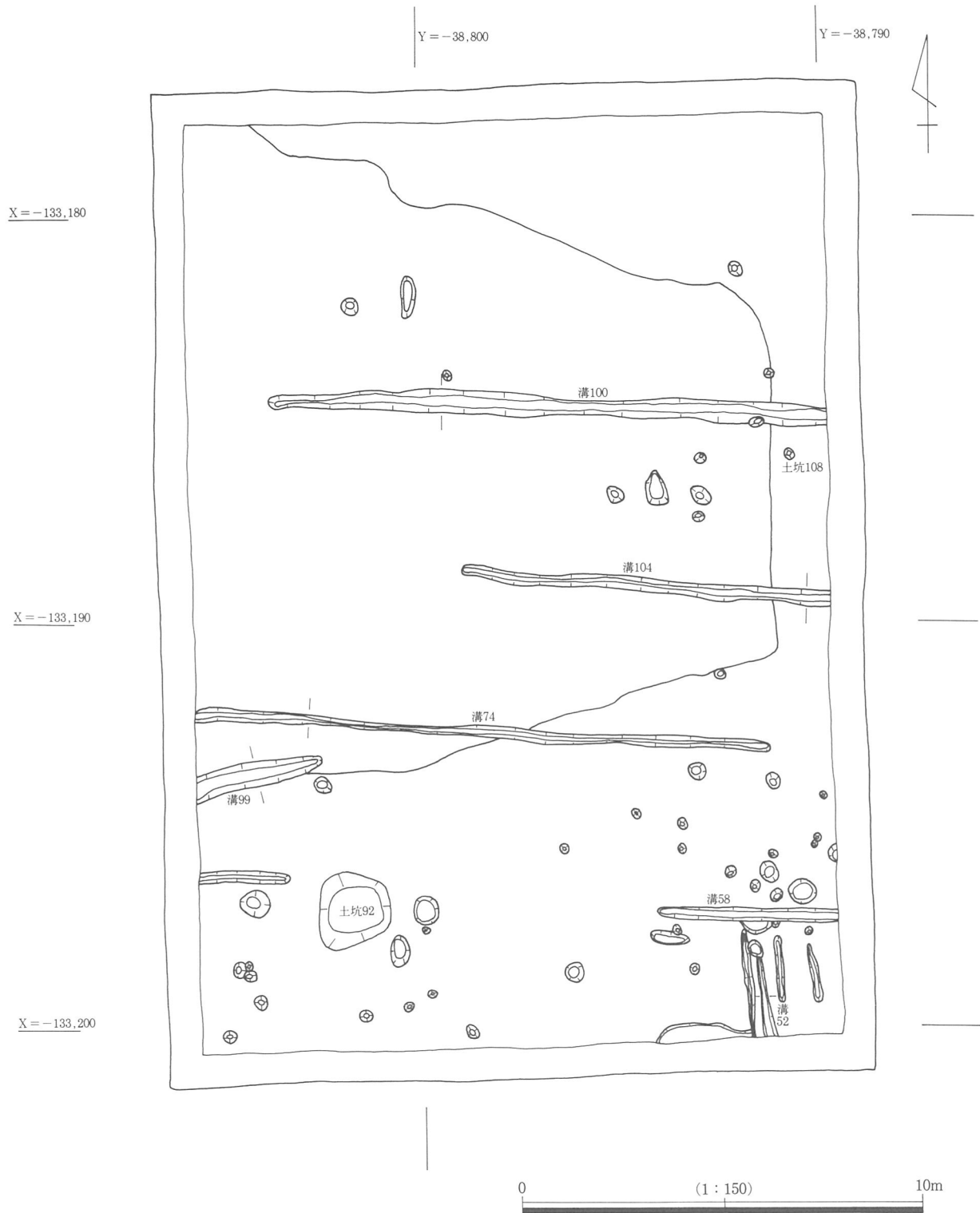
第163図 1B区第2遺構面平面図
