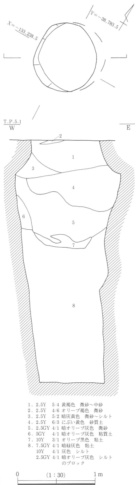
第159図 2 B区第1遺構面井戸1平面・断面図
