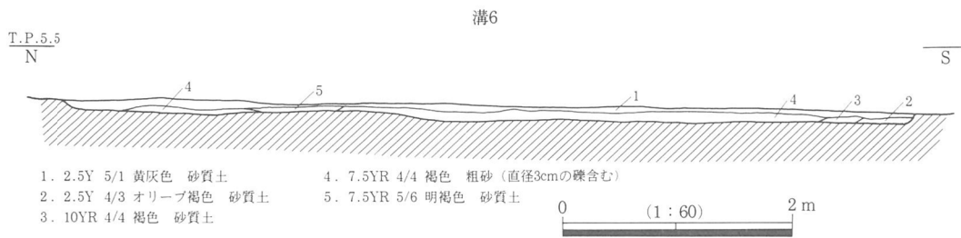
第161図 1 B区第1遺構面溝6断面図
