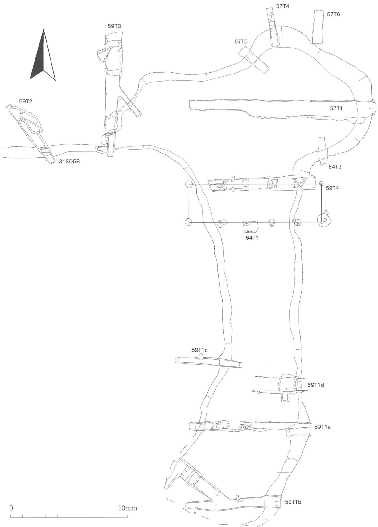
第30图 23SG1 (I期) 平面图
