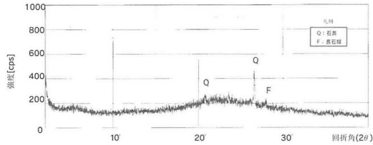
図4.1-1 X線回折図 (No.84 白色層)
