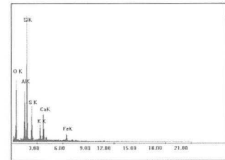
図4.1-6 スペクトル図 (サンプルNo.84)
