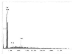
図4.1-9 スペクトル図 (サンプルNo.243)
