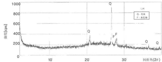
図4.1-2 X線回折図 (No.210 白色層)
