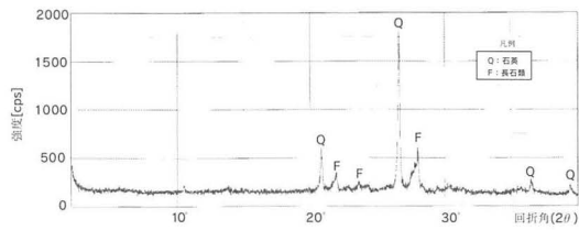
図4.2-5 X線回折図 (No.271 壁土)
