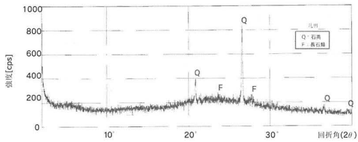
図4.1-5 X線回折図 (No.271 白色層)
