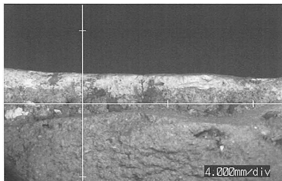
サンプルNo. 271 (白色層断面 ×25倍)
