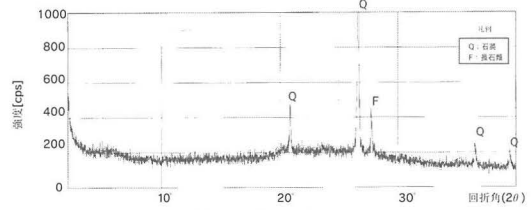
図4.1-4 X線回折図 (No.243 白色層)
