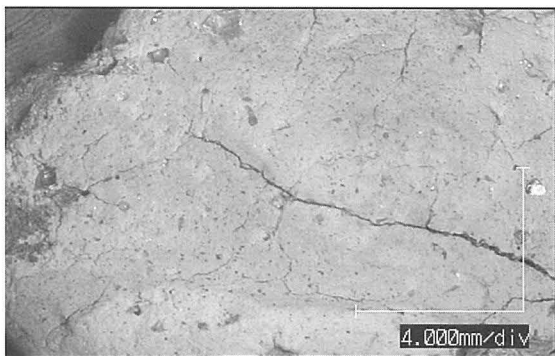
サンプルNo. 271 (白色層表面 ×25倍)
