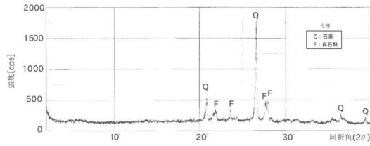
図4.2-1 X線回折図 (No.84 壁土)
