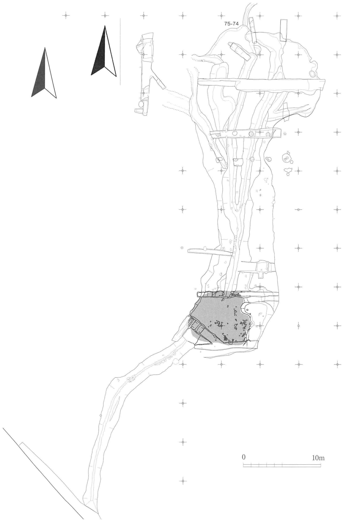
第32图 23SG1 (Ⅲ期) 平面图
