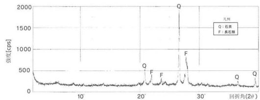
図4.2-4 X線回折図 (No.243 壁土)
