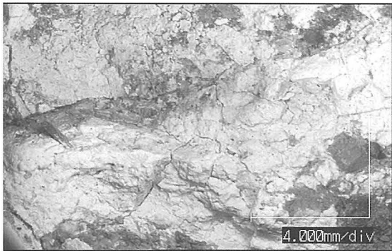
サンプルNo. 243 (白色層表面 ×25倍)
