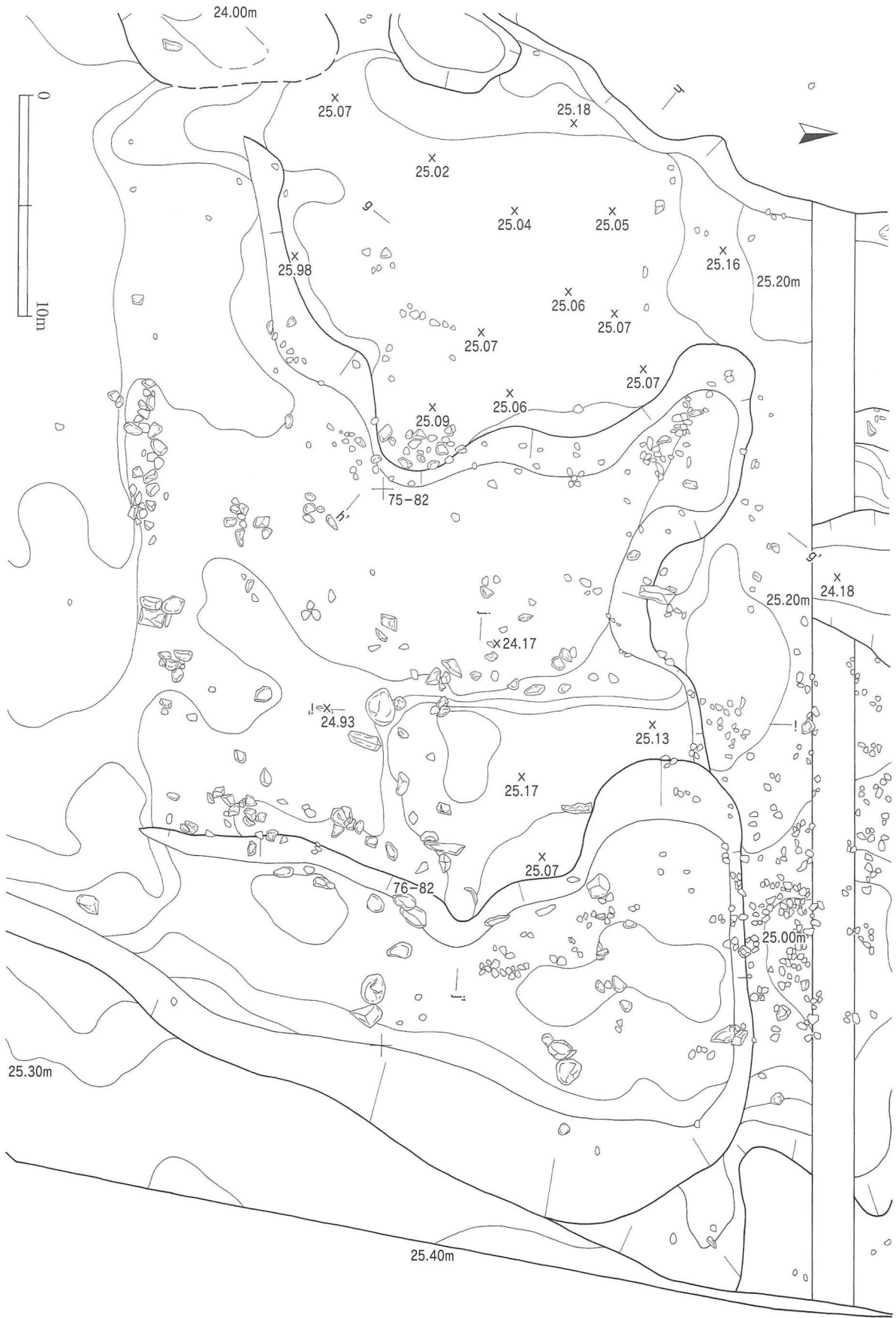
第8図 59T1 e~f 位置図
