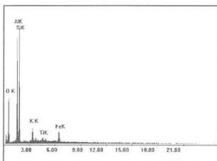
図4.1-8 スペクトル図 (サンプルNo.219)
