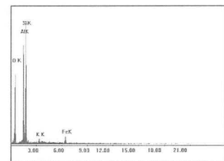
図4.1-7 スペクトル図 (サンプルNo.210)
