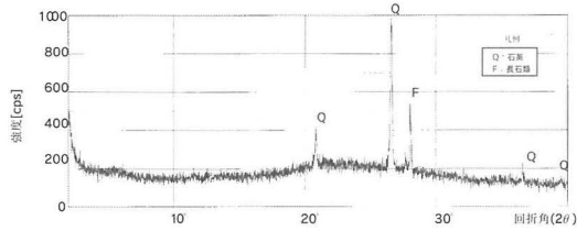
図4.1-3 X線回折図 (No.219 白色層)
