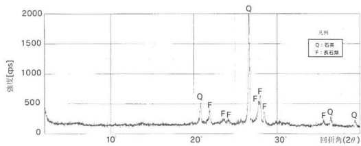
図4.2-3 X線回折図 (No.219 壁土)
