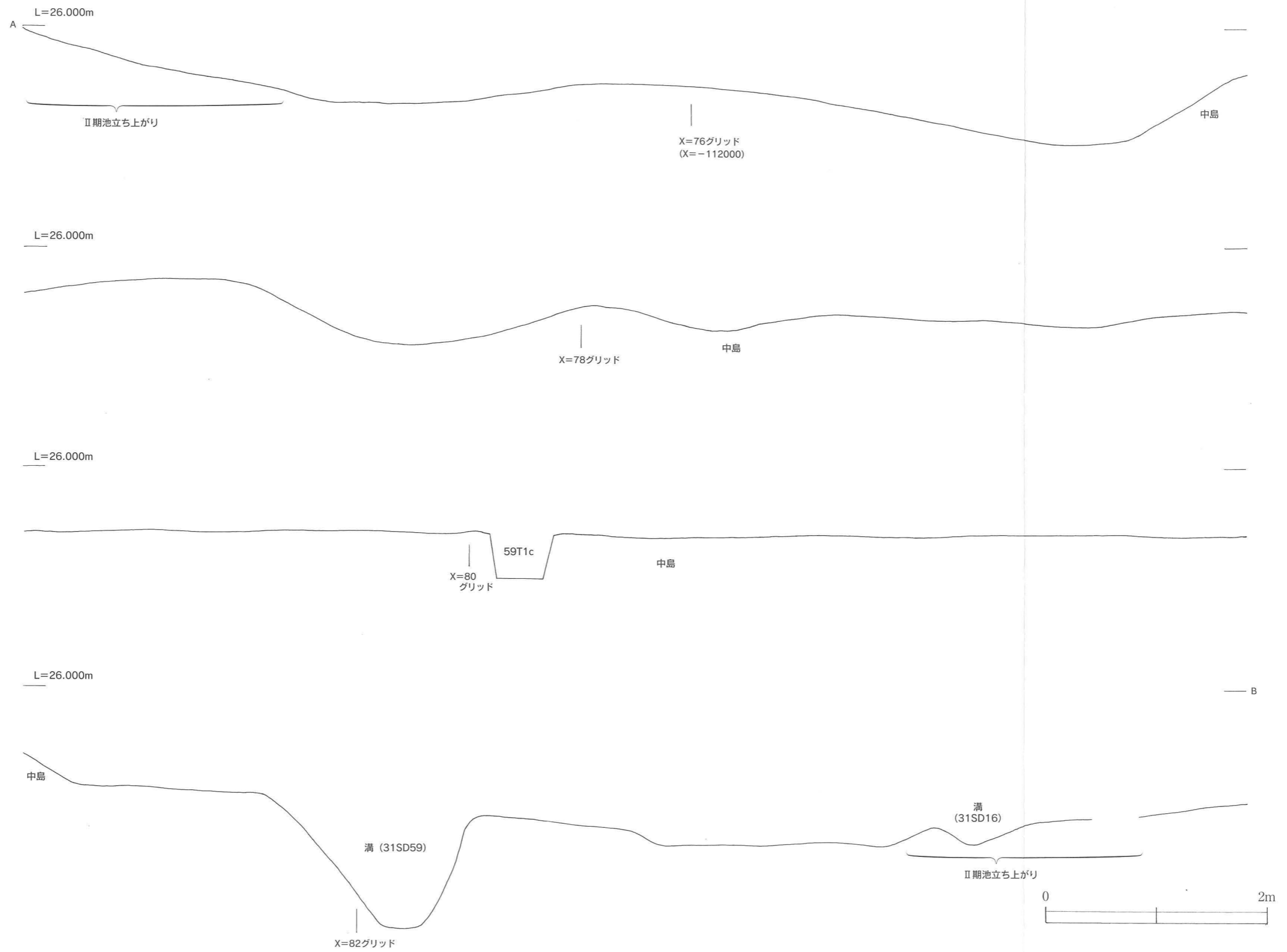
第23図 23SG1 縦断面図
