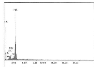
図4.1-10 スペクトル図 (サンプルNo.271)
