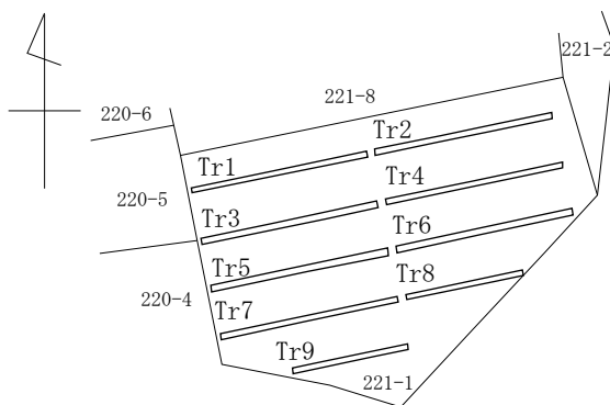
全体図 1:1,000
