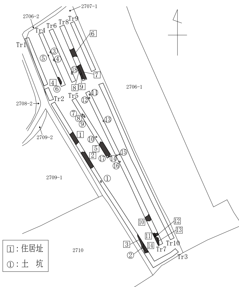
全体図 1:1,000
