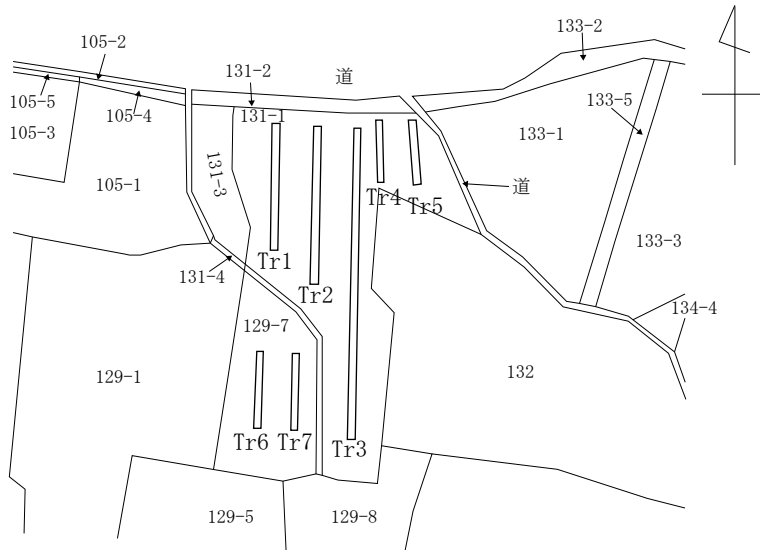
全体図 1:1,000
