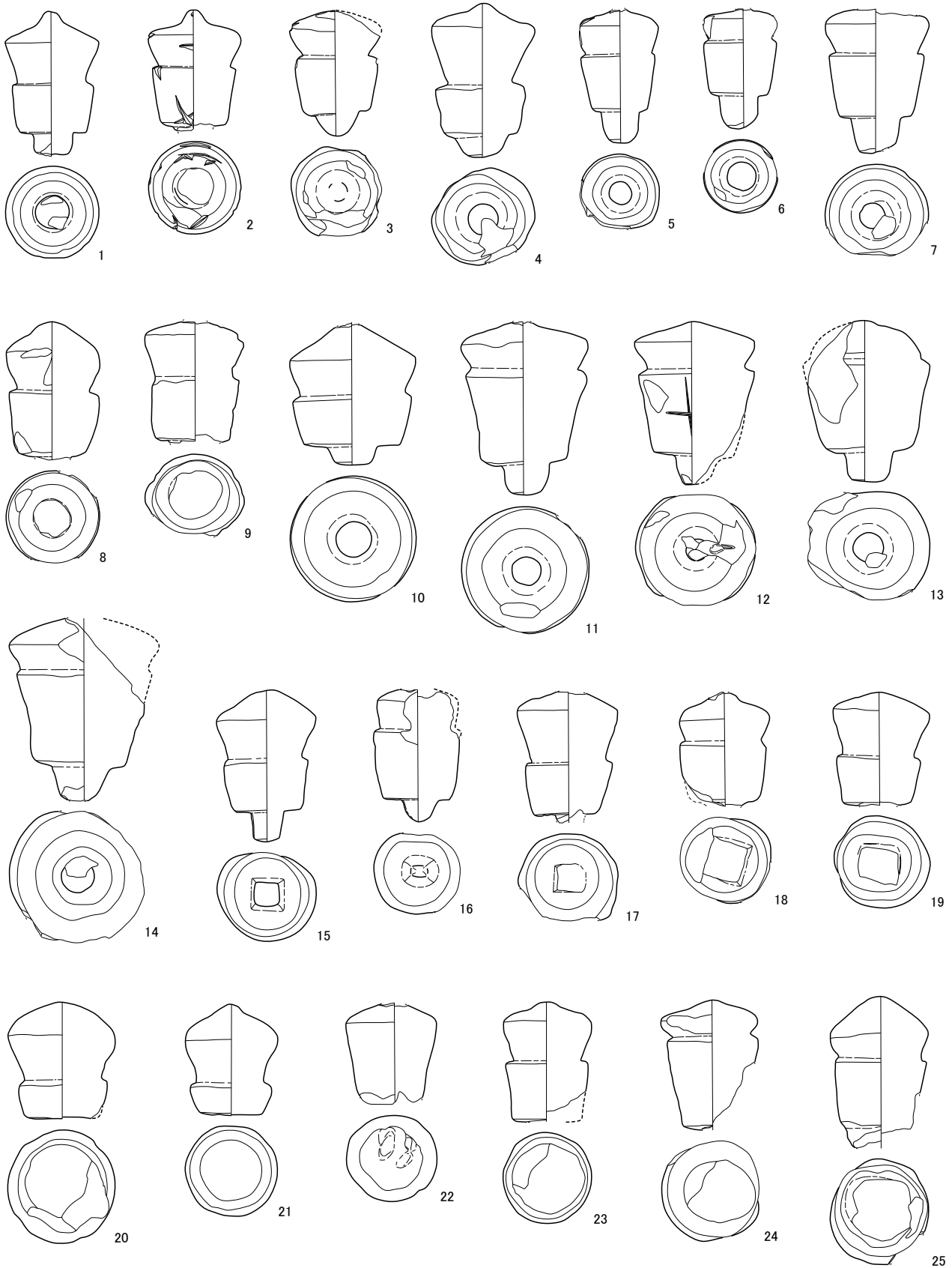
第189図 遺構外出土遺物実測図(10)
