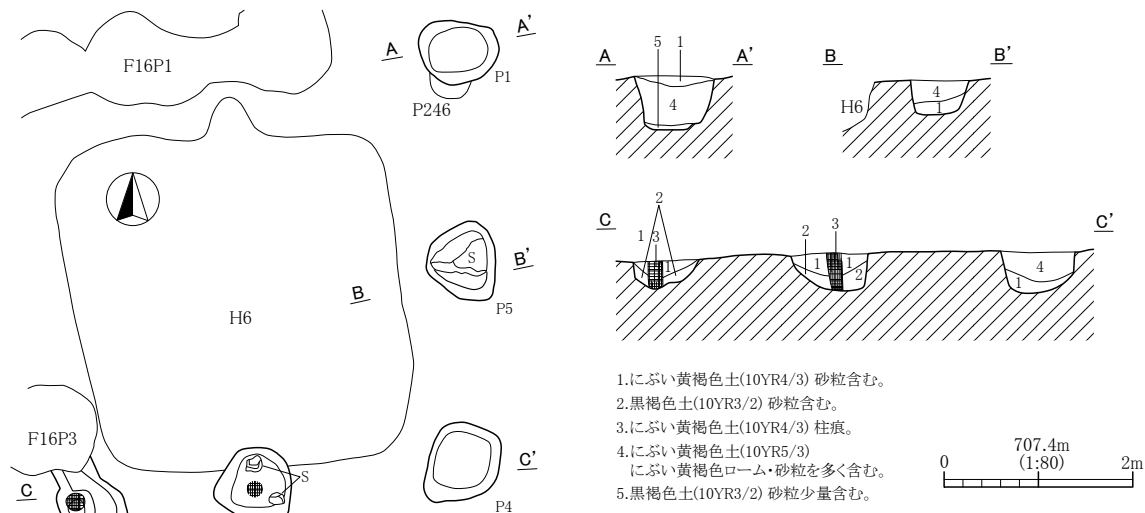
第117図 F 18号掘立柱建物跡実測図
