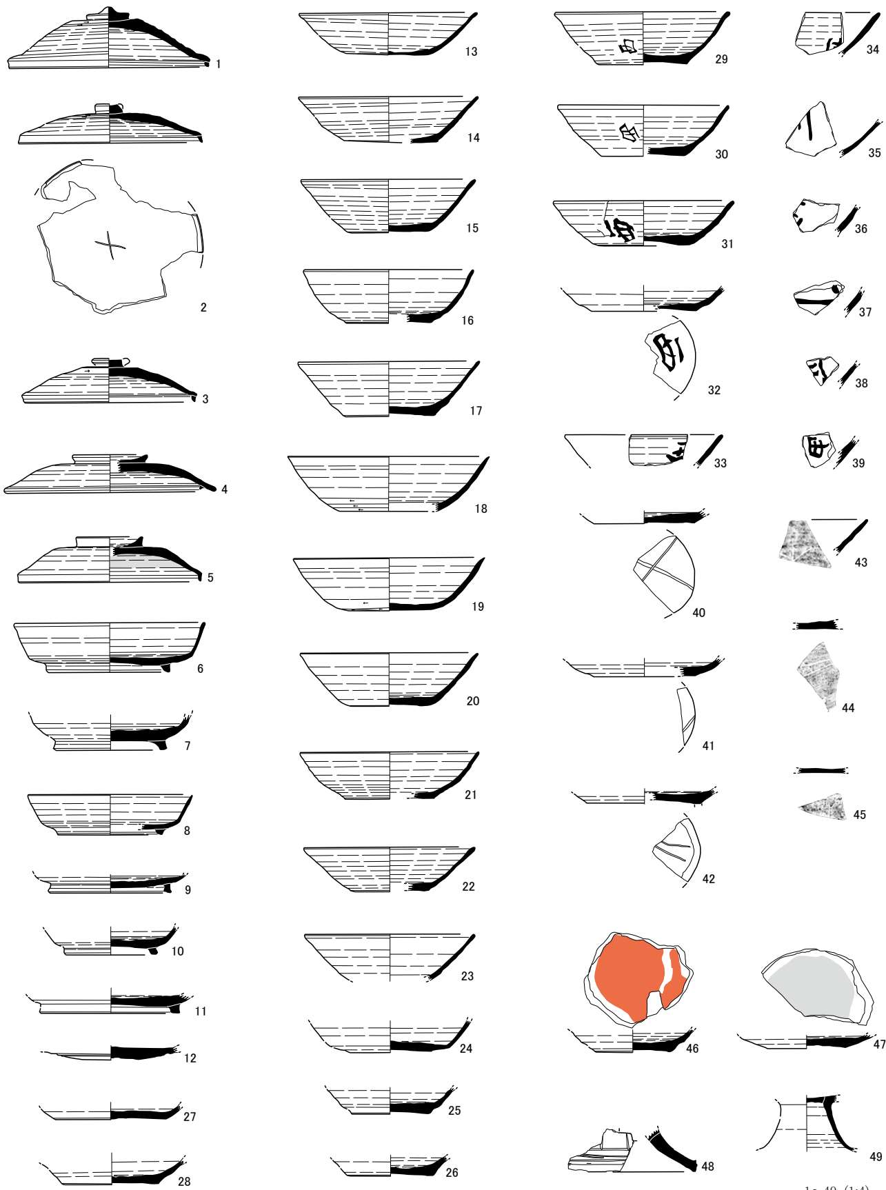
第36图 H20号住居跡出土遺物実測図(1)
