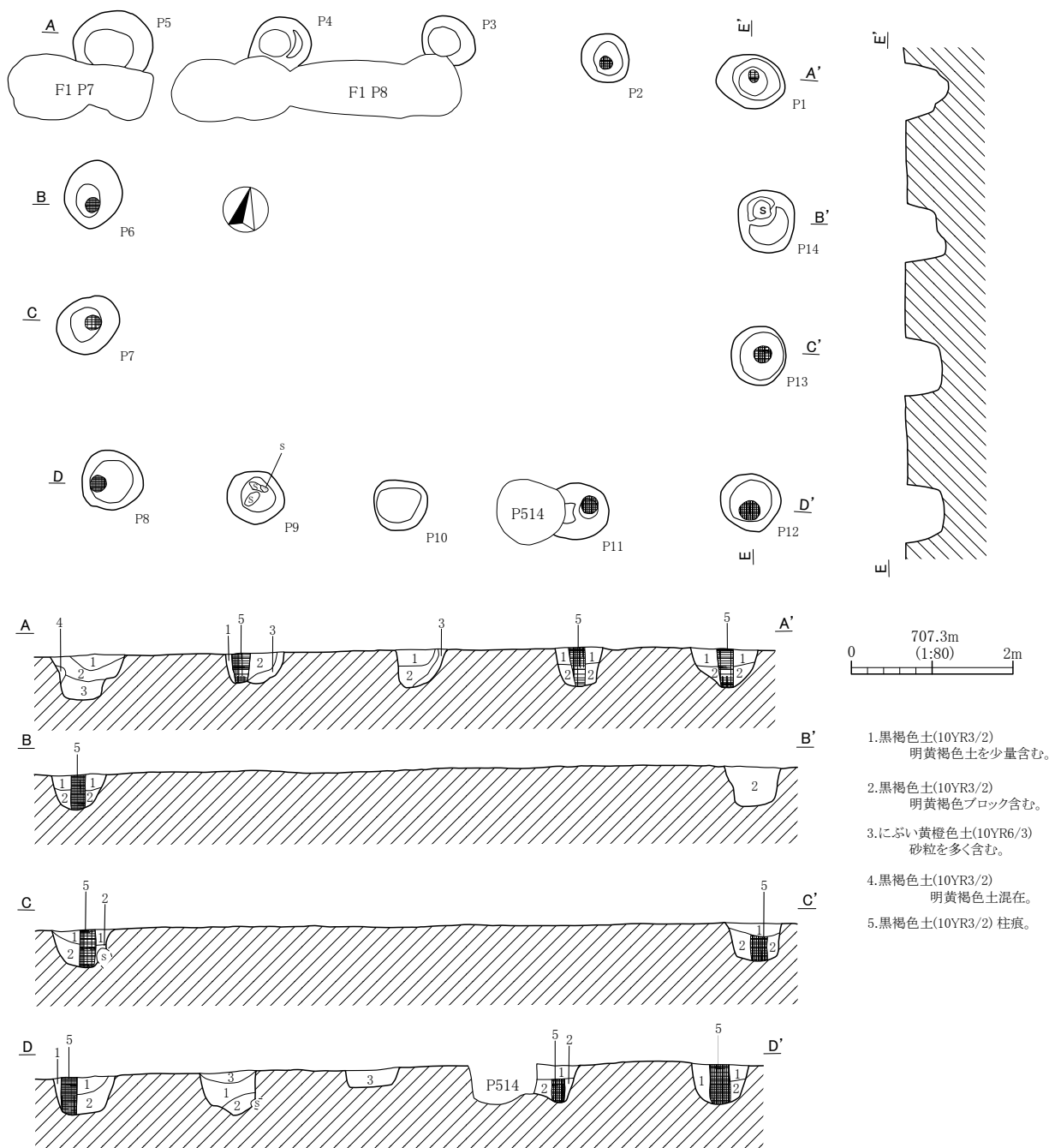
第101図 F 2号掘立柱建物跡実測図
