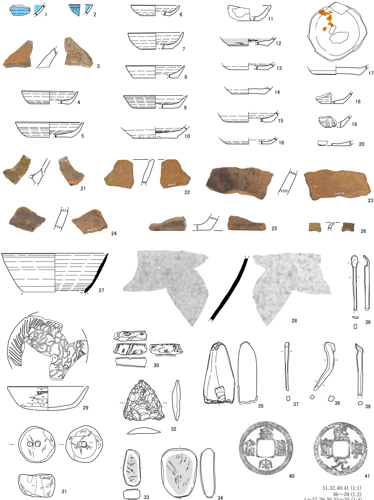
第144图 M9号沟状遺構出土遺物実測図
