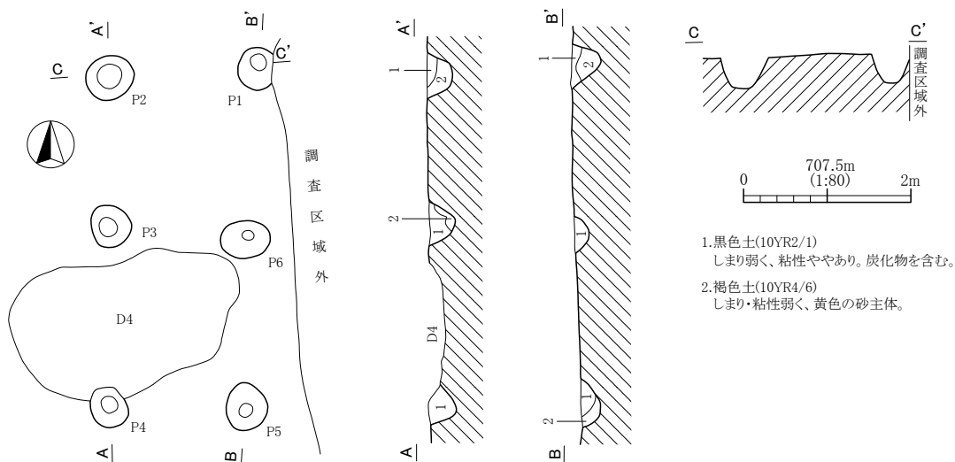
第104図 F 5号掘立柱建物跡実測図
