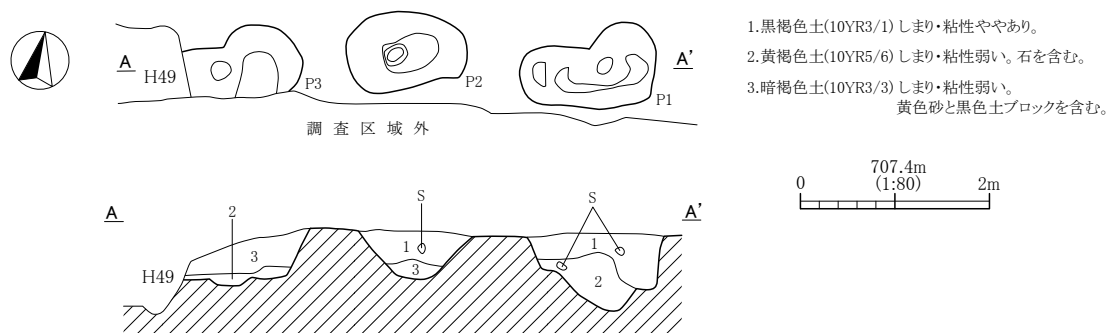
第130図 F 31号掘立柱建物跡実測図
