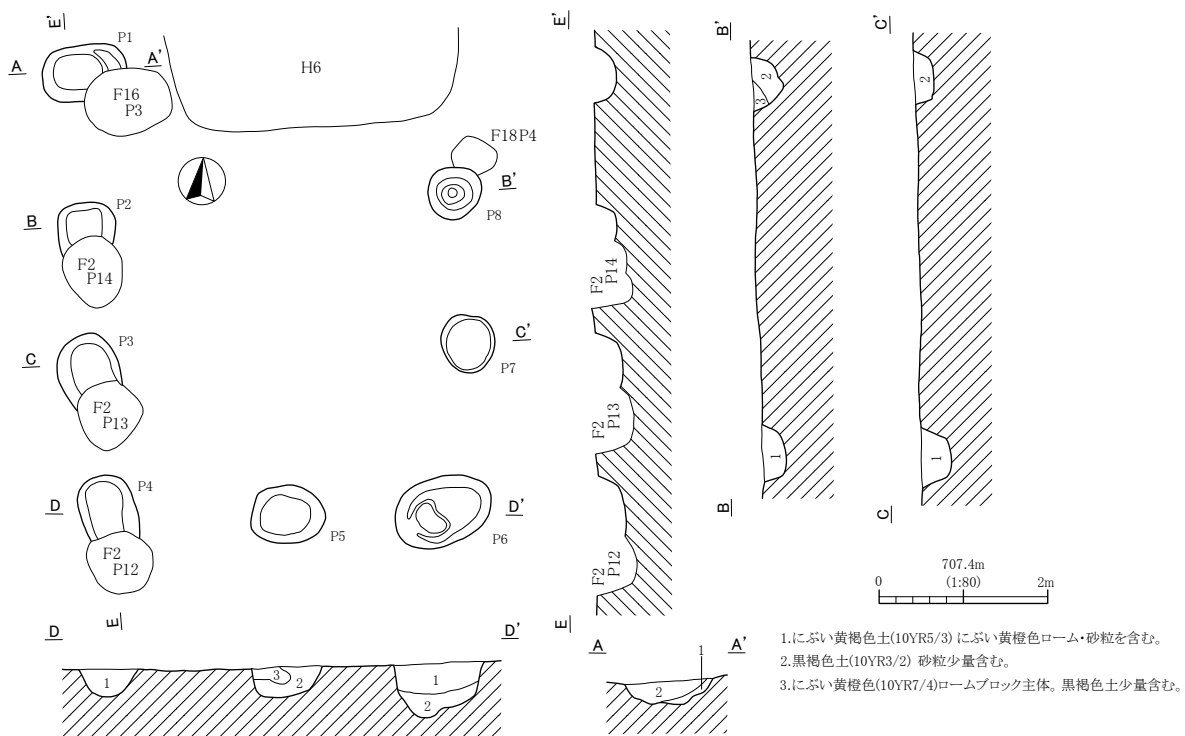
第114図 F 15号掘立柱建物跡実測図
