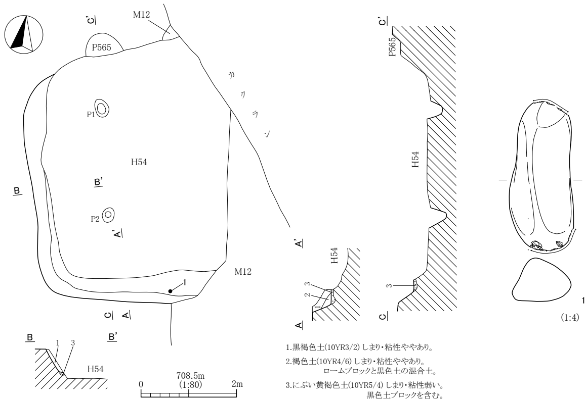
第90図 H57号住居跡及び出土遺物実測図
