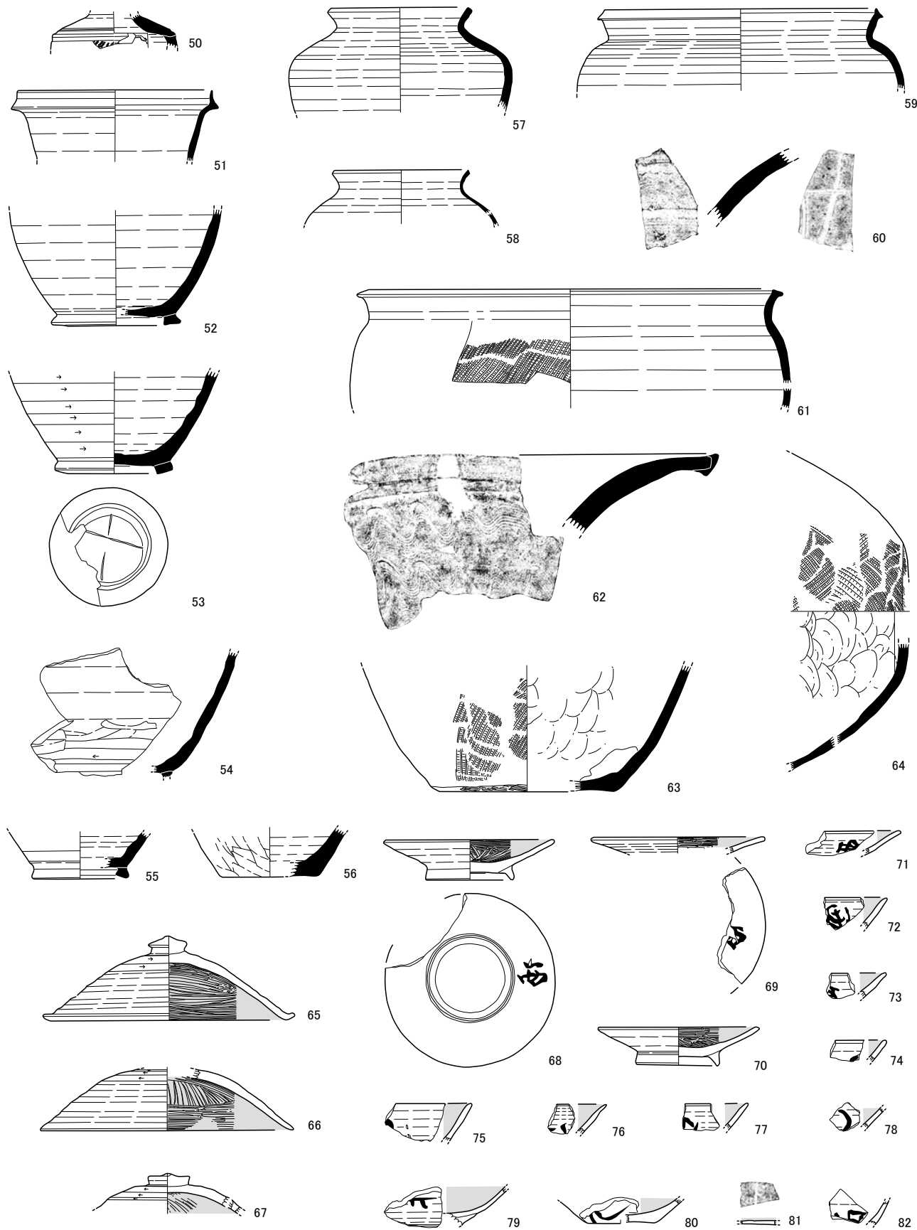
第37图 H20号住居跡出土遺物実測図(2)
