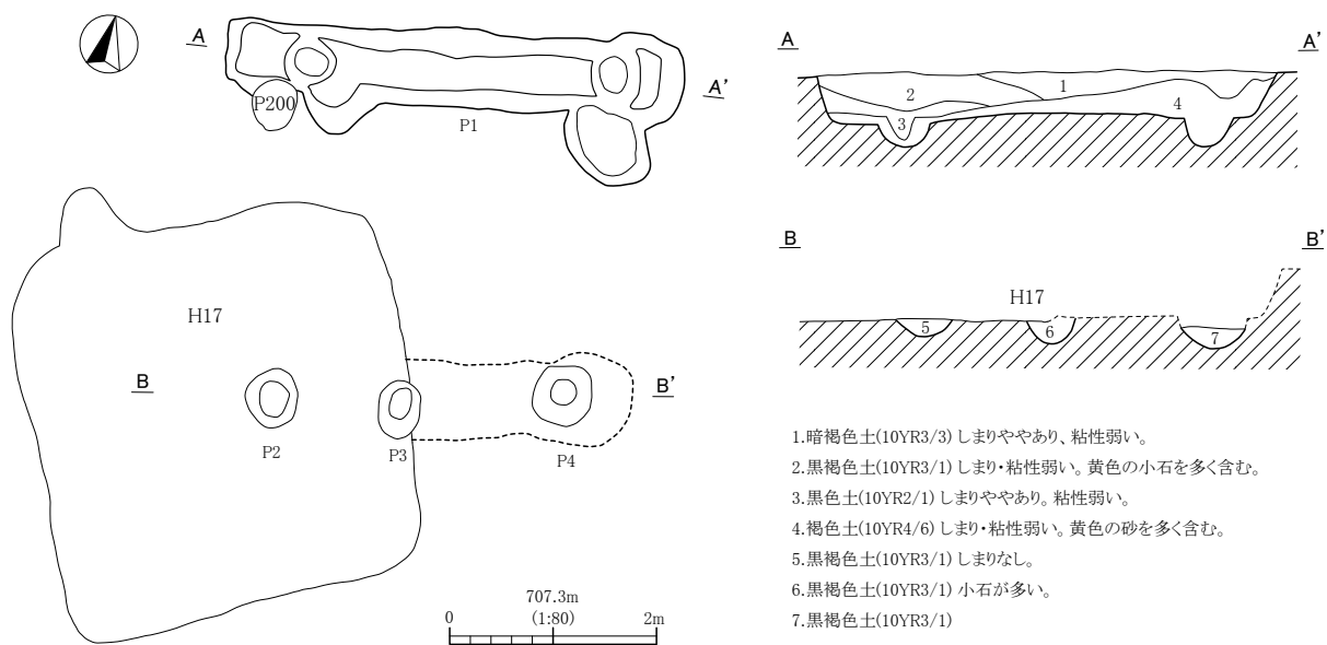
第125図 F 26号掘立柱建物跡実測図
