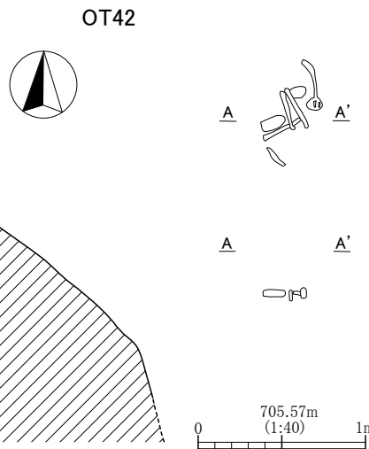
第 159 図 OT38 ~ 43 号火葬墓・土壙墓及び出土遺物実測図
