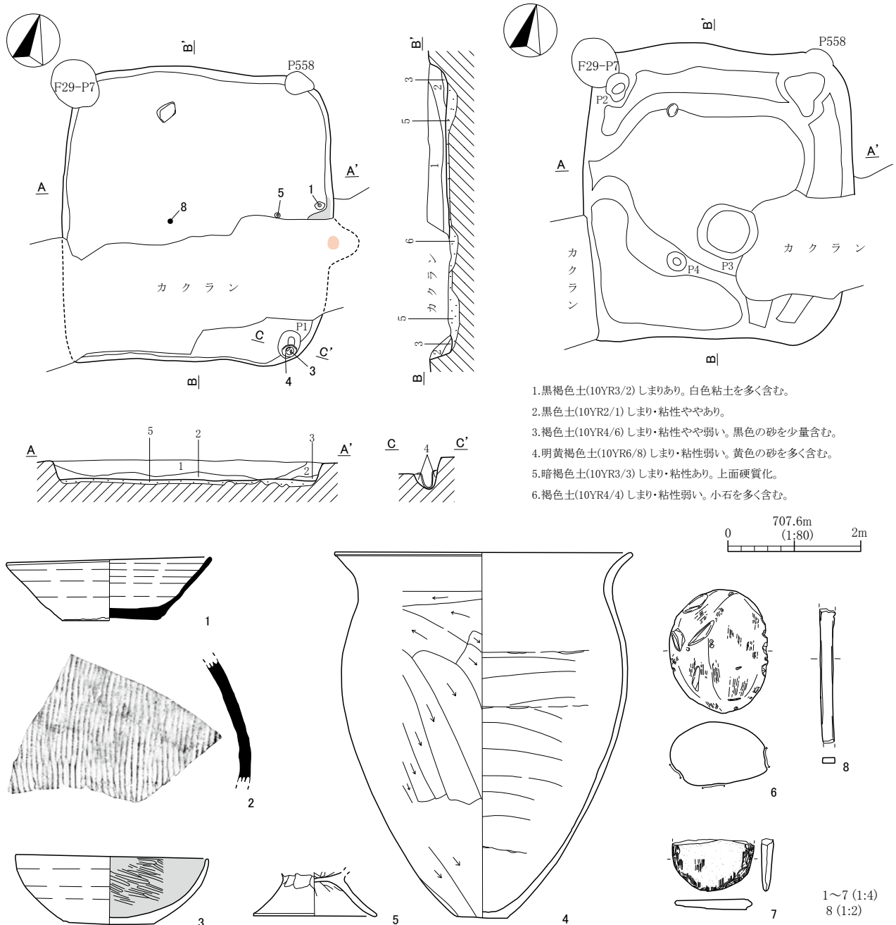
第69図 H42号住居跡及び出土遺物実測図
