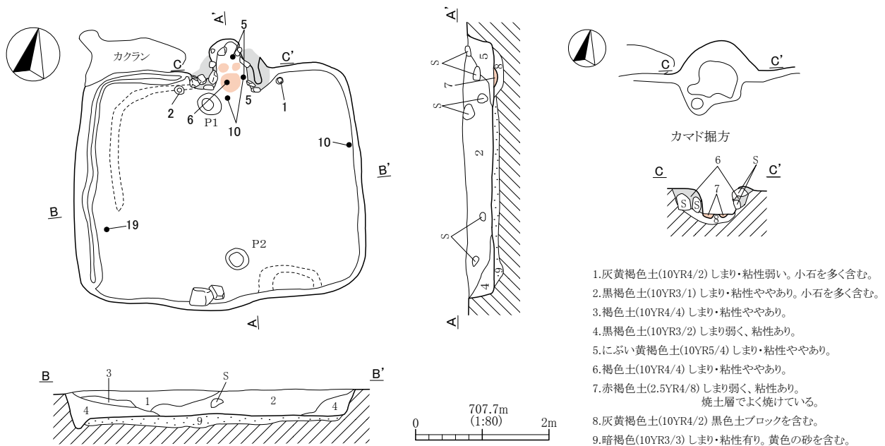
第67図 H41号住居跡実測図
