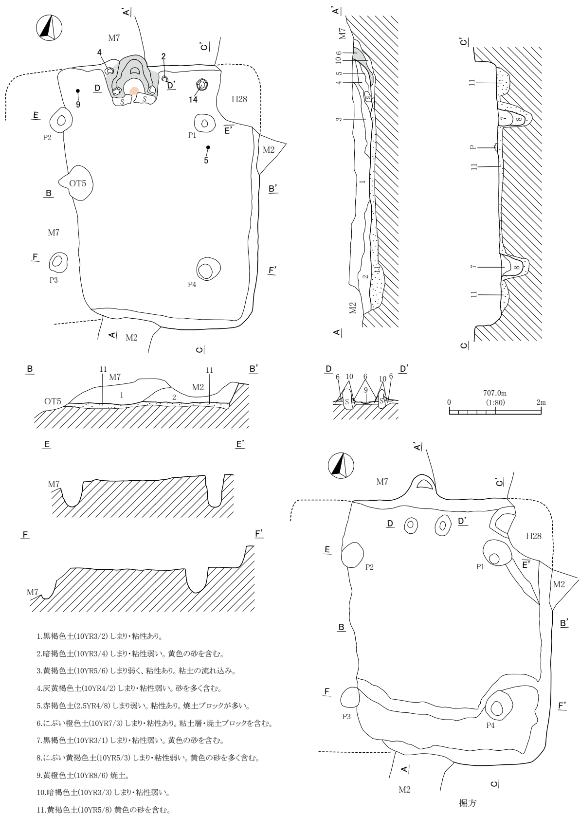
第56図 H33号住居跡実測図
