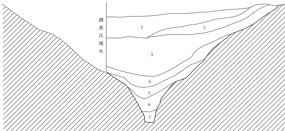
第143図 M9号溝状遺構実測図
