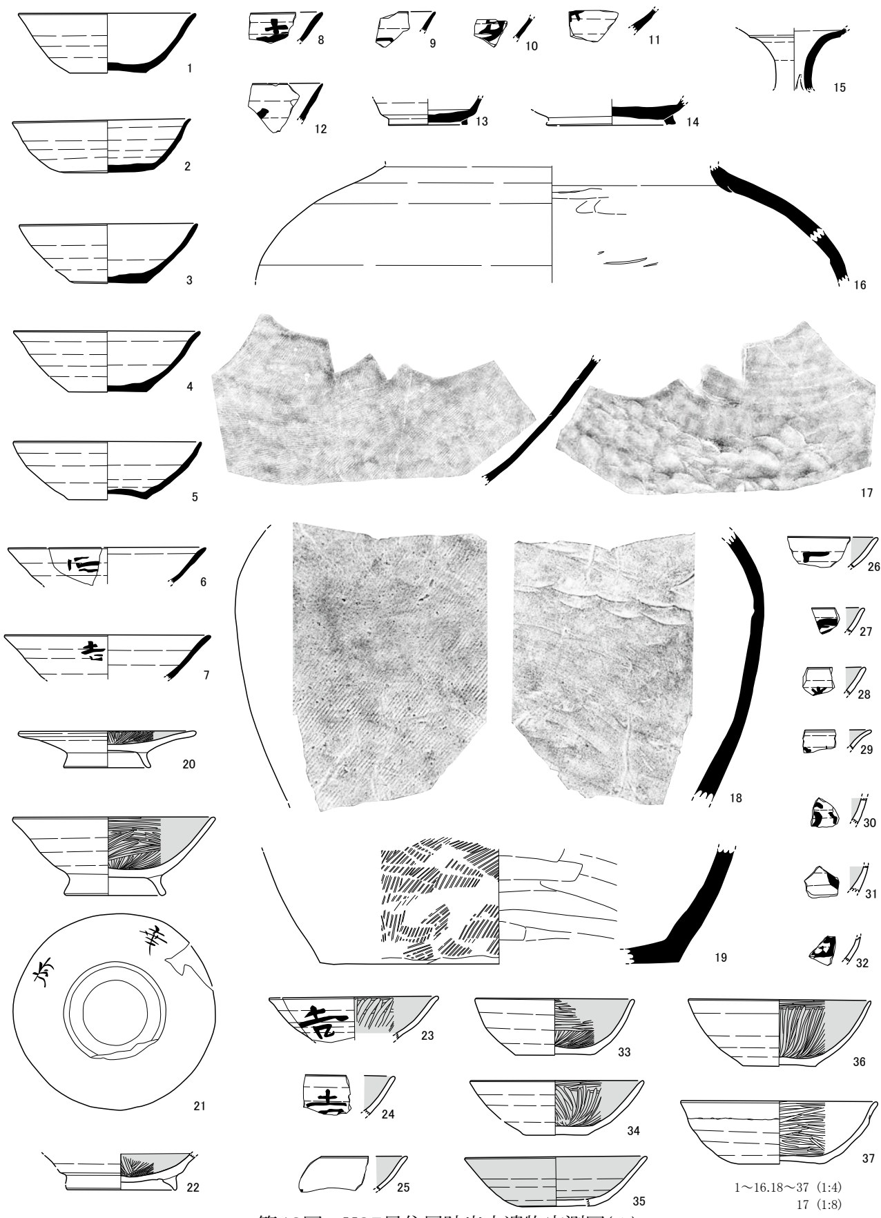
第48図 H27号住居跡出土遺物実測図(1)
