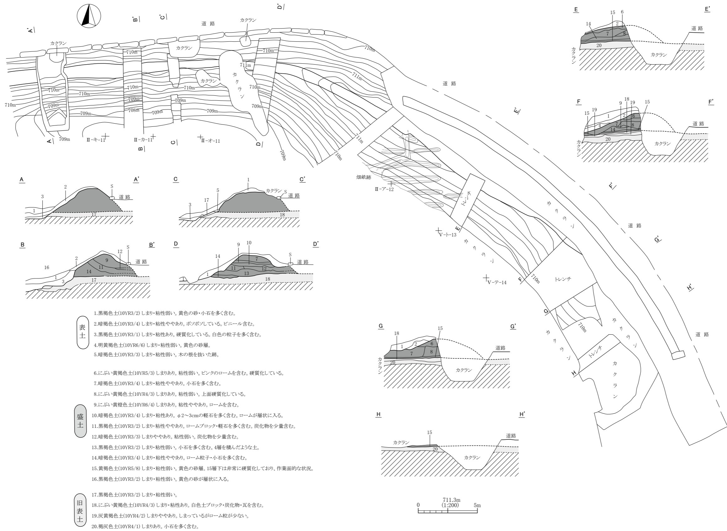
第178図 土塁実測図
