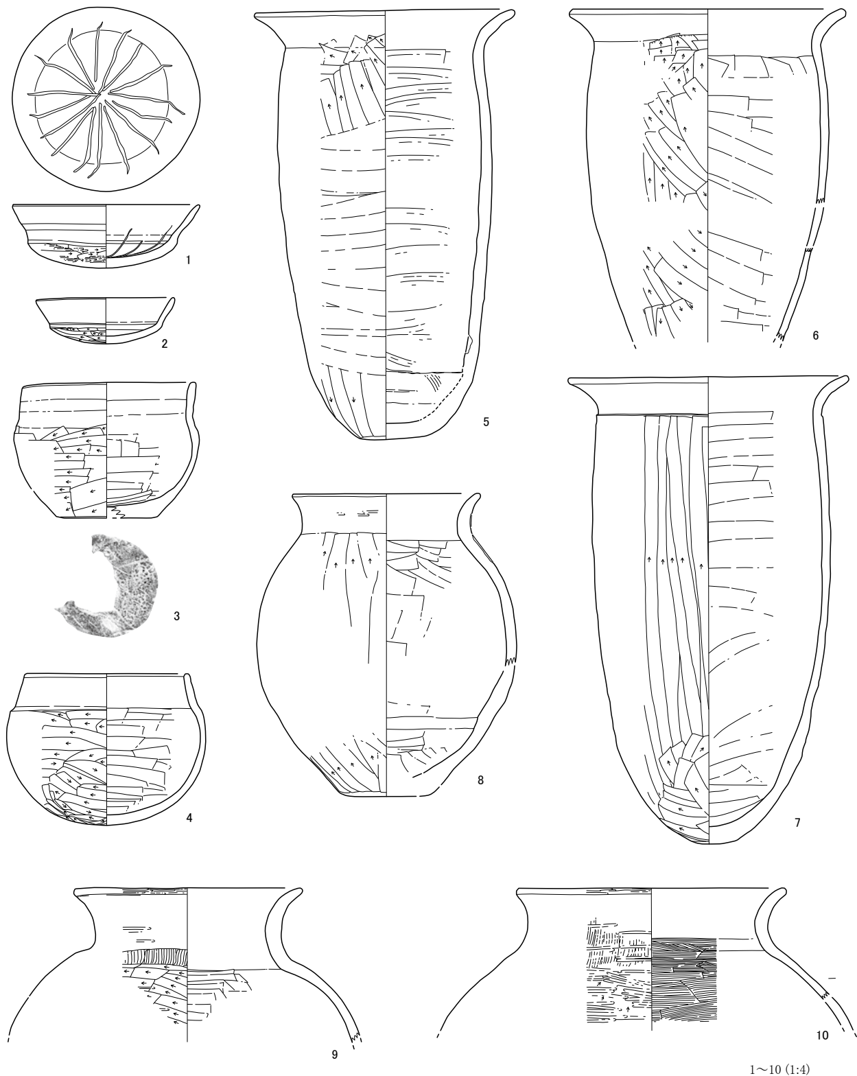
第75図 H46号住居跡出土遺物実測図(1)
