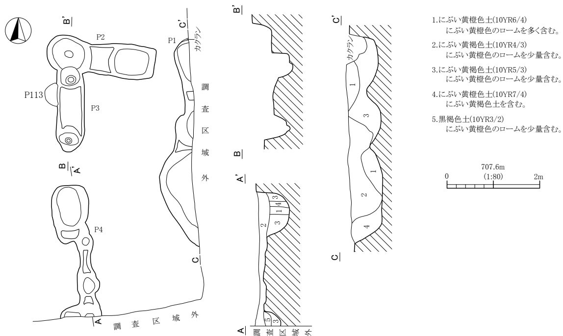
第123図 F24号掘立柱建物跡実測図
