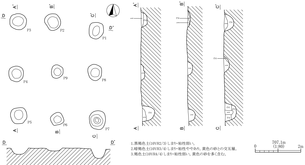
第118図 F 19号掘立柱建物跡実測図
