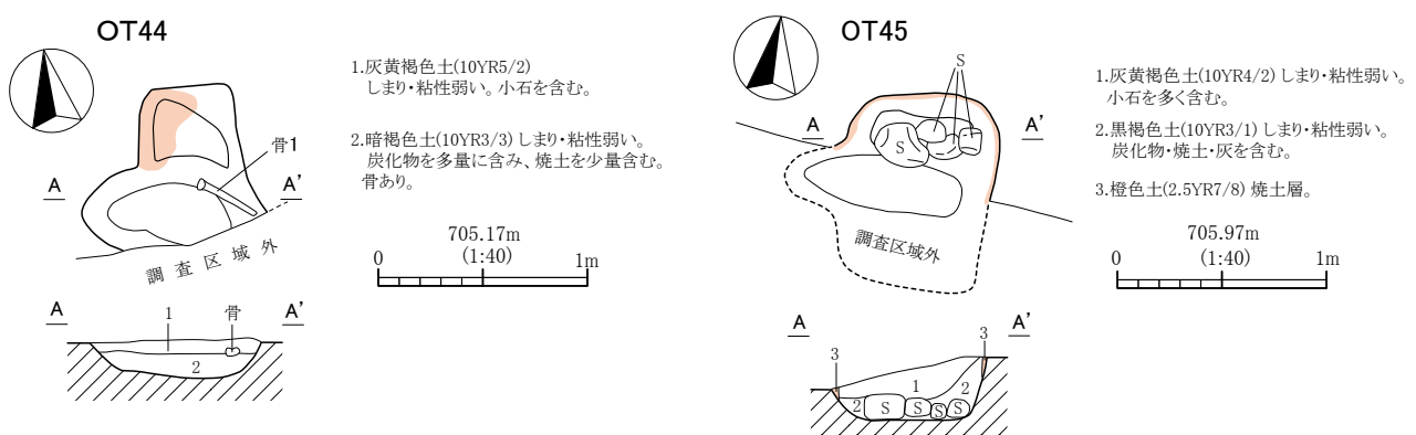
第160図 OT44・45号火葬墓実測図
