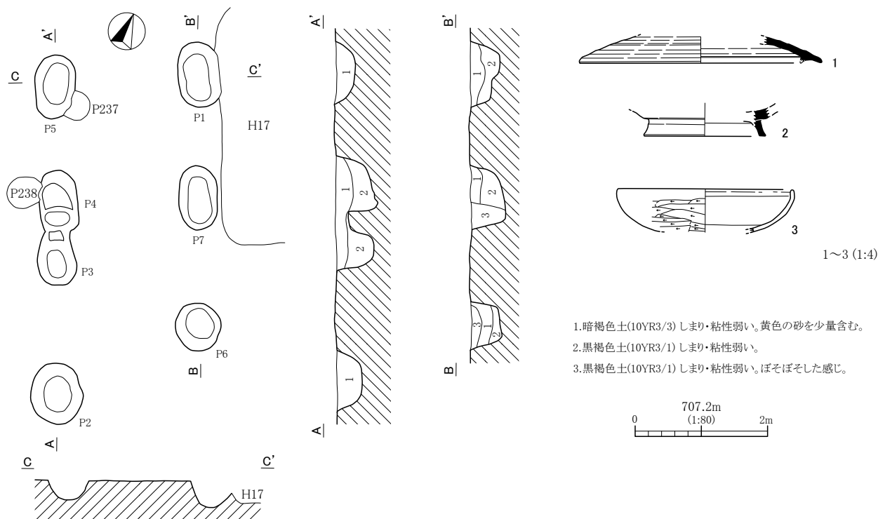
第116図 F17号掘立柱建物跡及び出土遺物実測図
