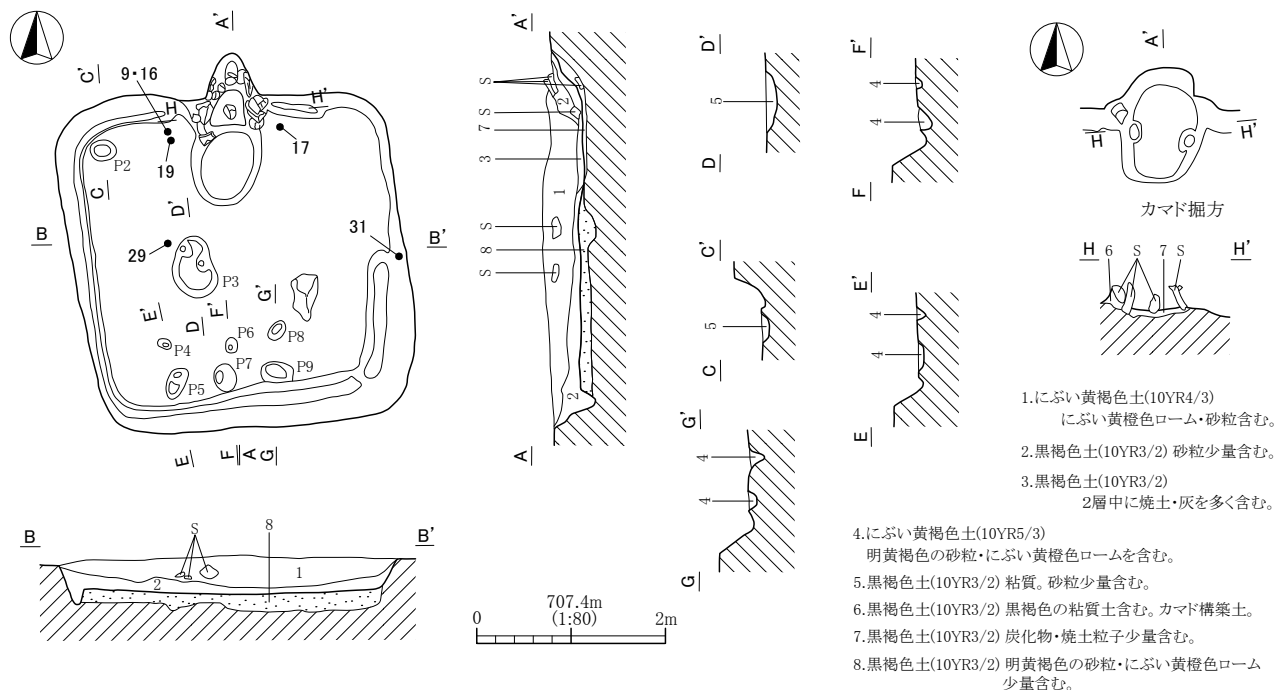
第15図 H6号住居跡実測図
