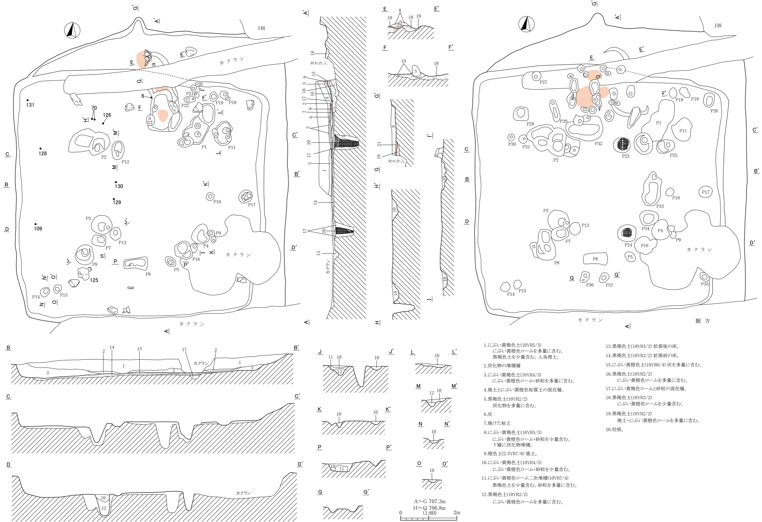
第35図 H20号住居跡実測図
