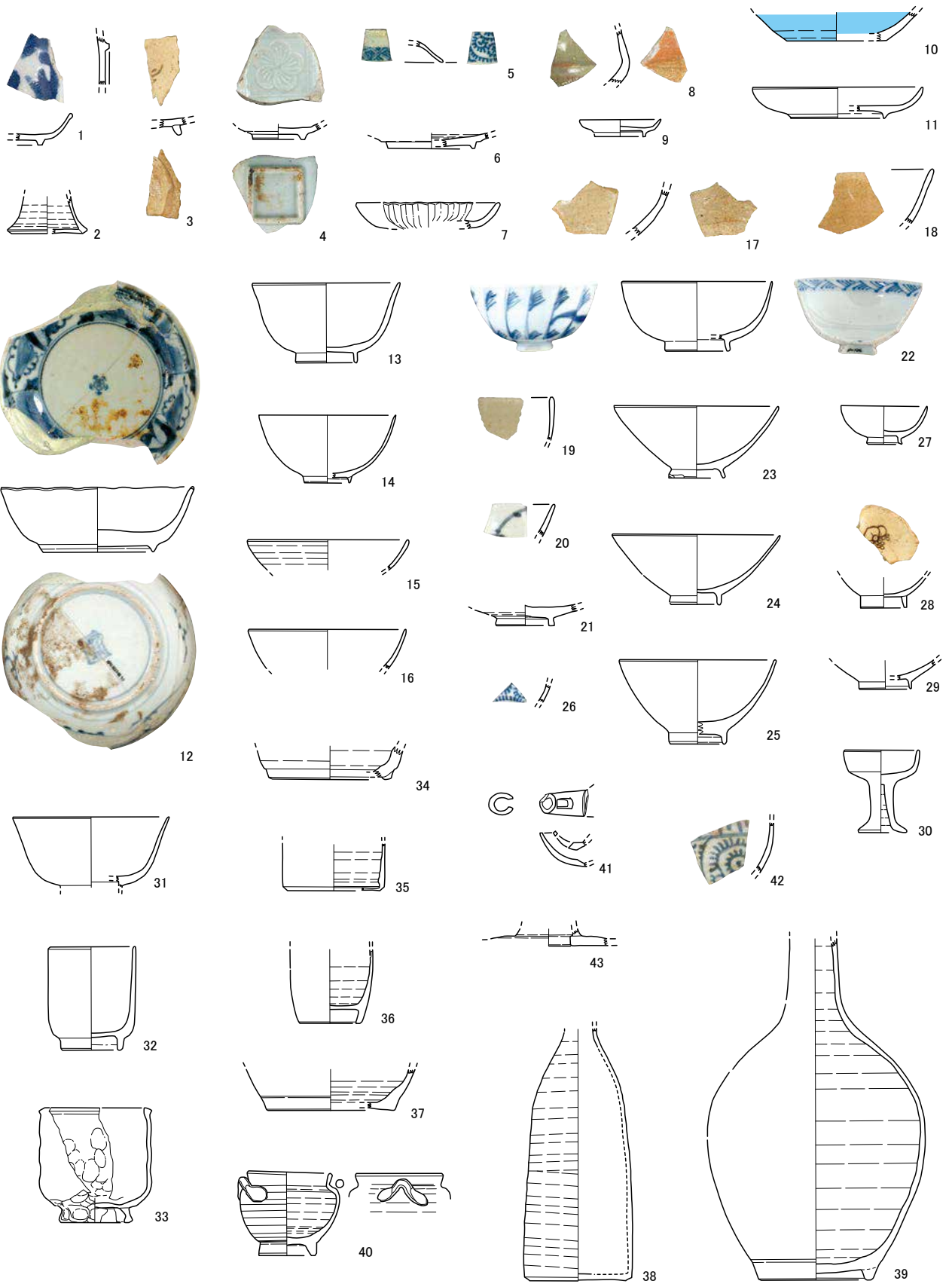
第182図 遺構外出土遺物実測図(3)
