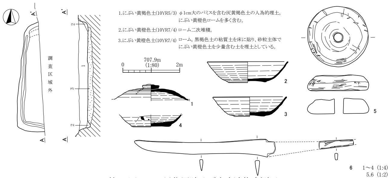
第27図 H14号住居跡及び出土遺物実測図
