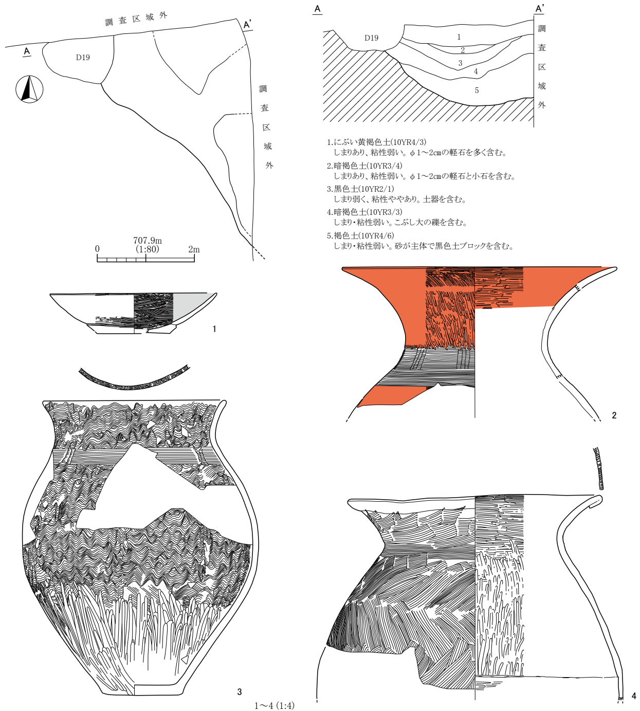
第140図 M1号溝状遺構及び出土遺物実測図
