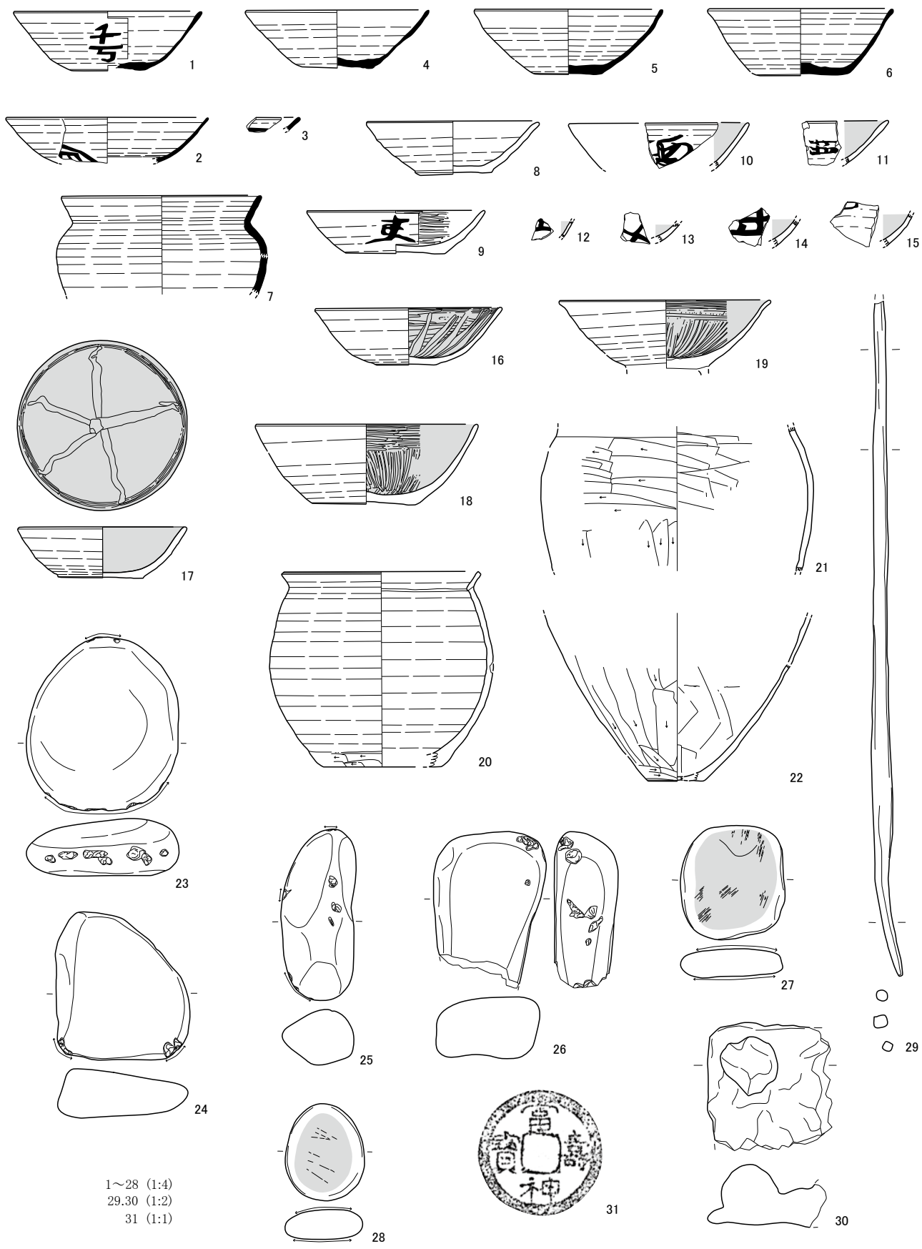
第16図 H6号住居跡出土遺物実測図
