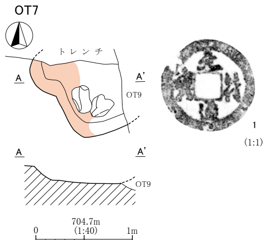
第151図 OT1~5・7・8号火葬墓及び出土遺物実測図
