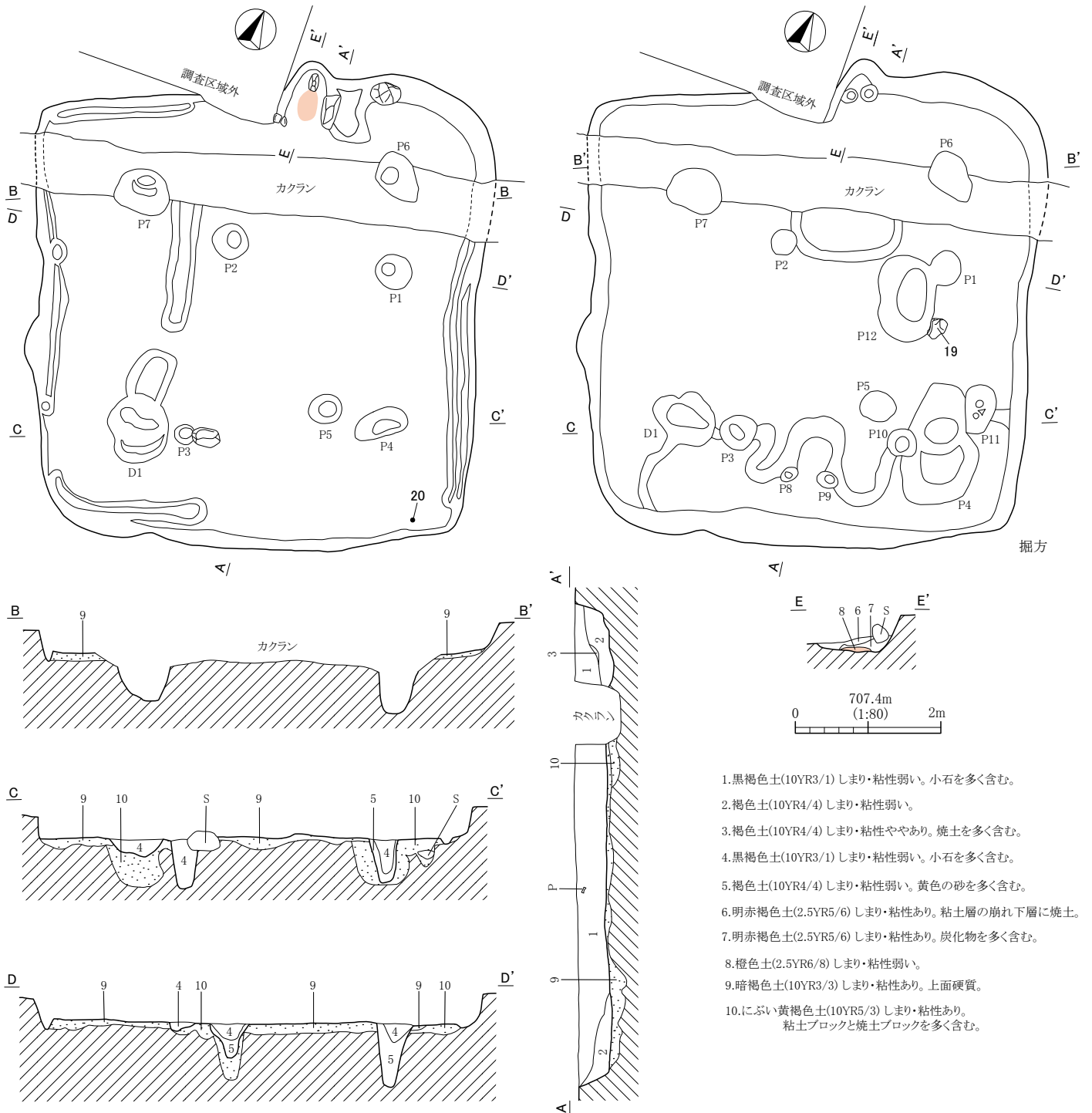
第7図 H2号住居跡実測図
