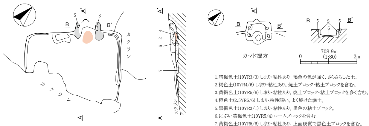
第86図 H53号住居跡実測図
