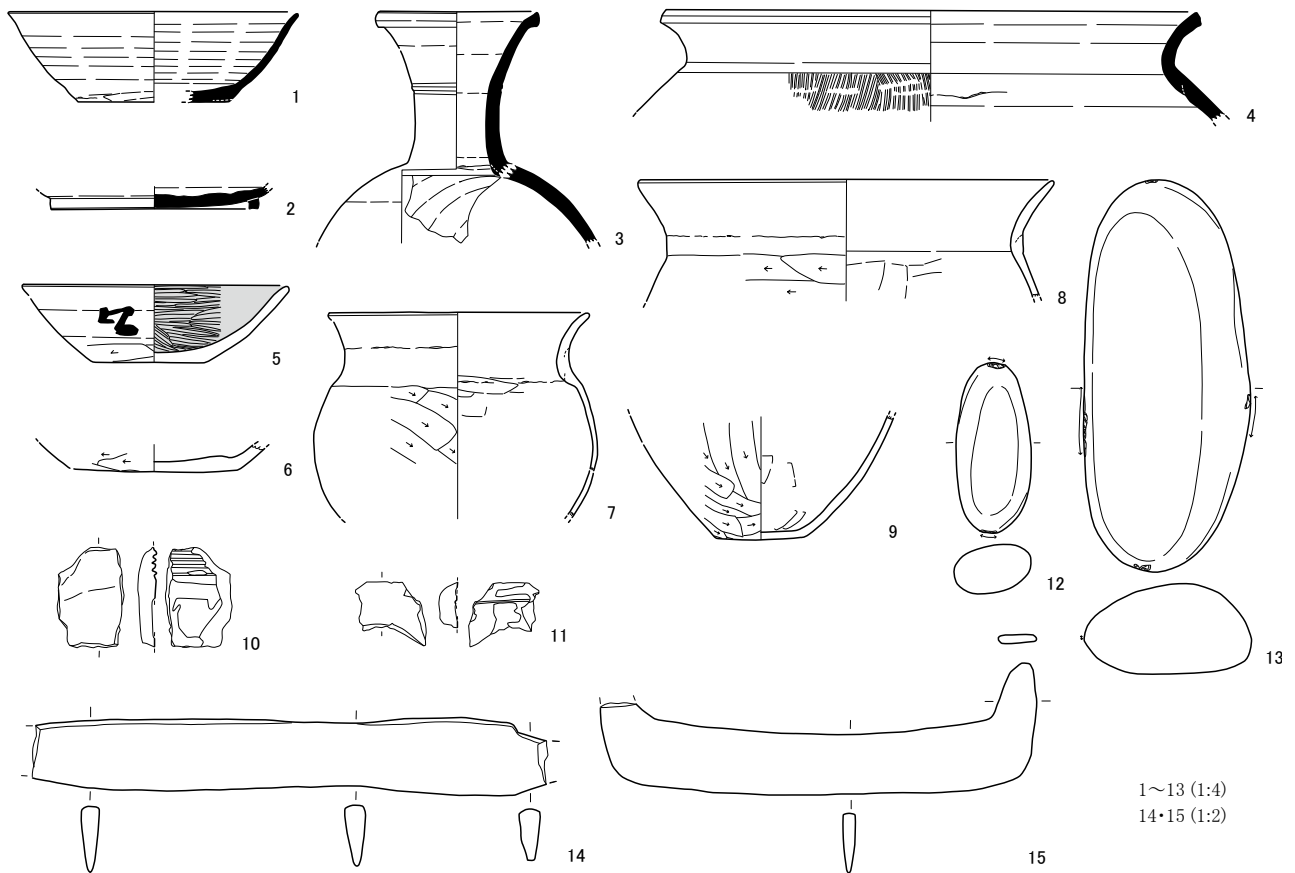
第59図 H35号住居跡出土遺物実測図
