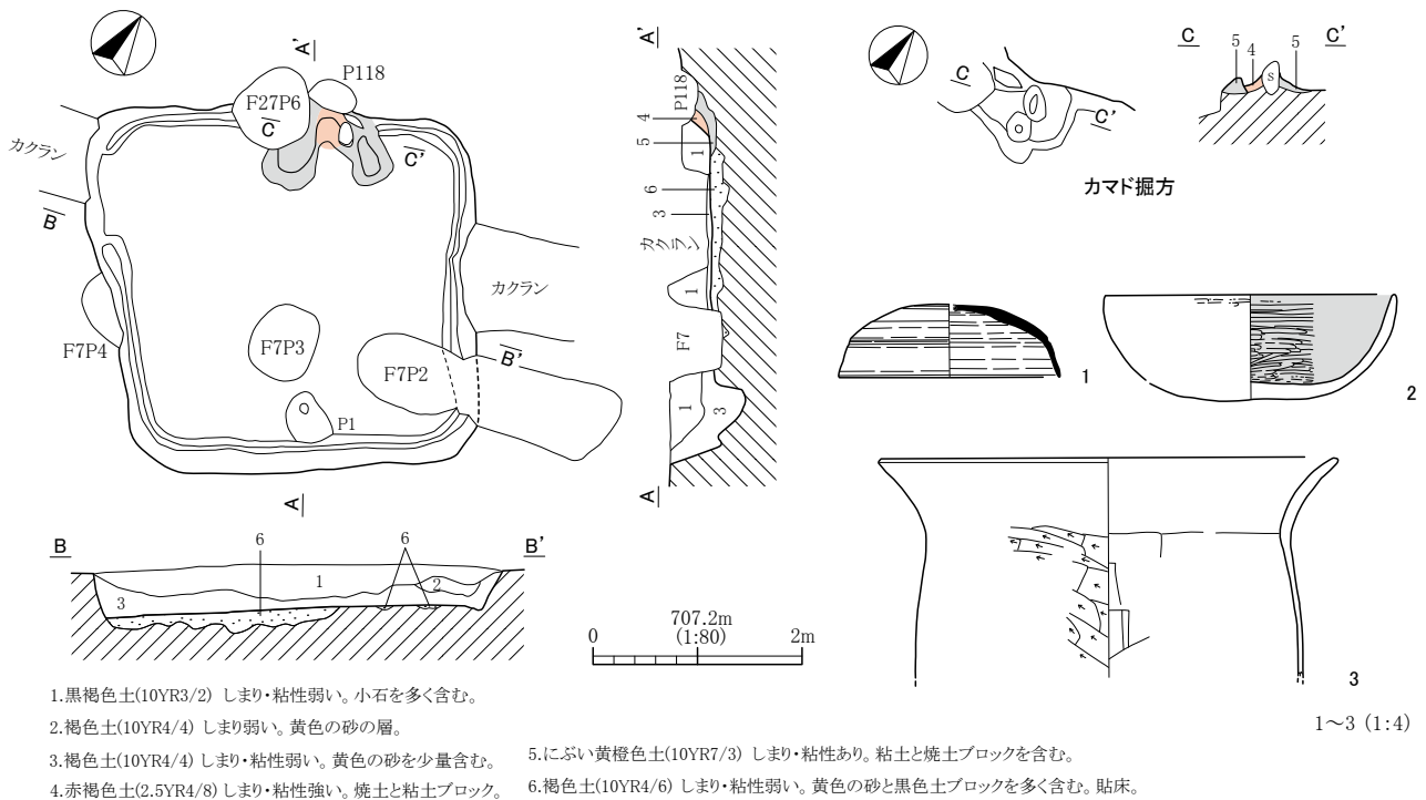
第28図 H15号住居跡及び出土遺物実測図
