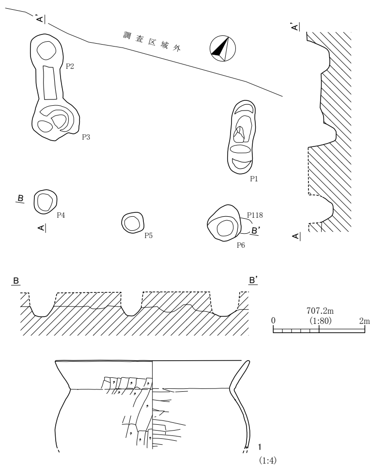
第126図 F 27号掘立柱建物跡及び出土遺物実測図
