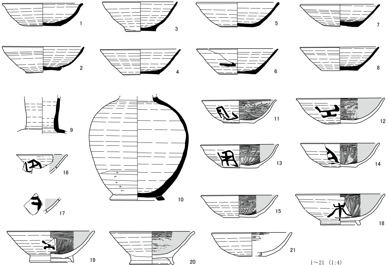
第62図 H37号住居跡及び出土遺物実測図
