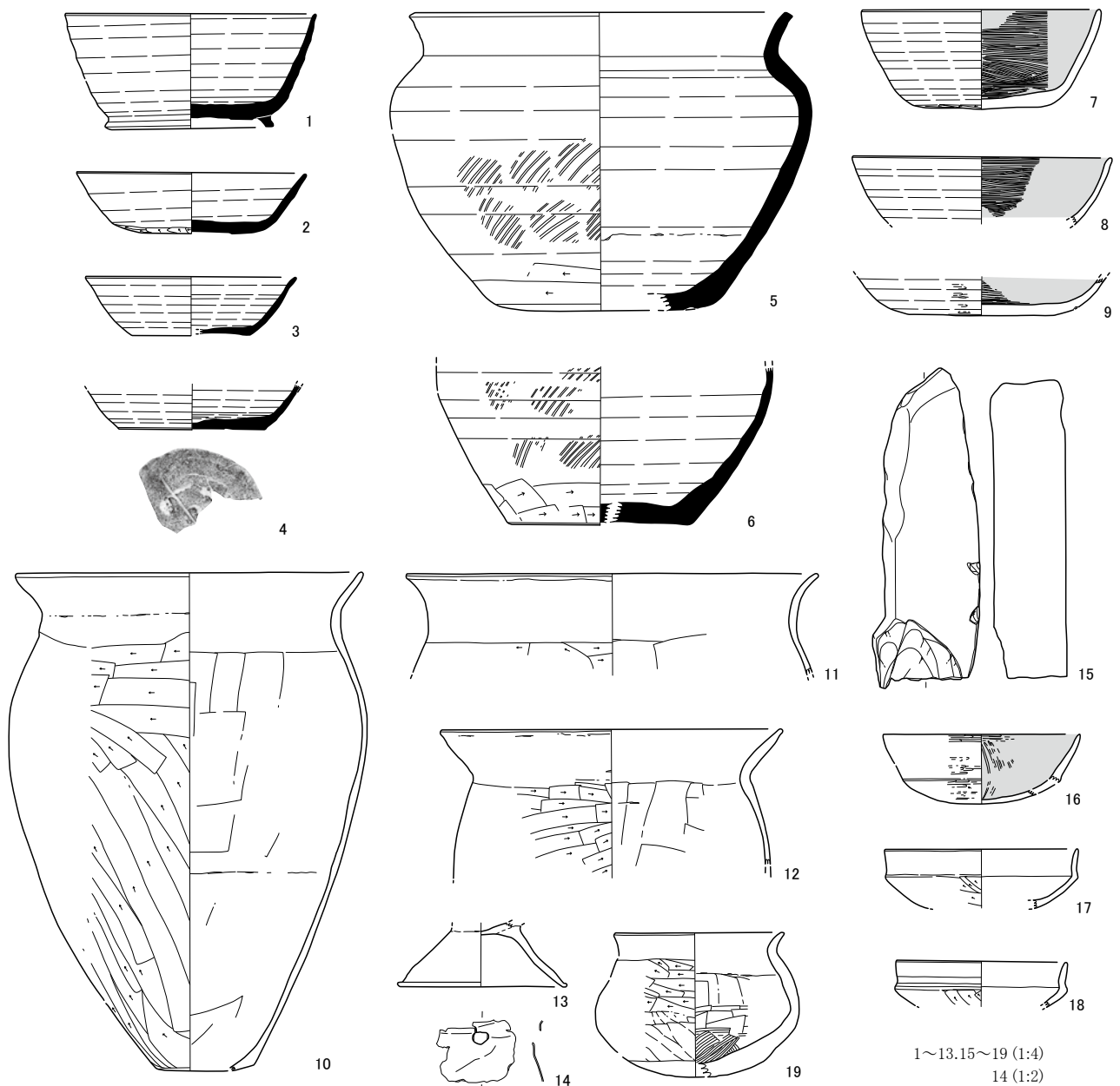
第68図 H41号住居跡出土遺物実測図
