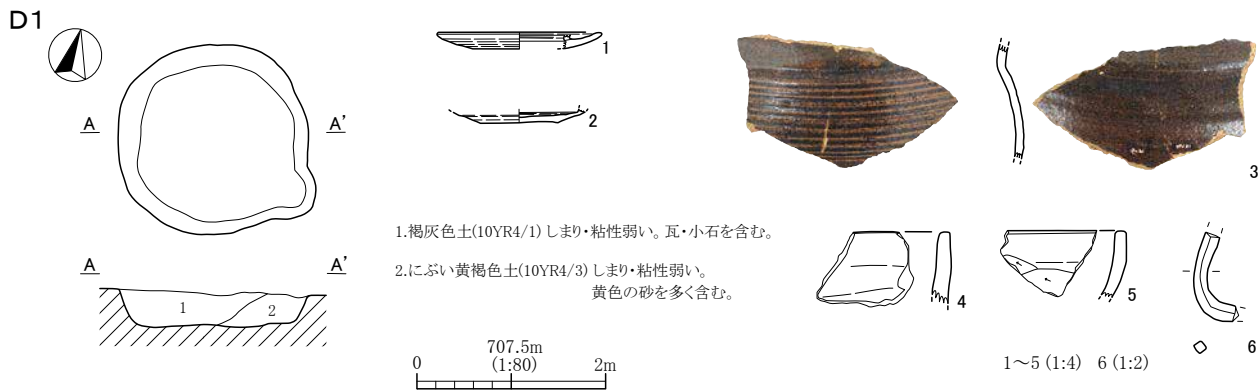
第131図 D1号土坑及び出土遺物実測図
