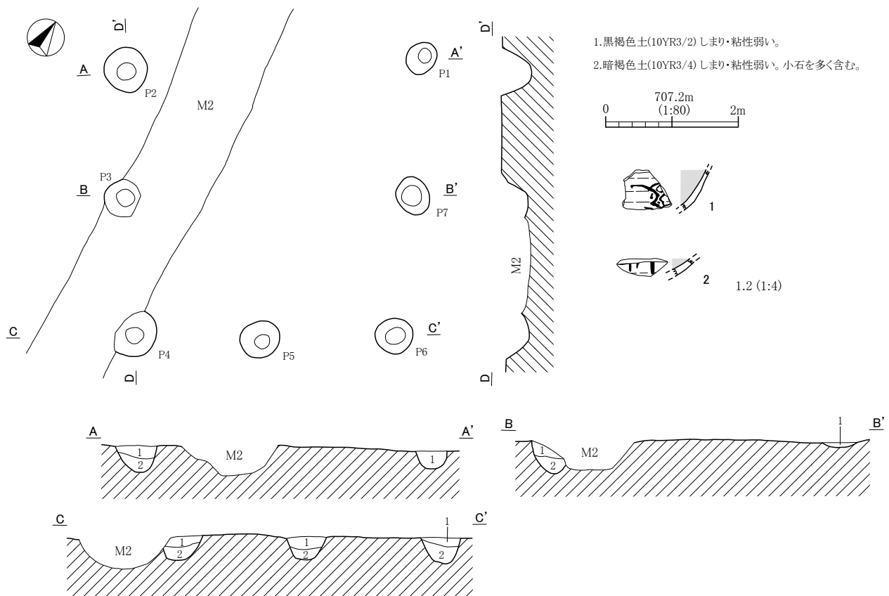
第112図 F 13号掘立柱建物跡及び出土遺物実測図
