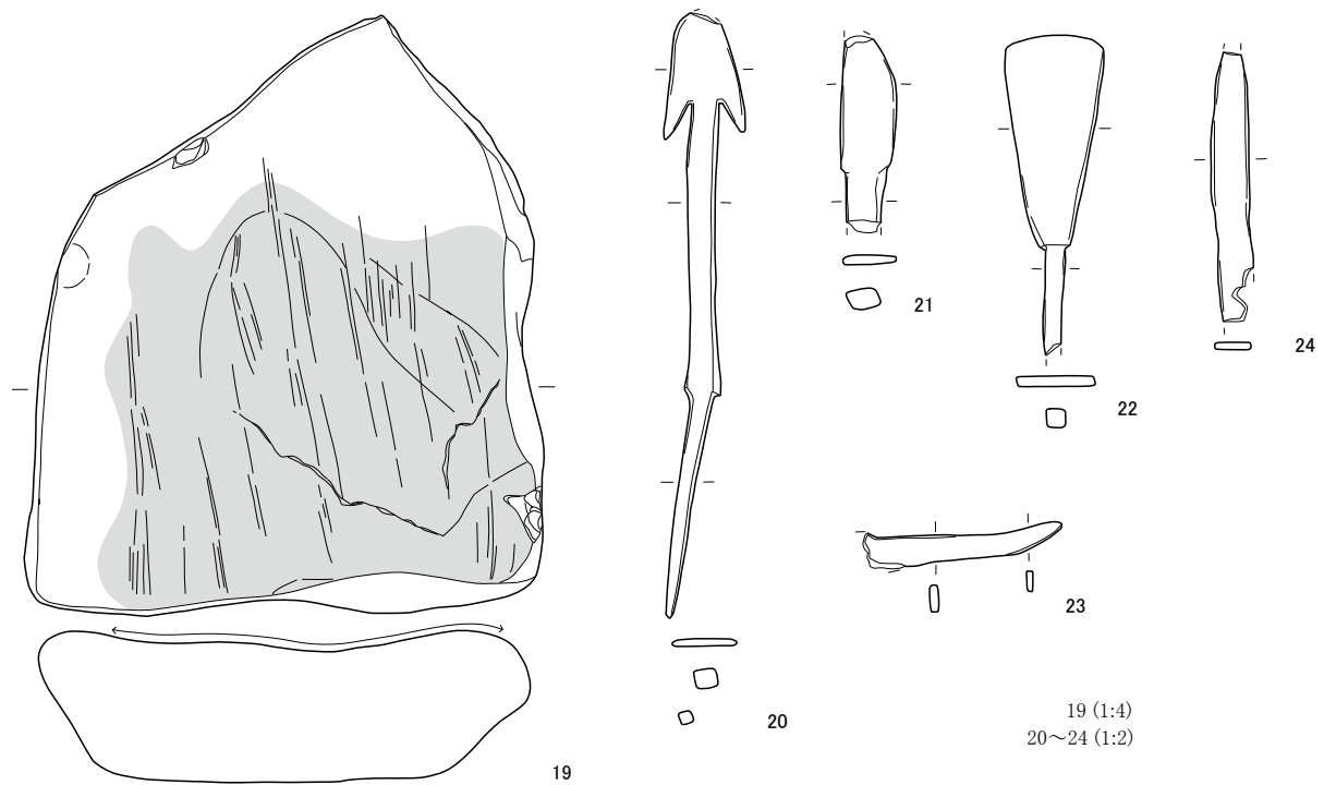
第9図 H2号住居跡出土遺物実測図(2)
