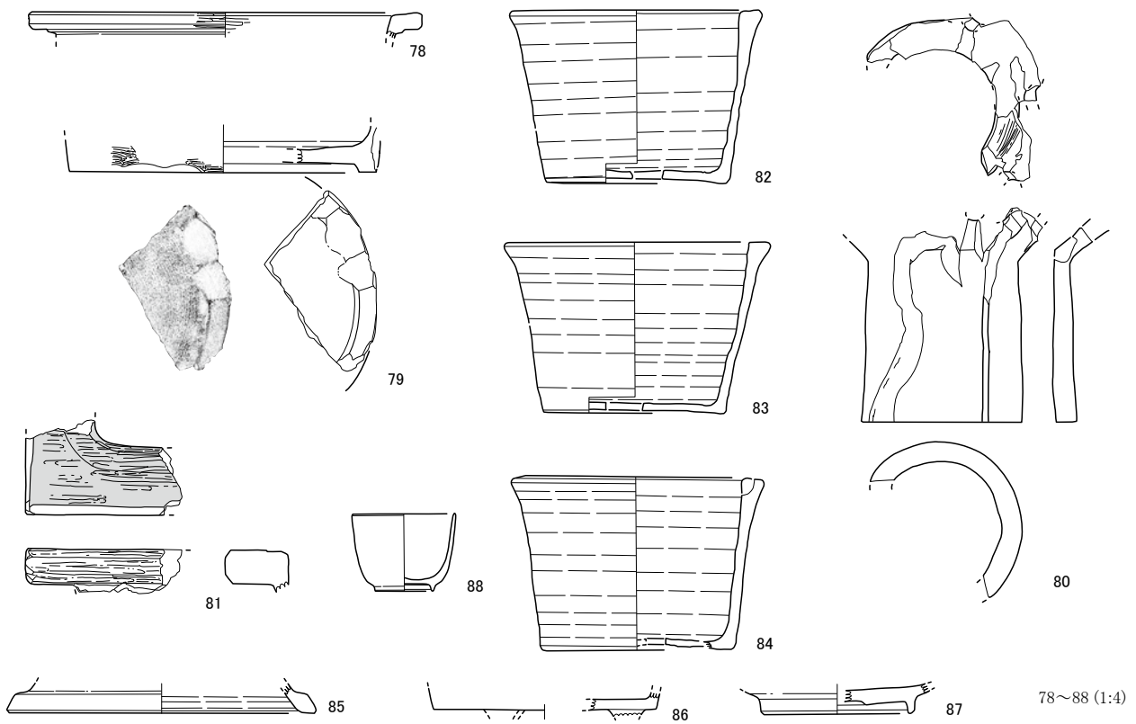
第185図 遺構外出土遺物実測図(6)
