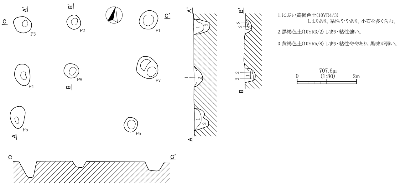
第128図 F 29号掘立柱建物跡実測図
