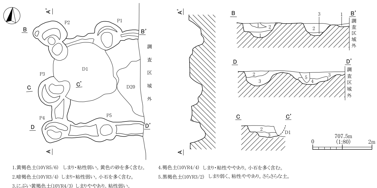
第102図 F 3号掘立柱建物跡実測図
