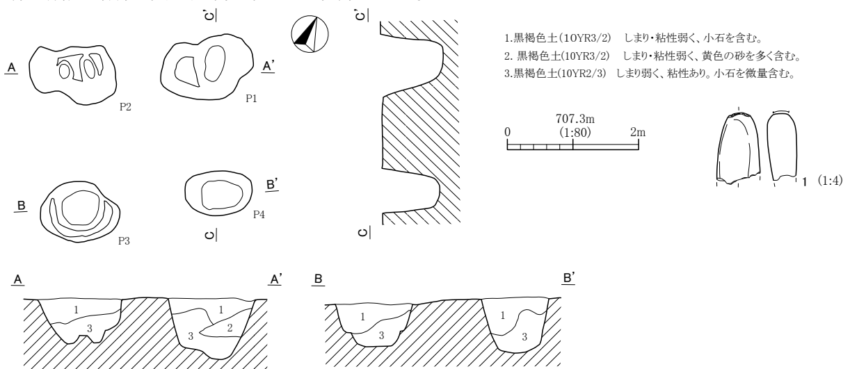
第110図 F 11号掘立柱建物跡及び出土遺物実測図
