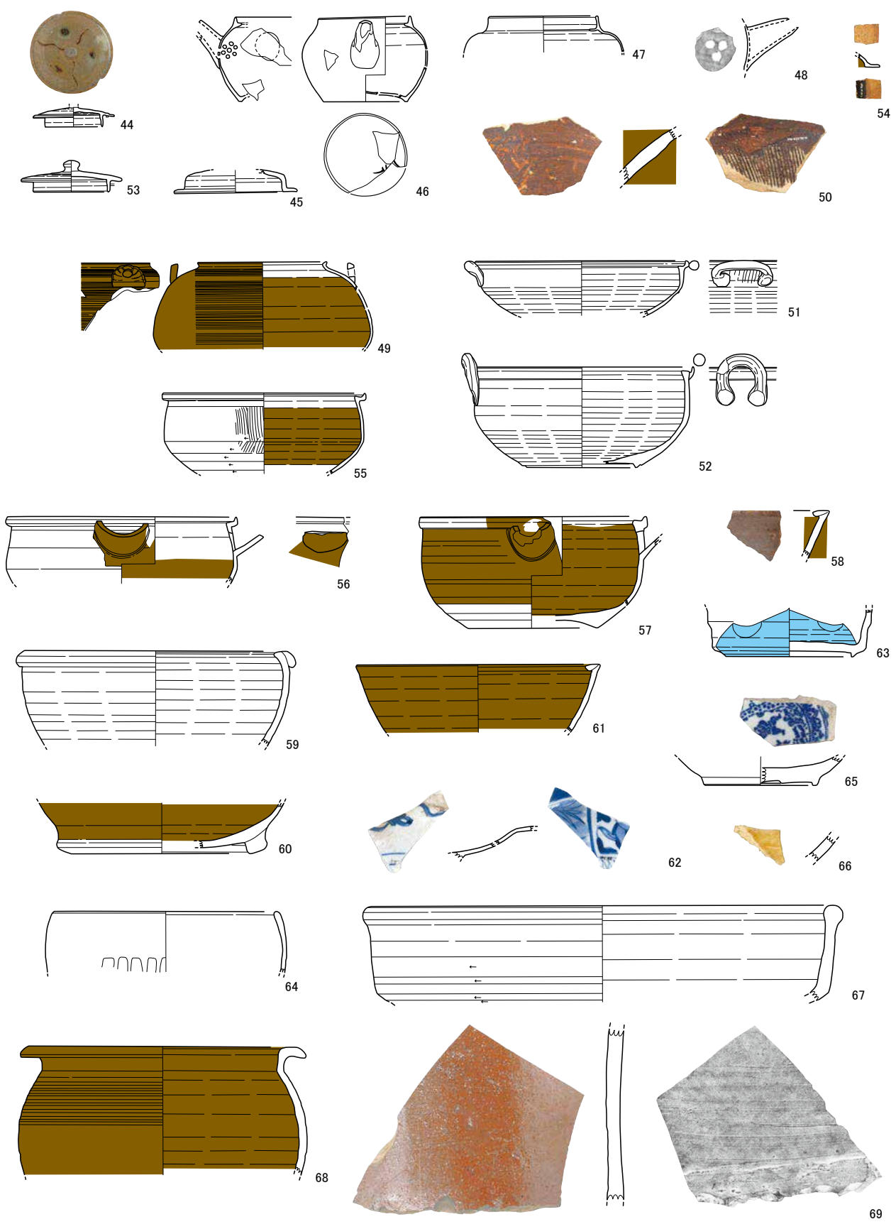
第183図 遺構外出土遺物実測図(4)
