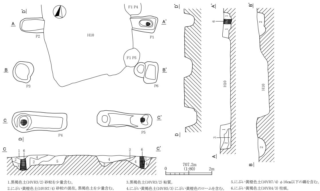
第113図 F 14号掘立柱建物跡実測図
