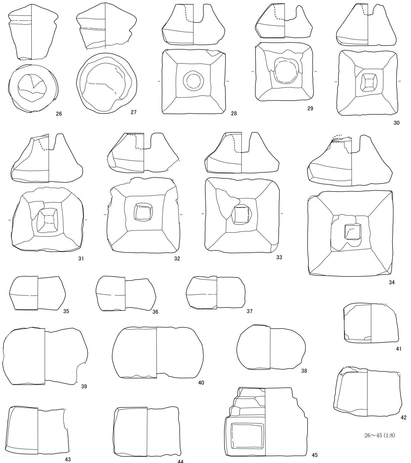
第190図 遺構外出土遺物実測図(11)
