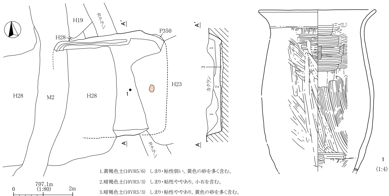
第 55 図 H32 号住居跡及び出土遺物実測図
