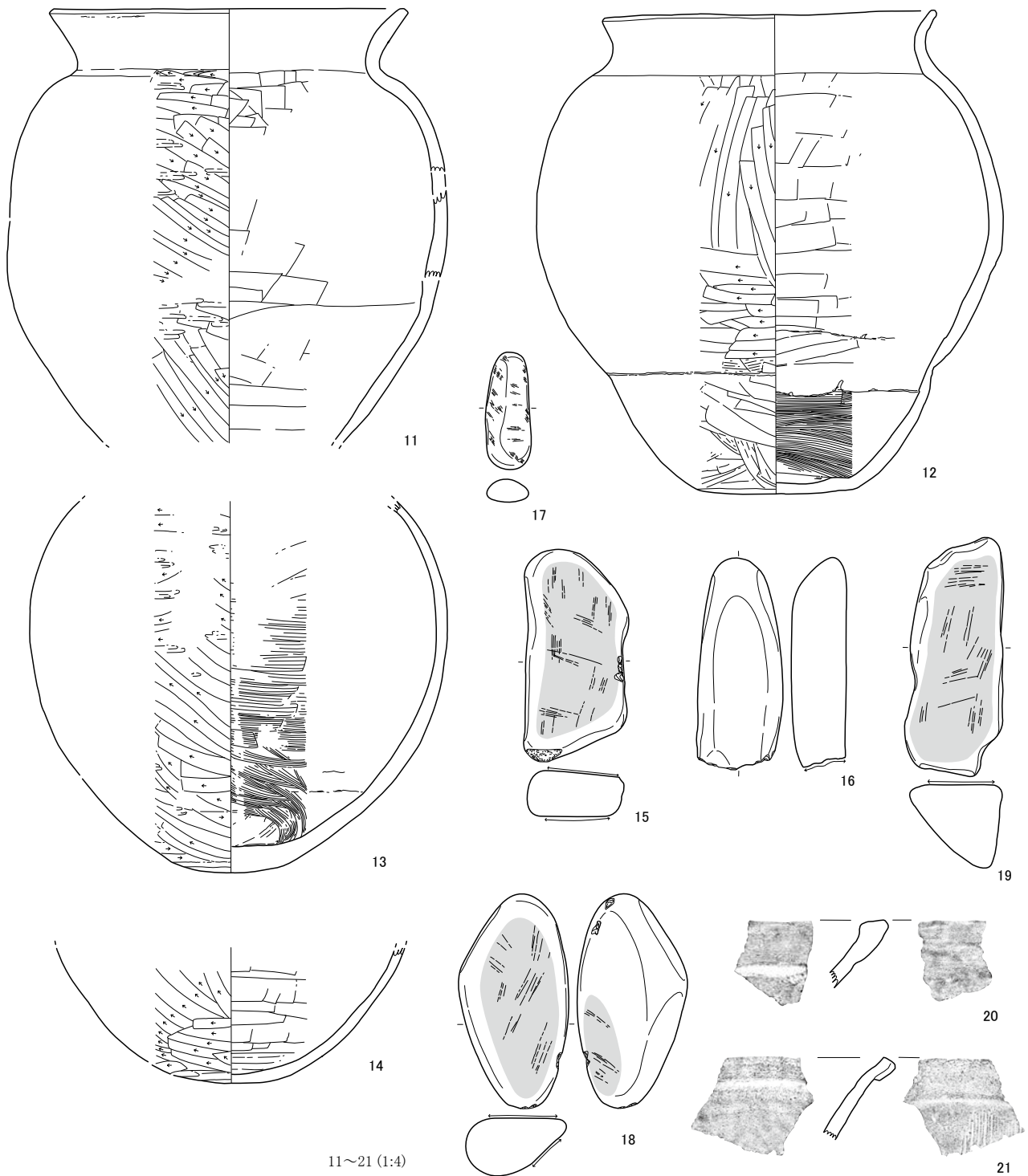
第76図 H46号住居跡出土遺物実測図(2)
