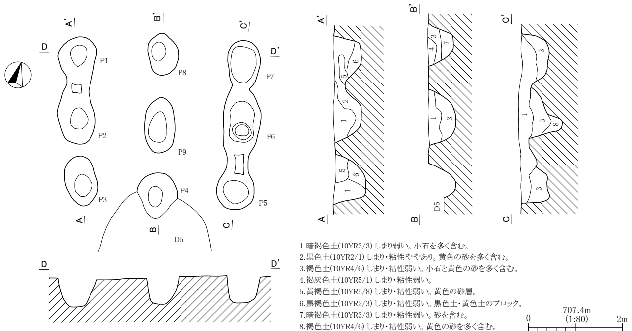
第105図 F 6号掘立柱建物跡実測図
