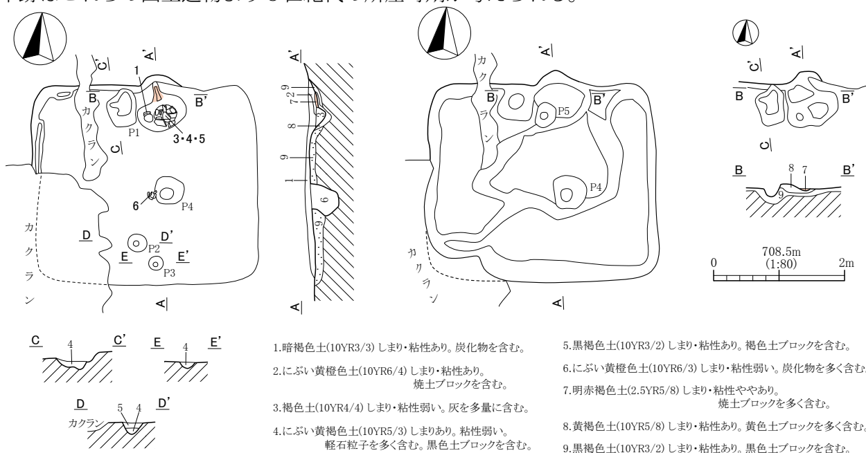
第84図 H52号住居跡実測図
