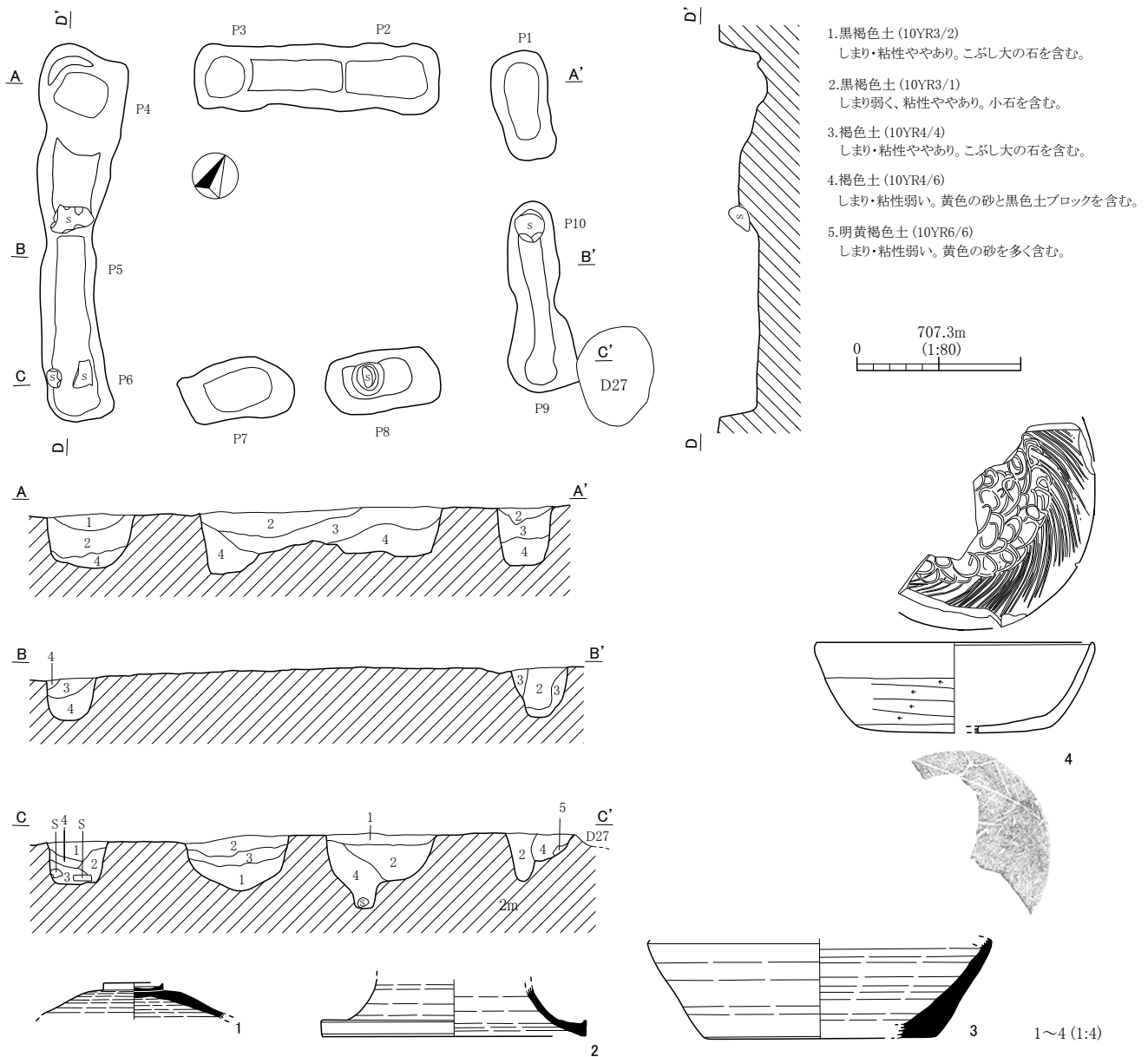
第107図 F 8号掘立柱建物跡及び出土遺物実測図
