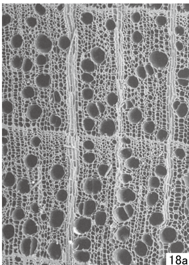
16.ヌルデ(分析No.75) 17.カエデ属(分析No.27) 18.モチノキ属(分析No.85) a:木口,b:柱目,c:板目
