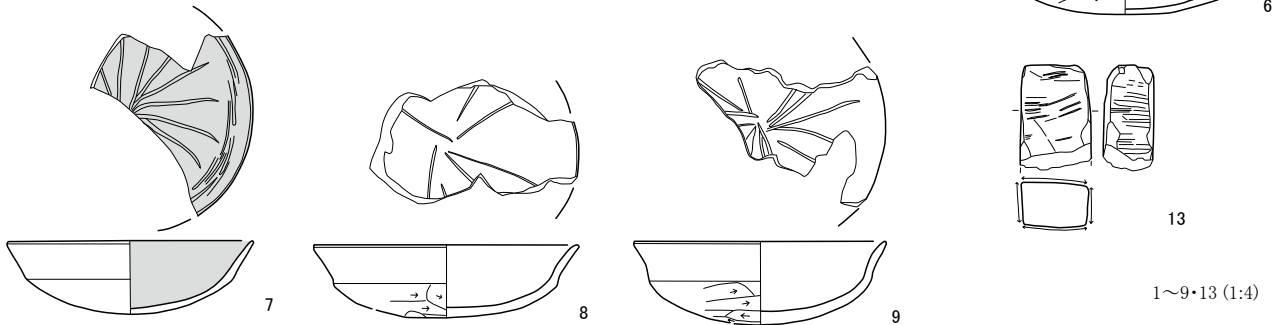
第19図 H8号住居跡及び出土遺物実測図
