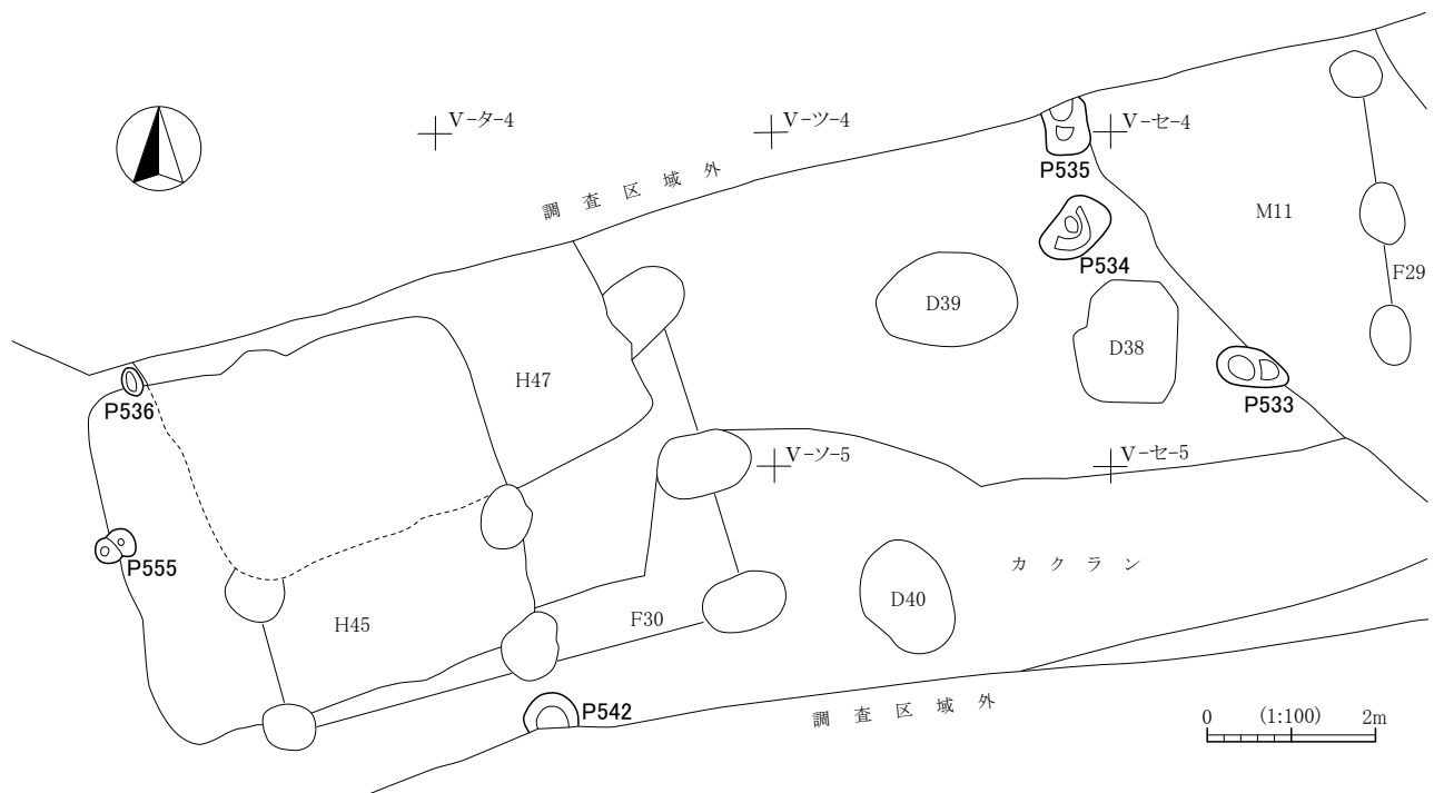
第174図 ピット平面図(13)
