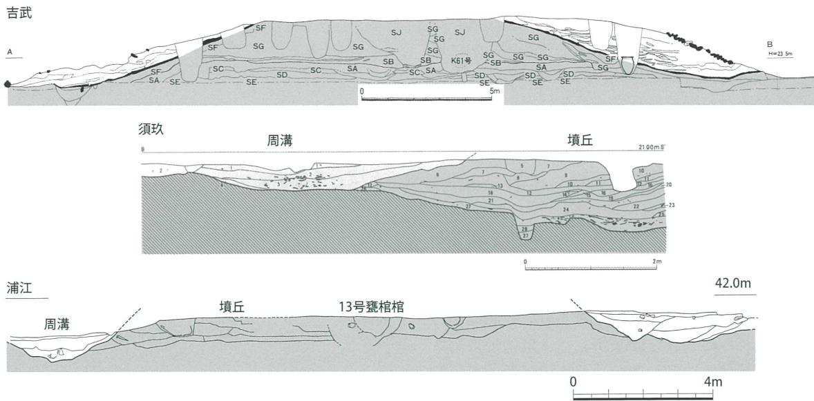
第15図 吉武樋渡墳丘墓墳丘断面図（上『吉武遺跡群Ⅷ』1998 福岡市教育委員会から転載） 須玖岡本遺跡第1次調査墳丘墓断面図（中『須玖岡本遺跡』1995 春日市教育委員会から転載） 浦江遺跡・墳丘墓断面図（下『浦江遺跡第5次調査2』2005福岡市教育委員会から作成）
