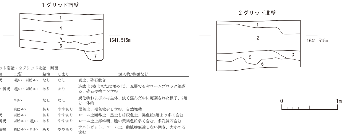
第9図 調査グリッド断面図 (S=1/40)
