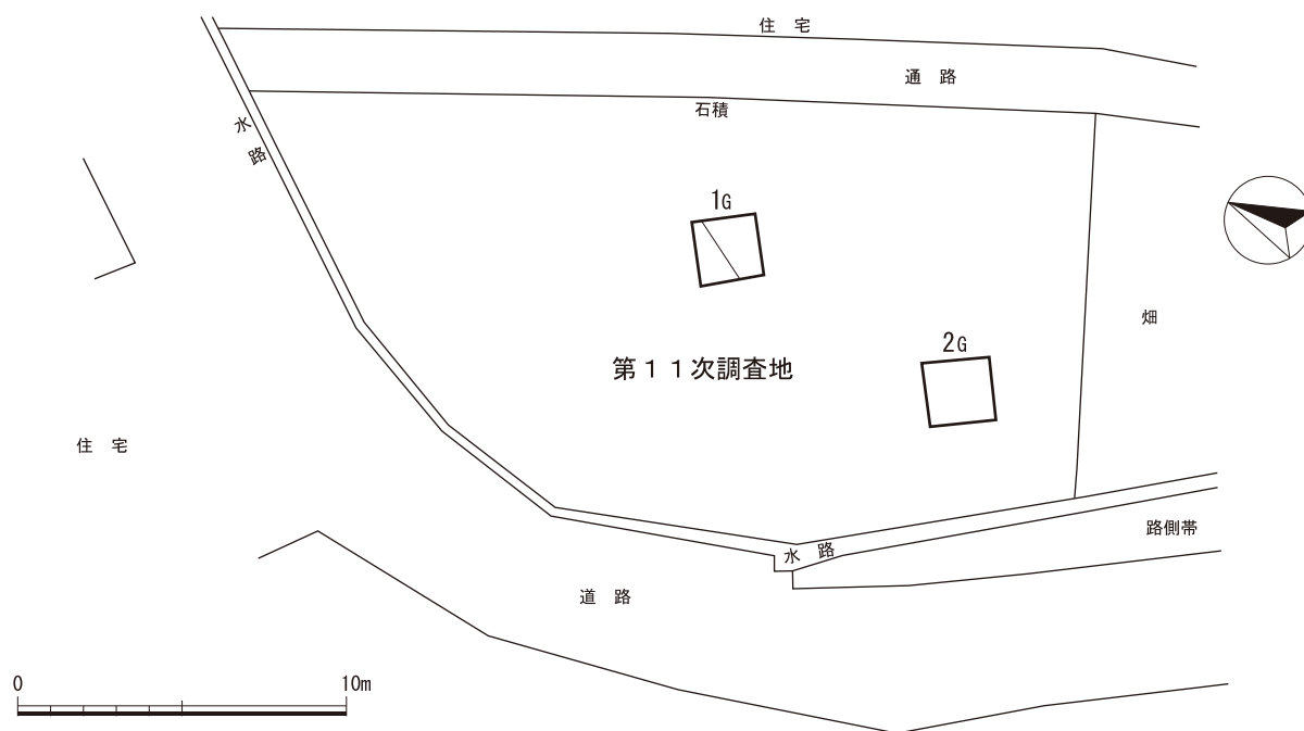
第 1 1 図 調査地全体図 (S=1/250)
