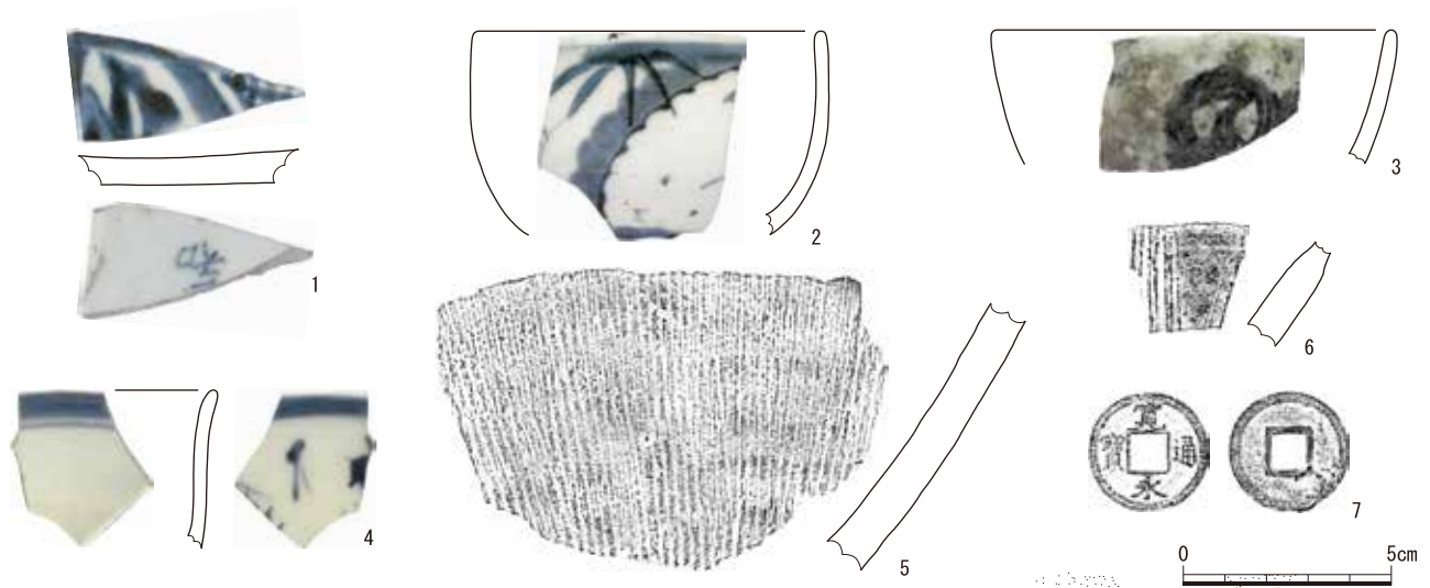
第19図 精進湯跡出土遺物 (S=1/2、7のみ1/1.5)
