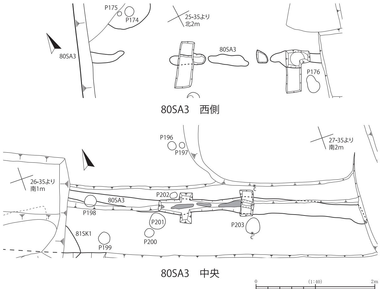
図18 80SA3 平面図 1 (1/40)
