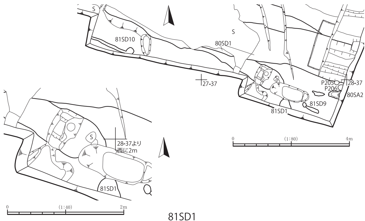
図14 81SD1 平面図
