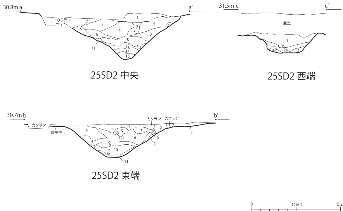
図12 80SC2 (25SD2) 断面図 (1/50)
