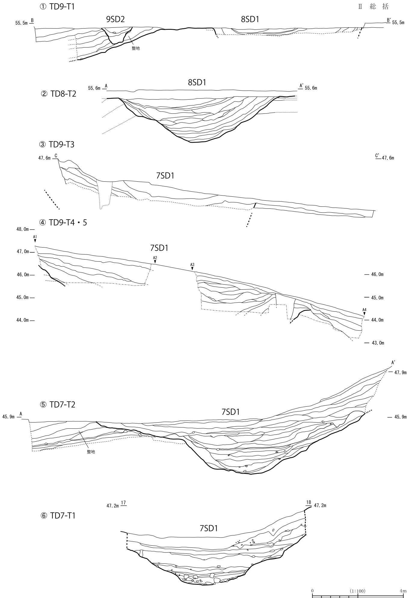
図10 堀跡の断面図 (I期)
