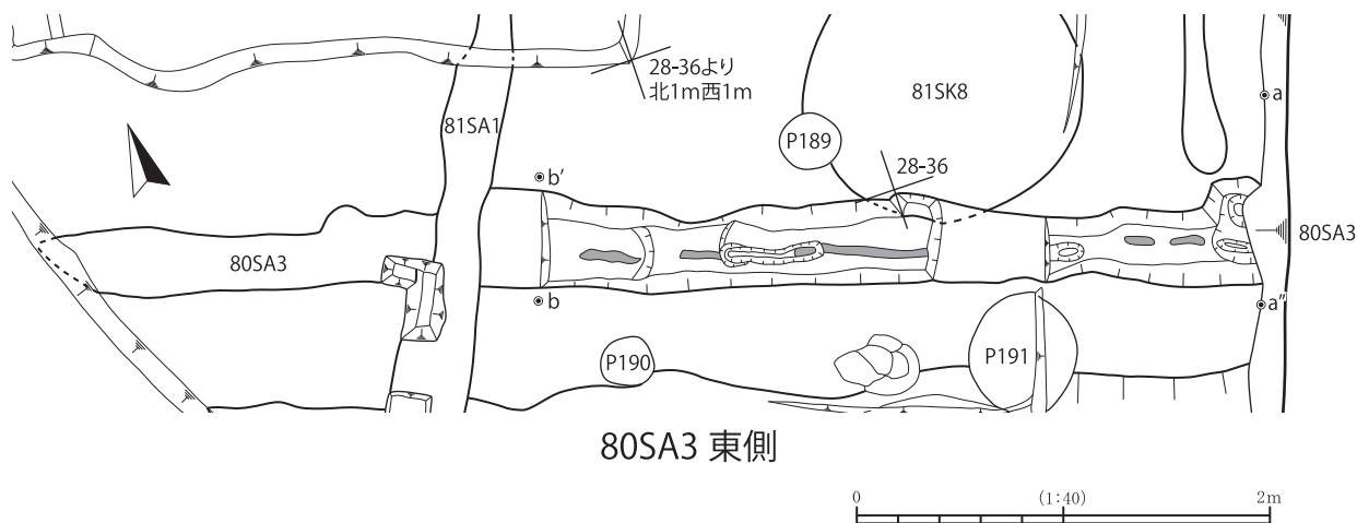
図19 80SA3 平面図2 (1/40)
