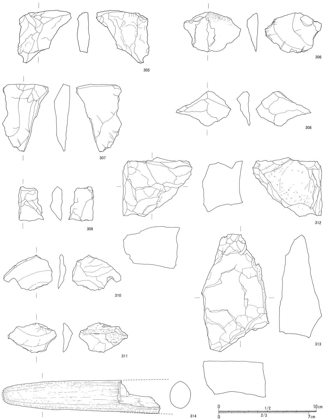
第 18 图 石器实测图 (2) (305 ~ 311:2/3、312 ~ 314:1/2)
