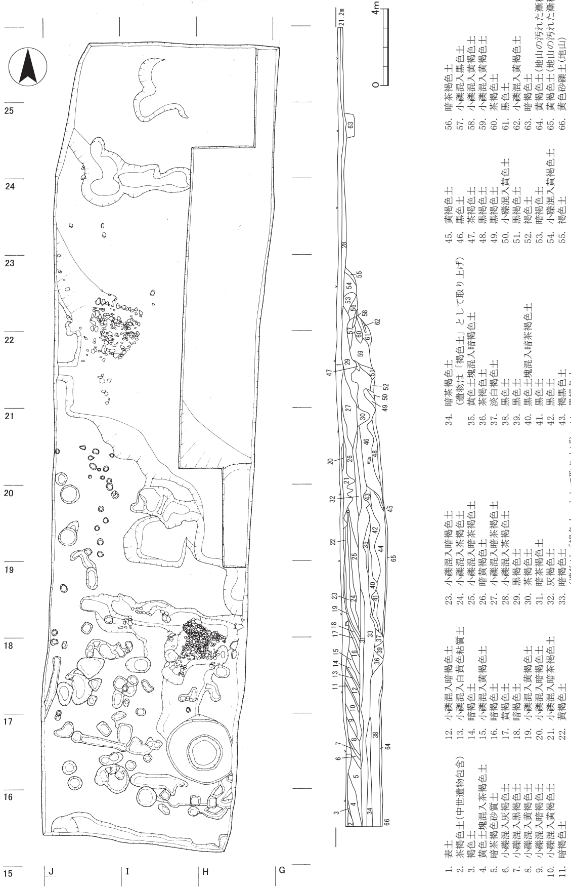
第3図 北地点平面・土層図 1/200(L=21.200m)
