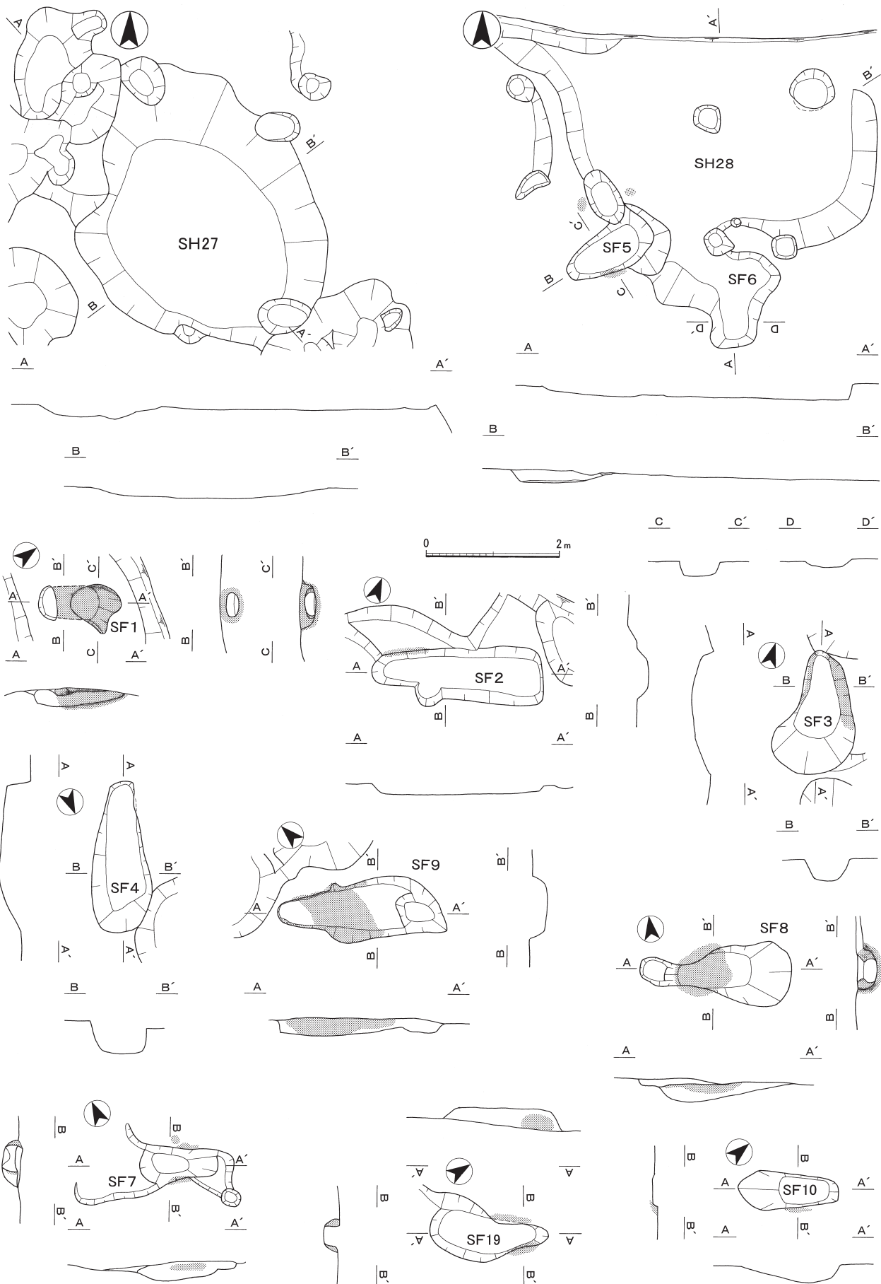
第6図 SH27・28、SF1~10・19実測図 1/80(L=23.800m)
