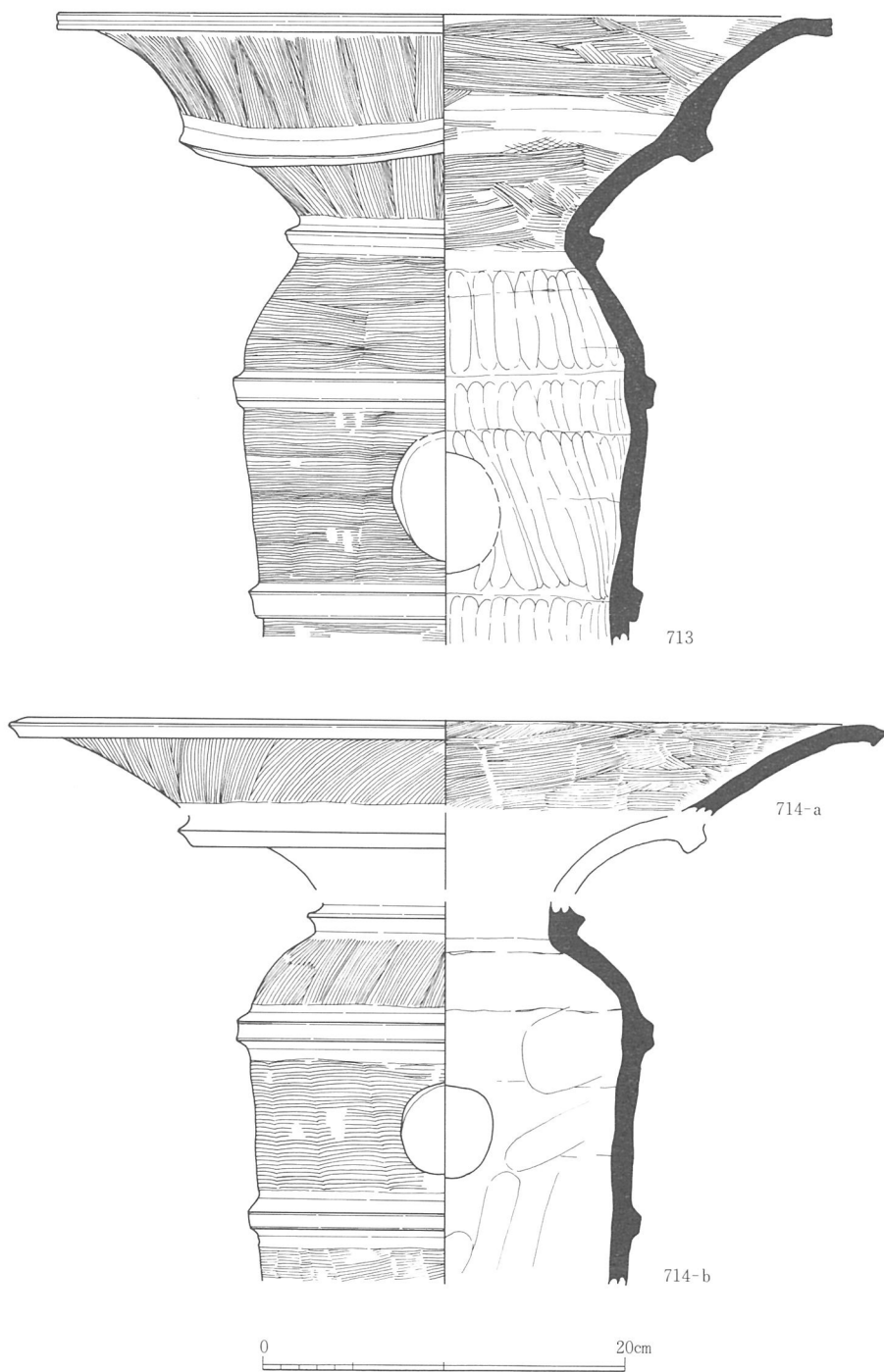
第183図 41-OG 出土埴輪 4 (1/4)
