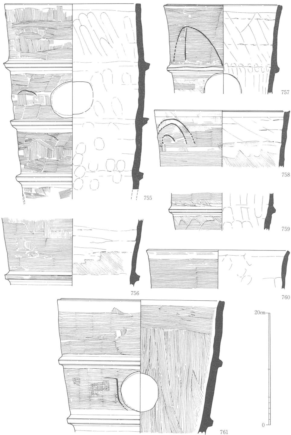
第190図 41-O G出土埴輪11(1/4)
