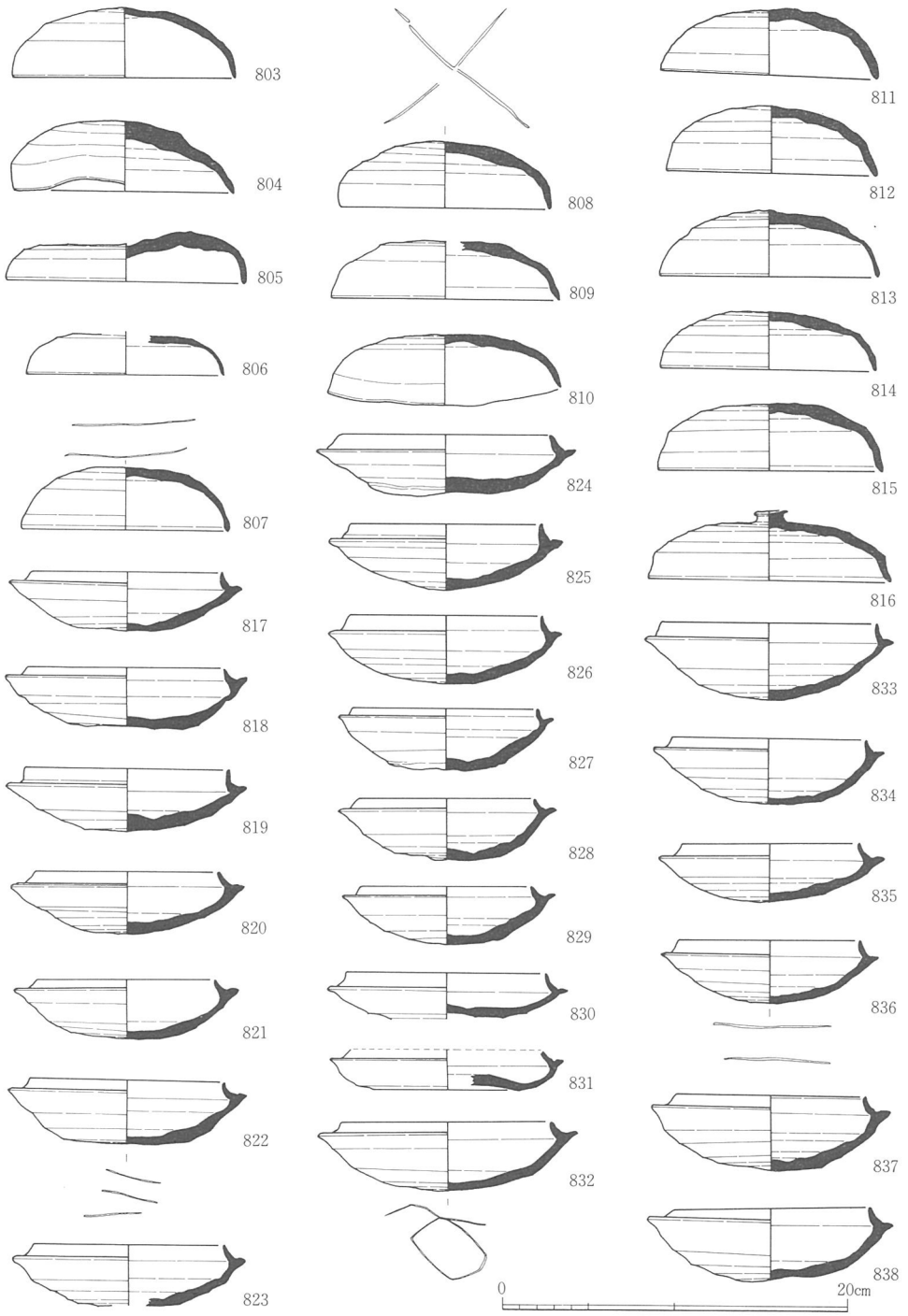
第204図 土坑群1 出土遺物1 (1/4)
