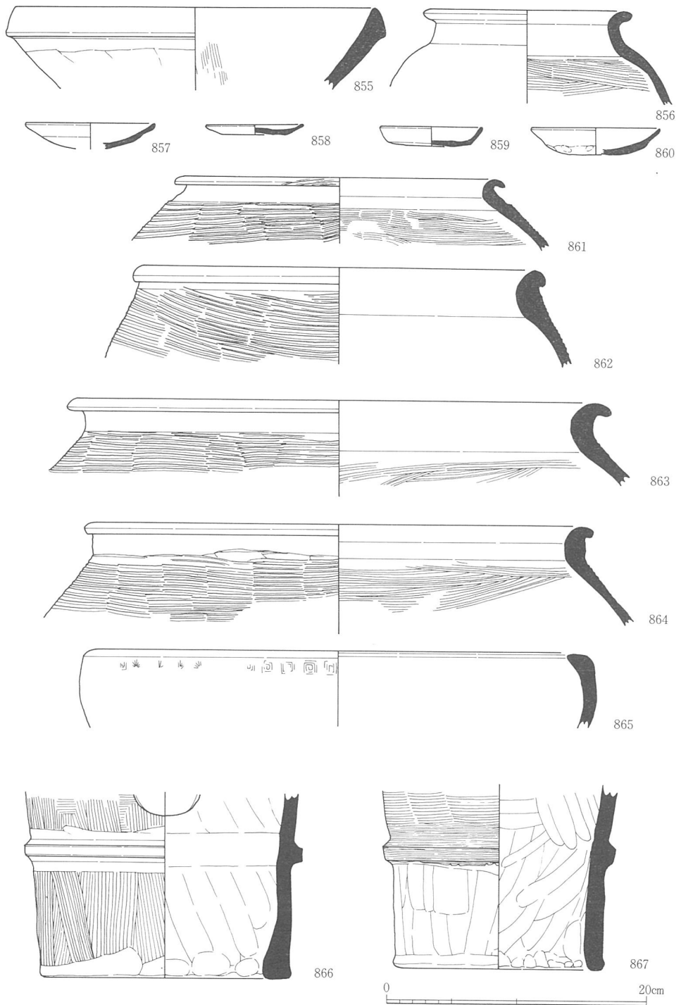
第208図 中世遺構出土遺物 1 (1/4)
