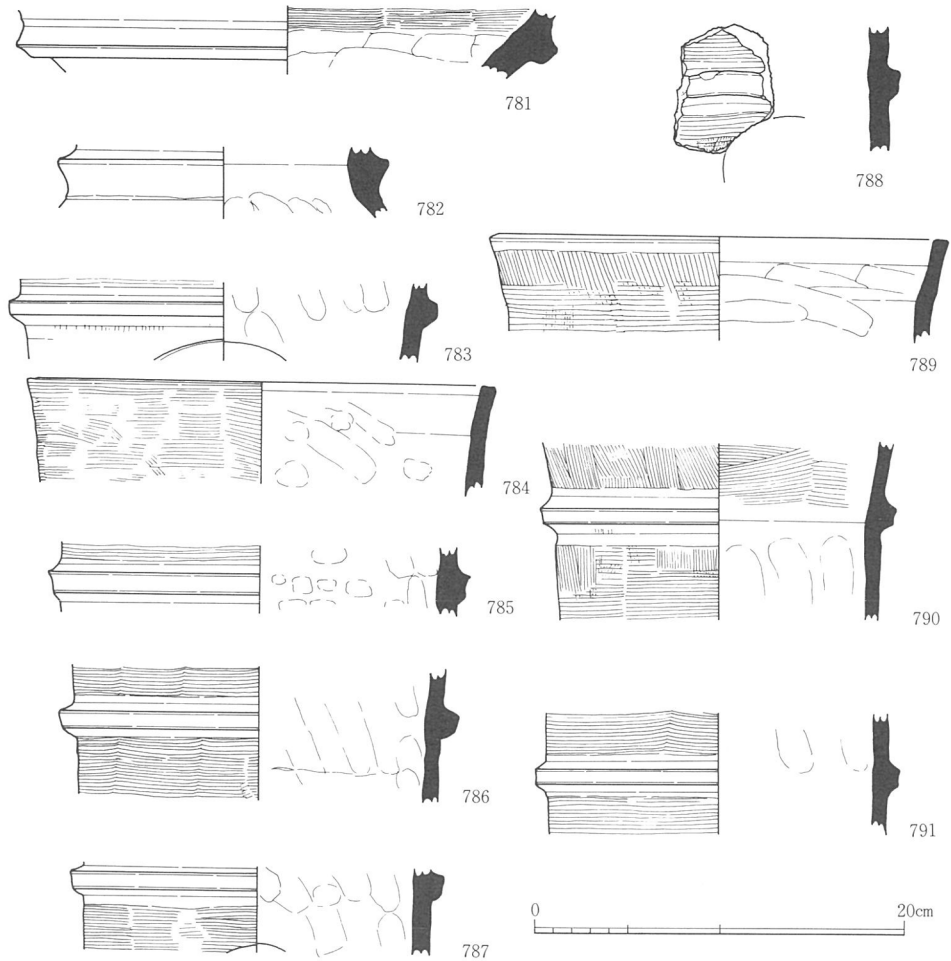
第197図 40-O G出土埴輪 (1/4)
