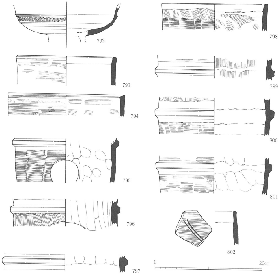
第200図 39-O G出土遺物 (1/4)
