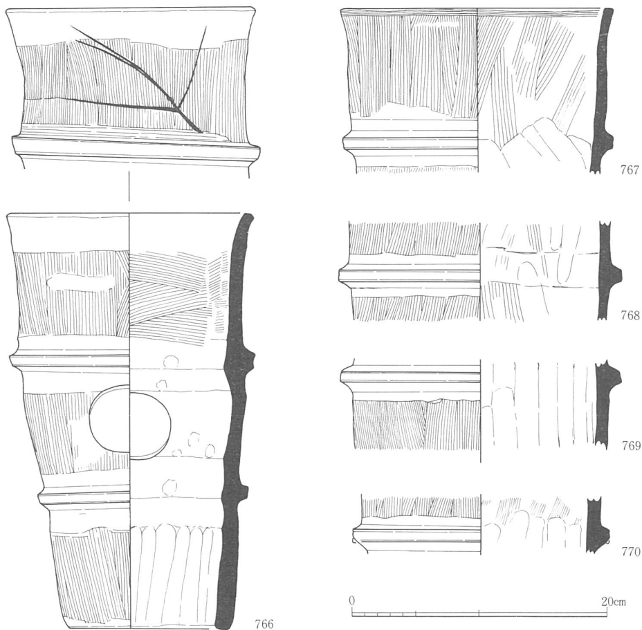
第194図 689-O G 出土埴輪 (1/4)
