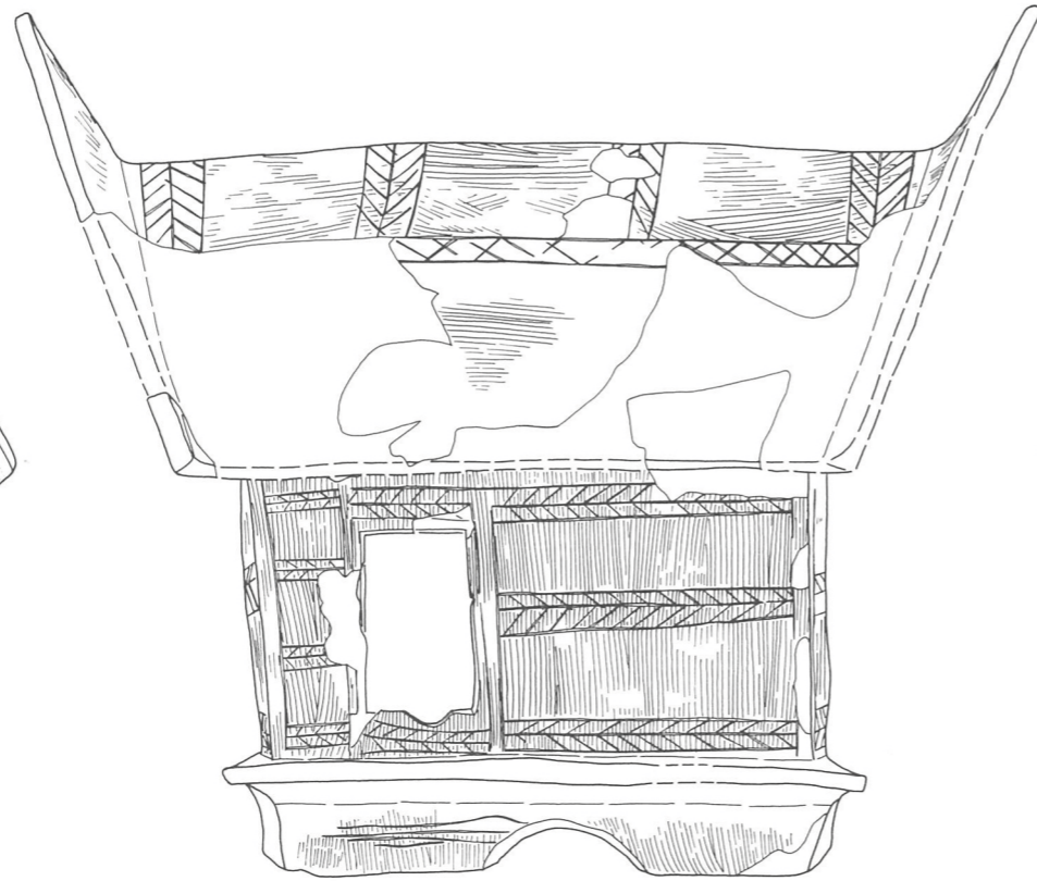
第181図 41-OG出土埴輪 2 (1/4)
