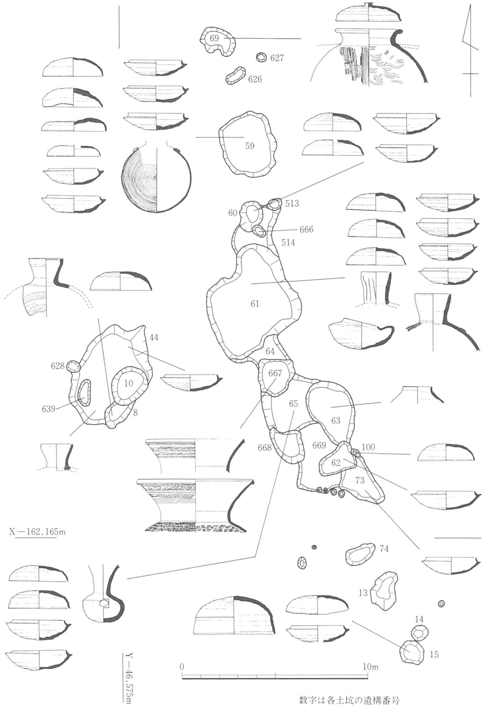
第201図 土坑群1・2平面図(1/200)
