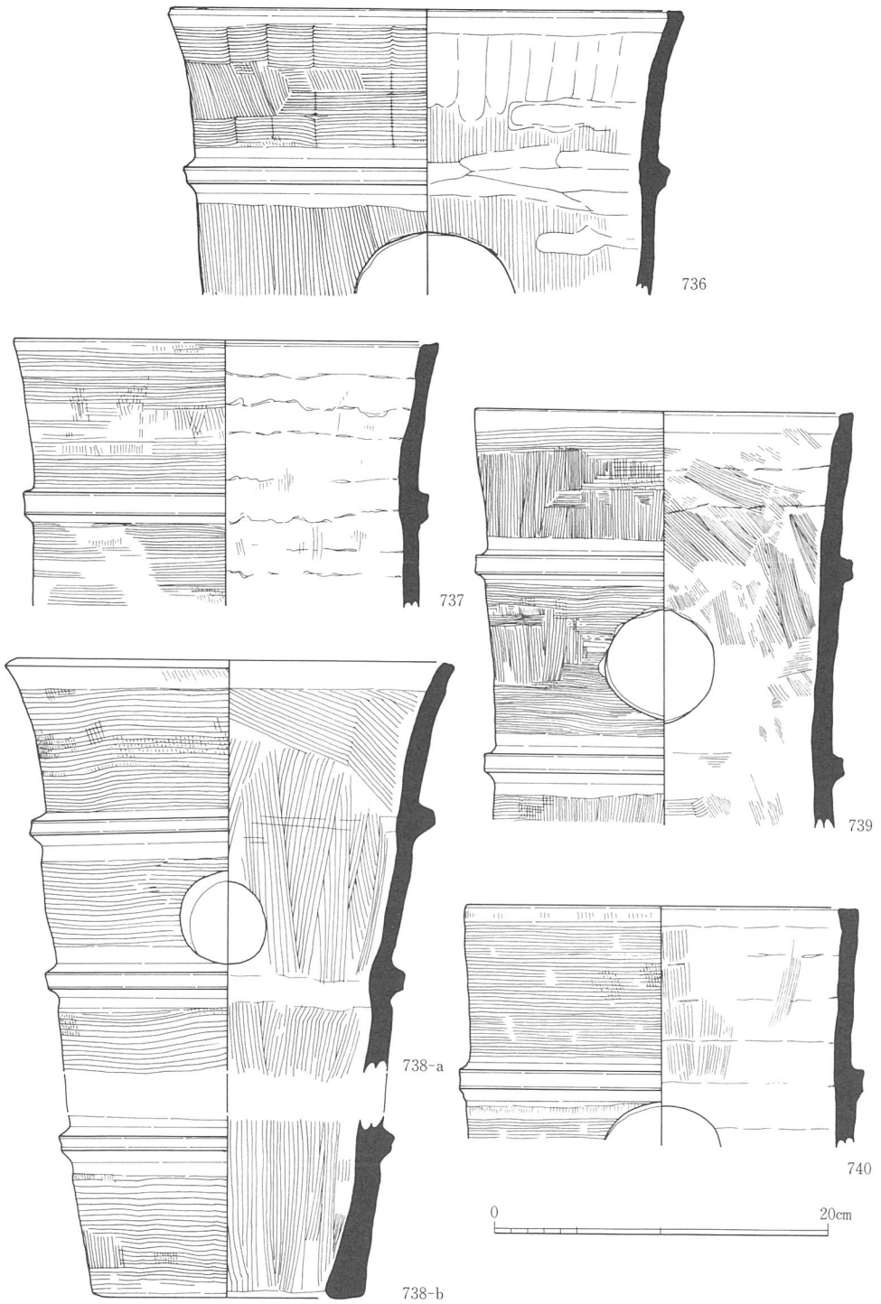
第187図 41-OG出土埴輪8 (1/4)
