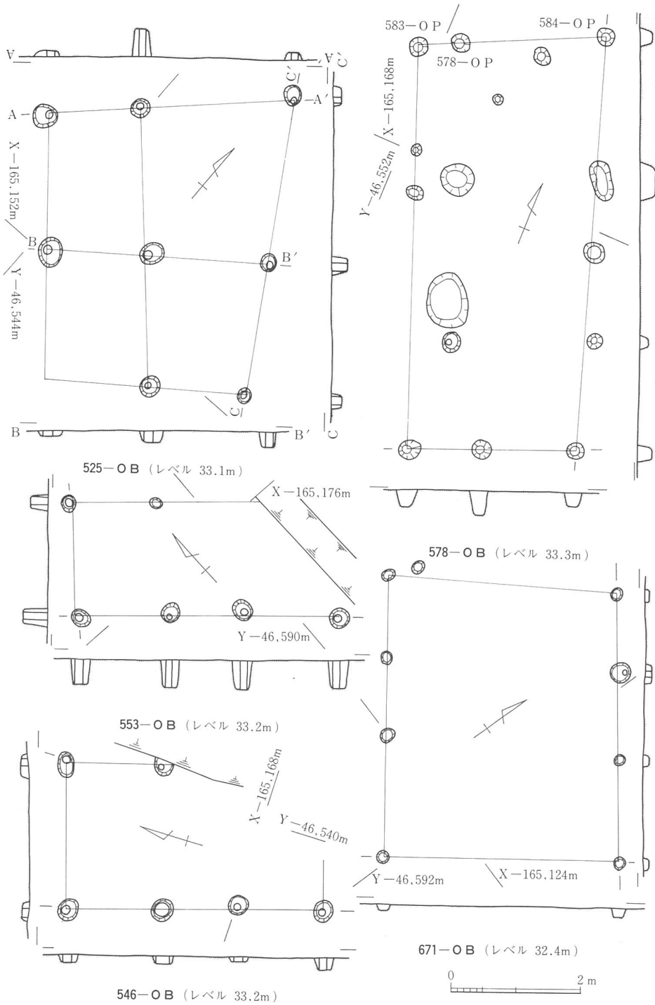
第207図 中世掘立柱建物平面・断面図 (1/80)
