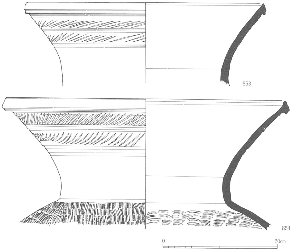
第206図 土坑群1 出土遺物2 (1/4)
