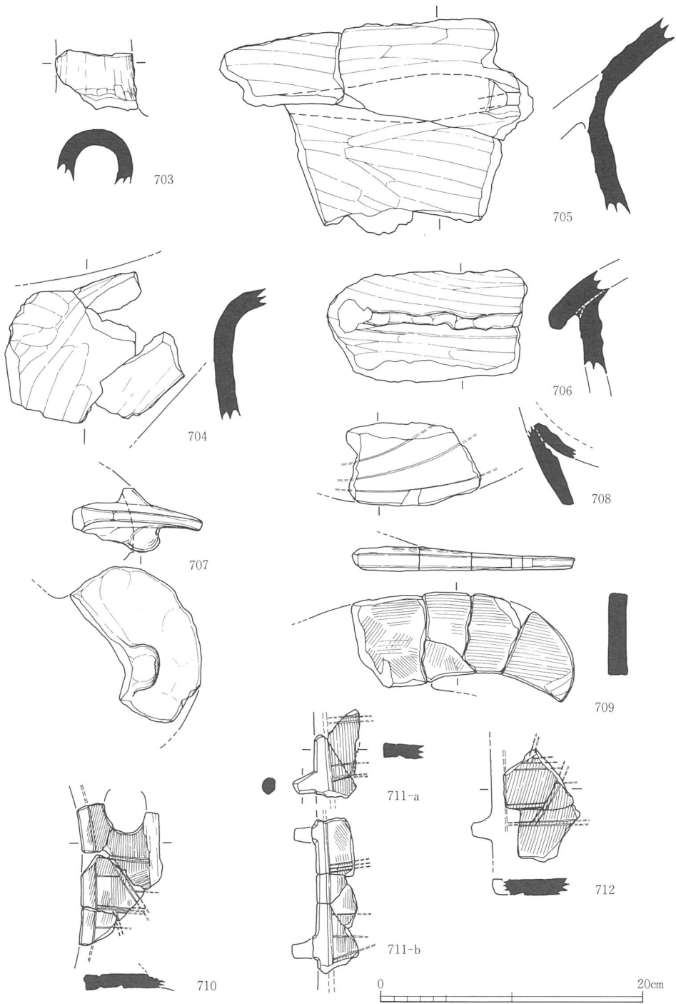
第182図 41-O G 出土埴輪 3 (1/4)
