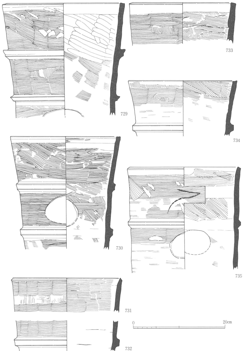
第186図 41-O G 出土埴輪 7 (1/4)
