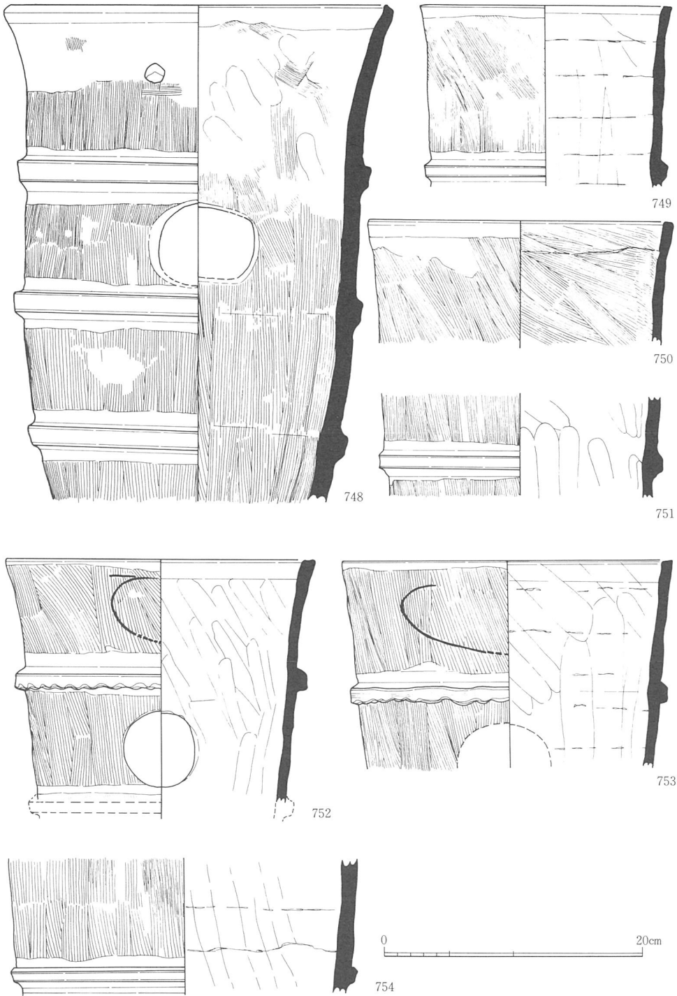
第189図 41-O G 出土埴輪10 (1/4)
