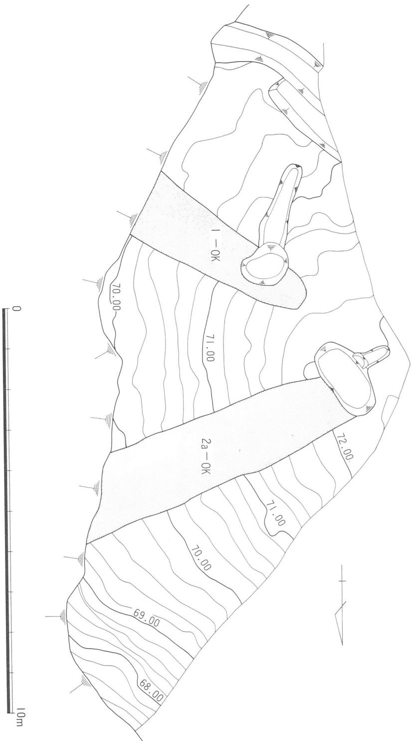
図版十七 遺跡B地区 信太山1・2号(新) 窯地形測量図
