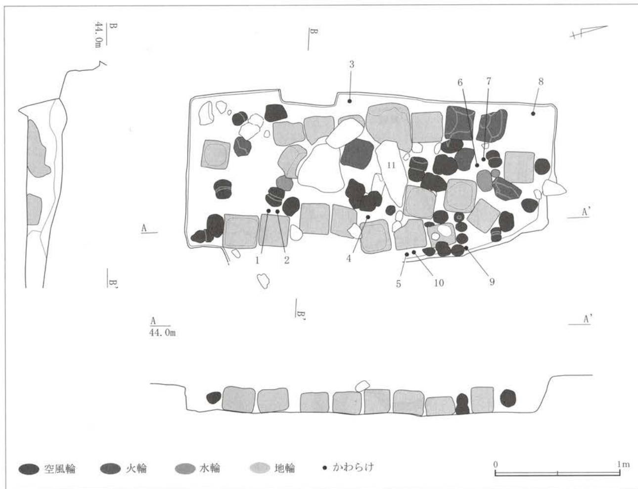
第7図 1号やぐら方形土坑 (S-1/30)
