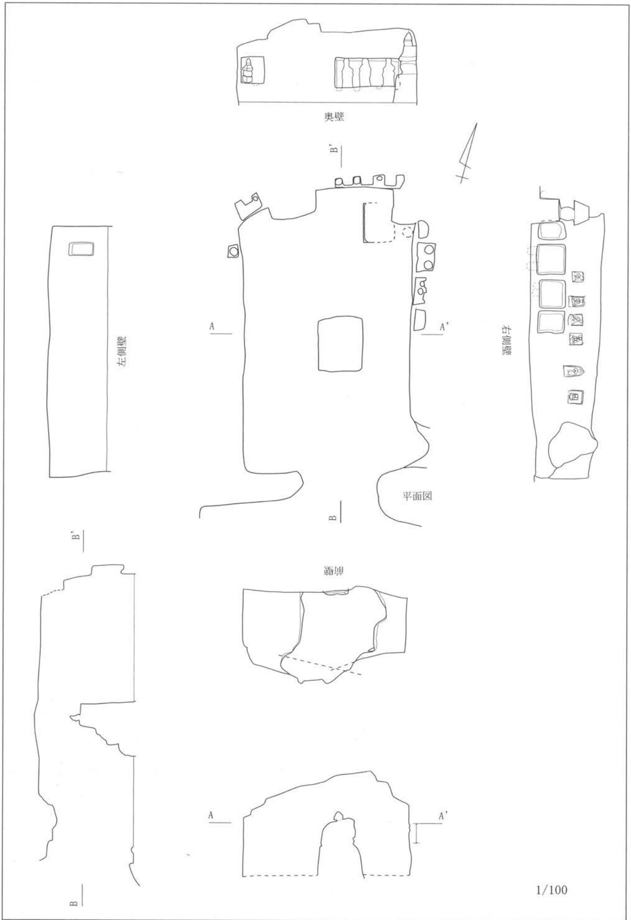
第18図 D地区 1号やぐら (S=1/100)
