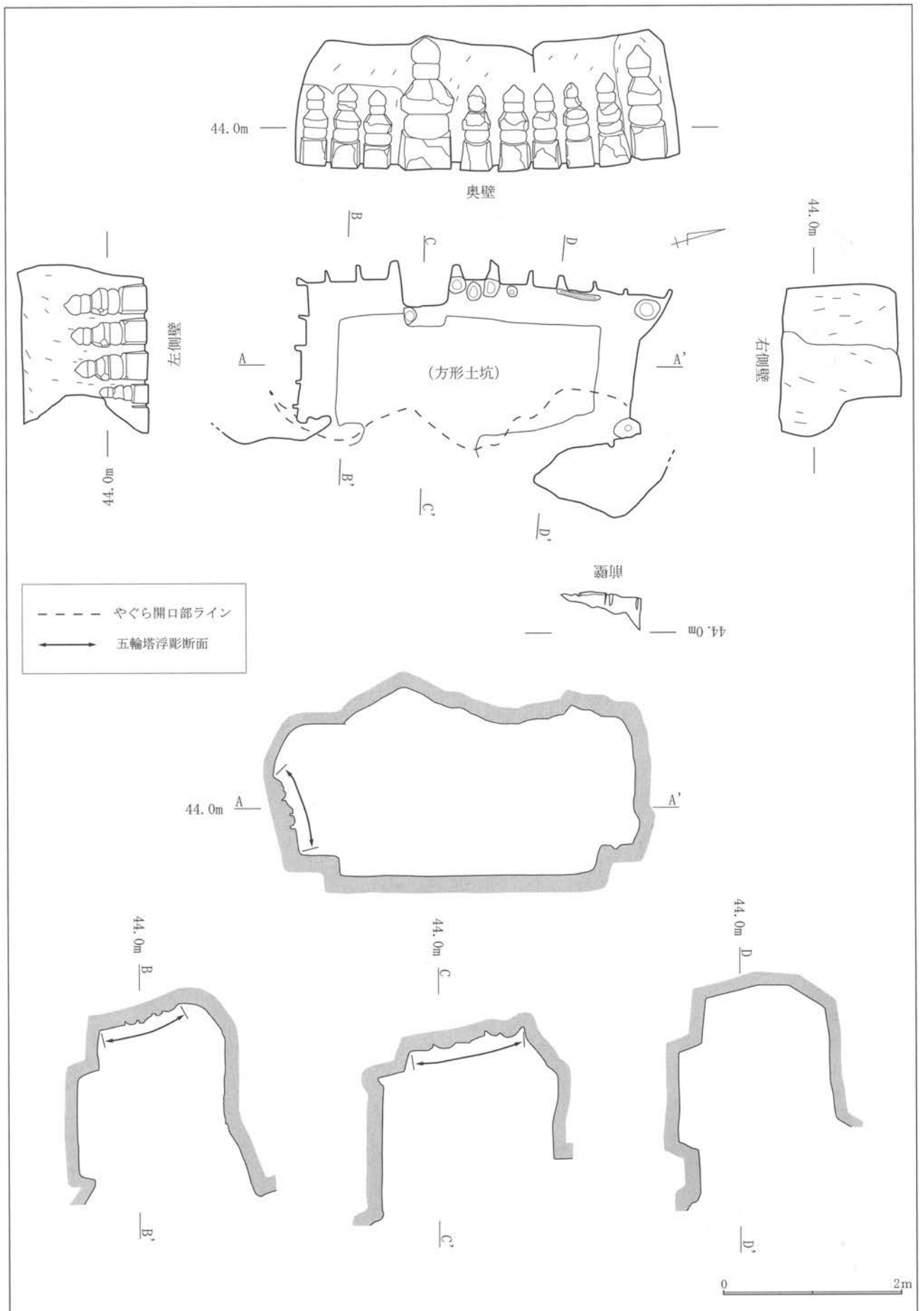
第6図 1号やぐら (S=1/60)
