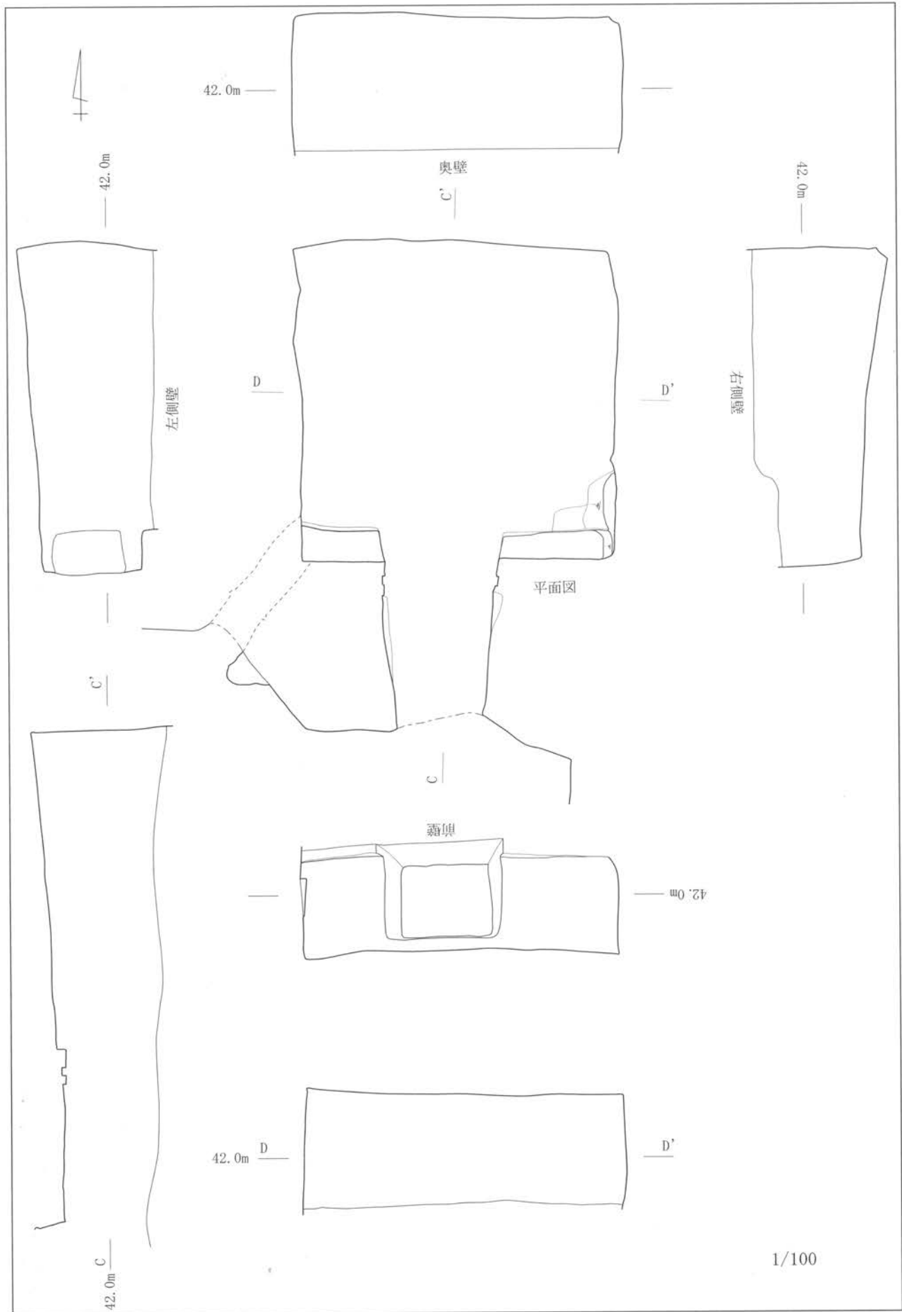
第17図 A地区 2号やぐら (S=1/100)
