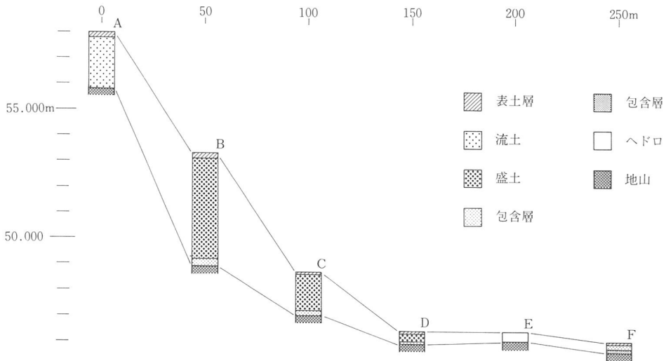
Fig. 9 基本層序模式図
