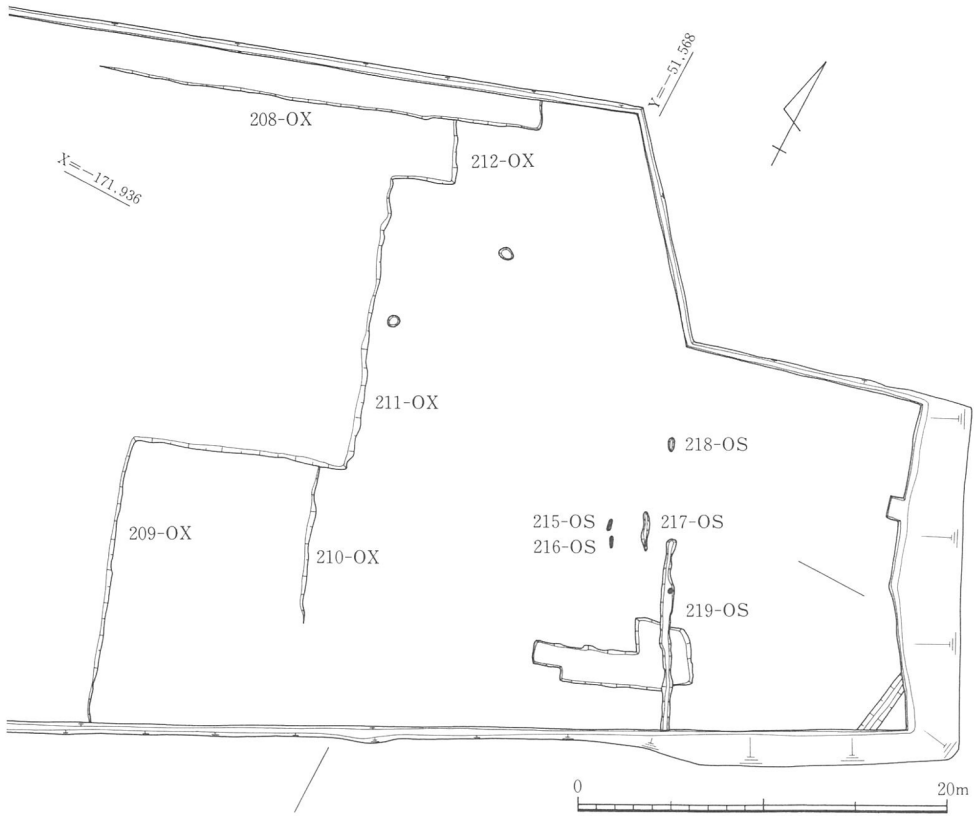
Fig. 24 IV区遺構配置図
