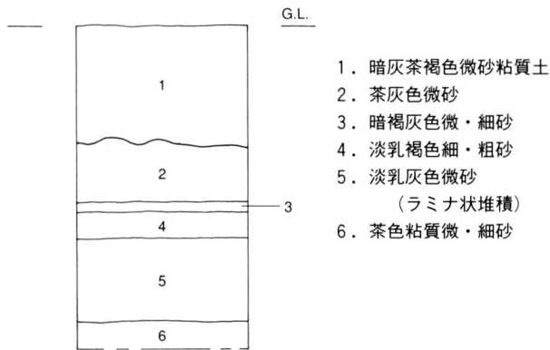
第32図 土層柱状図 (S=1/40)
