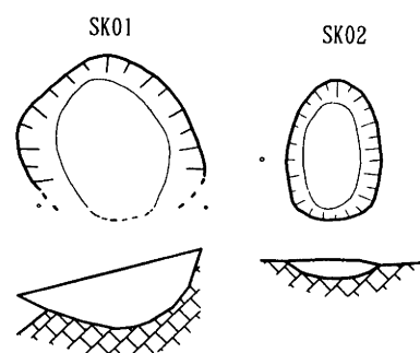
第19図 遺構平・断面図 (S=1/50)
