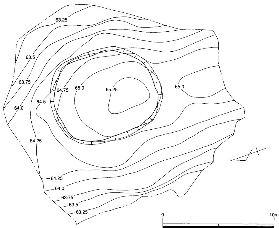
第48図 墳丘平面図 (S=1/200)
