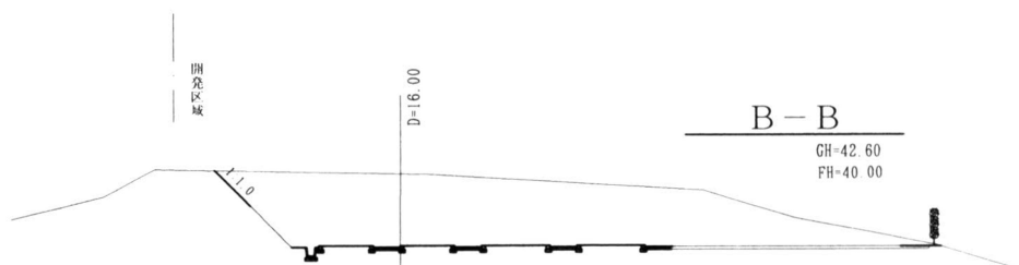
第20図 計画地横断面図（B-B，S=1/300）
