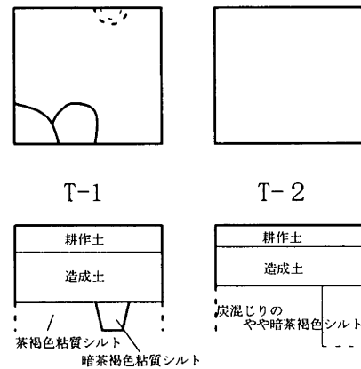
第30図 土層模式図 (S=1/50)
