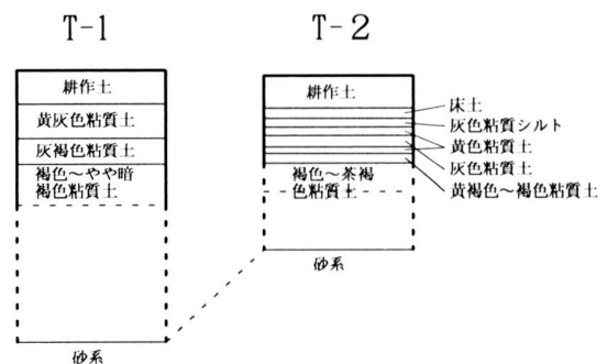
第7図 土層模式図 (S=1/50)
