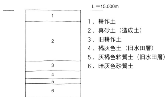
第26図 土層柱状図 (S=1/40)
