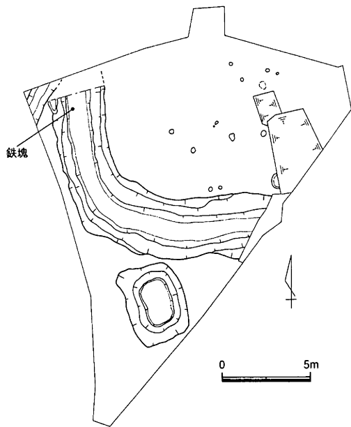
第35図 鷹尾手遺跡4区遺構配置図 (S=1/300) 第36図 鷹尾手遺跡溝-2断面図 (S=1/50)
