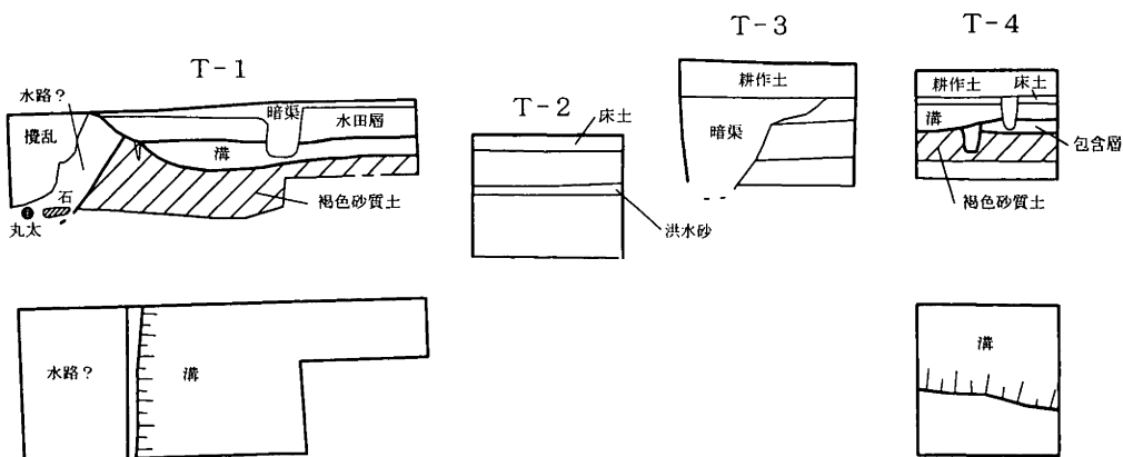
第9図 調査地平・断面図 (S=1/50)
