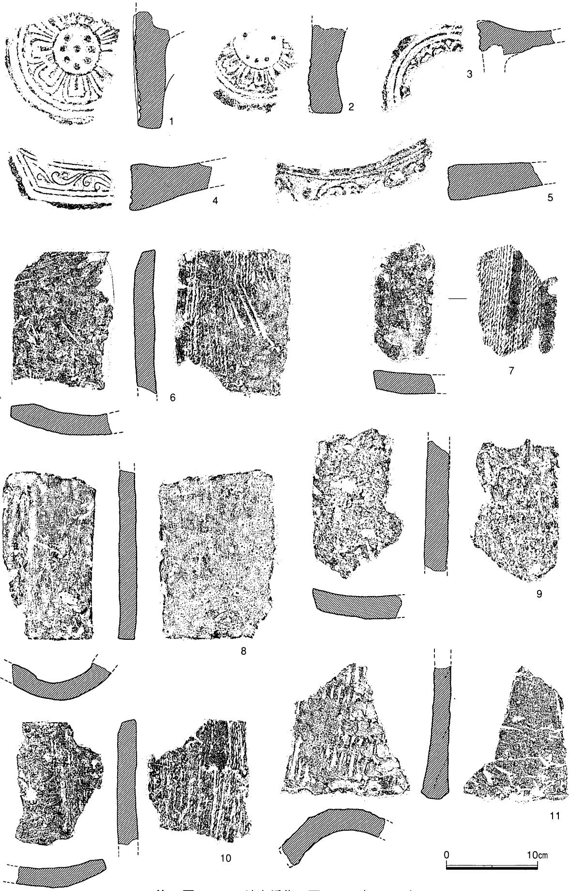
第40図 A・A'地点採集の瓦<1> (S=1/4)
