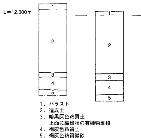
第29図 T-2・T3土層断面柱状図 (S=1/40)
