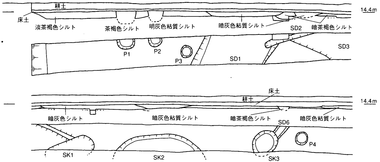
第5図 遺構平・断面図 (S=1/80)
