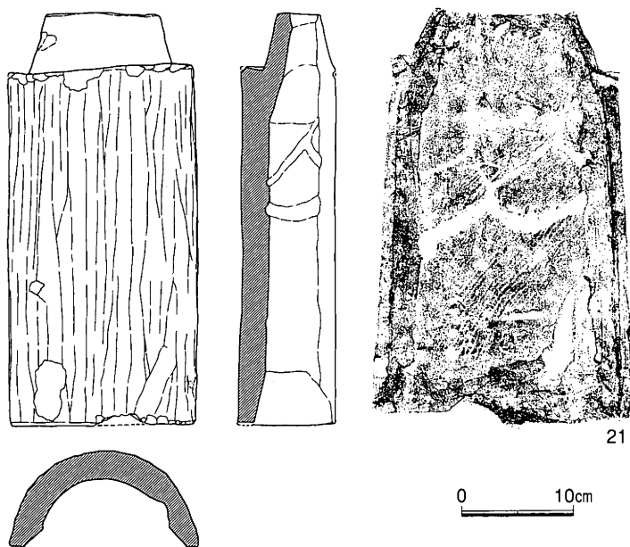
第43図 A・A'地点採集の瓦<4> (S=1/6)
