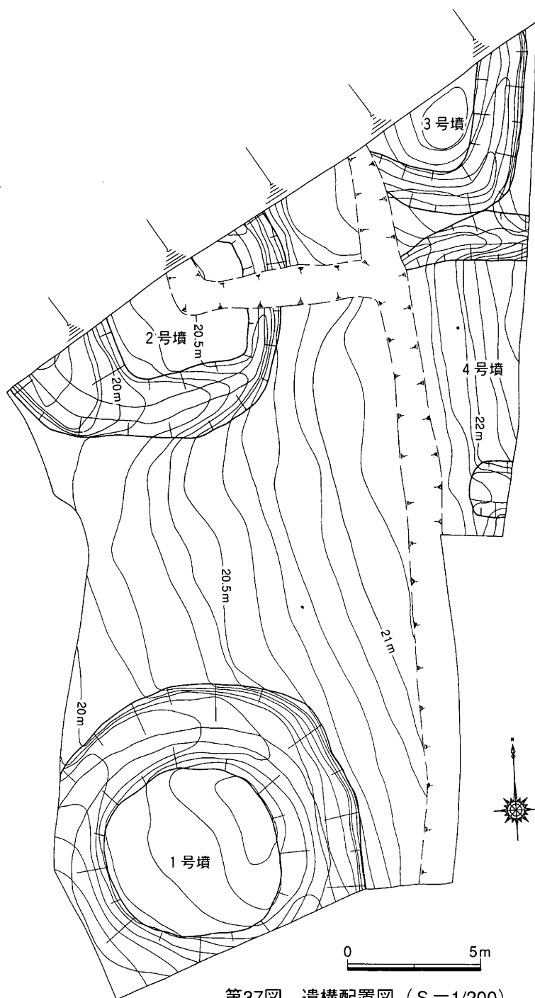
第37図 遺構配置図 (S=1/200)
