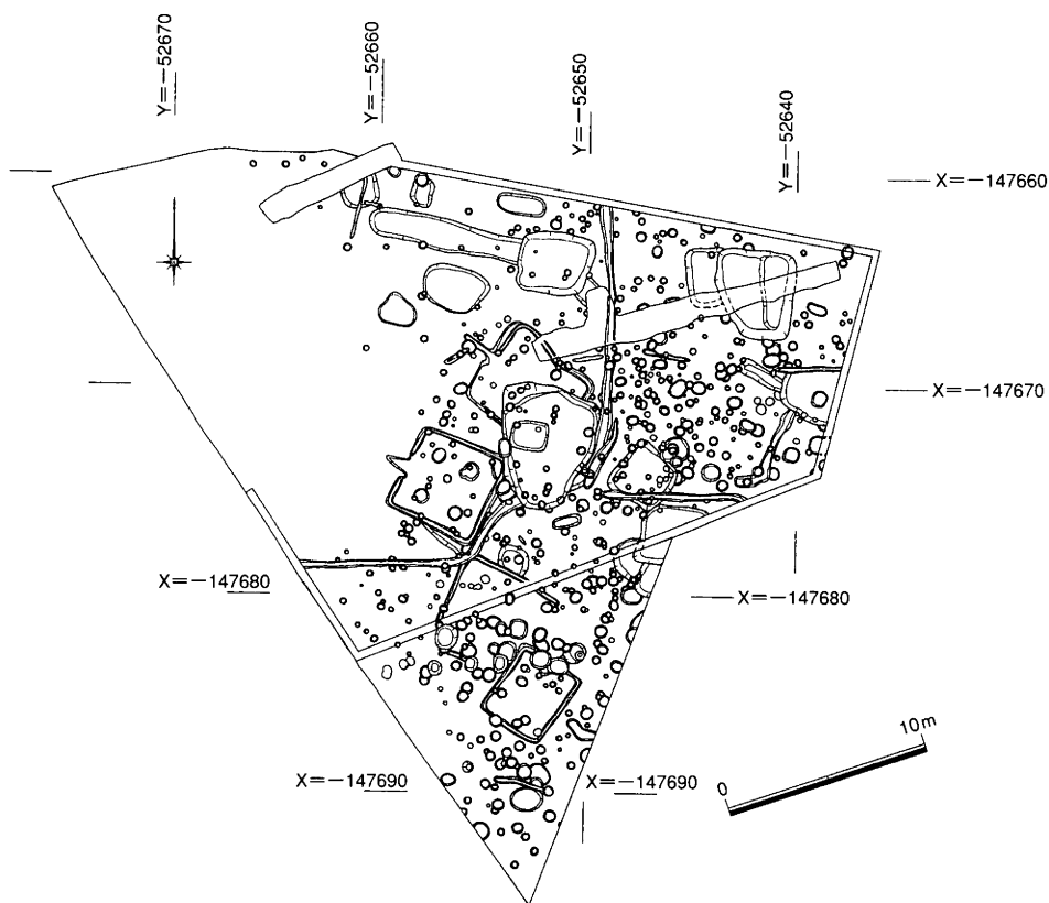
第30図 真壁遺跡出之向地区遺構配置図 (S=1/400)
