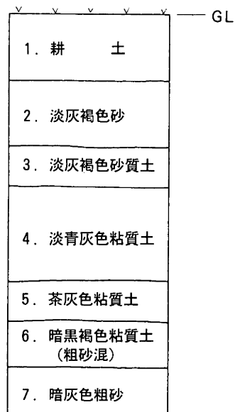
第7図 T-1南壁土層図 (S=1/20)
