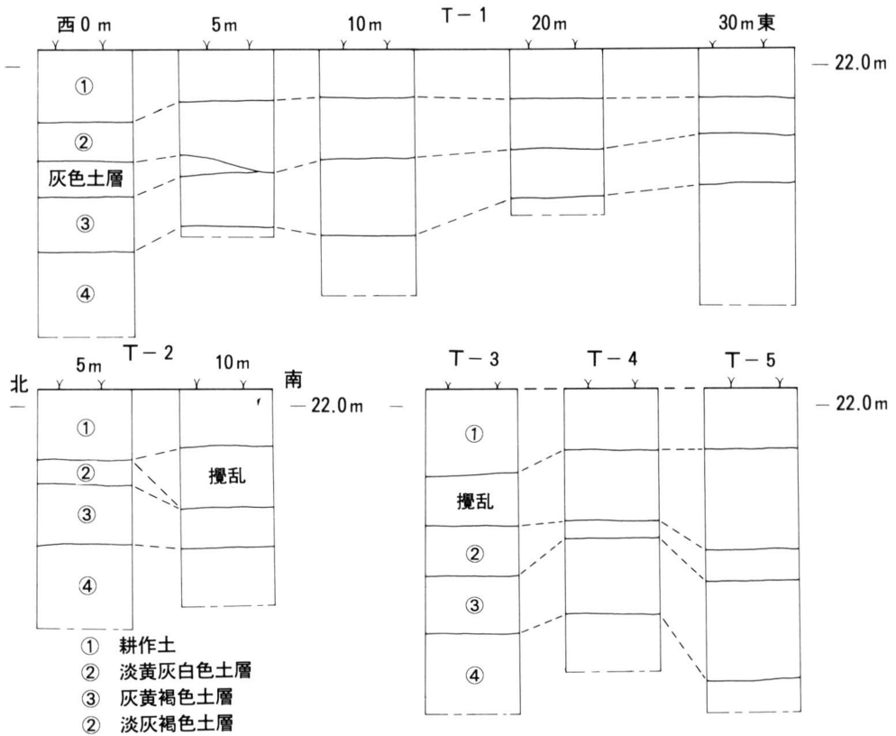
第20図 土層柱状図 (S=1/40)
