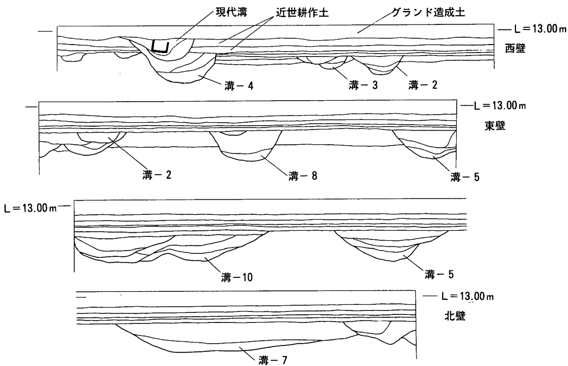
第34図 調査区土層図 (S=1/100)
