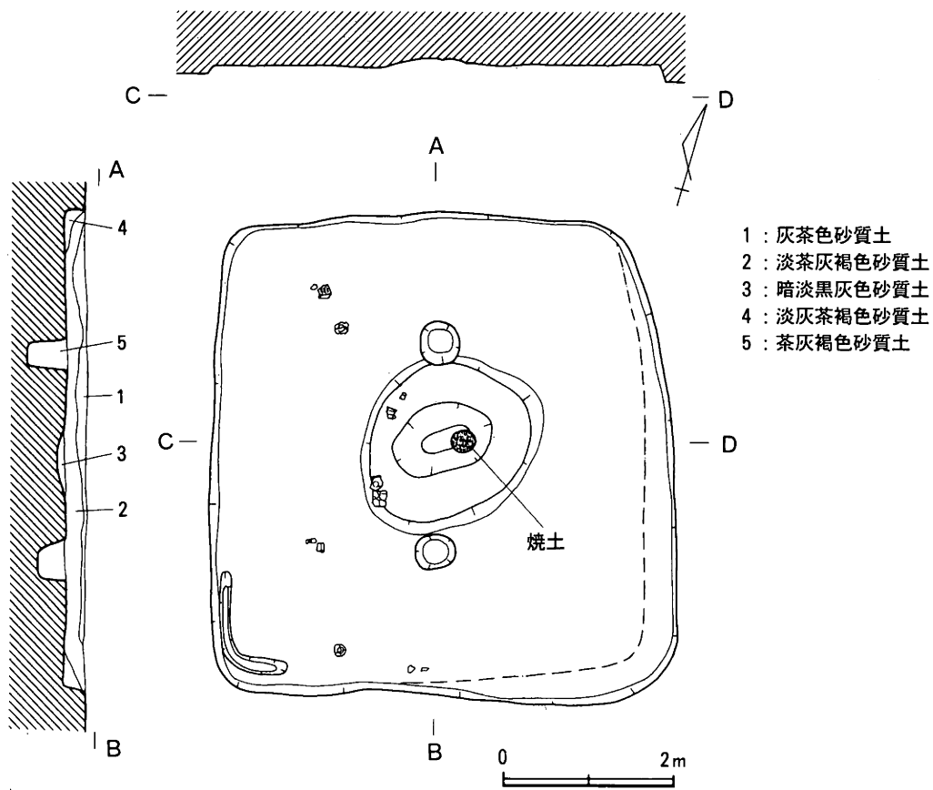
第46图 H-2 平·断面图 (S=1/80)
